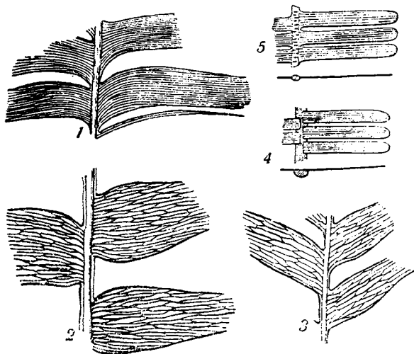
Рис. 25. 1 — Ctenis sp. 2 — Ctenis burejensis Pryn., схема. 3 — Ctenis Yokoyamai Krysh. et Pryn. 4 — Dioonites sp. 5 — Pterophyllum braunianum Гоерр.
