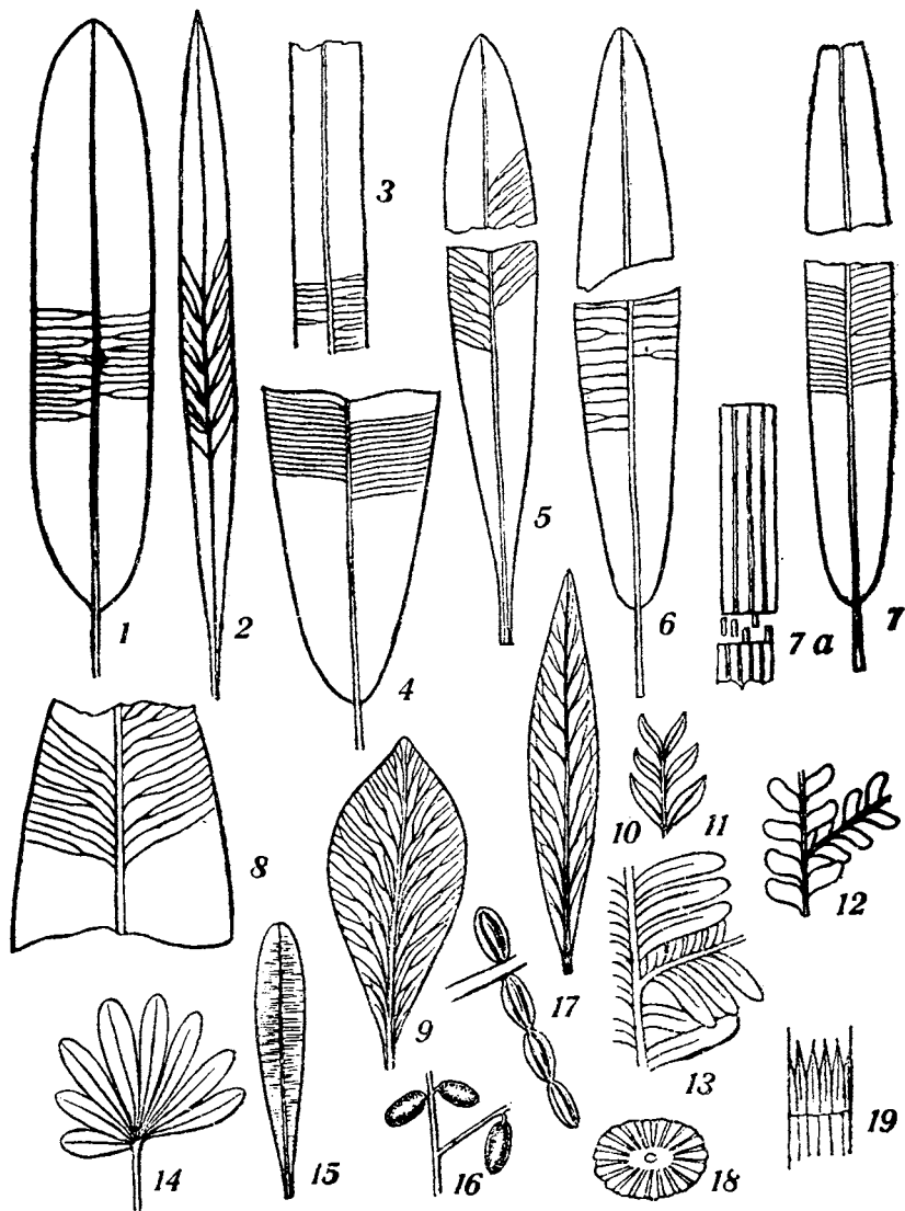
Рис. 18. 1— Taeniopteris vittata Brongn. 2— T. stenophylla Krysh. 3— T. spatulata McClell. 4— T. jimboana Krysh. 5— T. ensis Oldh. 6— T. amurensis Novopokr. 7, 7a— T. rhtidorhachis Krysh. 8— Macrotaeniopteris Richtofenii Schenk. 9— Sagenopteris goeppertiana Zigno. 10— Sagenopteris Phillipsii (Brongn.). 11— Lycopodites tenerrimus Hr. 12— L. ussuriensis Krysh. et Pryn. 13— L. Nosikovii Krysh. et Pryn. 14—15. Annulariopsis inopinata Zeill. 16— Equisetites Yokoyamai Sew. 17— Equisetites burejensis Hr. 18— E. ferganensis Sew., диафрагма. 19— E. columnaris Brongn., листовое влагалище.
