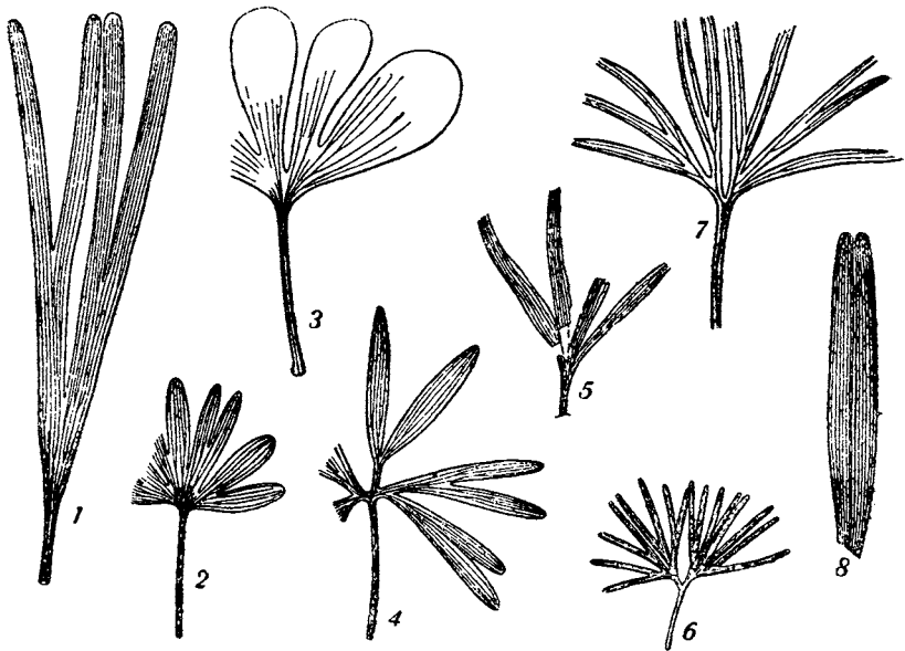
Рис. 35. 1— Baiera longifolia Ром. 2— Ginkgo sibirica Нр. 3— Ginkgo Huttonii (Sternb.) Нр. 4— Ginkgo lepida Нр. 5— Baiera Phillipsii Nath. — Ginkgo concinna Нр. 7— Baiera gracilis Bunb. 8— Baiera pulchella Нр.
