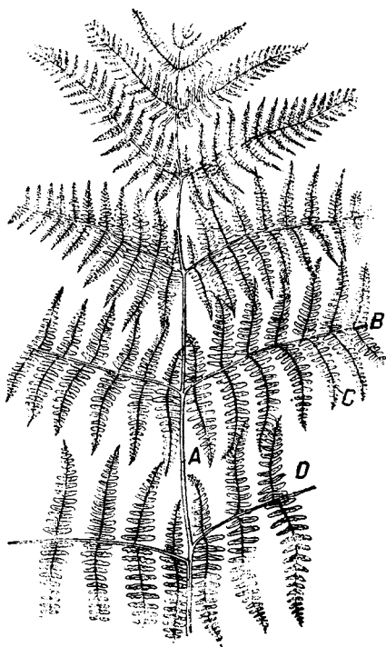
Рис. 1. Pteridium aquilinum . Современный папоротник пекоптероидного типа. Показан характер ветвления вайи. A — главный рахис, B — перо первого порядка, C — перо 2-го порядка, D — сегмент.
