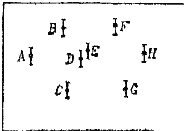
Рис. 5. Фотография, полученная с помощью искровой камеры. Взаимодействие в точке А даёт три следа: ABF , ACG , ADEH . Проведите треки. Раскрасьте их, как вам нравится, и проинтерпретируйте.
