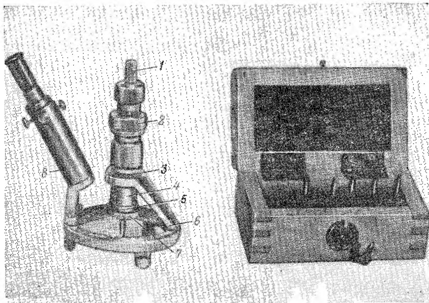
Рис. 78. Ручной кронциркуль (КР)
