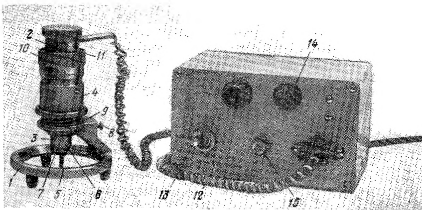
Рис. 76. Усовершенствованный электрический кронциркуль (ЭК-1)
