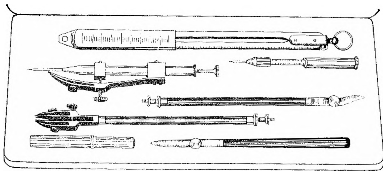
Рис. 10. Готовальня топографическая
