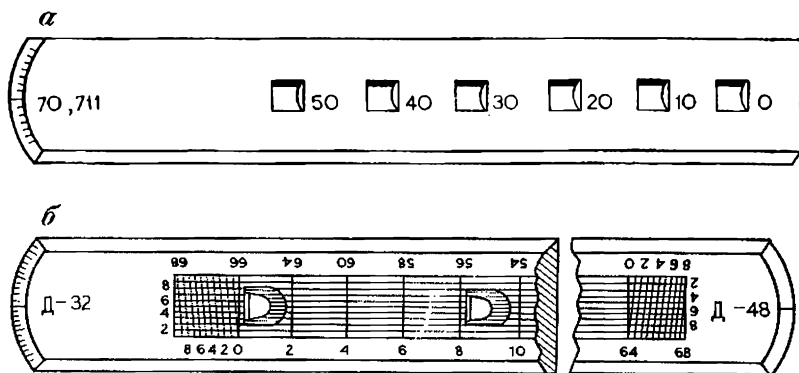
Рис. 4. Линейки: а — Дробьшеза; б — ЛБЛ
