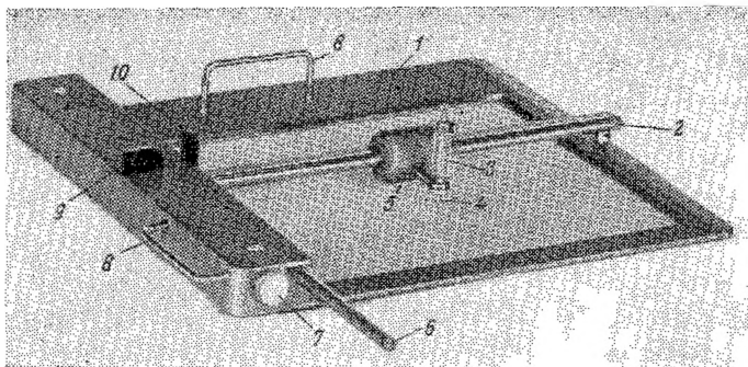
Рис. 82. Штриховальный прибор (ШП)
