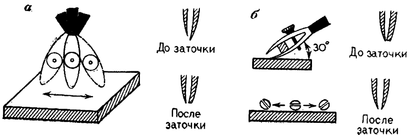
Рис. 29. Заточка рейсфедера: а — I прием; б — II прием
