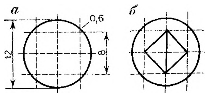
Рис. 64. Построение и вычерчивание условного знака полезного ископаемого «мрамор»
