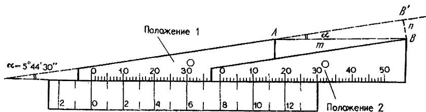
Рис. 11. Синусные линейки
