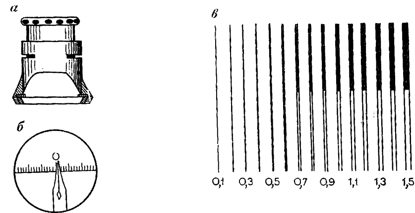
Рис. 23. Измерительная лупа (а); проверка чертежного пера (б); шкала толщин (в)
