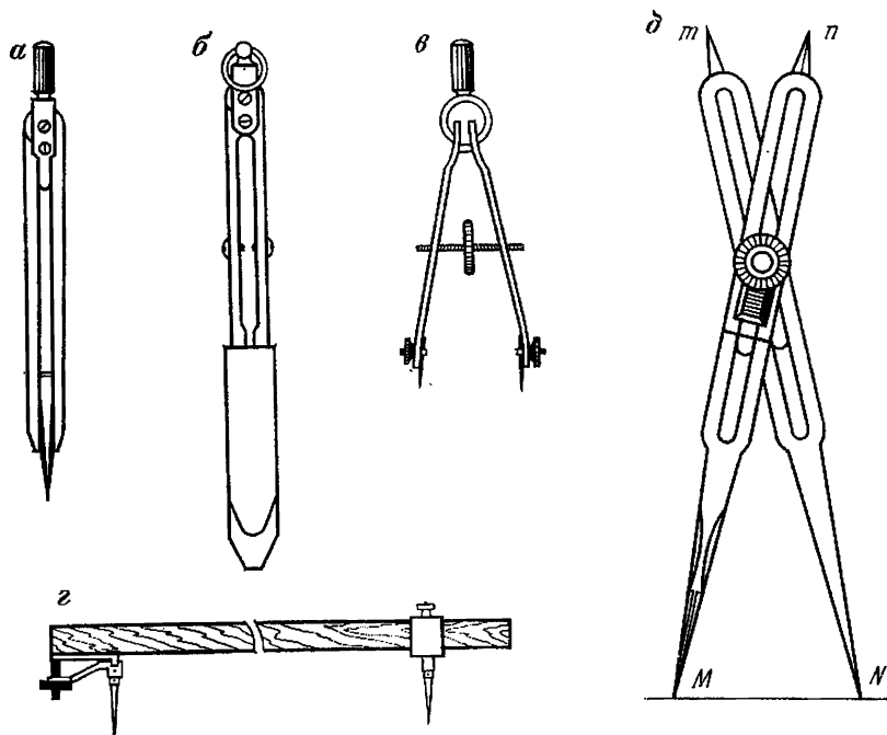
Рис. 9. Циркули:
