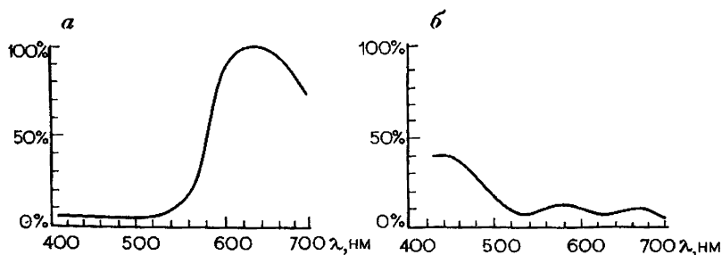
Рис. 87. Спектральные кривые отражения: а — кинновари; б — ультрамарины
