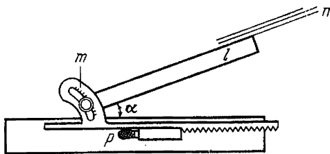
Рис. 12. Схема устройства штриховального прибора
