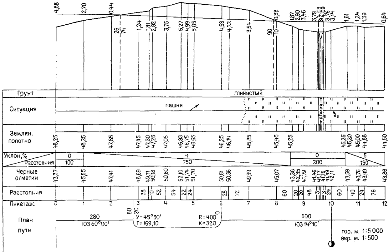
Рис. 63. Продольный профиль
