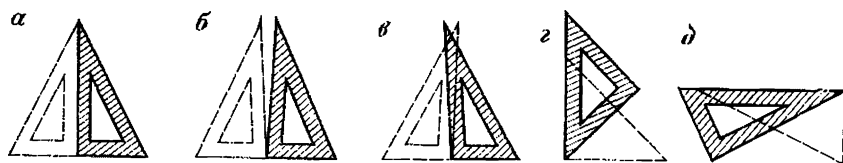
Рис. 5. Проверки треугольников
