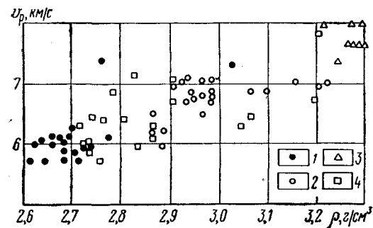
Рис. 54. Зависимость скорости распространения продольных волн в изверженных и метаморфических породах от плотности при p = 4000 кгс/см 2 :
