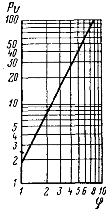
Рис. 23. Зависимость структурного коэффициента \varphi от относительного электрического сопротивления P_v
