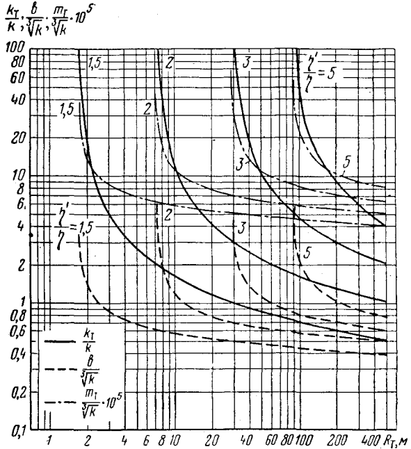
Рис. 70. Изменение величины отношений k_T/k , b/\sqrt{k} , \frac{m_T}{\sqrt{k}} \cdot 10^5 в зависимости от R_T . Цифры на кривых соответствуют величине отношений h'/h
