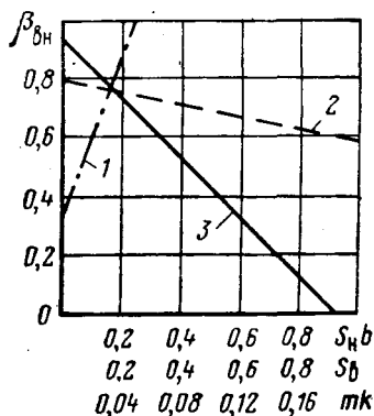
Рис. 87. Зависимость коэффициента вытеснения \beta_{вн} от остаточной нефтенасыщенности S_n b , содержания погребенной воды S_b и произведения пористости на проницаемость для пласта Д 1 Туймазинского месторождения:
