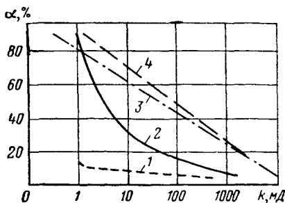
Рис. 73. Корреляционные зависимости между водонасыщенностью ( \alpha ) и проницаемостью параллельно напластованию ( k_{\parallel} ) для некоторых месторождений:
