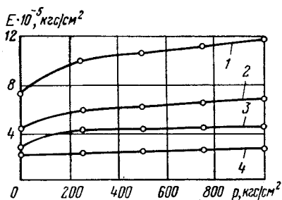
Рис. 51. График зависимости статического модуля Юнга E от всестороннего давления p для образцов горных пород по М. П. Воляровичу и Фан Вэй-цину:
