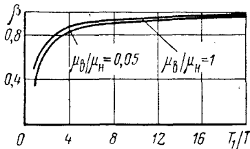
Рис. 82. Зависимость \beta = f(T_1/T) для соотношения вязкостей \mu_b/\mu_n = 0,05 \div 1
