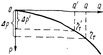
Рис. 67. Индикаторная кривая
