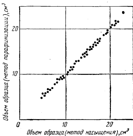
Рис. 5. График объемов образца, найденных разными способами
