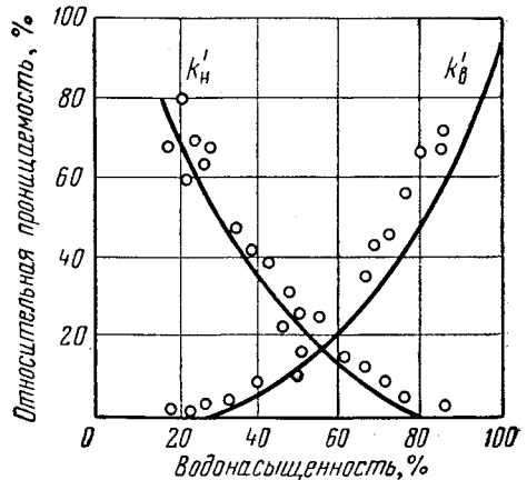
Рис. 38. Зависимость относительных проницаемостей k'_{H} = k_{H}/k и k'_{B} = k_{B}/k от водонасыщенности порового пространства
