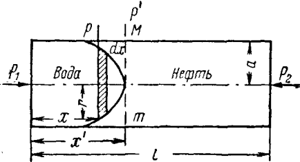
Рис. 80. Схема вытеснения нефти водой из капилляра
