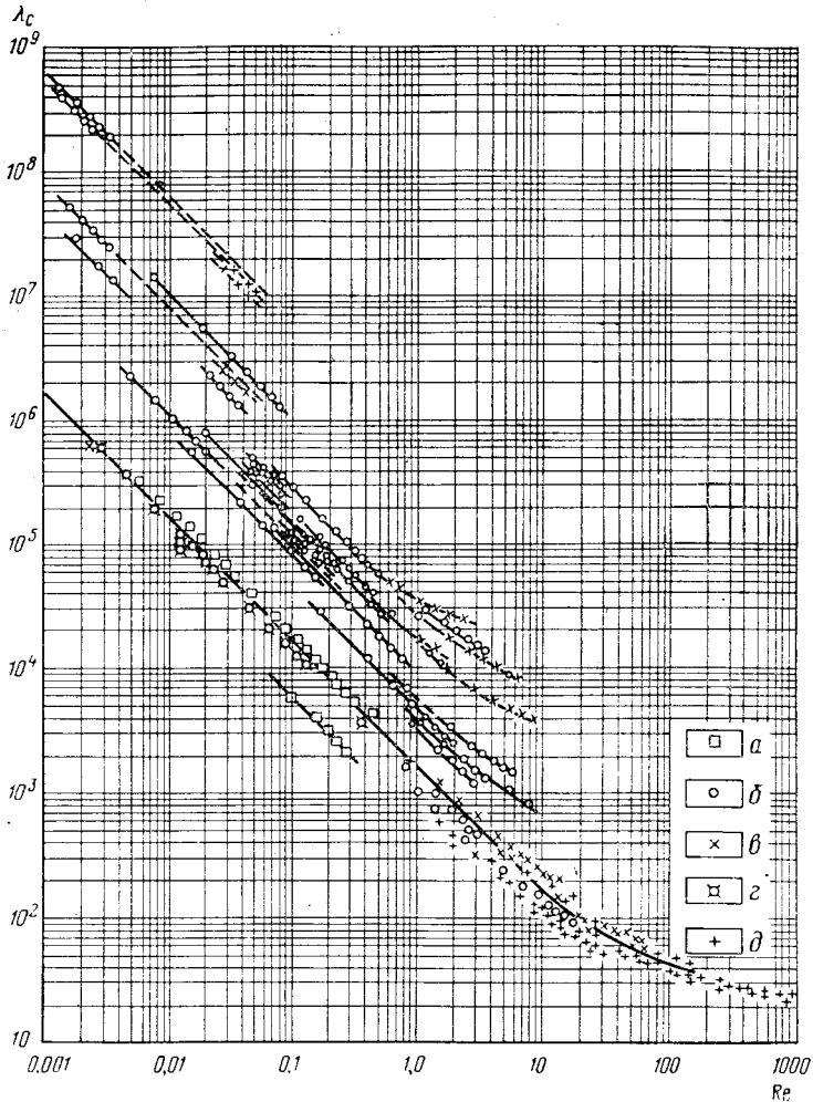
Рис. 30. Зависимость коэффициента гидравлического сопротивления \lambda_c от параметра Re для различных образцов пористых сред по Д. Фенчеру, Д. Льюису и К. Бернсу:
