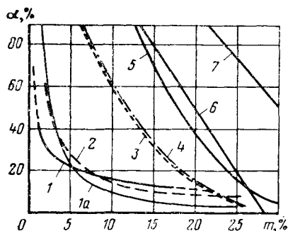
Рис. 72. Корреляционные зависимости между водонасыщенностью \alpha и открытой емкостью пустот матрицы m для некоторых месторождений:
