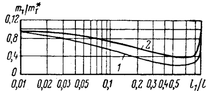
Рис. 21. Зависимость m_T/m_T^* от l_1/l по направлению потока:
