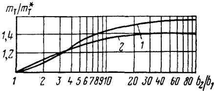
Рис. 19. Зависимость m_T/m_T^* от соотношения b_2/b_1 нормально потоку
