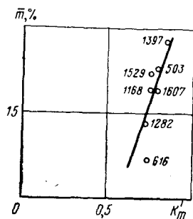
Рис. 14. Кривая зависимости средней пористости \bar{m} от коэффициента однородности K'_m для образцов из различных скважин. Цифры при точках — номера скважин
