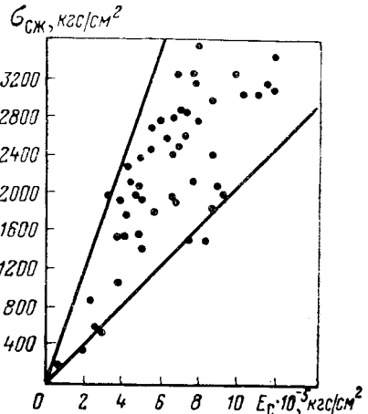
Рис. 57. Зависимость предела прочности на сжатие от статического модуля упругости для горных пород
