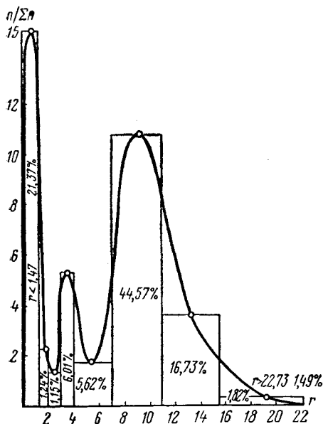
Рис. 26. Распределение пор по размерам при m_{п} = 23\% и k = 0,53 Д
