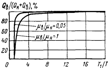
Рис. 84. Зависимость содержания воды в добываемой жидкости от соотношения суммарного времени вытеснения нефти к безводному периоду
