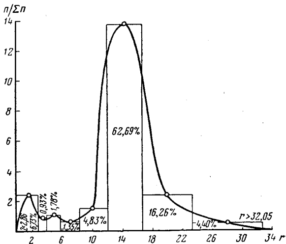
Рис. 25. Распределение пор по размерам для песчаников при m_{II} = 23,5\% и k = 2,574 Д: n — доля пор в заданном интервале
