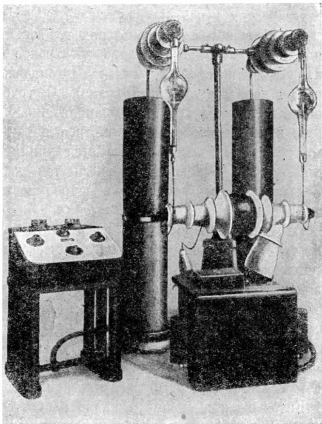
Стабилिवольт производства немецкой электротехнической фирмы Симепс. Это — установка, создающая постоянное электрическое напряжение в 200 000 вольт. Таким напряжением питают рентгеновские трубки, употребляющиеся для просвечивания металлических изделий.
