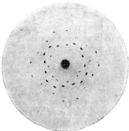
Фотография, снятая Лауэ, Фридрихом и Книппингом. Лучи Рентгена прошли сквозь кристалл сернистого цинка.
