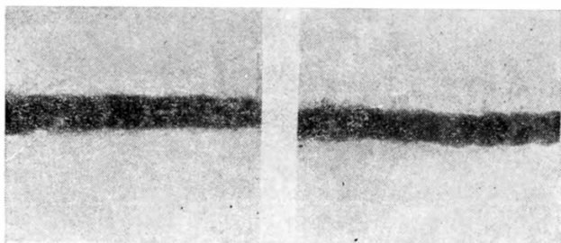
Сварка металлов (рентгеновский снимок). Слева плохая сварка (видны пузырьки воздуха), направо — хорошая сварка.
