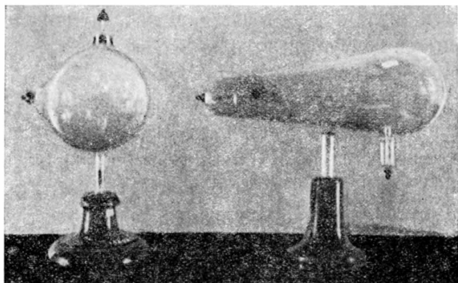
Баллоны с разреженным газом (разрядные трубки), которыми пользовался Рентген.
