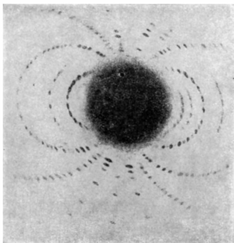
Фотография Лауэ. Лучи Рентгена прошли сквозь кристалл серно кислого вихеля (вверху) и берилла (внизу).
