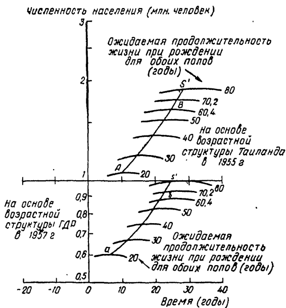
Рис. 7. Сравнение характеристик семейств кривых женского населения с постоянной смертностью, вычисленных на основе населения численностью 1 млн. человек: (А) с возрастной структурой женского населения Таиланда в 1955 г.; (а) с возрастной структурой женского населения ГДР в 1957 г.
