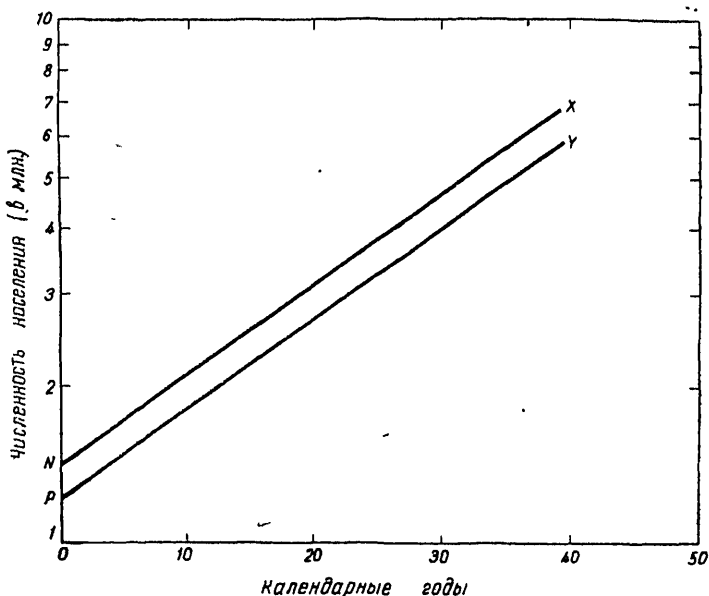
Рис 1. Иллюстративный график, показывающий, как можно вычислить коэффициент инерции населения
