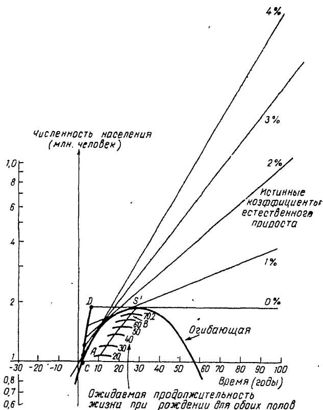
Рис. 11. Огибающая прямых численности населения, соответствующих максимальным значениям истинных коэффициентов естественного прироста для различных уровней плодovitости
