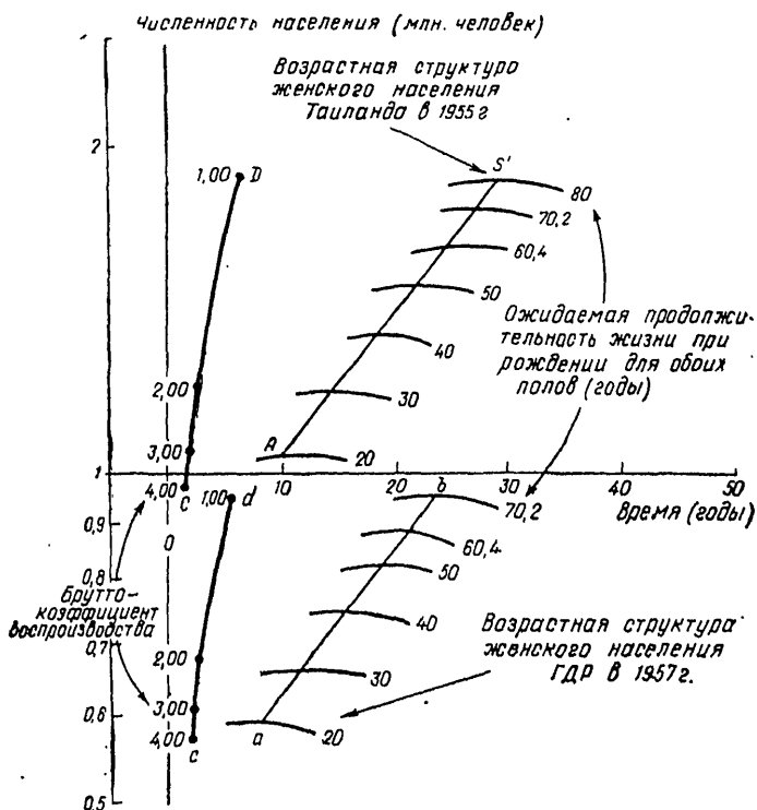
Рис. 10. Сравнение характеристик семей женских населений с постоянной плодородностью и постоянной смертностью, вычисленных на основе населения численностью 1 млн. человек: (А) с возрастной структурой женского населения Таиланда в 1955 г.; (а) с возрастной структурой женского населения ГДР в 1957 г.
