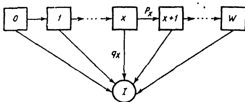
Рис. 1. Диаграмма состояний простого процесса выбытия
