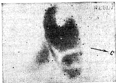
Рис. 17.1. Зарисовка Крабовидной туманности, сделанная лордом Россом.
