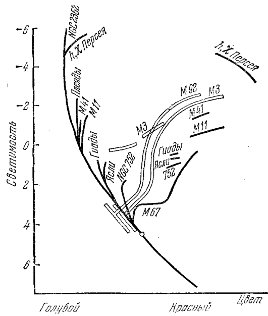
Рис. 12.8. Сводная диаграмма Герцшпрунга — Рассела для различных звездных скоплений.
