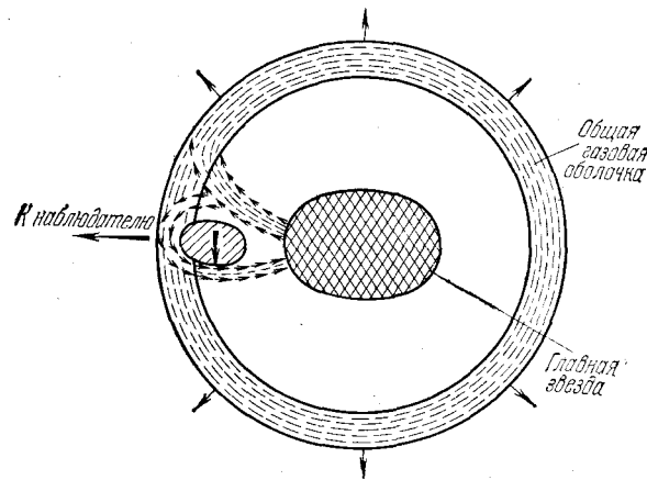
Рис. 14.3. Схематическое представление газовых потоков и диска в системе \beta Лиры.
