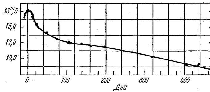
Рис. 15.1. Кривая блеска сверхновой, вспыхнувшей в 1937 г. в NGC 1003.
