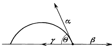
Abb. 8. Die statischen Verhältnisse eines aufliegenden Tropfens.
