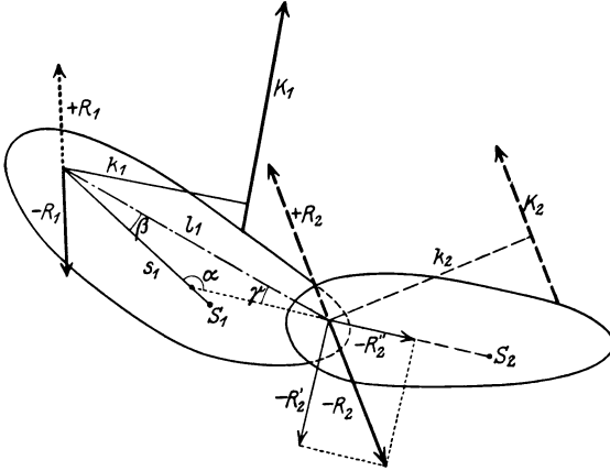
Abb. 122. Die zweigliedrige ebene Kette.
