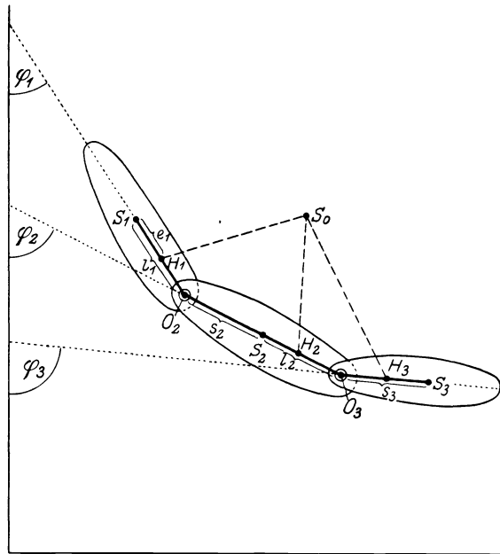
Abb. 123. Gesamtschwerpunkt S_0 , Einzelschwerpunkte S_1 , S_2 und S_3 , und Hauptpunkte H_1 , H_2 und H_3 (nach O. FISCHER).
