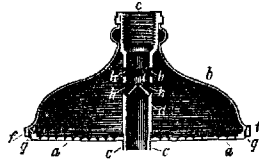
Рис. 3. Наконечник для дождевого душа: а—отверстие в сетке; б—кожух; с и d—закрепительный винт и трубка; f—резьба на кожухе; g—навернутая сетка с отверстиями; h—отверстия в трубке.
