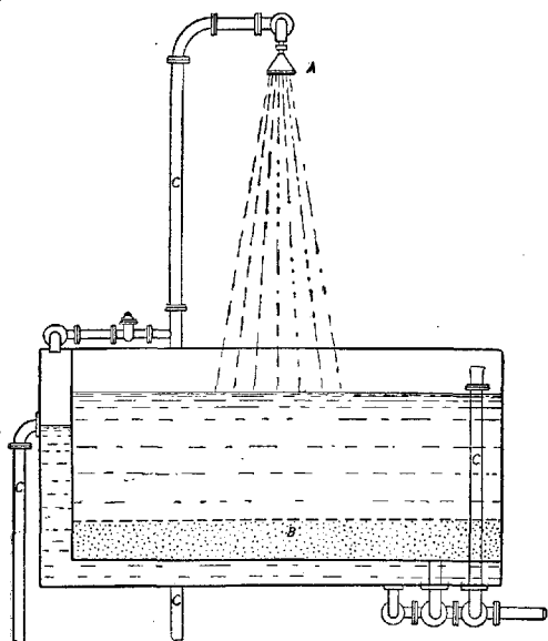
Рис. 2. Схема установки для деферризации по методу Эстена: A —сито; B —фильтр; C —трубопровод.
