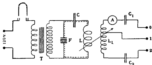
Рис. 2. Т—трансформатор; F—разрядник; C, C 1 , C 2 —конденсаторы; L—первичная спираль соленоида; L 1 —вторичная спираль соленоида; А—амперметр; 0, 1, 2—электроды для лечебных цепей.
