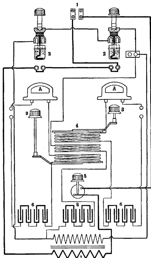
Рис. 2а. Монтажная схема для диатермии: 1—сеть; 2—спирт; 3—термоток; 4—самоиндукция; 5—выключатель; 6—конденсаторы; 7—трансформатор высшего напряжения; А—амперметр.
