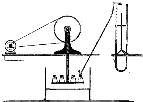
Рис. 6. Schüttel-аппарат Бателли-Штерн.
