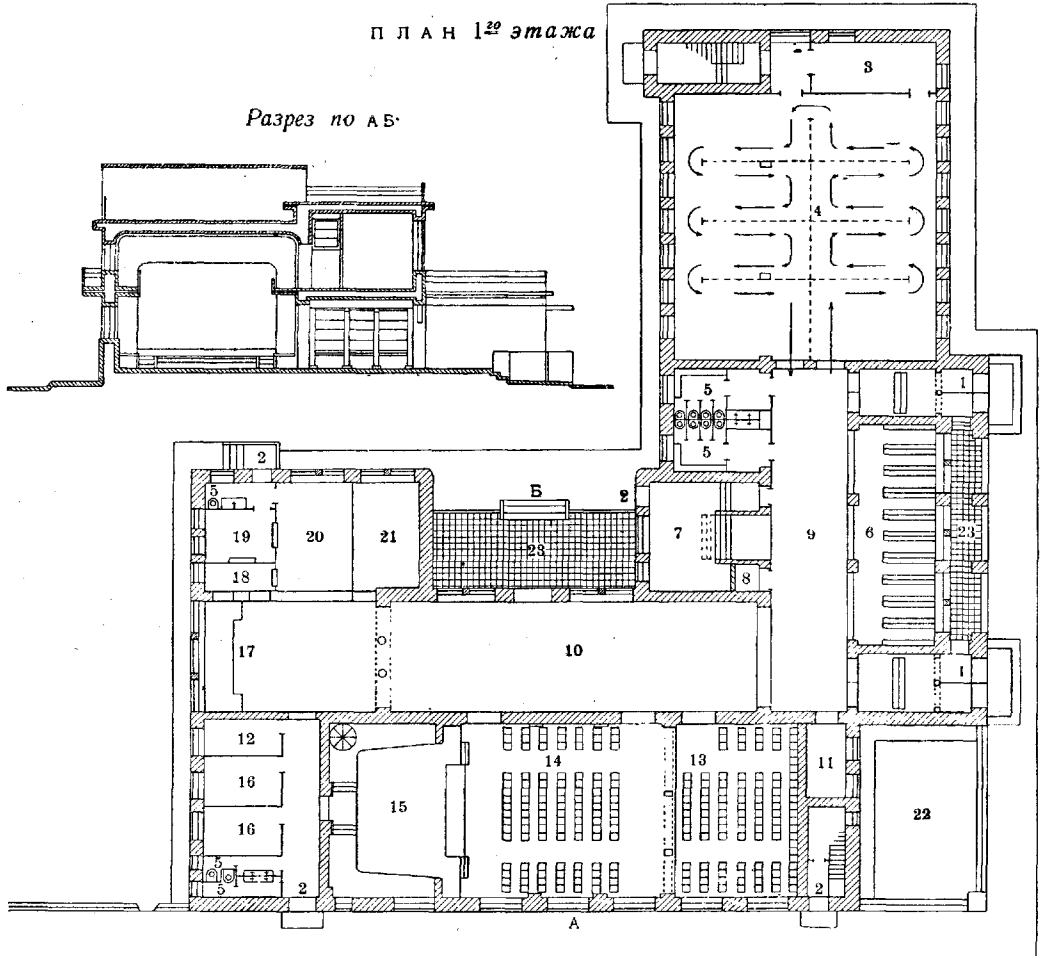
Рис. 2. План 1-го этажа: 1—парадный вход; 2—служебные входы; 3—запасная комната; 4—выставочный зал; 5—уборные; 6—гардероб; 7—лестница на 2-й этаж; 8—телефонная будка; 9—коридор; 10—помещение для специальных и временных выставок (фойе); 11—дежурная; 12—кладовая; 13 и 14—аудитория на 87 и на 138 мест; 15—эстрада; 16—лекторские комнаты; 17—буфет; 18—сервировочная; 19—мочная; 20—кухня; 21—курительная комната; 22—садик; 23—веранды.
