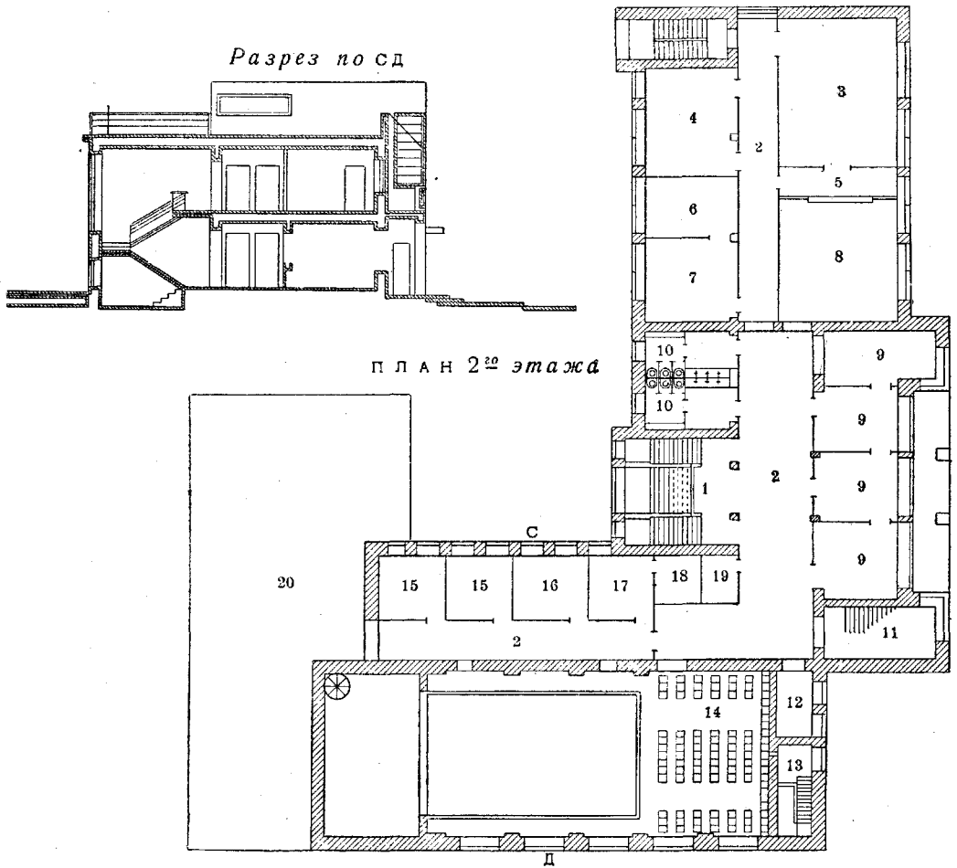
Рис. 3. План 2-го этажа: 1—лестничная клетка; 2—коридор; 3— книгохранилище; 4—фонд наглядных пособий; 5—выдача книг; 6—набинеет заведующего; 7—канцелярия; 8—читальный зал; 9—музей; 10—кухня; 11—ход на крышу; 12—дежурная комната; 13—кухня; 14—хоры; 15—набинееты для научных занятий и кружков; 16—запасный музей; 17—графика и фотографическая комната; 18—темная комната; 19—кладовая; 20—площадка на крыше.
