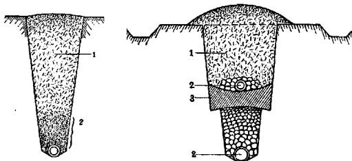
Рис. 2. Дренаж в целях осушения: 1—вынутый грунт; 2—гравий и песок.
