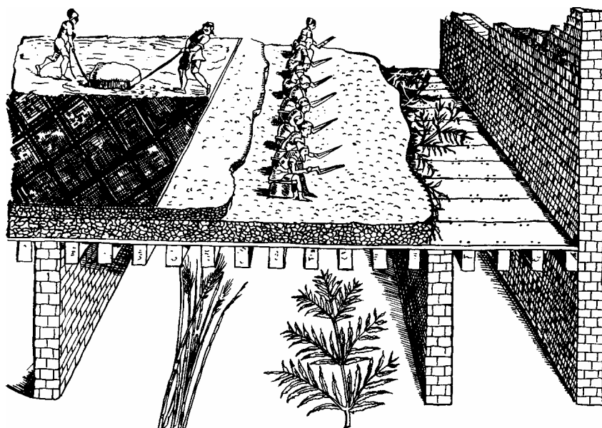
Устройство полов в закрытых помещениях (по Рускони)
