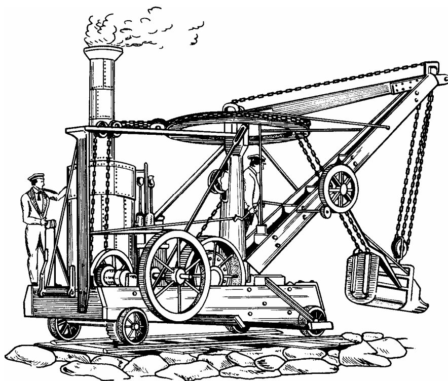
Паровой экскаватор инж. Отиса, США (1834—1836 гг.)
