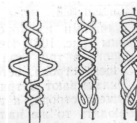
Рис. 108. Обвязывание стропами.
