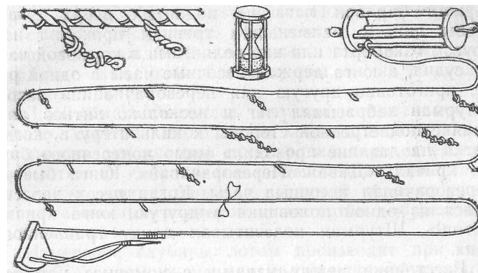
Рис. 113. Ручной лаг.
