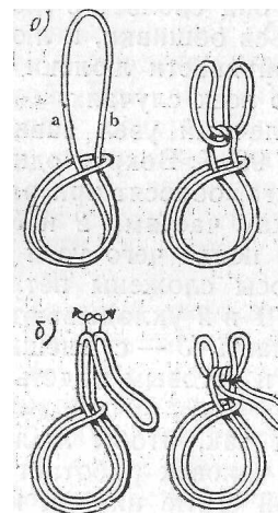
Рис. 95. Крепление на пале нескольких швартовных концов.
