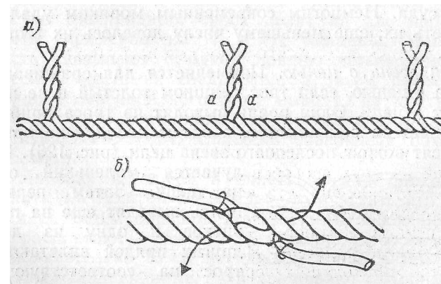
Рис. 125. Длинный сплесень.
