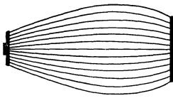
Abb. 59. Feldlinienverlauf bei verschieden großen Elektroden.
