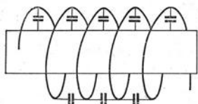
Abb. 76. Jede Spule besitzt auch eine Kapazität.
