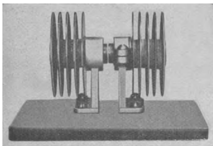
Abb. 32. Löschfunkenstrecke.
