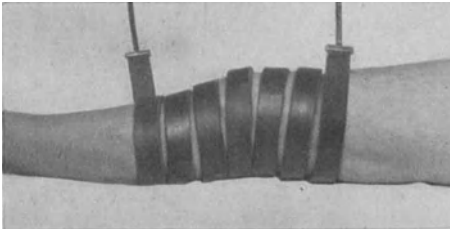
Abb. 98. Behandlung eines Kniegelenkes im Spulenfeld.
