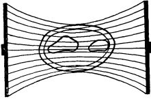
Abb. 58. Verdichtung des Feldes im Querschnitt eines Handgelenkes.
