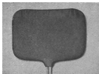
Abb. 132. Elektrode zur Hyperthermiebehandlung im Spulenfeld (Sanitas).
