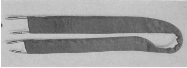
Abb. 133. Schleifenelektrode zur Hyperthermiebehandlung im Spulenfeld (Abb. 130).
