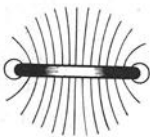
Abb. 14. Das Magnetfeld eines ringförmigen Leiters.
