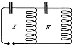
Abb. 26. Galvanische Koppelung.
