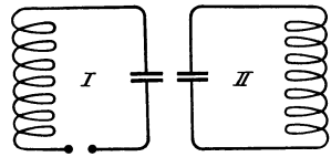
Abb. 28. Kapazitive Koppelung.
