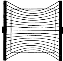
Abb. 57. Die Oberfläche der Elektroden ist größer als der Querschnitt des Behandlungsobjektes. Tiefenwirkung größer als 100%.
