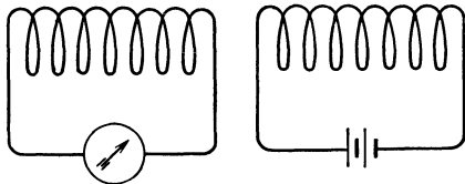
Abb. 18. Induktion durch das Magnetfeld einer stromführenden Spule (Elektromagnet).
