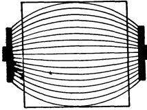
Abb. 55. Die Oberfläche der Elektroden ist kleiner als der Querschnitt des Behandlungsobjektes. Tiefenwirkung kleiner als 100%.
