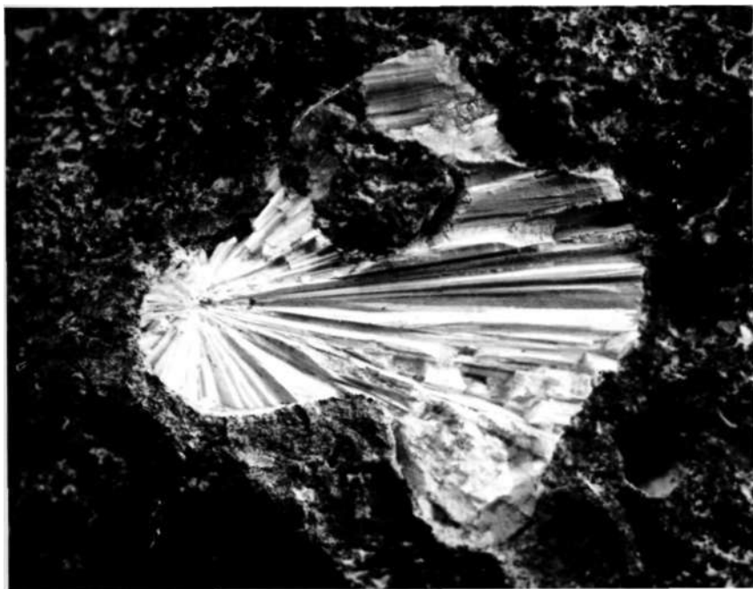
Рис. 58. Арагонитовая миндалина с лавовым пережимом в средней части в базальте. Кисарити, верховье р. Уравели, ГрузССР. Уа 3. № 83050.
