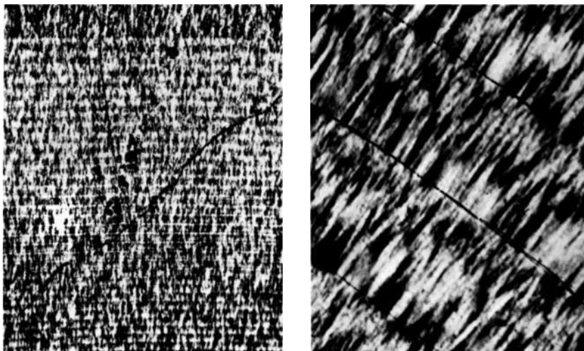
Рис. 41. Тонкоритмичное строение кварц-халцедоновой сферолитовой корки из зон волокнистого халцедона (широкие зоны \approx 25 мкм) и тончайших зоннок из зерен кварца с постепенно возрастающей толщиной (от \approx 1 мкм внизу до \approx 19 вверх). Ув. 35( + ). Чащын Нос, Сев. Тиман, № 79587. Я.
