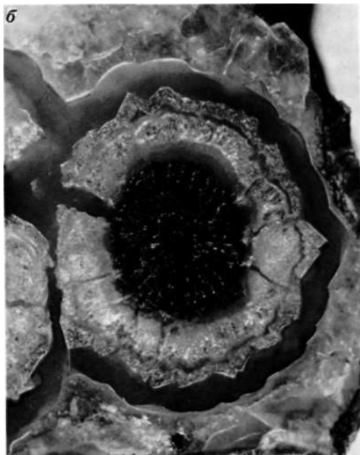
Рис. 82. Пирит-кварц-халцедоновые псевдосталактиты в агате: a — общий вид, ув. 10; б — поперечный срез одного из псевдосталактитов, ув. 40, мыс Теви, Камчатка. № 84454.
