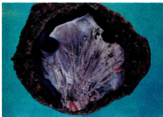
Фото 132. Псевдоморфоза халцедона и кварца (немного) по сноповидному сростку пластинчатых кристаллов ангидрита (?) или возможного барита (?), заполняющего центральную полость литофизы. Аягуз, КазССР. 8,0X7,5 см. № 84532.
