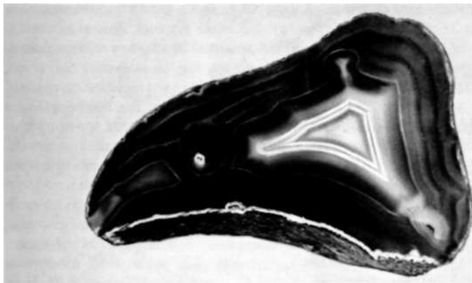
Рис. 7. Конусовидная халцедоновая (агатовая) миндалина с вдавненной формой дна (близкая к миндалинам типа 4 на рис. 6); слева — поперечный срез псевдосталактита на настыльной сосульке (?). Мыс Теви, Камчатка. 0,75 нат. вел. № 82990.
