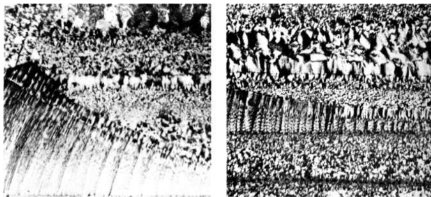
Рис. 57. Переход зон мелкозернистого и параллельно-шестоватого халцедона параллельно-слоистого агата в концентрически-зональную (облегающую) сферолитовую корку халцедона с постепенным их расширением. Правая часть — сопряжение параллельно-слоистой зональности с зонально-концентрической, левая — расширение зон параллельно-слоистого агата. Мулина Гора, Читинская обл. Ув. 15(+). № 7/7.
