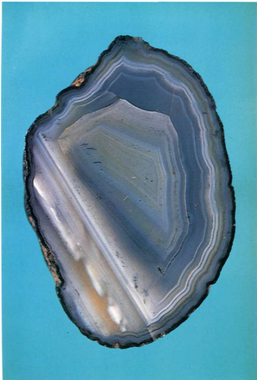
Фото 33. Ониксовый агат с изменением угла наклона слоев и постепенным увеличением толщины ониксовых слоев, переходящих в облегающую зональность; в широком белом нижнем ониксовом слое хорошо видна его перекристаллизация с образованием ящичных элементов текстуры. Магаданская обл. 6,0X3,5 см. № 84749.
