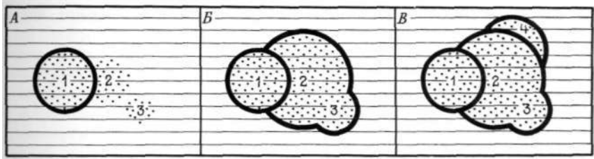
Рис. 22. Диаграмма, иллюстрирующая рост и коалесценцию сферолоидов; после образования корки-коры (черная) дальнейшее расширение сферолоида прекращается [159].
