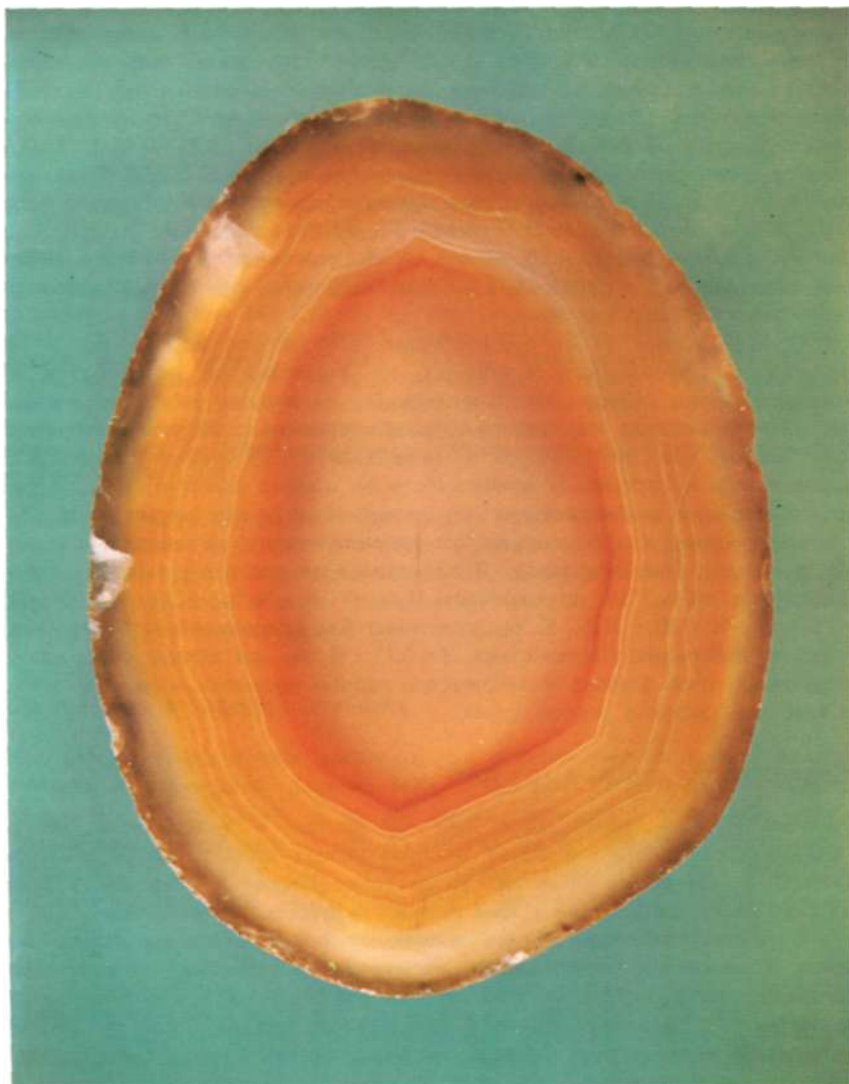
Фото 16. Халцедоновый карнеол-агат зонально-концентрического строения. Россыпи по р. Зея, Амурская обл. 4,5X3,0 см. № 83910.
