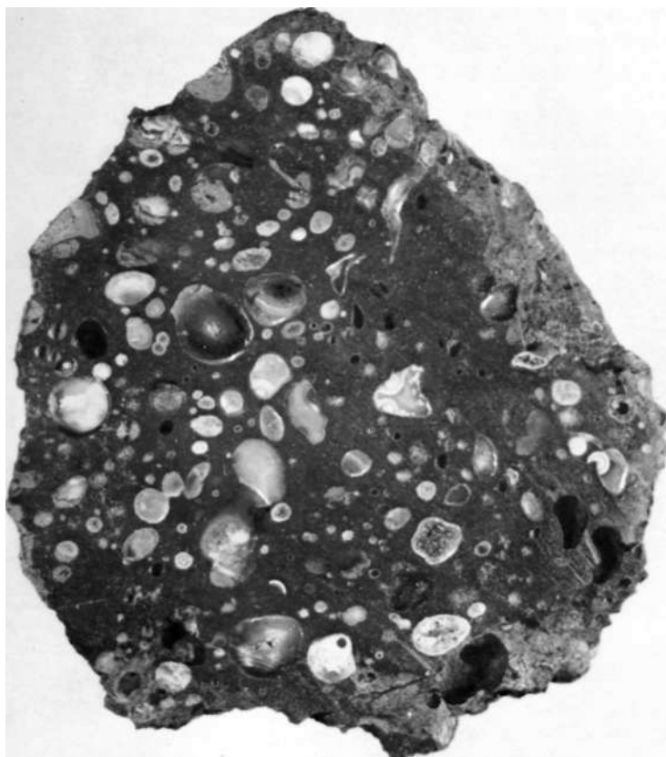
Рис. 2. Миндалекаменный базальт с газовыми пузырями, частично заполненными халцедоном (агатом), кальцитом и яшмой. Гора Мурунда, Читинская обл. Нат. вел., № 83035.
