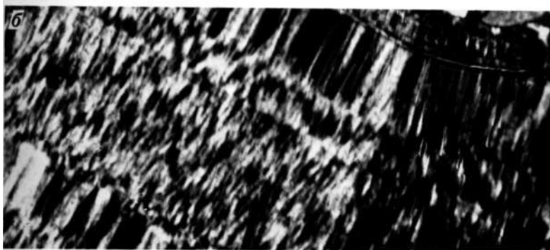
Рис. 34. Ритмично-зональное строение сферолитовой корки халцедона, состоящей из зон близкой структуры, но разной толщины; хорошо видно, что одни и те же зоны продолжаются в обоих соседних сферолитах. Идар — Оберштейн, ФРГ. Ув. 35 ( + ). № 48280. Я.
