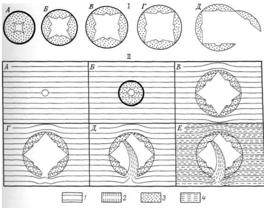
Рис. 23. Схема формирования центральной полости в литофизе в форме реберного куба и открытия литофизы наружу (I) и взаимоотношения образующейся литофизы с флюиальностью вмещающего риолита, внедряющегося в виде языка в литофизу (II), по В. Х. Брайану, с дополнениями авторов
