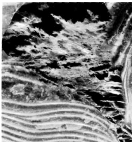
Рис. 66. Тонкопластинчатая ромбоэдрическая сетка, халцедона, развивающаяся по спайности крупнокристаллического кальцита, закупоривающего «питающий» канал; хорошо видно утонение части халцедоновых слоев при их повороте в канал и резорбция части халцедоновых слоев кальцитом. Кальцит вытравлен 10% -ной HCl. Чаицын Нос, Сев. Тиман. Ув. 8.
