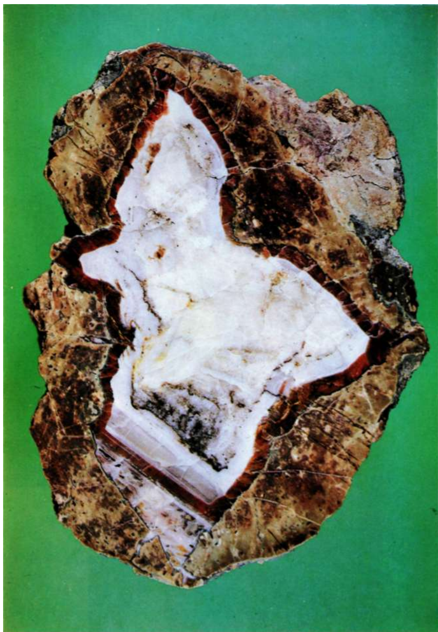
Фото 120. Агат с плинтоидной текстурой в нижней части, сменяющейся параллельно-слоистой (ониксовой) текстурой, переходящей, начиная с карнеолового слоя, в зонально-концентрическую текстуру; в ядре — кварц и кальцит. Айнабулак, КазССР. 14,0X10,0 см. № 83218 (повернут примерно на 45°).
