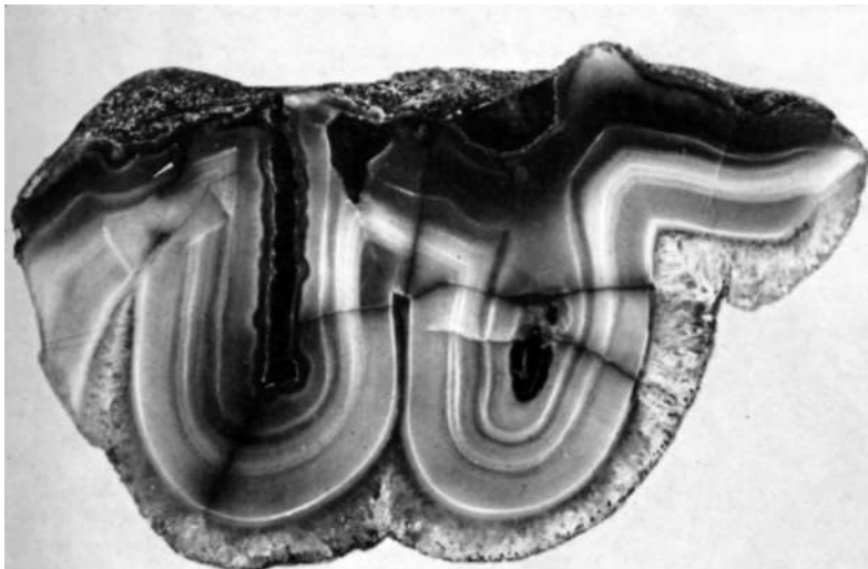
Рис. 12. Зональность полосчатого халцедона, облекающего настильные сосульки (темное в центре псевдосталактитов) и кровлю миндалины, подтверждающая псевдосталактитовую природу этих образований; наружная корка — кварц. Камчатка. Ув. 1,5. № 82991.
