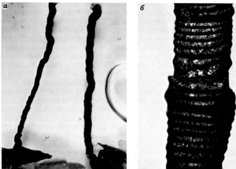
Рис. 91. Мембранные трубки силикатного соединения меди, полученные при взаимодействии медного купороса с силикатным клеем
