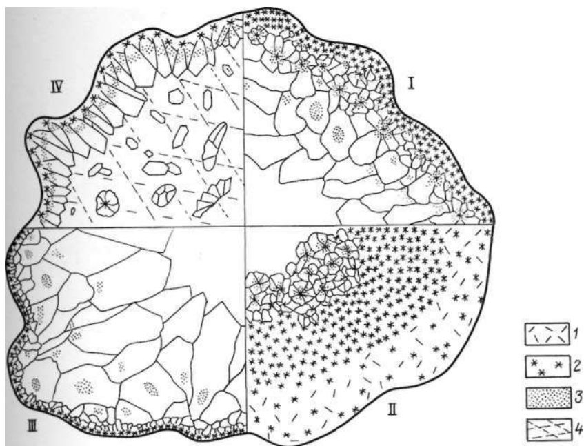
Рис. 25. Схематическая зарисовка строения псевдоморфоз минералов кремнезема по ангидритовым конкрециям с различным типом минерализации (I—IV): 1— волокнистый разноориентированный микрокристаллический кварц; 2— сферолиты кварца; 3— включения ангидрита; 4— кальцит [214].
