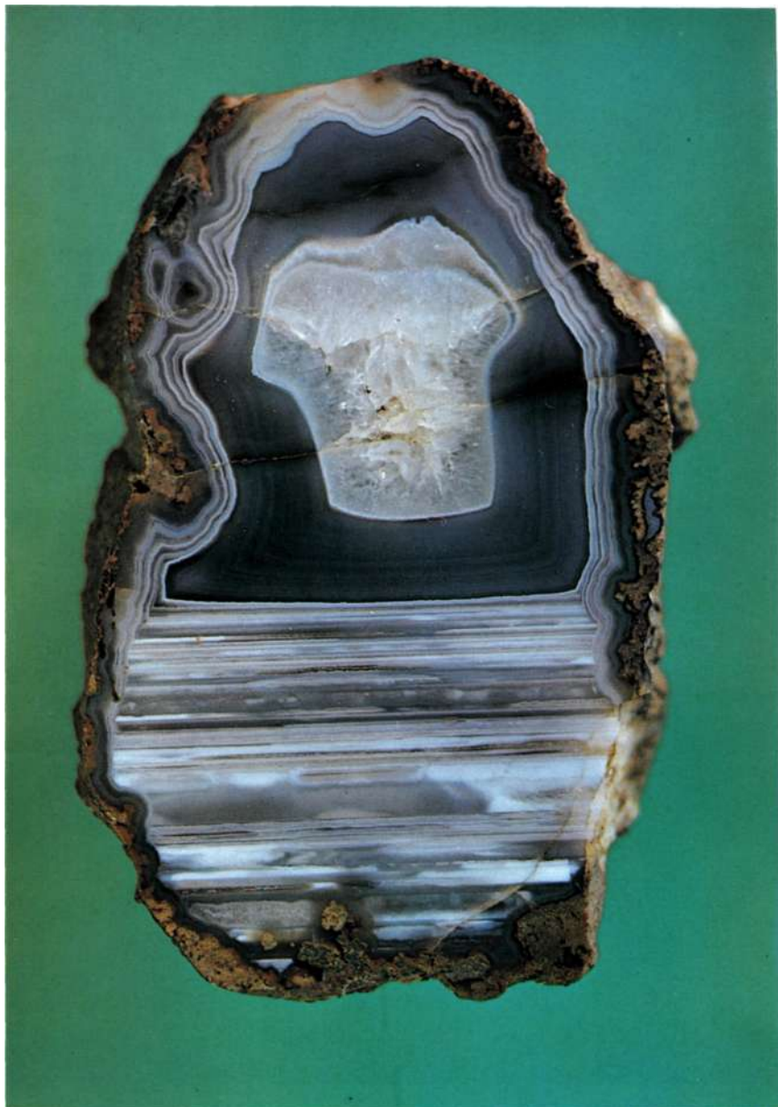
Фото 4. Вертикально вытянутая овальная миндалина с параллельно-слоистым (ониксовым) агатом, слои которого упираются в халцедоновую корку снизу и, начиная с последнего верхнего белого слоя, переходят в зонально-концентрический (облекающий) халцедон; полость вверху заполнена крупнокристаллическим кварцем. На нижних горизонтальных слоях оникса — многочисленные отчетливые следы перекристаллизации. Арц-Богдо, Монголия. 12,5X7,5 см. вел. № 83053.
