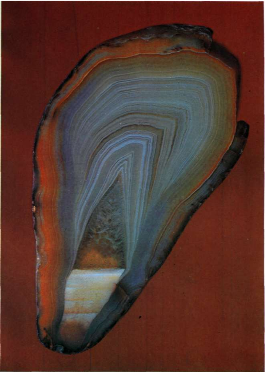
Фото 6. Грушевидная миндалина с широким «питающим» каналом, снизу заполненным халцедоновым ониксом; выше — крупнозернистый кварц. Хорошо видно выклинивание отдельных зон халцедона, облегающего стенки миндалины и заполняющего верхнюю ее часть по мере их приближения к периферии. Россыпи по р. Зея, Амурская обл. 6,5X4,0 см.
