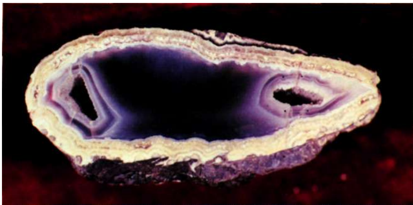
Фото 95. Поперечное сечение плоской кальцит-халцедоновой миндалины с кольцевым каналом; кальцит образует корку по периферии миндалины; внутренняя полость канала покрыта тончайшей корочкой мелких кристалликов кварца. Мыс Теви, Камчатка. 8,0X3,5 см. № 83754.
