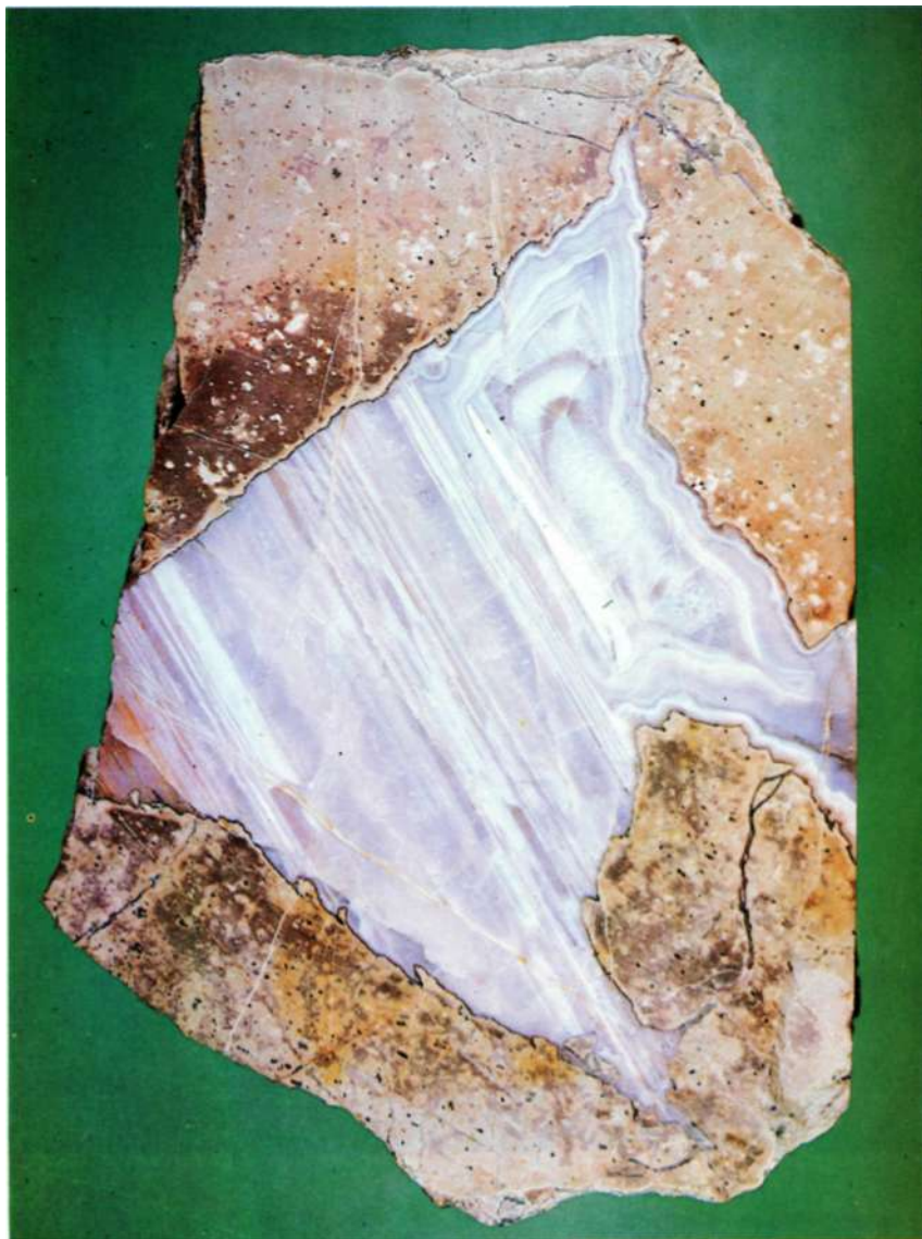
Фото 119. Агат с ониксовой и облекающей зональностью в центральной полости фельзитовой литофизы; хорошо видны следы перекристаллизации ониковых слоев. Айнабулак, КазССР. 22,0X14 см. № 84528.
