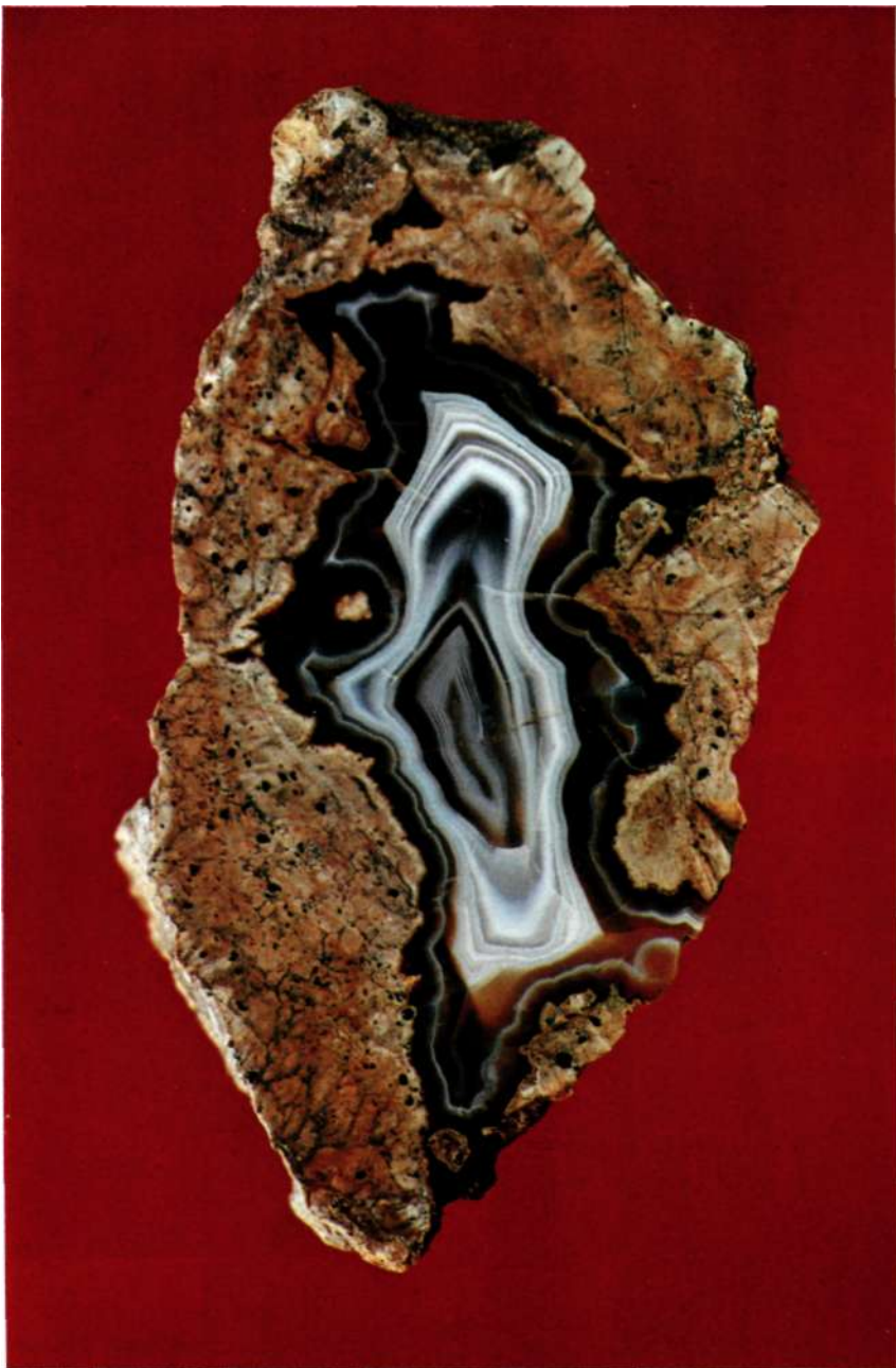
Фото 115. Агагы из риолиток а — Тарбалджей, Читинская обл., 13,0X8,0 см. № 83232; б— Канэнмывеем, Чукотка, 10,5X6,5 см. № 84760.
