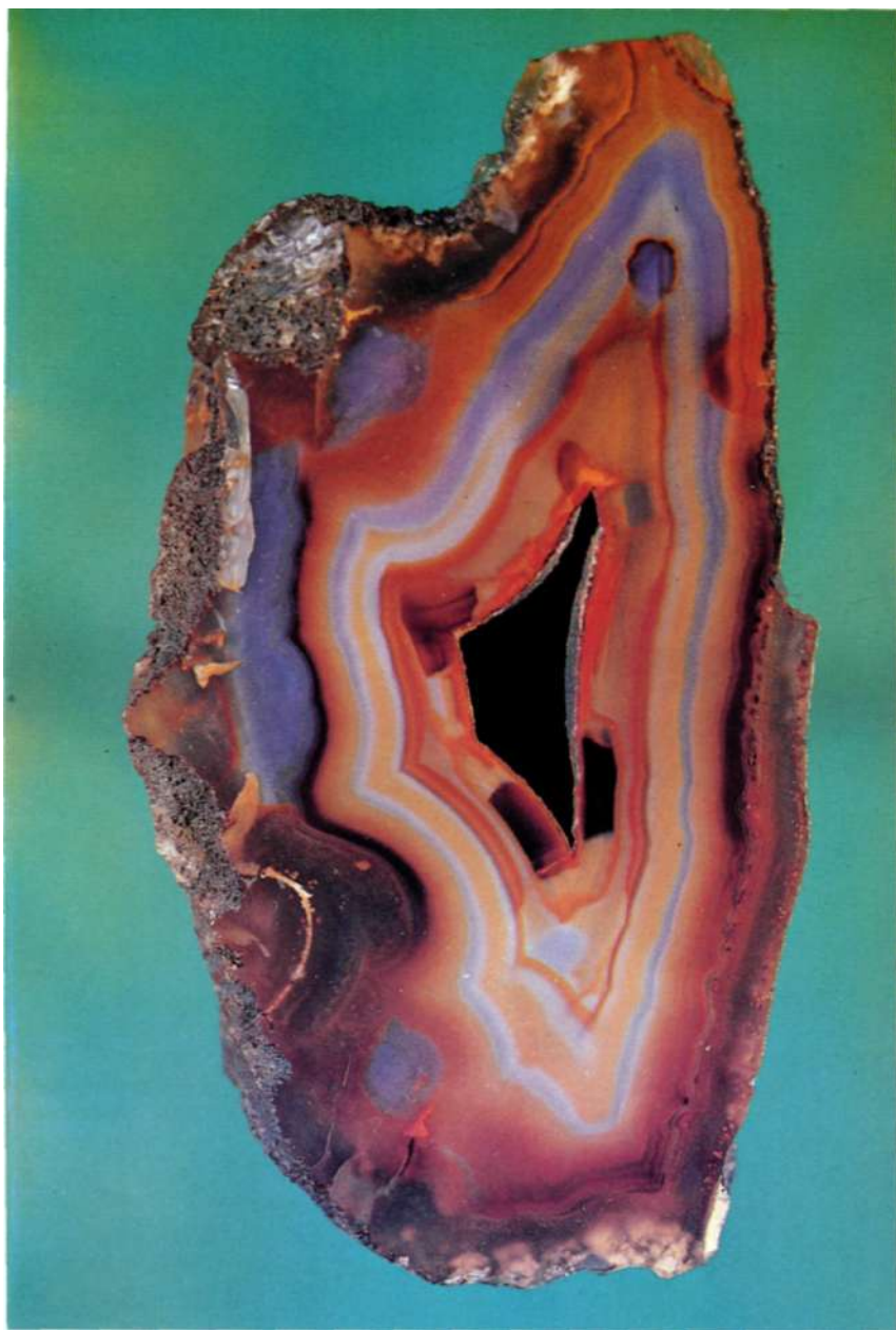
Фото 19. Зонально-концентрический халцедон в уплощенно-округлой миндалине с полостью в центре; окраска предпоследнего слоя свидетельствует о его сильной перекристаллизации с образованием отдельных «кирпичиков», интенсивно вторично окрашенных. Арц-Богдо, Монголия. 8,0X4,5 см. № 84759
