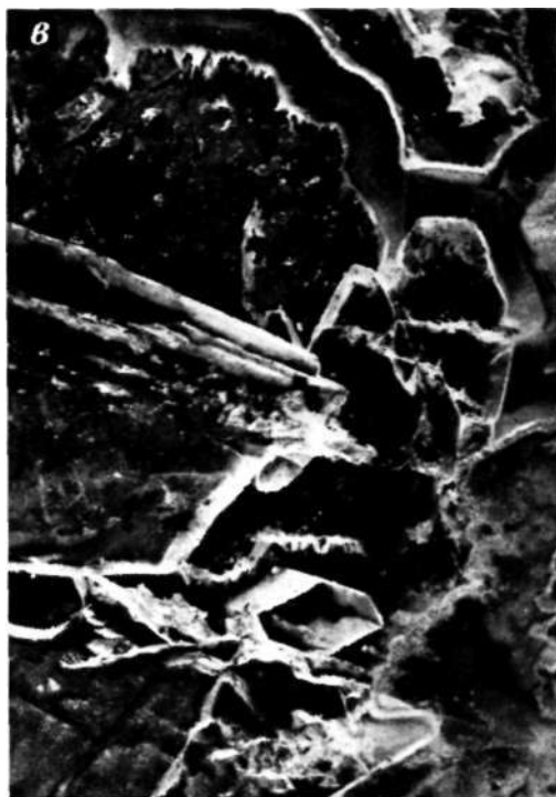
Рис. 65. Начальные стадии замещения крупных скаленоэдрических кристаллов кальцита халцедоном:
