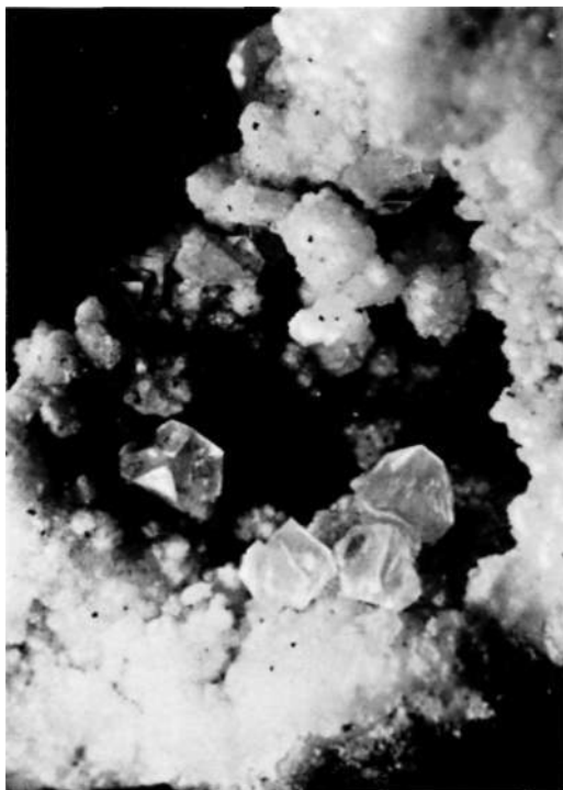
Рис. 81. Крупные воднопрозрачные кубические, кубооктаэдрические кристаллы флюорита и двойники прорастания, нарастающие на корку мелкокристаллического флюорита, покрывающего шетки кварца в полости псевдоморфозы минералов кремнезема по конкреции кальцита. Окрестности Бейнеу, горы Туаркыр, ТССР. Ув. 2. № 84535.
