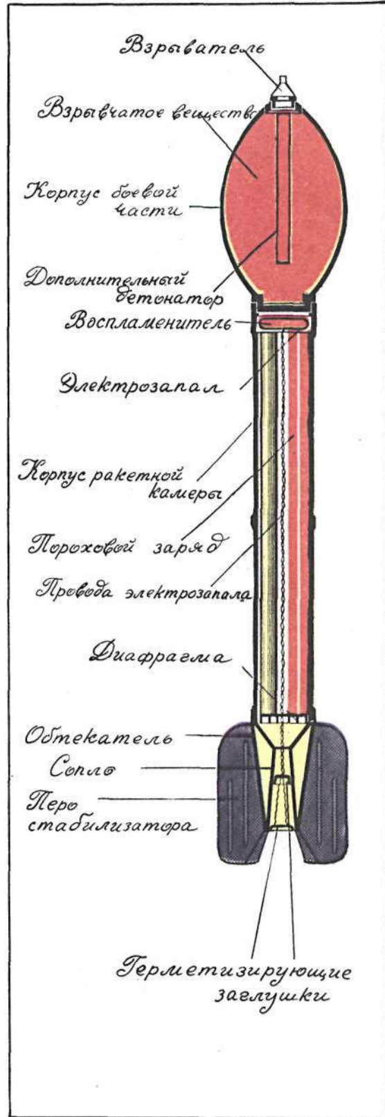
Устройство фугасного реактивного снаряда М-31.
