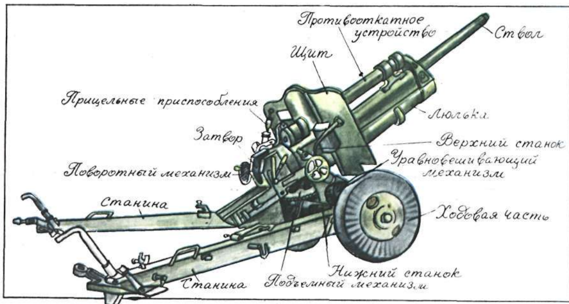
Устройство артиллерийского орудия.
