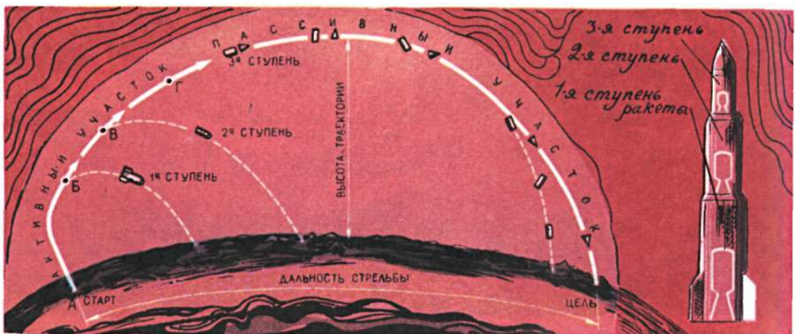
Траектория полета трехступенчатой баллистической ракеты.
