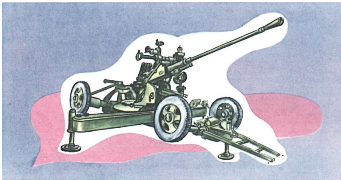
37-миллиметровая автоматическая пушка.
