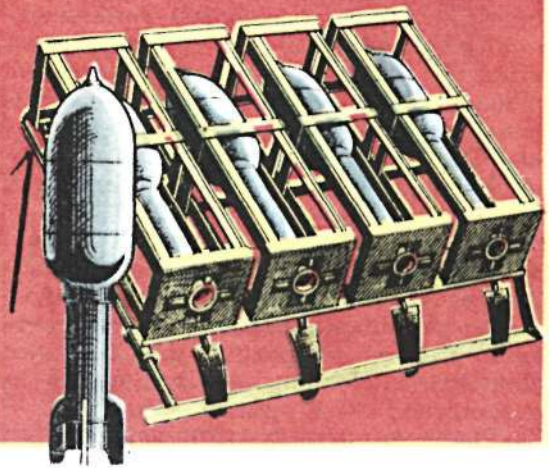
Фугасный реактивный снаряд М-30 и наземная пусковая установка
