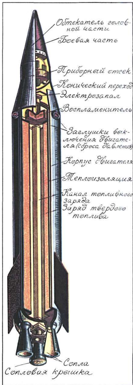
Устройство управляемой баллистической ракеты на твердом топливе.
