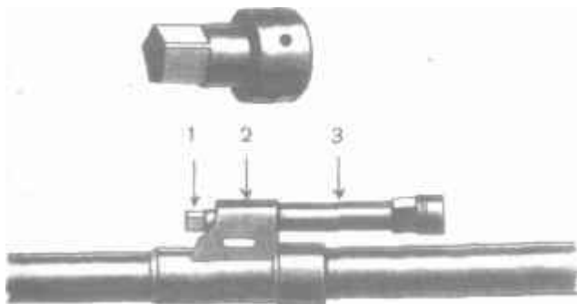
Газовый регулятор. На верхнем рисунке видны отверстия, которые регулируют дозу газов, поступающих в камеру. На нижнем рисунке показано, как соединены между собой регулятор 1, газовая камера 2 и патрубок 3.
