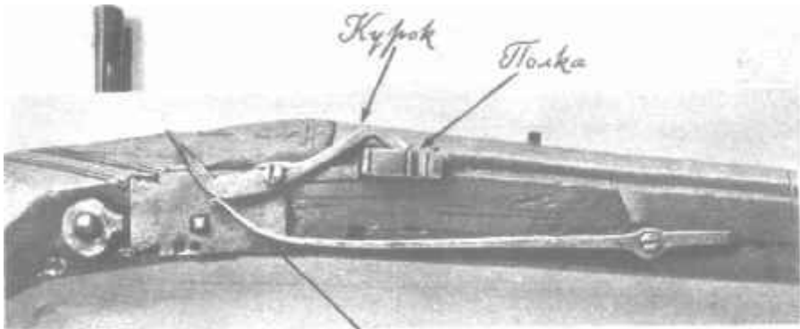
На таких фитильных ружьях стреляли в XVI веке. На верхнем снимке видно, как устроен фитильный замок.
