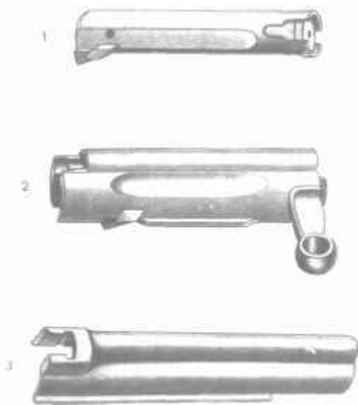
1 — остов затвора; в нем помещаются ударник и выбрасыватель; 2 — стебель затвора; 3 — эта крышка соединяет затвор со ствольной коробкой.
