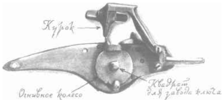
Кремневый колесный замок. Перед выстрелом пружину, прикрепленную к колесу, закручивали специальным ключом.
