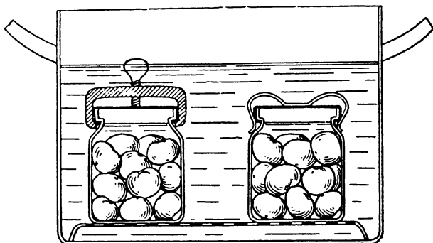
Рис. 8. Стерилизация укупоренных банок: слева — на крышку одет винтовой зажим; справа — пружинящий зажим.
