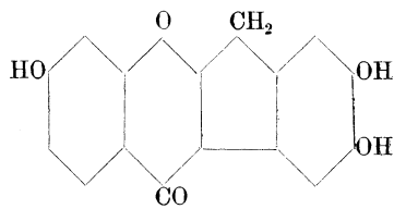
Brasilin
