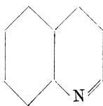
Chinolin.
