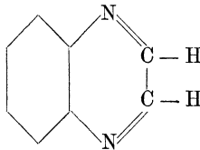
Chinoxalin
