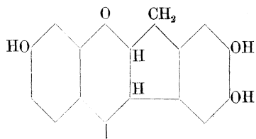
Brasilin
