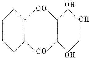
Purpurin 1:2:4
