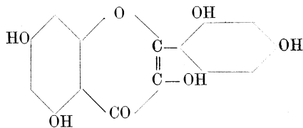
Morin.
