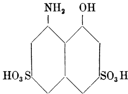
Amidonaphtoldisulfosäure H.
