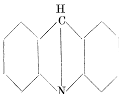
Acridin.
