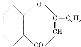
Flavon.
