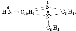
Rosindulin.
