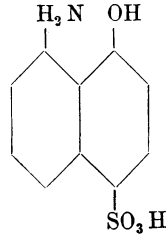
Amidonaphtolsulfosäure S.
