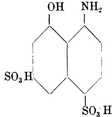
Amidonaphtoldisulfosäure K.
