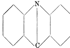
Acridin.
