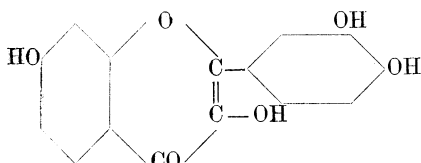
Fisetin.
