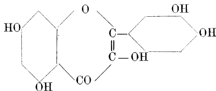
Quercetin.
