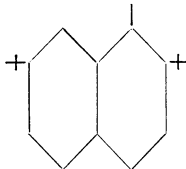
Bender. Ber. 22. 996.
