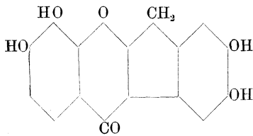
Hämatein
