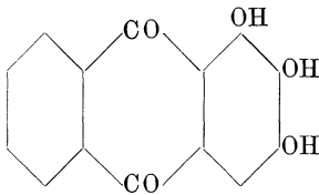
Anthragallol 1:2:3
