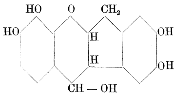
Hämatoxylin
