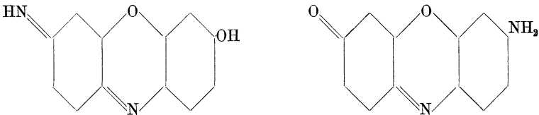
Resorufamin.
