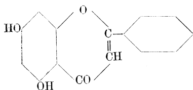
Chrysin.
