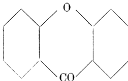
Xanthon.
