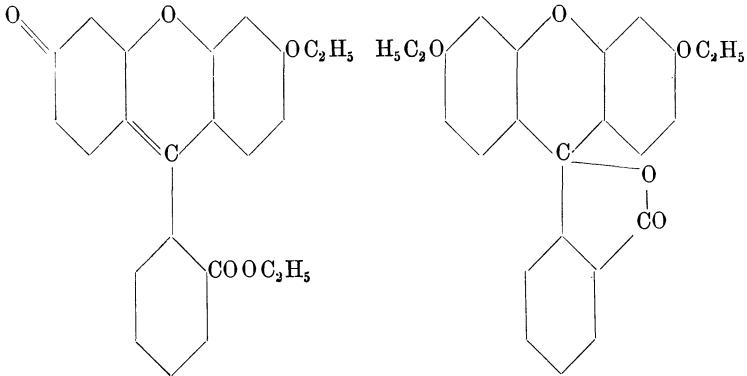
Chinoïder Diäthyläther.
