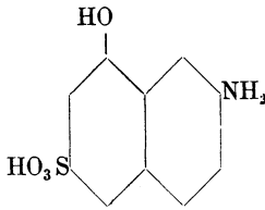
Amidonaphtolsulfosäure G.
