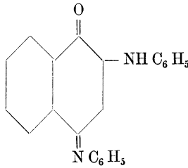
Rosindulin.
