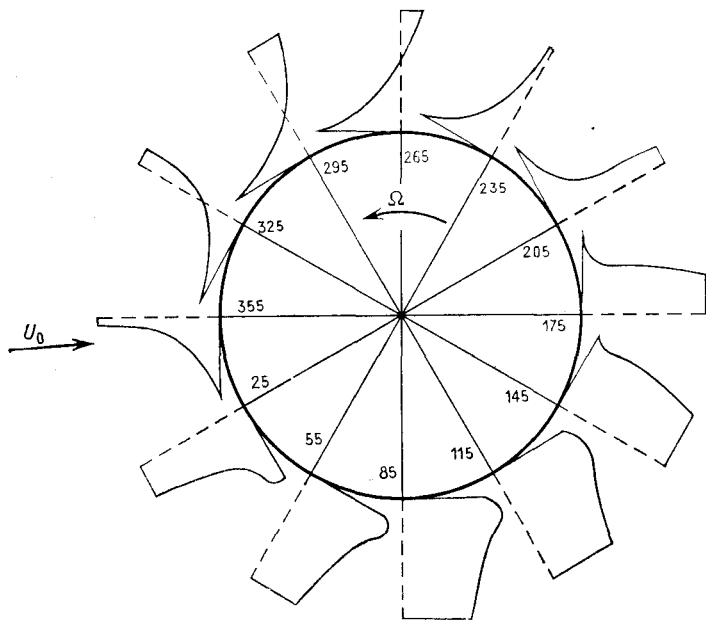
Рис. 7.11. Профили скорости в пограничном слое на вращающемся цилиндре; Re = 200 , отношение скоростей V_{танг}/U_0 = 2 . (Из работы Томана и Шевчика [1966].)
