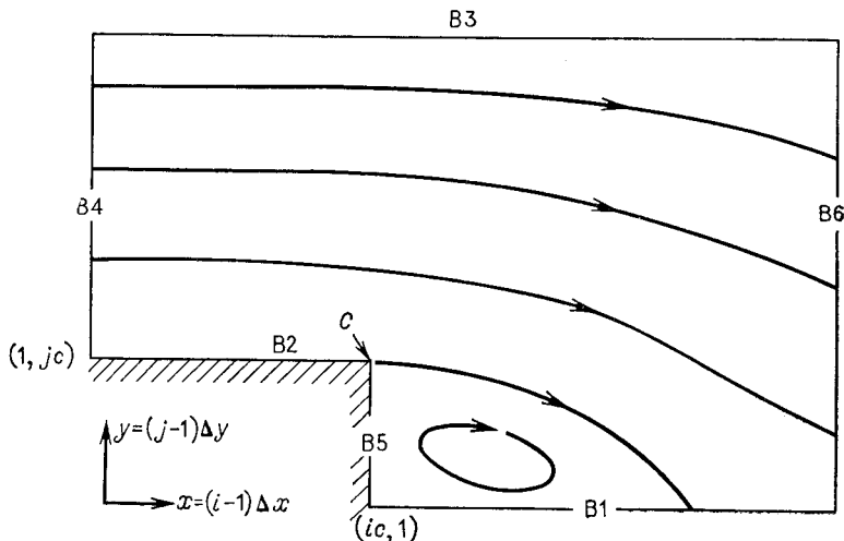
Рис. 3.22. Границы расчетной области в задаче об обтекании обратного уступа. В 1 — осяевая линия (линия симметрии), В 2 — наветренная часть твердой поверхности, В 3 — верхняя граница, В 4 — входная граница потока, В 5 — основание уступа, В 6 — выходная граница потока.
