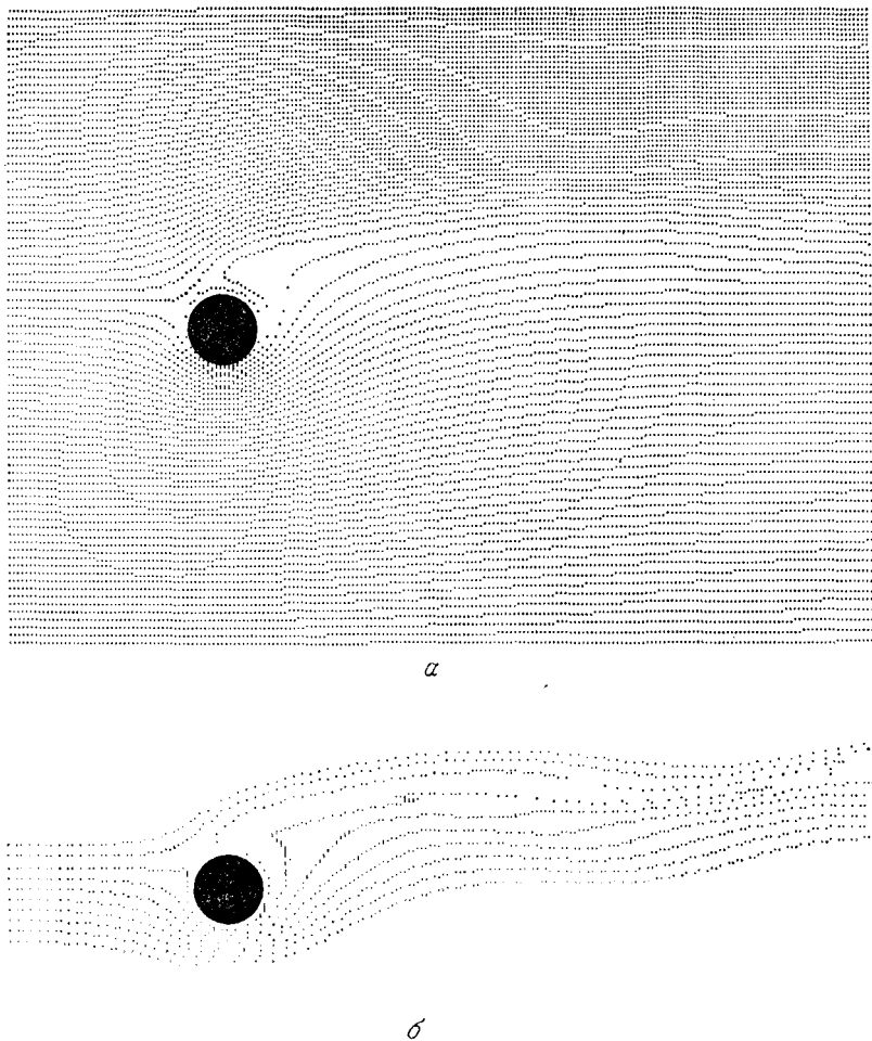
Рис. 7.4. Построенные на печатающем устройстве линии тока и линии отмеченных частиц при циркуляционном обтекании кругового цилиндра с отношением скоростей V_{\text{танг}}/U_0 = 2 ; Re = 200 , безразмерное время 21.139. (Из работы Томана и Шевчика [1966].) а — линии тока, \Delta\psi = 0.000196 ; б — линии отмеченных частиц.
