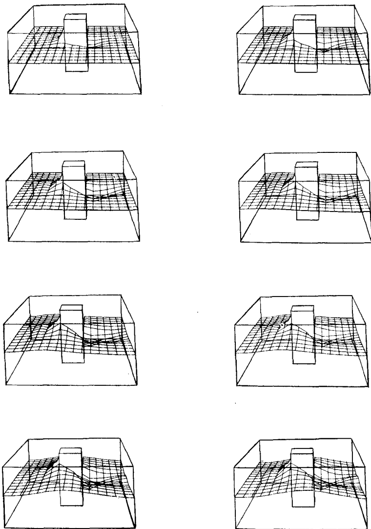
Рис. 7.6. Последовательность кадров кинофильма о нестационарном обтекании препятствия. В изометрической проекции показана поверхность воды вблизи свая квадратного сечения. Расчет проведен в Лос-Аламосской лаборатории У. Николсом, использовавшим трехмерный алгоритм метода маркеров и ячеек (данные любезно предоставлены С. Хёргом из Лос-Аламосской лаборатории).
