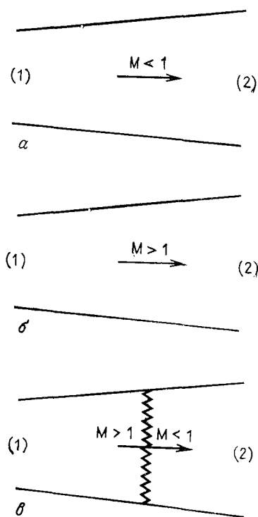
Рис. 3.28. Парадокс, связанный с влиянием граничных условий на выходной границе потока; квазиодномерное течение невязкой жидкости. a — полностью дозвуковое течение; б — полностью сверхзвуковое течение; в — течение со сверхзвуковой скоростью во входном сечении и с дозвуковой скоростью в выходном сечении.
