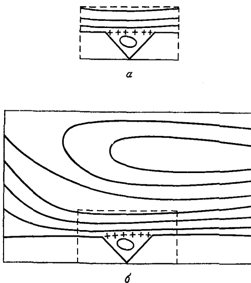
Рис. 7.2. Картина линий тока при ошибочном расчете течения над V-образной выемкой. Крестиками показана разделяющая линия тока. a — фрагмент поля течения, б — все поле течения.
