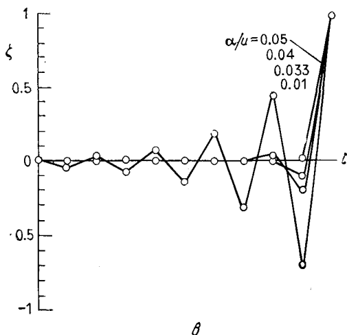
Рис. 3.27. Аналитические и конечно-разностные решения стационарного линейного модельного уравнения 0 = -u (\partial \xi / \partial x) + \alpha (\partial^2 \xi / \partial x^2) , включающего конвективный и диффузионный члены; \xi(0) = 0 , \xi(1) = 1 , u = \text{const} . Решение с центральными конечными разностями, \Delta x = 1/10 . Сеточное число Рейнольдса Re_c = u \Delta x / \alpha . а — аналитические решения; б — конечно-разностные решения при Re_c \leq 2 ; в — конечно-разностные решения при Re_c \geq 2 .
