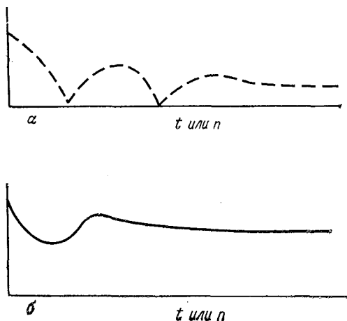
Рис. 3.32. Зависимость от времени некоторых характеристик решения задачи о течении вязкой жидкости в области с заданными входной и выходной границами. a — по оси ординат отложена величина \max_{i,j} |\zeta_{i,j}^{n+1} - \zeta_{i,j}^n| ; b — по оси ординат отложена величина \zeta_{i,j}^n или \sum_{i,j} |\zeta_{i,j}^n| .
