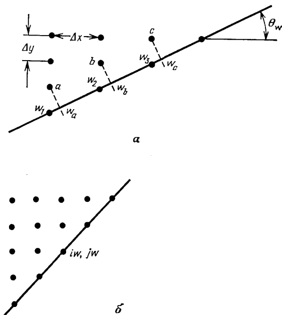
Рис. 3.23. Определение значения вихря на стенке, не параллельной оси x . a — произвольный угол наклона стенки \theta_w , б — угол наклона стенки \theta_w = 45^\circ .
