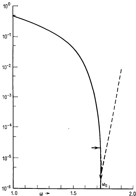
Рис. 3.16а. Поведение итераций в методе последовательной верхней релаксации в зависимости от величины параметра релаксации \omega . Размер сетки I=J=21 , \Delta x=\Delta y , оптимальное значение \omega в этом случае \omega_0=1.7295 .
