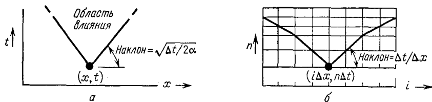
Рис. 3.9. Область влияния точки (x, t) для уравнения (3.118) гиперболического типа. а — область влияния для дифференциального уравнения; б — область влияния для конечно-разностного уравнения.
