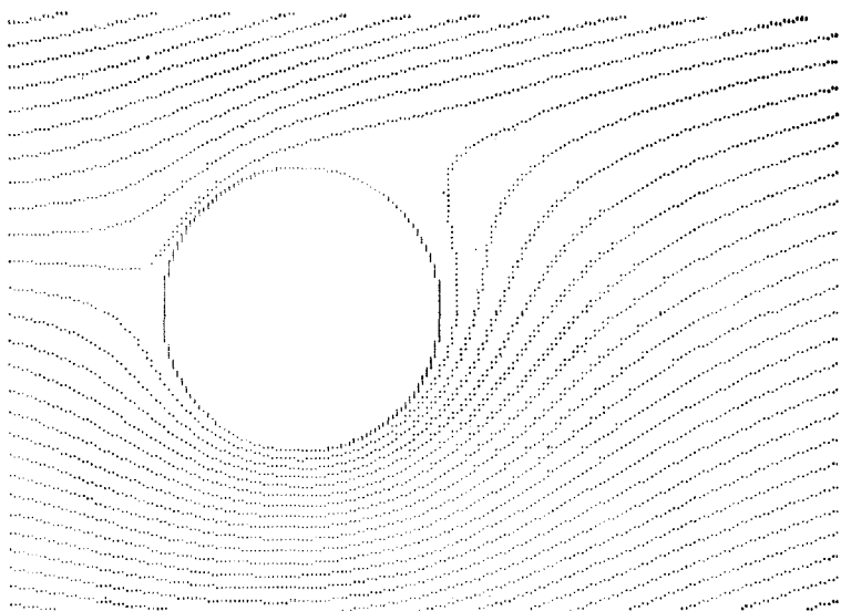
Рис. 7.8а. Линии тока при нестационарном обтекании кругового цилиндра для наблюдателя, движущегося вместе с обтекаемым телом (система координат связана со стенками аэродинамической трубы). Из работы Томана и Шевчика [1966].
