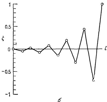
Рис. 3.26. Точное решение уравнения 0 = -u (\delta \zeta / \delta x) + \alpha (\delta^2 \zeta / \delta x^2) . Решение с центральными конечными разностями, \Delta x = 1/10 , \zeta_1 = 0 , \zeta_{11} = 1 , u = \text{const} . а: \alpha/u = 1 , Re = 1 , Re_c = 0.1 ; б: \alpha/u = 0.01 , Re = 100 , Re_c = 10 .
