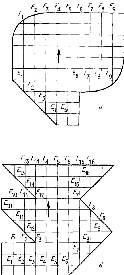
Рис. 3.19. Метод расчета распространения вектора ошибки для областей не-регулярной формы. E_m — составляющие вектора начальной ошибки, F_l — составляющие вектора конечной ошибки. Стрелкой указано направление продвижения расчета.
