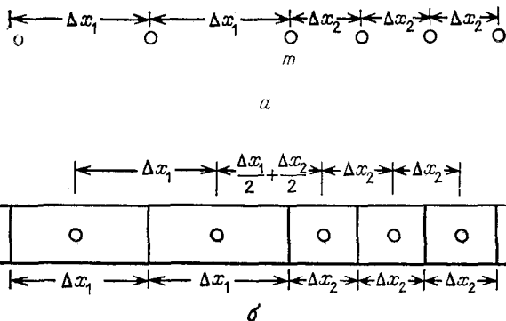
Рис. 6.1. Изменение шага сетки по пространству. a — однократное изменение расстояния между узлами сетки, б — однократное изменение размера ячейки.
