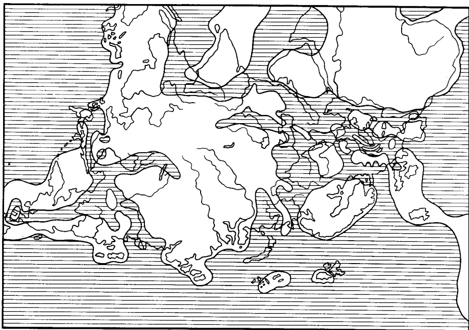
Рис. 45. Схематическая палеогеографическая карта верхнеюрского времени (по Терье, 1952)
