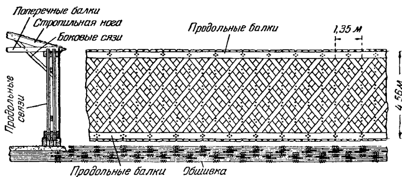
Рис. 101. Мост Тауна.
