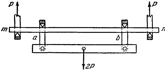
Рис. 88. Прибор Вёлера для статических испытаний на изгиб.
