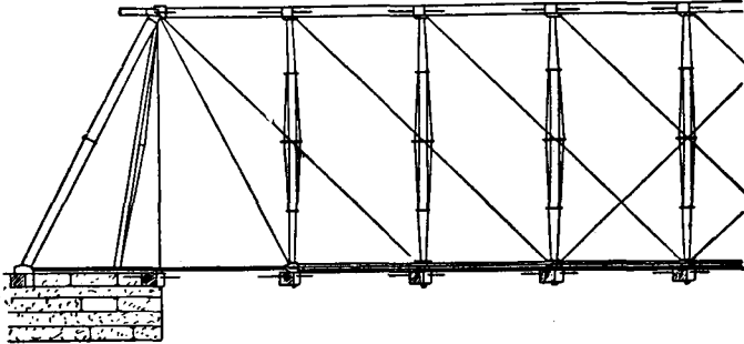
Рис. 104. Мост Уиппла на железной дороге Ренселер—Сарагога.
