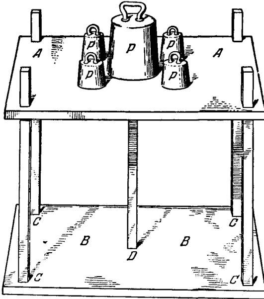
Рис. 34. Установка Мусшенбрука для испытаний на сжатие.
