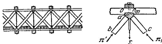
Рис. 102. Ферма Гау.
