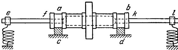
Рис. 85. Машина Вёлера для усталостных испытаний.
