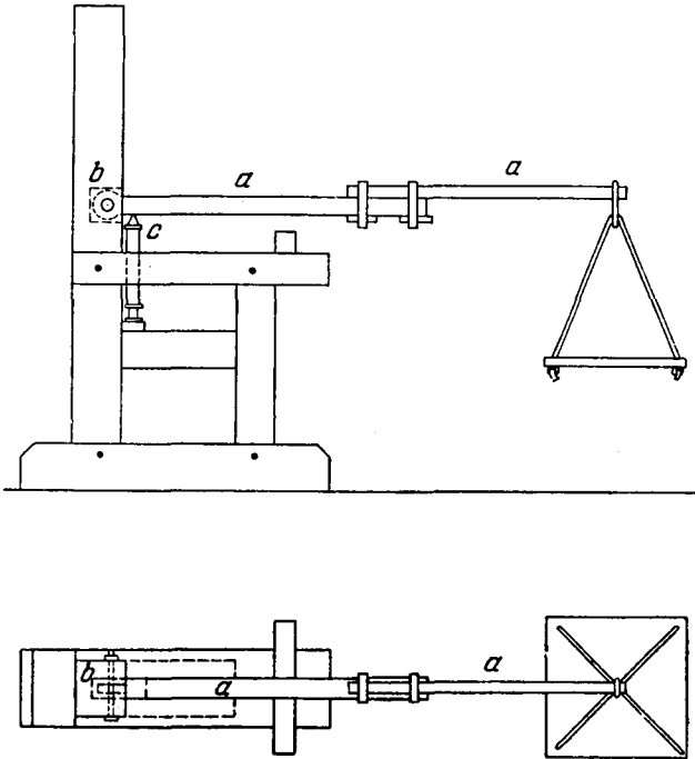
Рис. 35. Испытательная машина Готэ.
