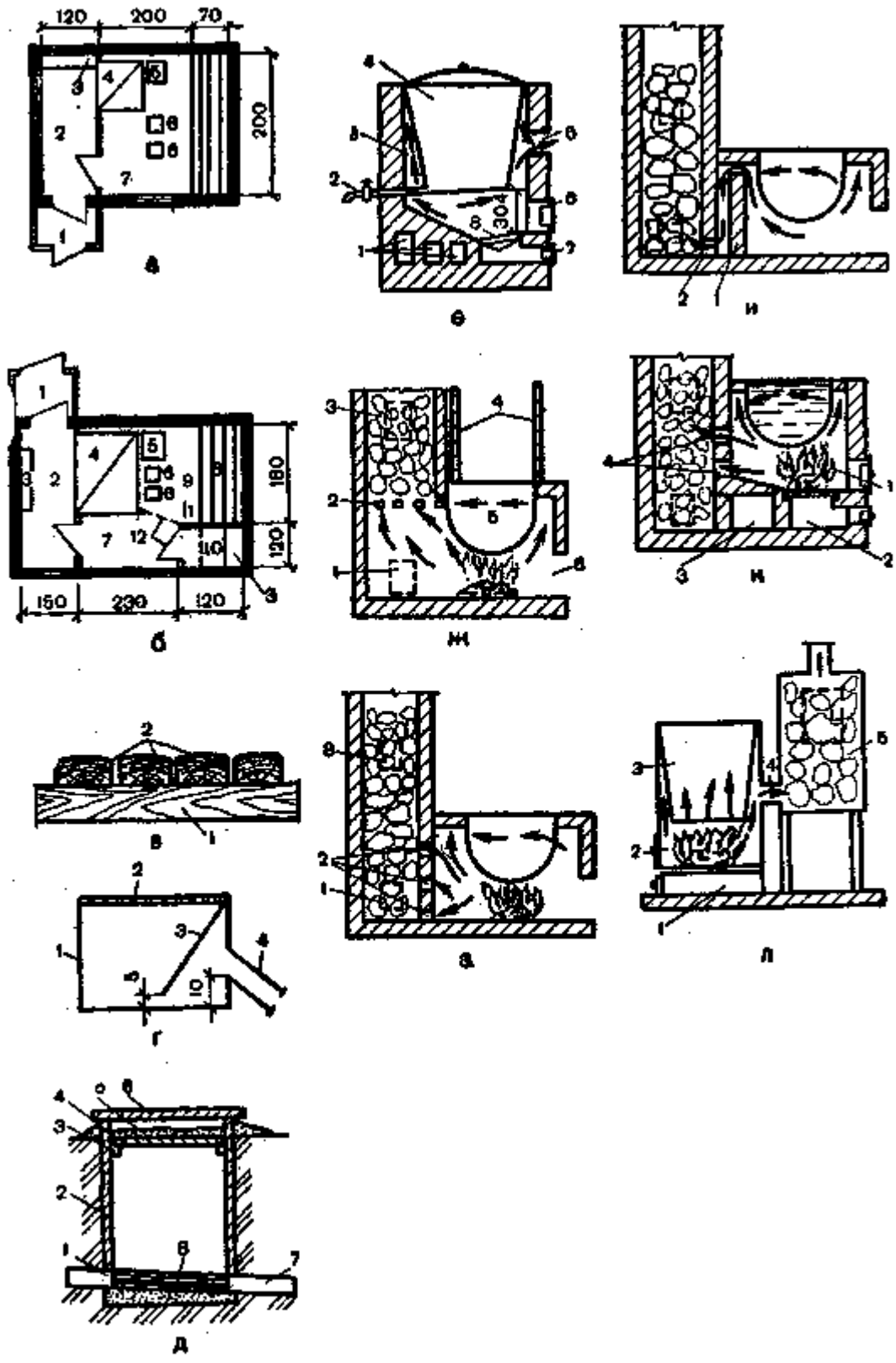
Рис. 227. Баня (размеры в см и мм): а — простая баня: 1 — тамбур; 2 — предбанник; 3 — скамья; 4 — печь; 5 — бак для холодной воды; 6 — табуреты; 7 — моечная; б — улучшенная баня с парилкой: 1 — тамбур; 2 — предбанник; 3 — скамья; 4 — печь; 5 — бак для холодной воды; 6 — табуреты; 7 — моечная; 8 — полка; 9 — парильня; 10 — раздевалка; 11 — стенка, отделяющая парильню от раздевалки; 12 — дверь; в — конструкция пола: 1 — лага; 2 — доски или бруски; г — трап: 1 — коробка; 2 — решетка; 3 — пластина; 4 — труба; д — смотровой колодец: 1 — труба входная; 2 — стенка; 3 — брусоч; 4 — внутренняя крышка; 5 — засыпка утепляющая; 6 — наружная крышка; 7 — труба выходная; 8 — бетонный лоток; е — печь для отопления и нагрева воды: 1 — каналы для выхода тепла; 2 — кран; 3 — пазуха для горячих газов; 4 — котел; 5 — канал для отвода газов в трубу; 6 — топочная
