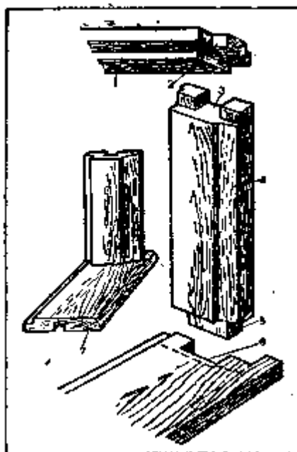
Рис. 59. Устройство коробки: 1 — вершник; 2, 5 — шипы; 3, 6 — проушина; 4 — стояк; 7 — слезник
