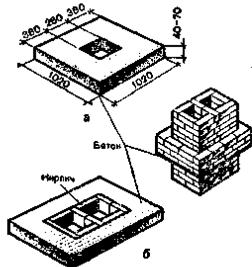
Рис. 197. Устройство железобетонной плиты под разделку:
