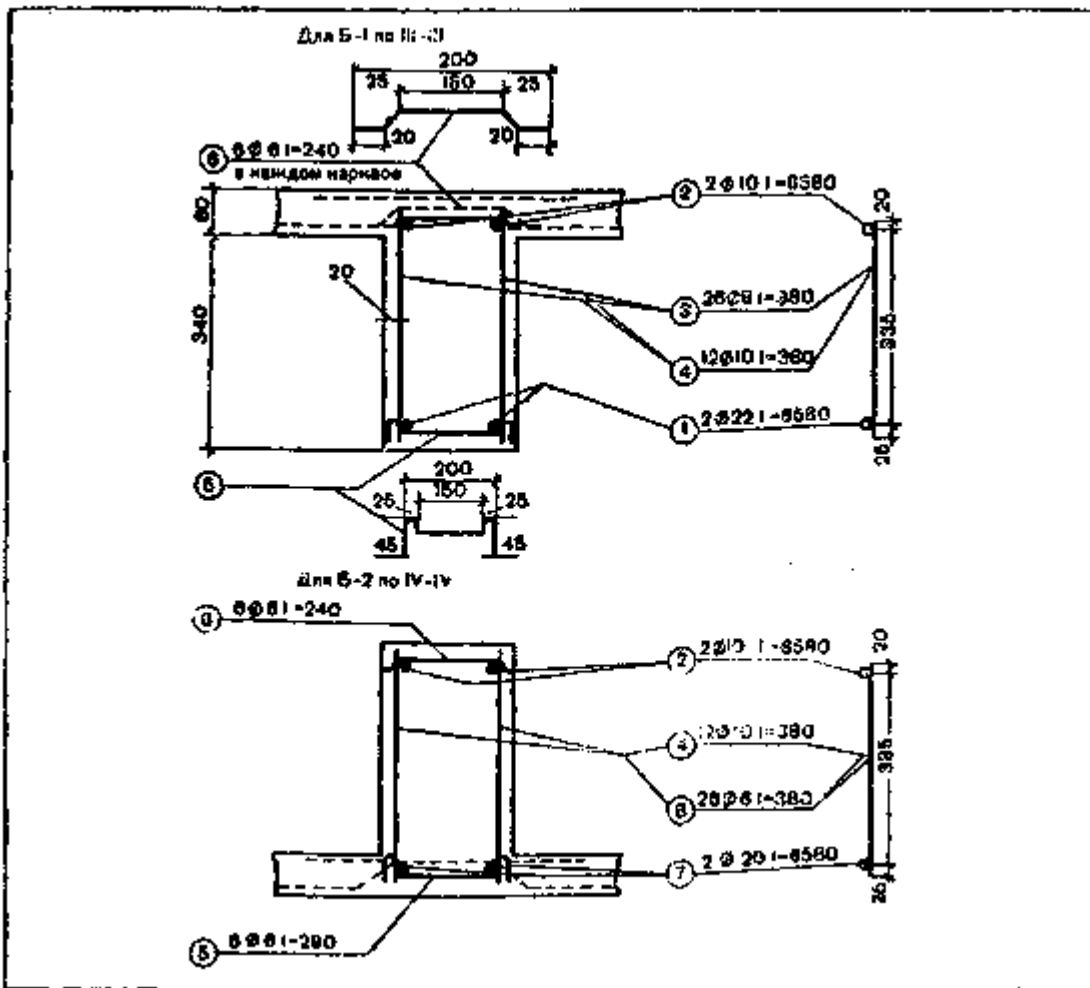
Рис. 139. Разрез сварного каркаса двух балок по толщине
