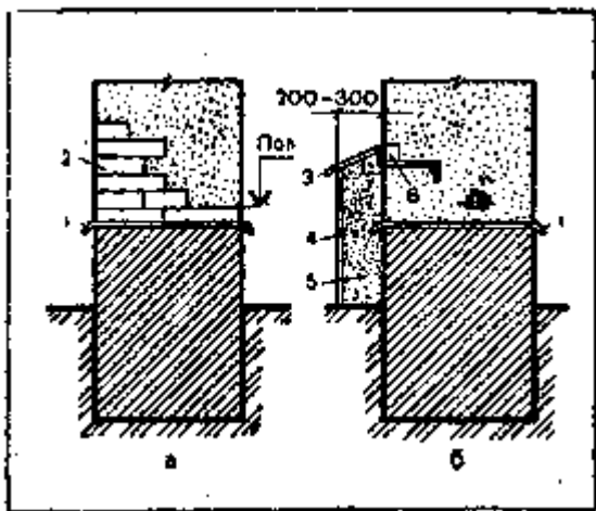
Рис. 88. Цоколи:
