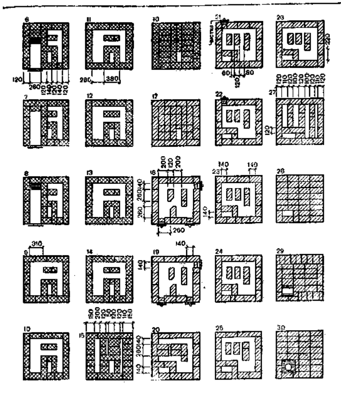
Рис. 202. Отопительная печь конструкции Н. С. Подгородникова (типа двухъярусный колпак): 1,2 — чистка; 3 — гидроизоляция; 4 — фундамент
