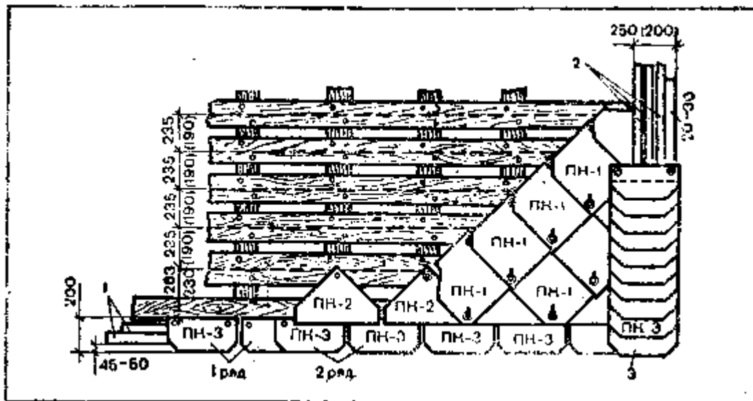
Рис. 164. Покрытие кровли с фризом: 1 и 2 — уравнительные рейки; 3 — фриз
