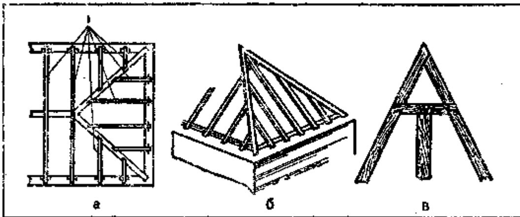
Рис. 155. Сопряжение отдельных частей стропильных ног: а — план; б — сопряжение стропильных ног; в — вариант сопряжения сковороднем; нарожники
