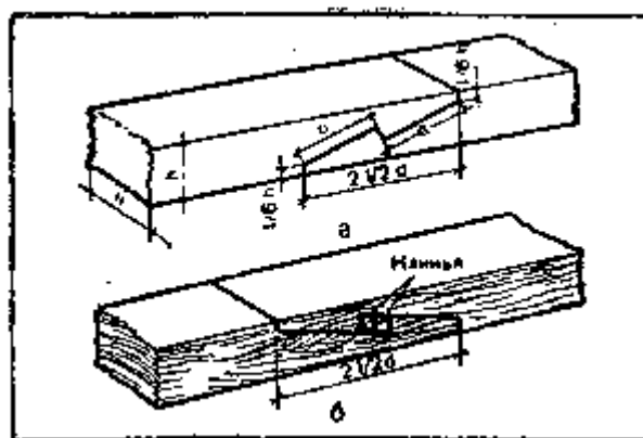
Рис. 45. Сращивание брусков косым замком: a — косой замок из брусков; b — косой замок с натяжным клином
