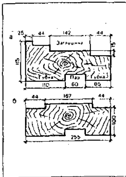
Рис. 55. Бруски коробок: а — для переплетов, открывающихся внутрь; б — для переплетов, открывающихся в разные стороны
