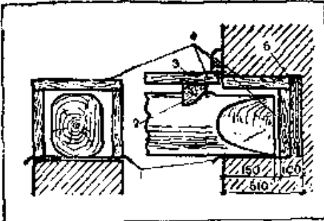
Рис. 132. Заделка концов деревянных балок междуэтажных перекрытий
