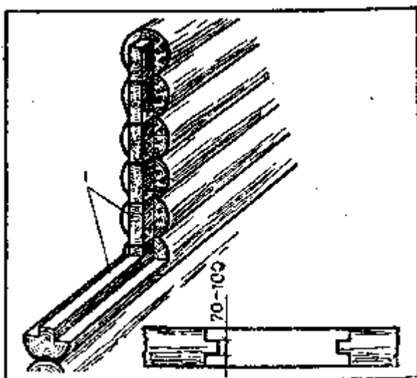
Рис. 58. Подушка с подоконной доской: 1 — гребень
