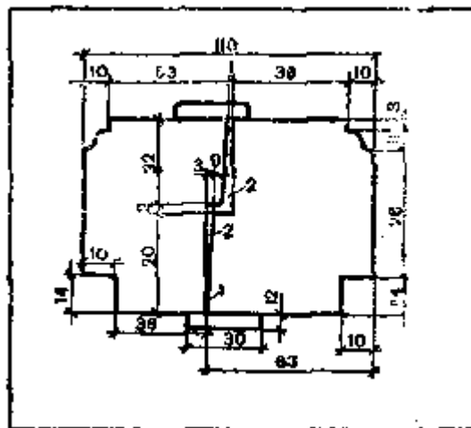
Рис. 71. Притвор створок
