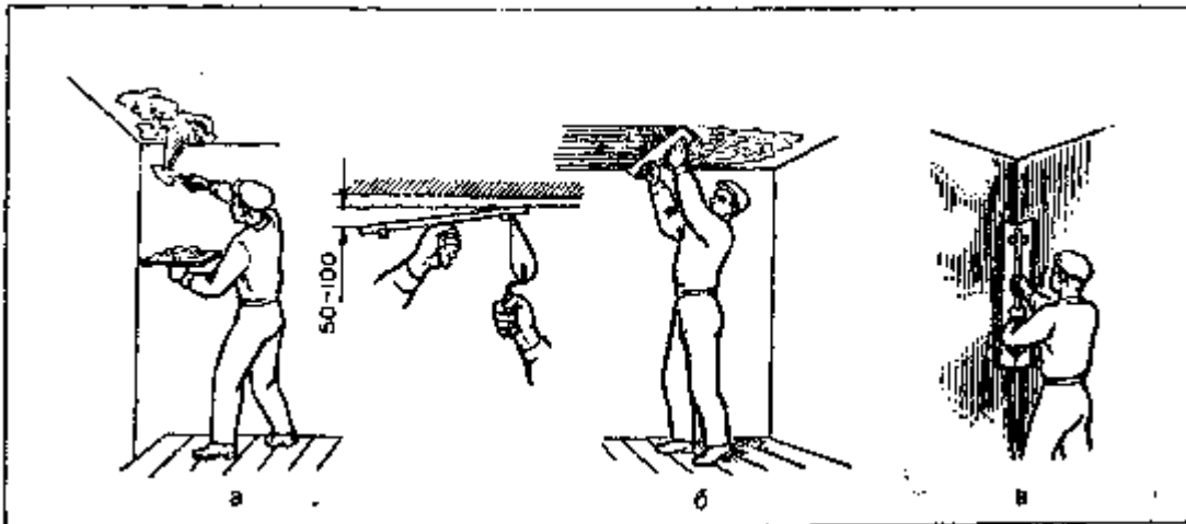
Рис. 215. Оштукатуривание потолка: а — нанесение раствора; б — разравнивание раствора соколом и полутерком; в — натирка лужга на стенах
