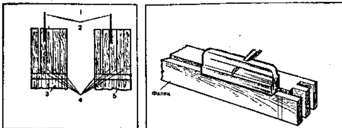
Рис. 65. Порядок запиловки шипов и проушин:
