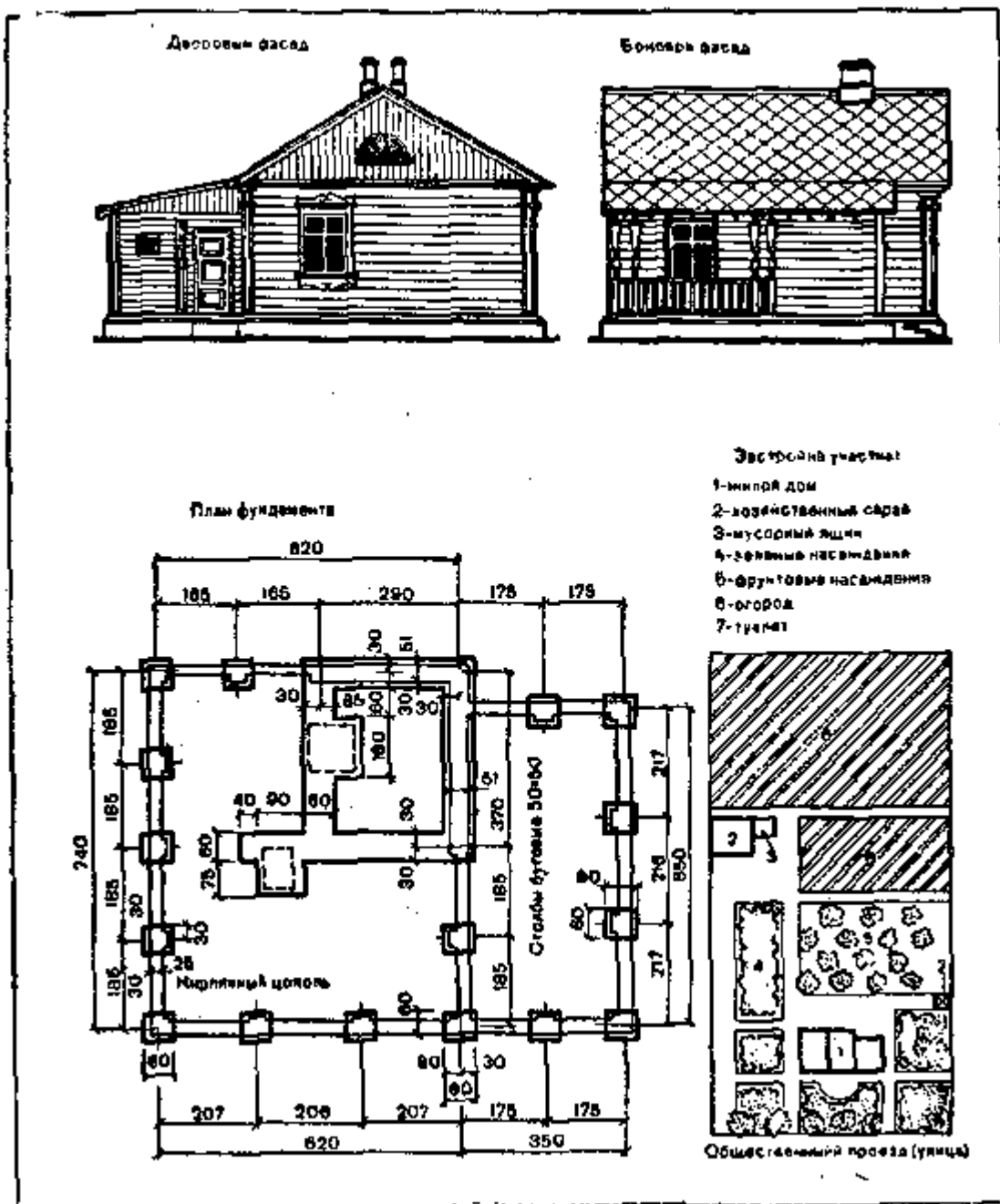
Рис. 2. Дворовой и боковой фасады, планы фундамента и участка (размеры в см)
