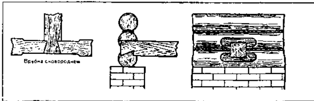
Рис. 118. Врубка балок в деревянные рубленые стены, укладываемые на сплошном цоколе
