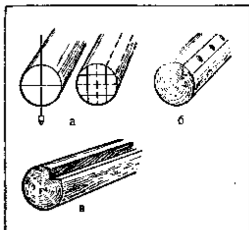
Рис. 37. Выборка четверти в бревне: а — разметка четверти; б — устройство насечек; в — четверть
