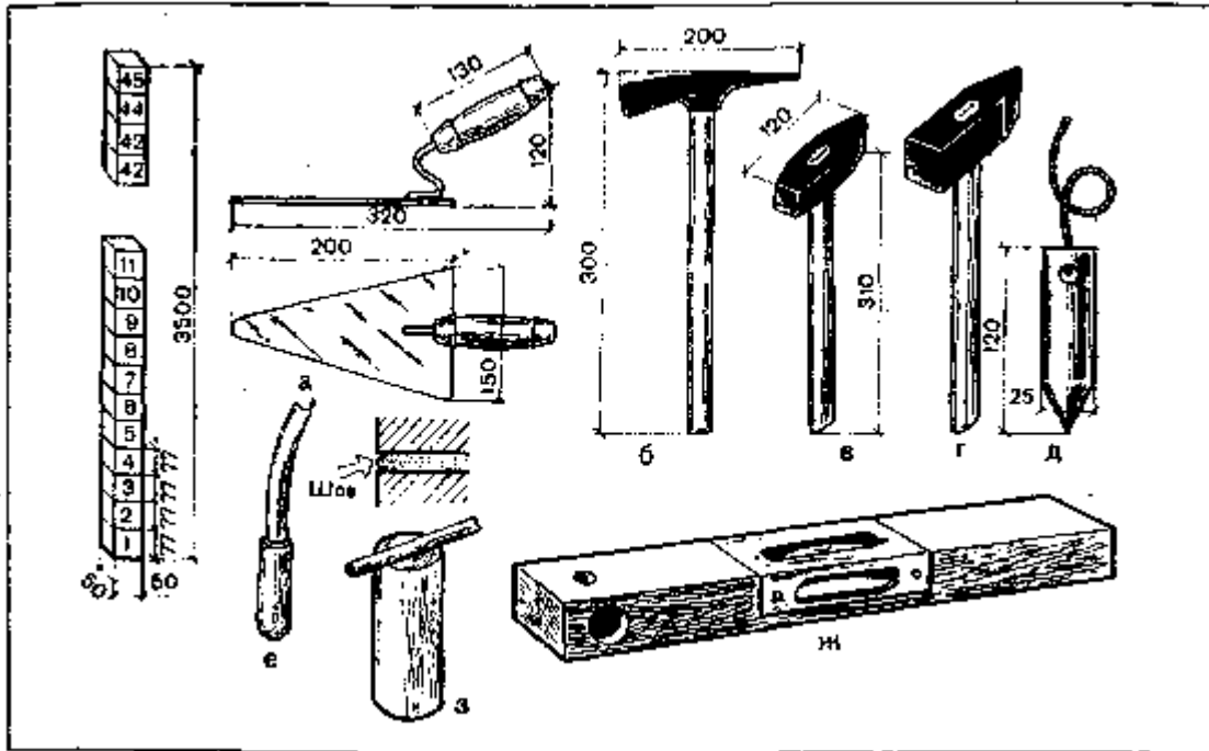
Рис. 22. Инструменты для выполнения каменных работ: кельма; б — молоток-кирочка; в — молоток; г — кувалда остроносая; д — весок; е — расшивка; ж — уровень; з — трамбовка
