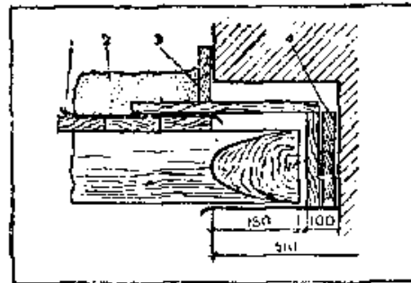
Рис. 133. Заделка концов деревянных балок в чердачном перекрытии в стену толщиной в два кирпича: 1 — толь; 2 — засыпка; 3 — доска толщиной 25 мм; 4 — войлок в 3 слоя
