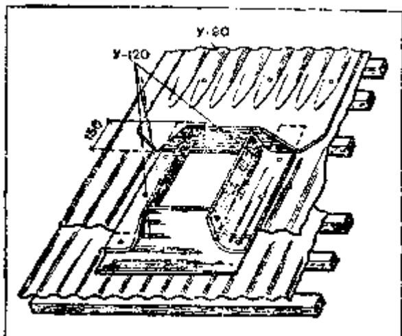
Рис. 170. Устройство воротника вокруг дымовой трубы из уголковых элементов
