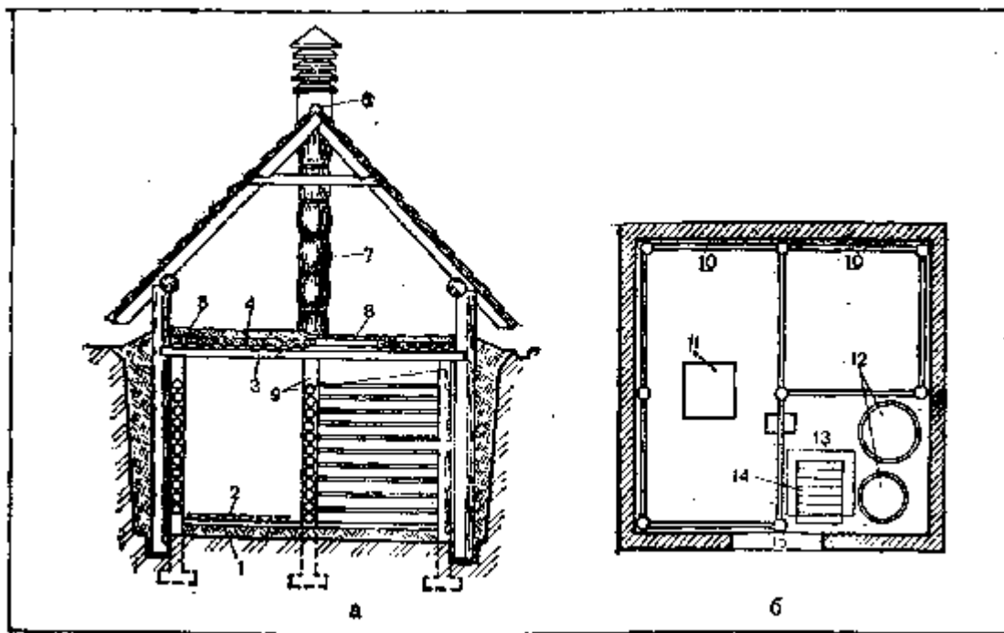
Рис. 10. Погреб-ледник:
