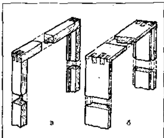
Рис. 53. Оконные коробки для каменных, кирпичных и других зданий:
