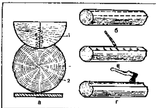
Рис. 39. Разметка и выборка овального паза в бревне: а — лекало для паза; б — отбивка ниток; в — насечки по пазу; г — готовый паз; 1 — лекало; 2 — бревно
