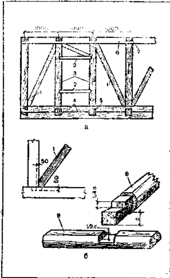
Рис. 104. Конструкция каркаса и его детали: a — общий вид; b — врубка подкоса; 1 — подкос; 2 — ригель; 3 — стойка; 4 — нижняя обвязка; 5 — половая балка; 6 — верхняя обвязка; 7 — потолочная балка; 8 — балка; 9 — обвязка
