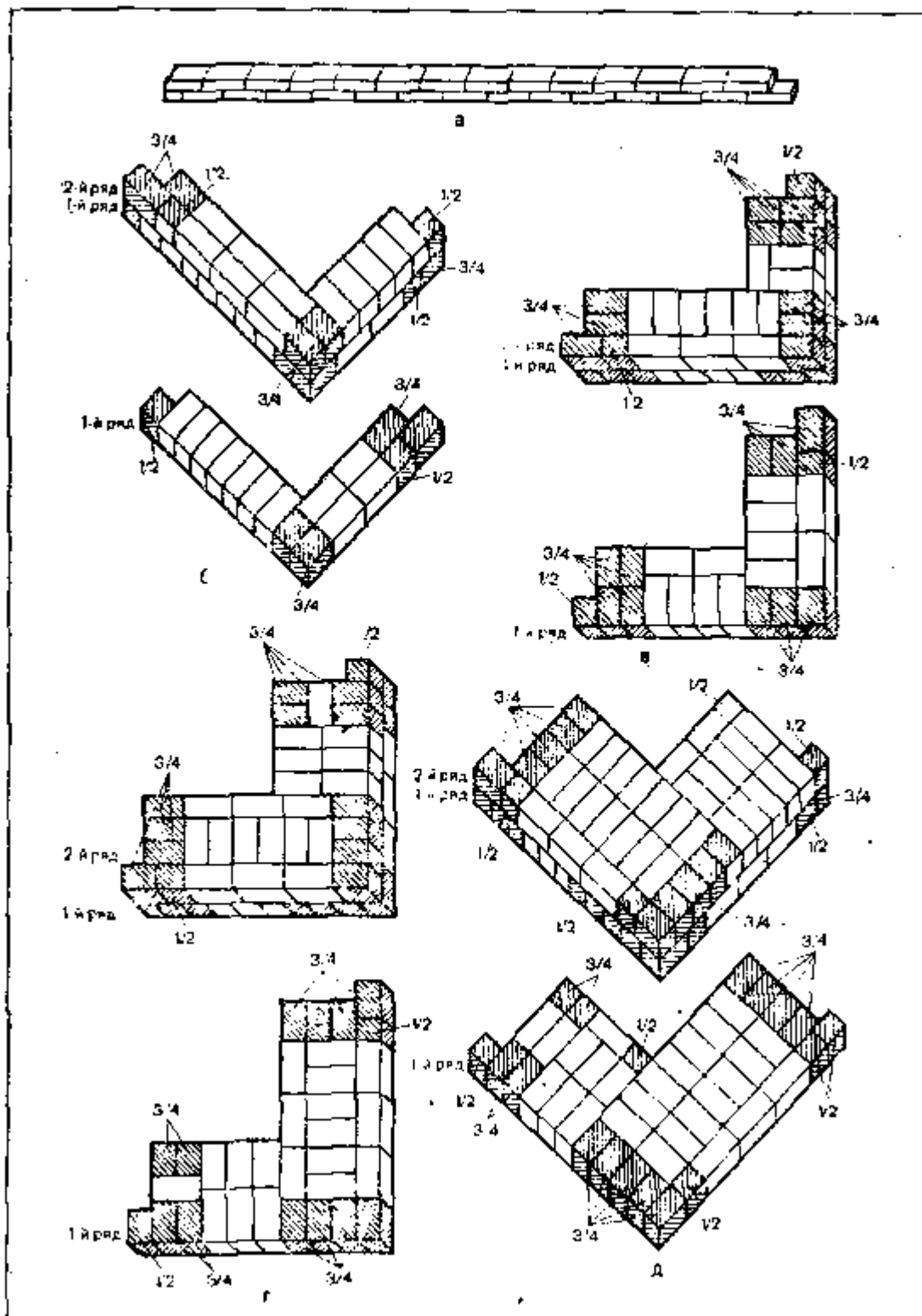
Рис. 24. Кирпичная кладка стен различной толщины: a — в 1/2 кирпича; б — в 1 кирпич; в — в 1 1/2 кирпича; г — в 2 кирпича; д — в 2 1/2 кирпича
