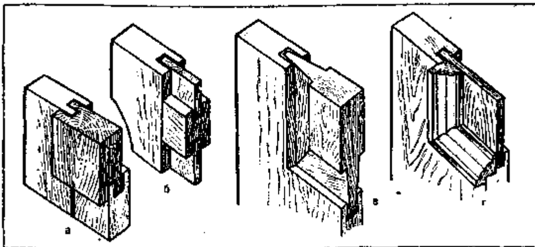
Рис. 76. Типы филенок: а — наплавная; б — плоская; в — с фигурейми; г — с окладными калевками
