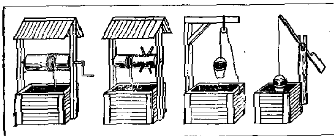
Рис. 16. Деревянные колодцы:
