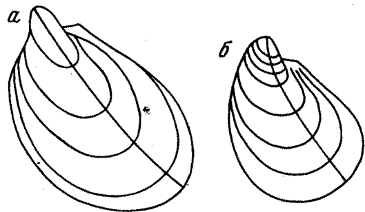
Рис. 38. Изменчивость очертаний (индивидуальная и в онтогенезе) правых (а – № 555/197, б – № 555/198, в – № 555/199, г – № 555/200, д – № 555/151, е – № 555/201) и левых (ж – № 555/124, з – № 555/125, и – № 555/126, к – № 555/127, л – № 555/130, м – № 555/131, н – № 555/132) створок Buchia tenuistriata . Курвоидный тип онтогенеза. Выборка правых створок из единой конкреции серых песчаников с р. Пижмы, обн. 10, осыпь, совместно с Aulacostephanus cf. eudoxus . Выборка левых створок из единой фосфоритовой конкреции с р. Пижмы, обн. 13, сл. 1. Слой с Aulacostephanus cf. eudoxus . Верхний кимеридж
