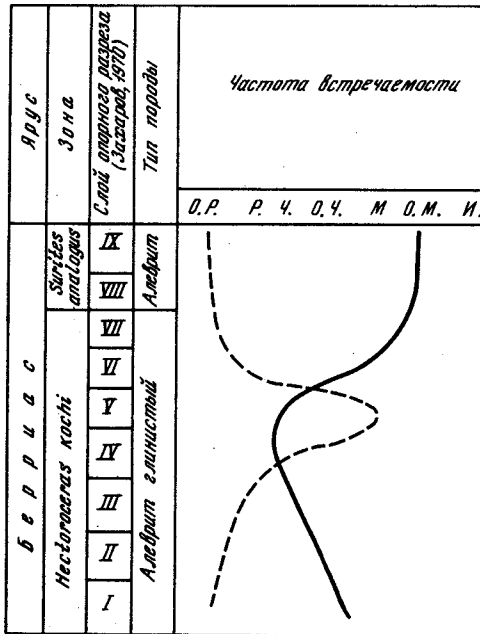
Рис. 81. Кривые, отражающие биотопическое исключение бухий (сплошная линия) и иноцерамов (пунктир) в берриасе на р. Боярке, Хатангская впадина, север Сибири
