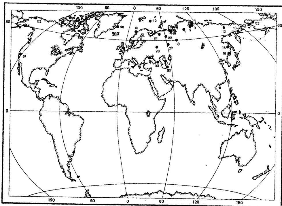
Р и с. 66. Местонахождения Buchia volgensis (Lah.). Условные обозначения см. рис. 30
