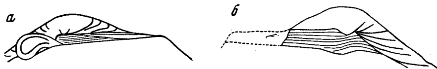
Р и с. 26. Схема строения лигаментной площадки правой (а) и левой (б) створок Praebuchia orientalis gen. et sp. nov. Эти же экземпляры изображены на рис. 24б
