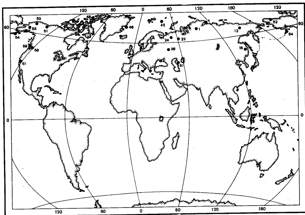
Р и с. 62. Местонахождения Buchia okensis (Pavl.) Условные обозначения см. рис. 30
