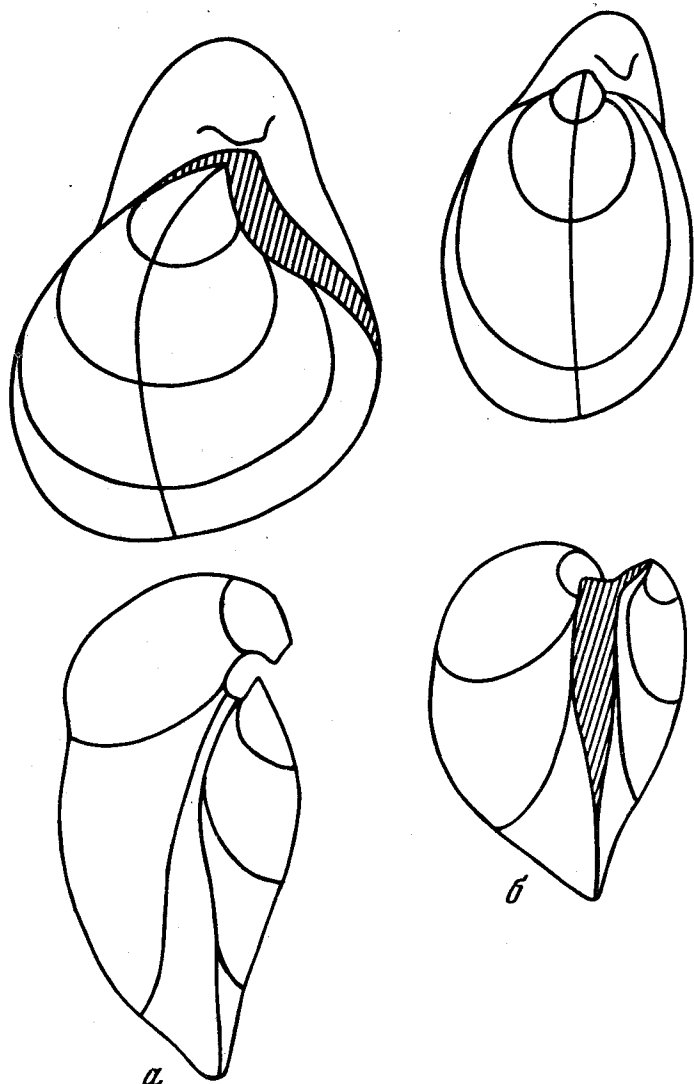
Р и с. 76. Изменение очертаний раковины двух форм с округленной (а) и весьма высокой правой створкой Buchia crassicollis в онтогенезе а — № 546/134 (фото на табл. LX, фиг. 70б,в); б — № 555/632 (фото на табл. LX, фиг. 4)
