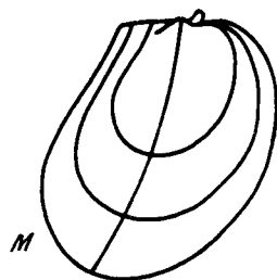
Р и с. 12. Курвоидный онтогенез левых (а-е) и правых (ж-м) створок Buchia mosquensis . Выборки из ископаемой популяции
