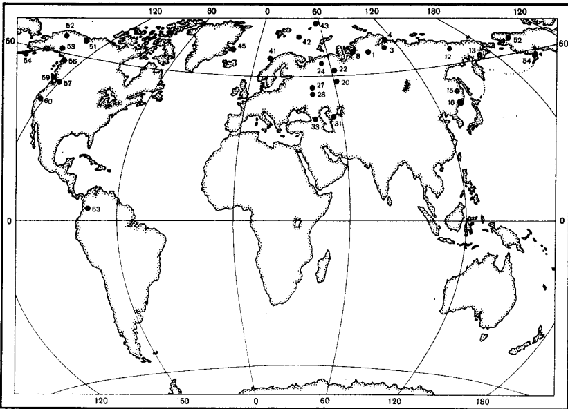
Р и с. 101. Местонахождения рода Vuchia в основании берниаса (зона Nectroceras kochi ) Условные обозначения см. рис. 30
