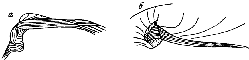
Р и с. 56. Схема строения замка правой створки Buchia terebratuloides (Lah.). № 555/376
