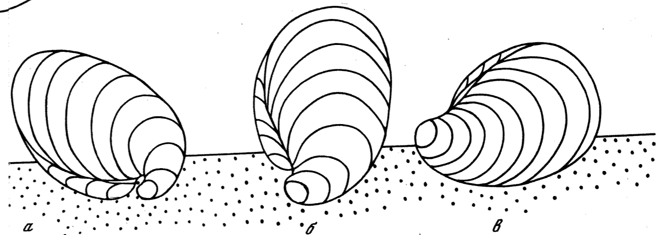
Р и с. 78. Положение на грунте Buchia keyserlingi (реконструкция) а — вид со стороны заднего края, б — вид со стороны макушек, в — вид со стороны левой створки
