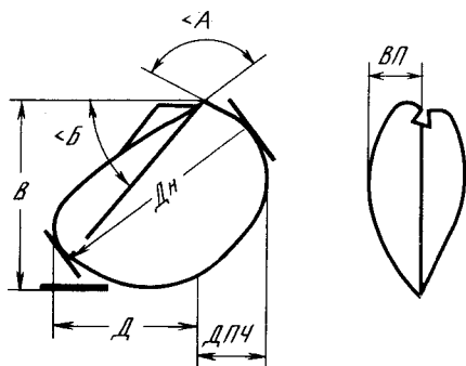
Р и с. 4. Схема замеров раковин бухий
