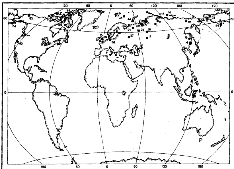
Р и с. 106. Местонахождения рода Buchia в верхнем валанжине Условные обозначения см. рис. 30
