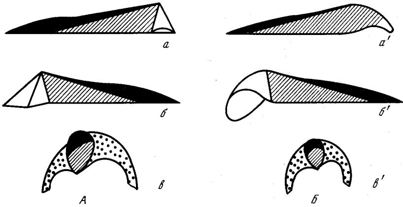
Р и с. 6. Схема строения и положения лигамента (реконструкция) у Buchia (А) и Praebuchia (Б). Лигаментная площадка левой (а, а') и правой (б, б') створок и положение вещества связки (вв') — поперечное сечение: пластинчатой (зачернено) и волокнистой (заштриховано); точками показана раковина в сечении
