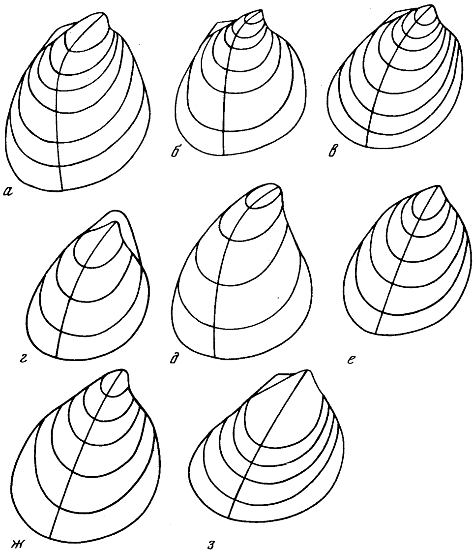
Р и с. 14. Инверсионный онтогенез и изменчивость очертаний правых створок Buchia inflata . Север Сибири, р. Попигай, обн. 8, слой 8 (а – № 555/502, б – № 555/503, в – № 555/504, г – № 555/505), обн. 12, осьшь (д – № 555/506, е – № 555/507, ж – № 555/508, з – № 555/509). Слой переходные между берриасом и валанжином
