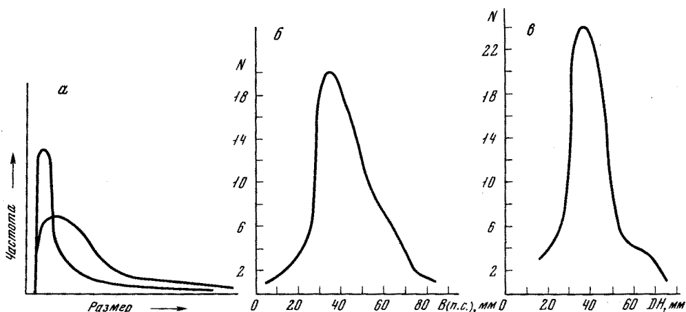
Р и с. 3. Размерно-частотные кривые распределения экземпляров в ископаемых популяциях а — теоретическая (из Boucot, 1953, стр. 28, фиг. 5), б—в — природные: б — Buchia okensis . Север Сибири, р. Боярка, обн. 16, слой 5. Берриас, зона Nectoceras kochi , слой V опорного разреза неокома; в — B. jaskovi , там же, граница слоев 5—6. Интервал мощи. 2,5 м между зонами N. kochi и Surites analogus
