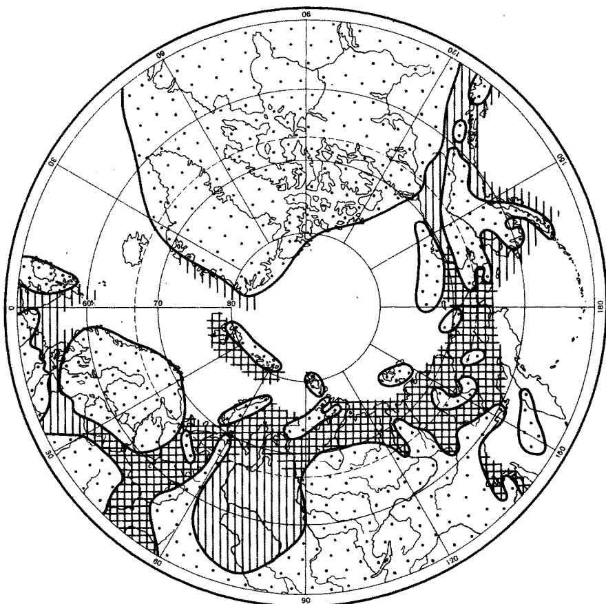
Р и с. 98. Распространение рода Buchia в средневолжское время. Двойная штриховка – поселения с высокой популяционной плотностью, одинарная – с низкой
