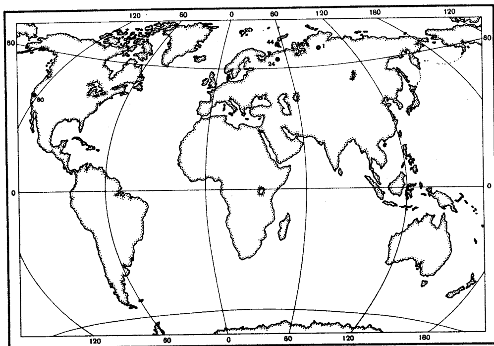
Р и с. 54. Местонахождения Buchia obliqua (Tull.) Условные обозначения см. рис. 30
