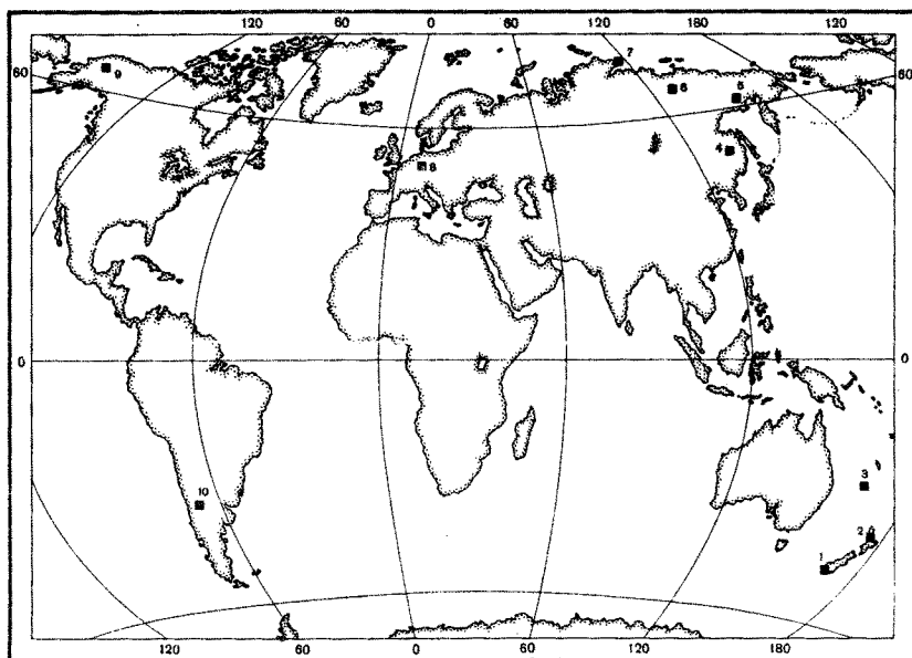
Р и с. 88. Местонахождения рода Otapiria в отложениях нижнего лэйаса
