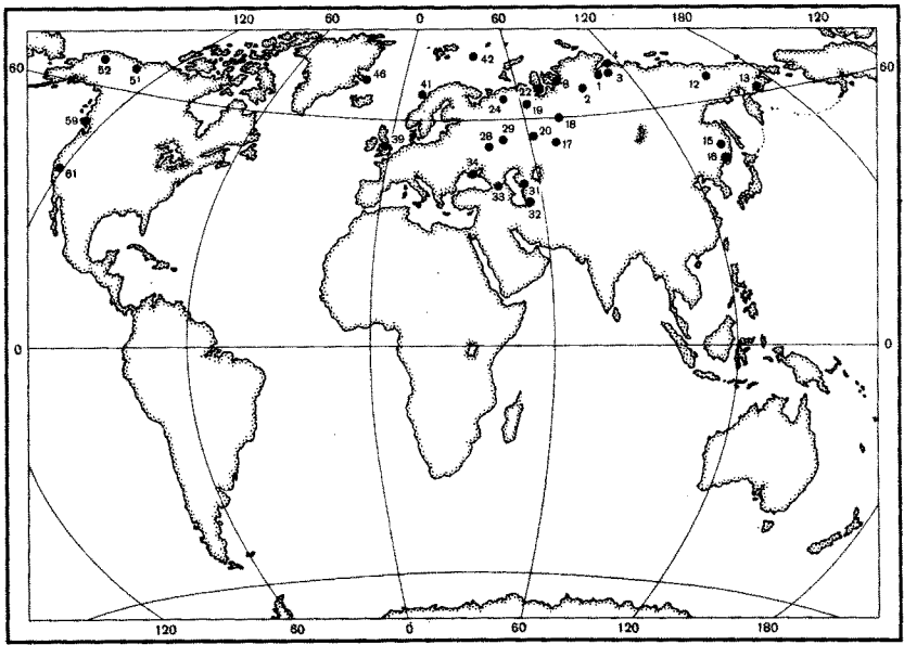
Р и с. 103. Местонахождения рода Buchia в верхней части берриаса (зоны Surites analogus и Bojarkia mesezhnikowi )
