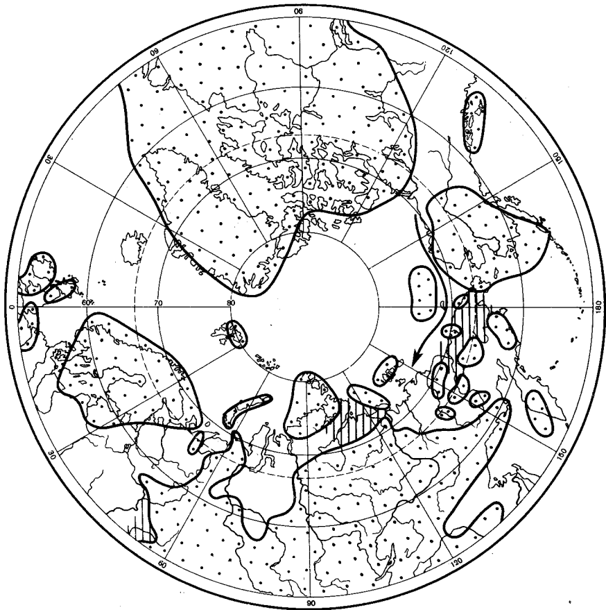
Р и с. 91. Распространение рода Praebuchia в келловее Евразии. Стрелкой показан предполагаемый путь иммиграции наиболее ранних бухид. Одинарная штриховка – поселения с низкой популяционной плотностью. Крапом показана суша
