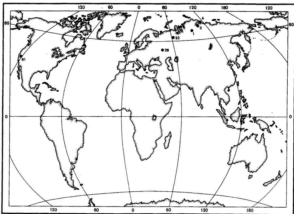
Р и с. 63. Местонахождения Buchia jasikovi (Pavl.) Условные обозначения см. рис. 30
