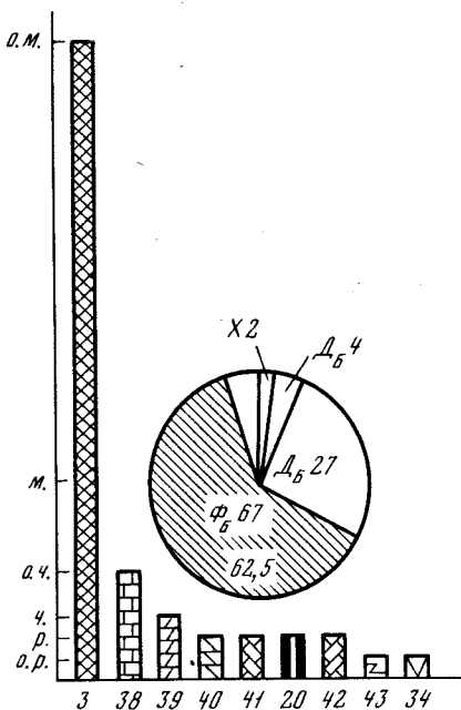
Р и с. 86. Структура среднесублиторального бухиевого сообщества. Бухии доминировали (62,5% от ФБ). Реконструкция по ориктоценозу слоя V, интервал 0,0–0,5 м, зона Nectoceras kochi , берриас, р. Боярка, север Сибири (Граница юры и мела, 1972, с. 25)
