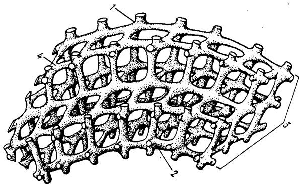
Рис. 2. Правильная диктиональная конструкция интерваллюма, заполненная стерженьками в трех взаимно перпендикулярных направлениях — род Duliscosyathus Debr., реконструкция (рисунок В.Д. Фомина, передан им специально для настоящей работы)
