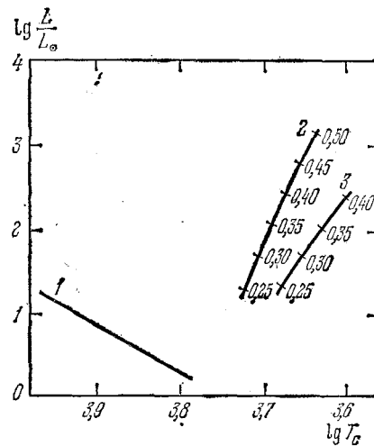
Рис. 12.6. Теоретические треки звезды с M = 1,2M_{\odot} с разным содержанием тяжелых элементов, 1 — главная последовательность, 2 — звездное население II типа, 3 — население I типа.
