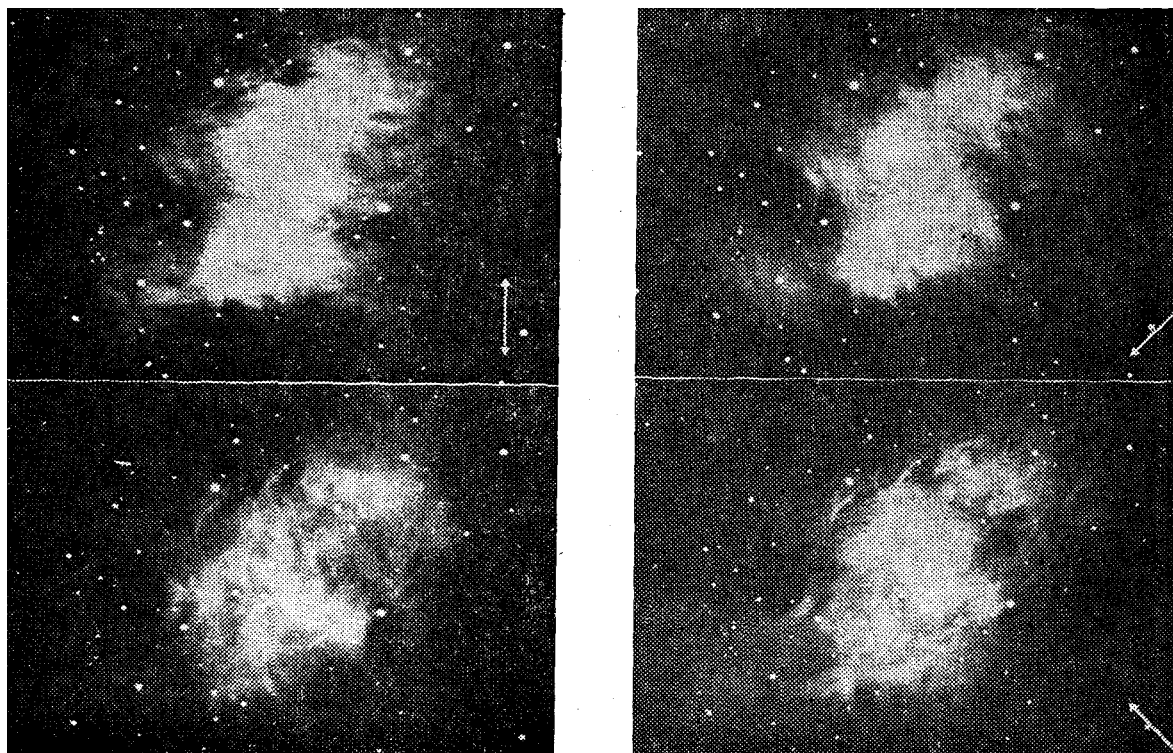
Рис. 17.7. Фотографии Крабовидной туманности через различно ориентированные поляриды.
