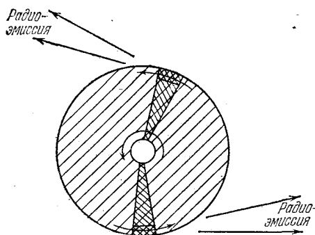
Рис. 20.1. Модель пульсара по Голду.
