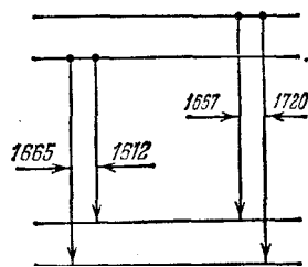
Рис. 3.2. Схема, поясняющая образование четырех радиочастот молекулы OH.
