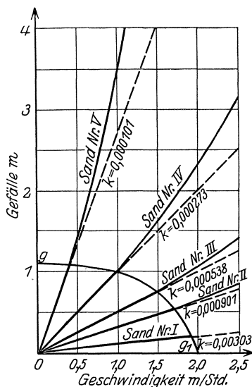
Abb. 12. Angenäherte Gültigkeitsgrenze des Darcyschen Gesetzes auf Grund der Piefkeschen Versuche nach E. Prinz.
