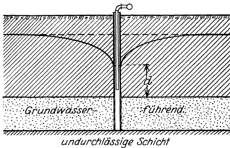
Abb. 8. Artesischer Brunnen.
