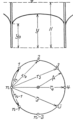
Abb. 22. Mehrbrunnenanlage von kreisförmigem Grundriß mit einer Brunnenstaffel in Betrieb.
