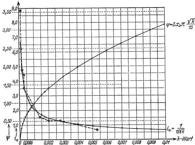
Abb. 15. Beziehungen zwischen dem Grenzgefälle i_0 , dem Fassungswert \varphi und dem k -Wert unter Zugrundelegung der Formeln i_0 = \frac{1}{15\sqrt{k}} und \varphi = 2x_0\pi \frac{\sqrt{k}}{15} .
