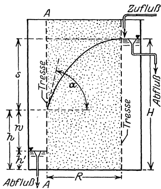
Abb. 13. Versuchseinrichtung zur Beobachtung des Grenzgefälles des Grundwasserspiegels.
