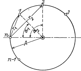
Abb. 23. Beziehungen zwischen den Strahlen r und dem Brunnenhalbmesser A sowie dem Zentriwinkel \alpha .
