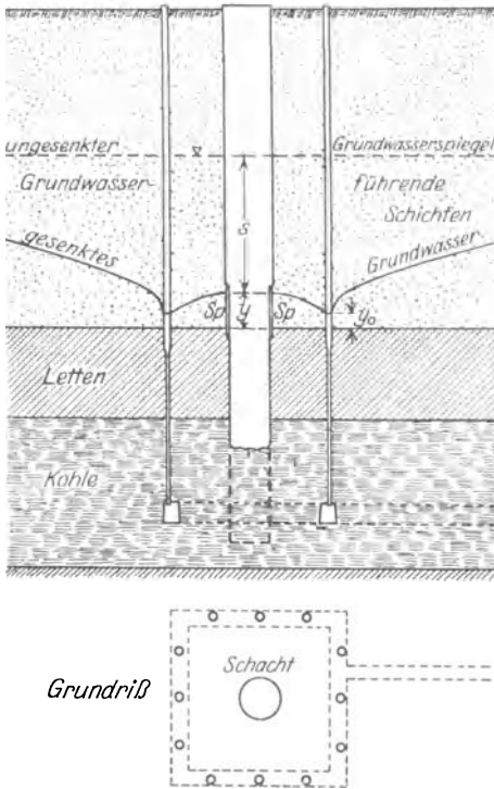
Abb. 11. Sickerbrunnenanlage der Matador-Bergbau-gesellschaft in Senftenberg (Nieder-Lausitz).
