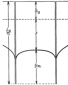
Abb. 38. Bohrtiefe der Brunnen.
