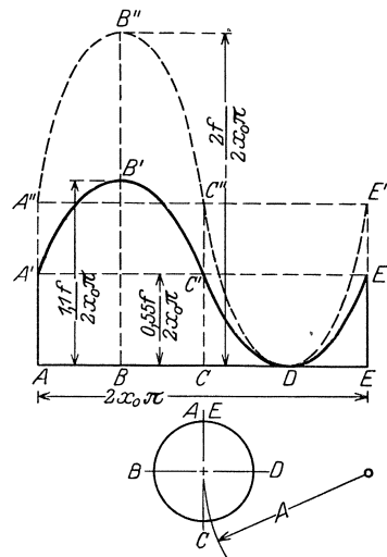
Abb. 33. Drosselung des Fassungsvermögens bei zu geringem Brunnenabstand, dargestellt durch Auftragung der auf den laufenden Zentimeter des abgewickelten Brunnumfanges entfallenden Sickermenge.
