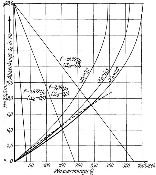
Abb. 19. Absenkung s_0 in einem Brunnen von bestimmtem Halbmesser x_0 in Abhängigkeit von der Wasserentnahme Q nach Kyrieleis, jedoch unter Berücksichtigung des durch das Brunnenfassungsvermögen gegebenen Geltungsbereichs.
