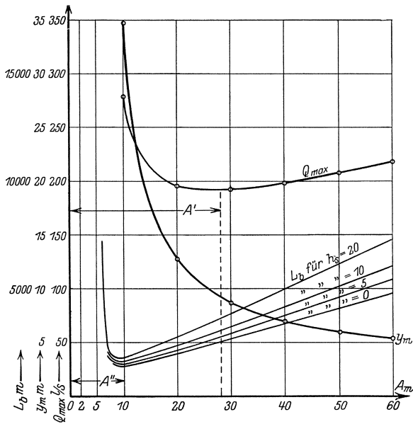
Abb. 37. Abhängigkeit des größten zu bewältigenden Wasserandranges Q_{max} , der günstigsten Eintauchtiefe y_m (gerechnet von der Absenkung im Mittelpunkt des Brunnenkreises) sowie der Gesamttiefe L_b der Brunnen vom Halbmesser A des Brunnenkreises bei einer gegebenen Absenkung s .
