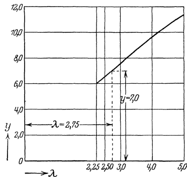
Abb. 40. Graphische Bestimmung des Wertes \lambda bzw. des Brunnenabstandes ( b = \lambda \cdot 2 \cdot x_0 \cdot \pi ) für den Fall, daß die Größen A , s und y festliegen.
