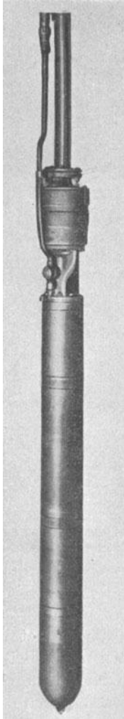
Abb. 6. Motorsenkpumpe für Tiefbrunnen. Die bei der Grundwasserabsenkung für den Umbau und die Erweiterung der Staatsoper Unter den Linden in Berlin zur Verwendung gekommene Tauchmotorpumpe der Siemens-Schuckertwerke.
