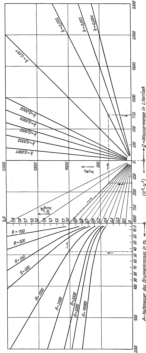
Abb. 25. Graphische Auswertung der Grundformel H^2 - y^2 = \frac{Q}{\pi k} \ln \frac{R}{A} . Beispiel: H = 20 m, y = 6,3 m, R = 1000 m, H^2 - y^2 = 360 , k = 0,002 , dafür Q \approx 750 l/sek.
