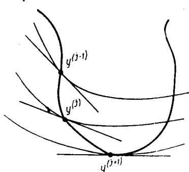
Рис. 4.2. Интерпретация алгоритма самообучения
