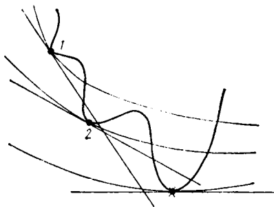
Рис. 4.3. Локальные экстремумы (точки 1 и 2), не являющиеся неподвижными точками
