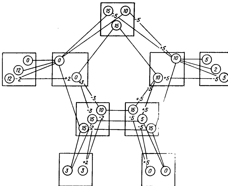
Рис. 3.9. Состояние алгоритма после пятой итерации (получена грамматика с пустым ядром)
