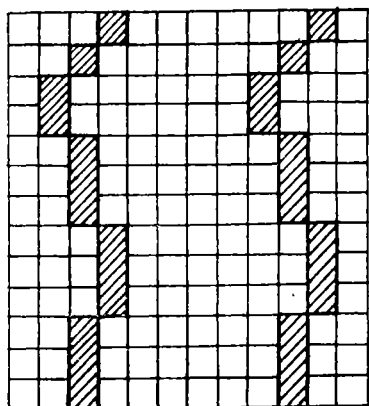
Рис. 2.5. Примеры допустимых ( a, б ) изображений кривых полос постоянной ширины и недопустимых ( в, z )
