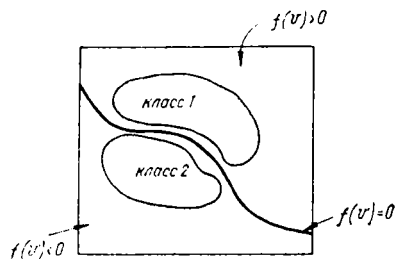
Рис. В.1. Геометрическая интерпретация задачи распознавания
