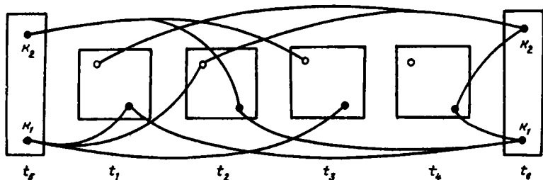
Рис. 1.4. Задание локально-конъюнктивного предиката третьего порядка двумерной грамматикой
