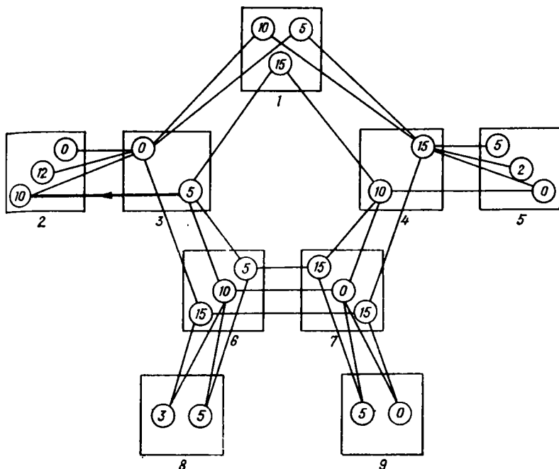
Рис. 3.6. Исходные данные задачи двумерного программирования и вычеркивание на первой итерации
