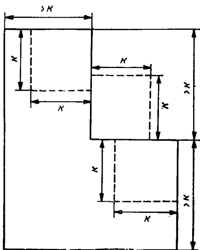
Рис. 1.3. Изображение, изолированное на структуре \mathcal{T}_k
