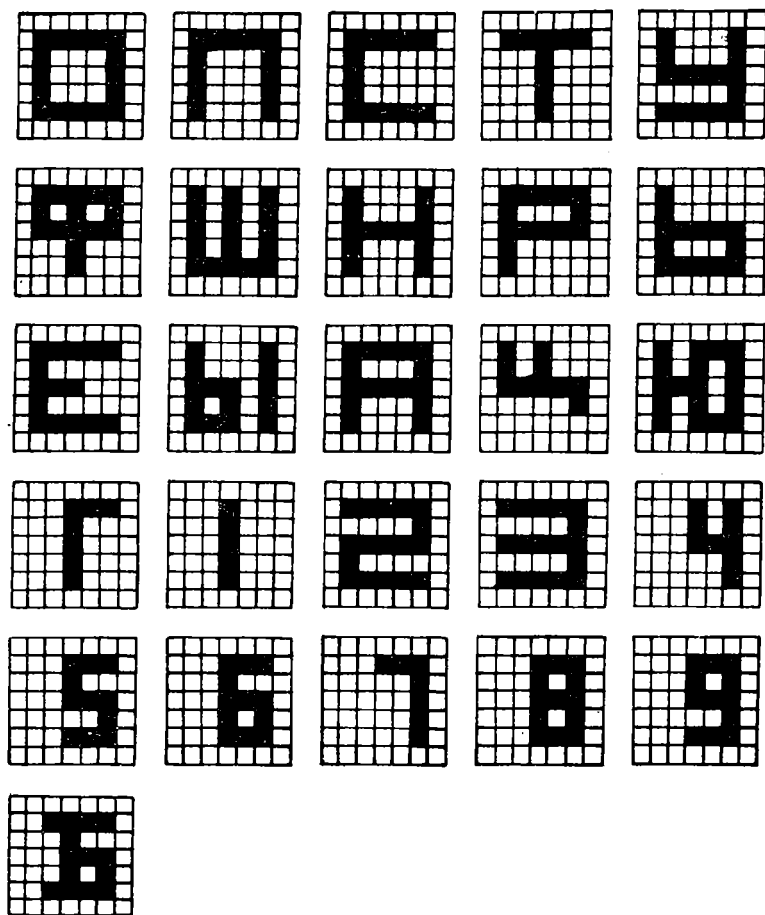
Рис. 2.11. Функции \varphi для различных алфавитно-цифровых знаков
