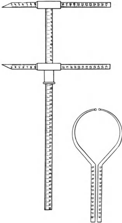
Abb. 2. Stangenzirkel (oberstes Teilstück des Anthropometer) mit eingesteckten Linealen, zum Gebrauch fertig. Daneben die beiden Lineale mit Tasterarmen. \frac{1}{6} n. Gr.
