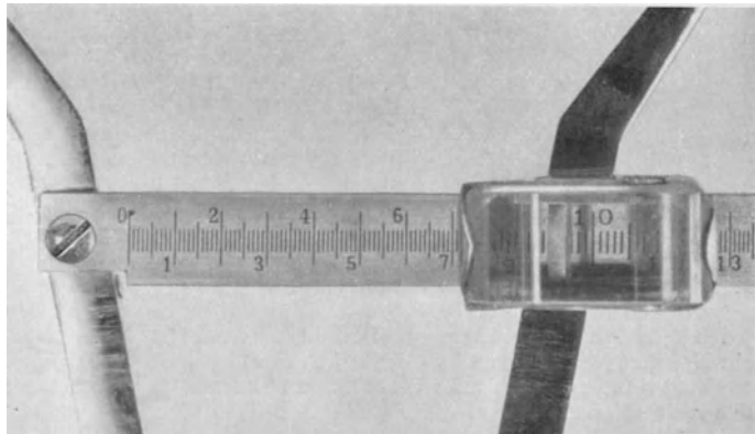
Abb. 6. Aufsetzlinse für den Taster zum besseren Ablesen der Skala. Plankonvexer Kronglaszylinder in Metallrahmen nach DAVIDSON BLACK.
