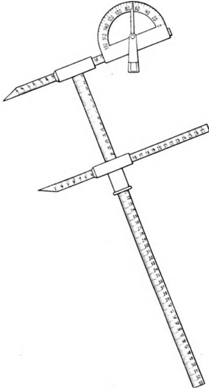
Abb. 7. Ansteckgoniometer, an dem Stangen- zirkel angebracht. \frac{1}{8} n. Gr.
