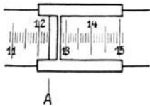
Abb. 5. Ablesung der Maßzahl am Tasterzirkel. A = Kante des Index, wo die Ablesung erfolgt. Aus SCHLAGINHAUFEN, O. 1927. Leitfaden für die anthrop. Untersuchungen an den schweiz. Stellungspflichtigen. Zürich. S. 12.
