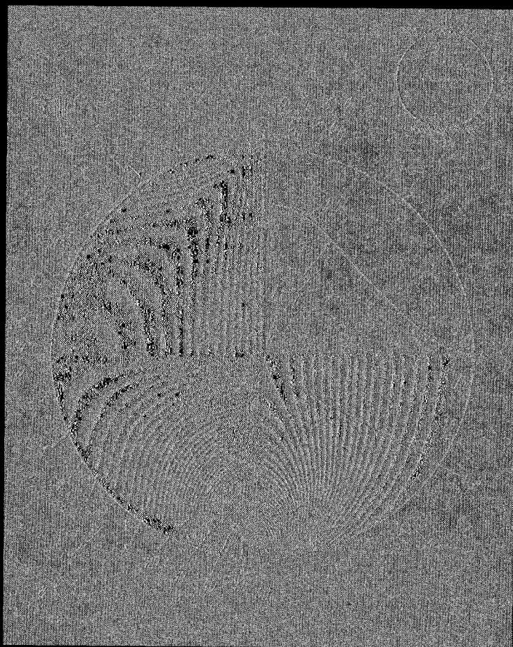
Рис. 112. Картины муаровых полос, изохромы и нормализованные разности главных нормальных напряжений по горизонтальной оси для диска, нагруженного по диаметру сосредоточенными силами. 1 - изохромы \sigma , 2 - изохромы \sigma , 3 - эталонная решетка, 4 - изохромы, 5 - метод «муара», 6 - метод фотоупругости.
