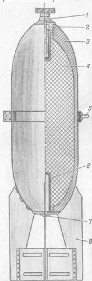
Рис. 12. ФАБ-100 СЛ (с пенолитным корпусом):
