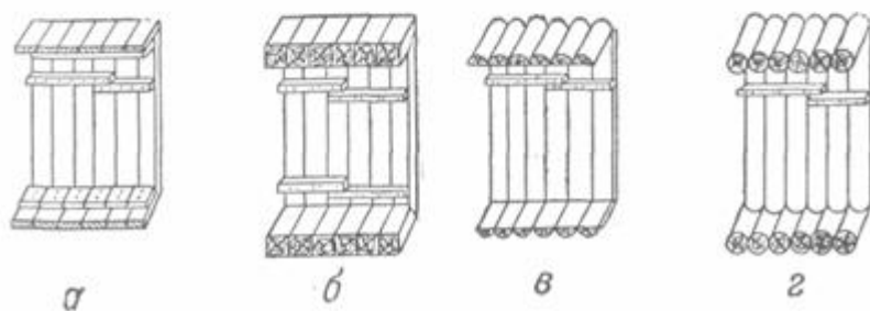
Рис. 149. Крепление горизонтального хода полными рамами: а — дощатые; б — брусчатые; в — пластинчатые; г — бревенчатые
