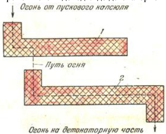
Рис. 78. Схема пиротехнического дистанционного механизма:
