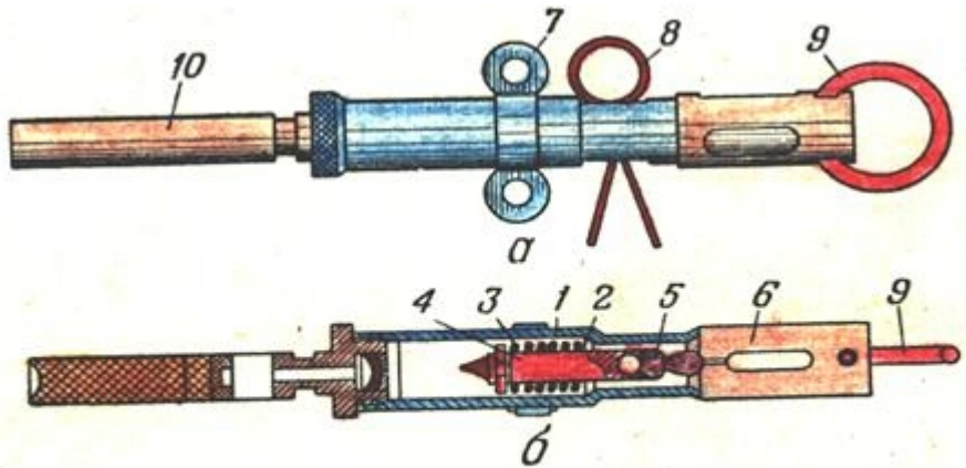
Рис. 118. Взрыватель ВПФ:
