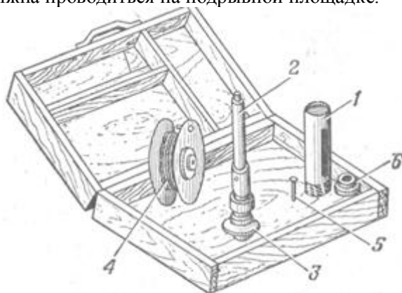
Рис. 156. Дистанционный извлекатель взрывателей:
