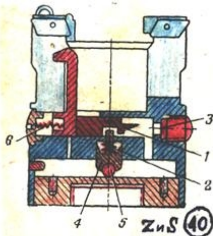
Рис. 80. Германское противосъемное приспособление (ликвидатор):
