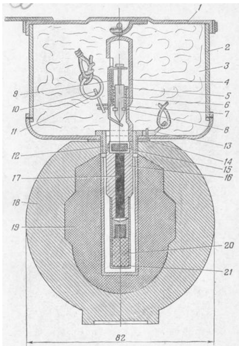
Рис. 21. Авиационная граната АГ-2:
