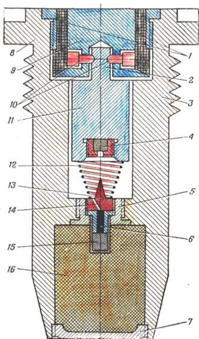
Рис. 71. Пиротехнический механизм взведения взрывателя РД:
