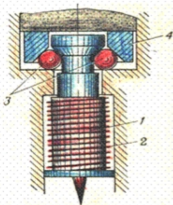
Рис. 74. Шариковый предохранитель: 1 — ударник; 2 — боевая пружина; 3 — шарики; 4 — конусное кольцо
