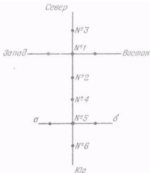
Рис. 131. Уточнение места нахождения авиабомбы по методу наибольших показаний прибора
