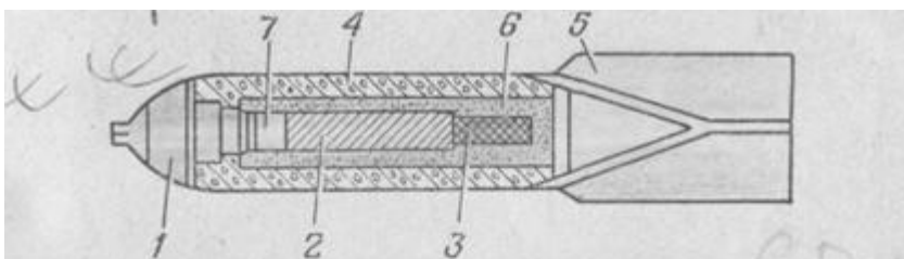
Рис. 30. Осколочная авиабомба калибра 10 кг:
