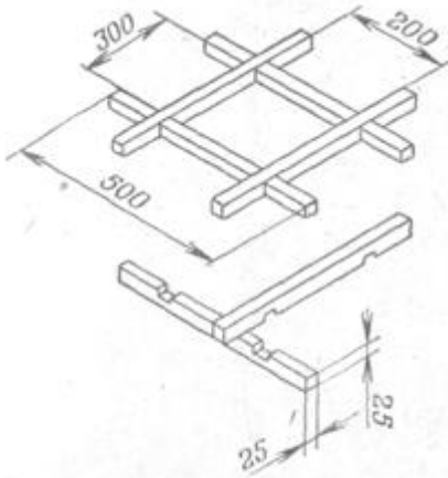
Рис. 145. Обчинная рама из брусьев
