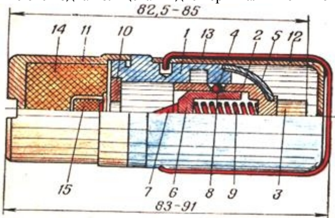
Рис. 120. Взрыватель МВ-3: 1 — корпус; 2 — втулка; 3 — выступ; 4 — шарик; 5 — жестяной колпачок; 6 — ударник; 7 — жало; 8 — кольцевой паз; 9 — пружина; 10 — донышко; 11 — стакан; 12 — предохранительный колпачок; 13 — держатель; 14 — промежуточный детонатор; 15 — капсюль-детонатор
