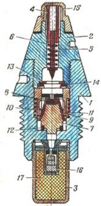
Рис. 101. Взрыватель (КТ-1) полупредохранительного типа:
