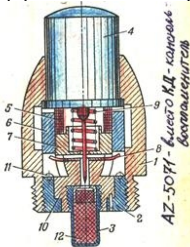
Рис. 114. Германский минный ударный взрыватель AZ5075:
