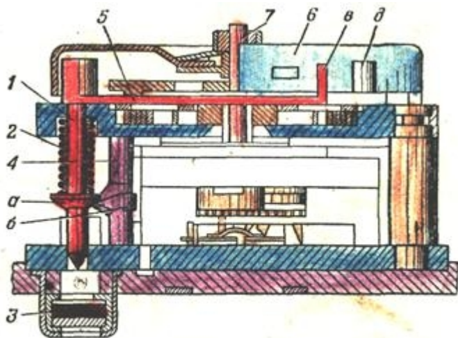
Рис. 105. Часовой и дистанционный механизмы трубки:
