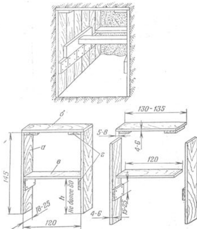
Рис. 151. Крепление горизонтального хода неполными дощатыми рамами:
