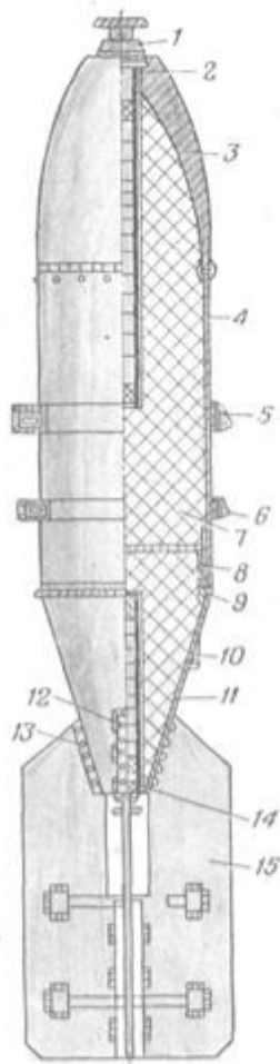
Рис. 10. ФАБ-1000:
