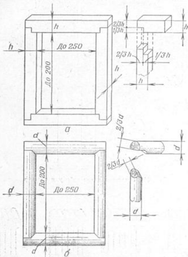
Рис. 150. Рамы горизонтального хода: а — брусчатая рама; б — бревенчатая рама
