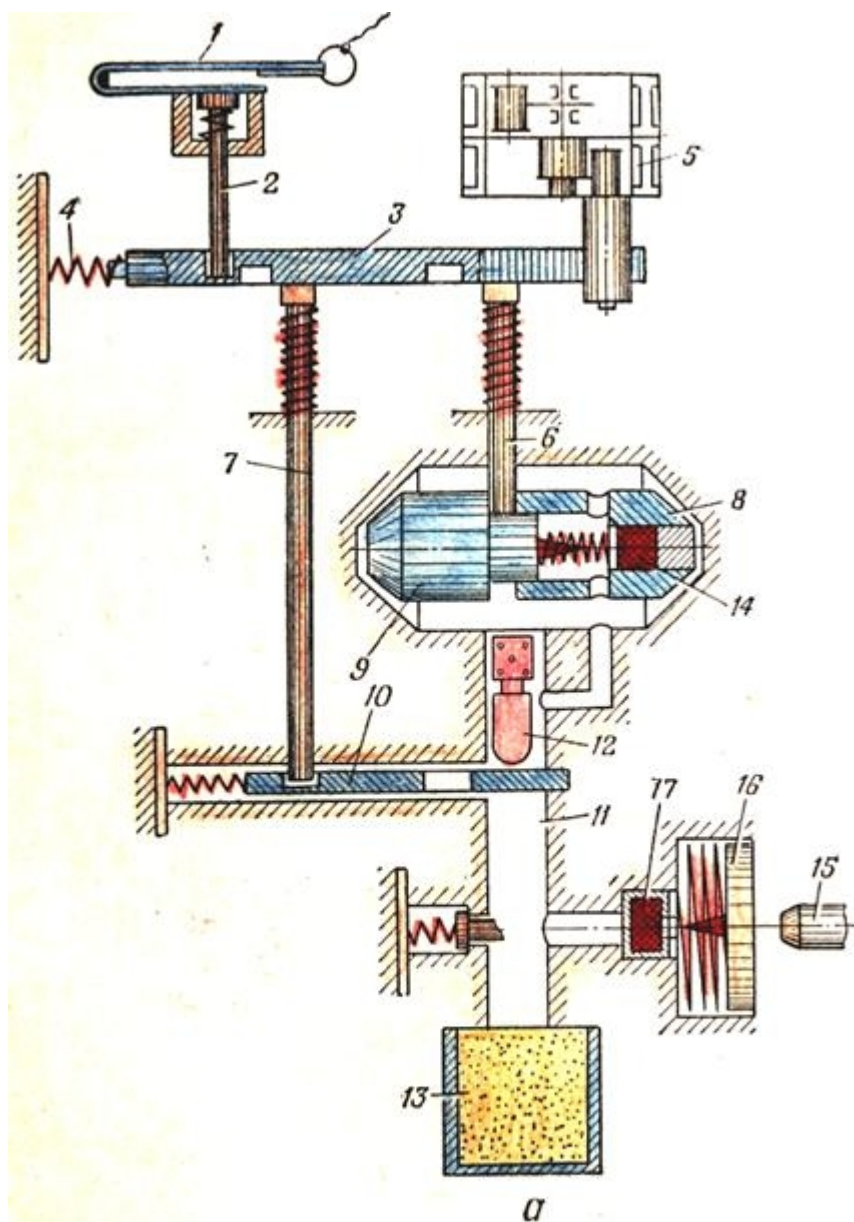
Рис. 93. Схема механизма
