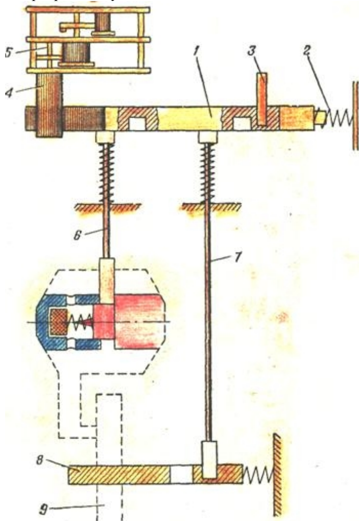
Рис. 70. Схема часового механизма взведения:
