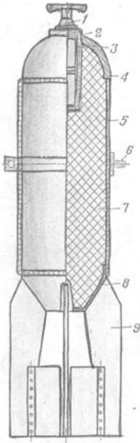
Рис. 7. ФАБ-50 ШГ:
