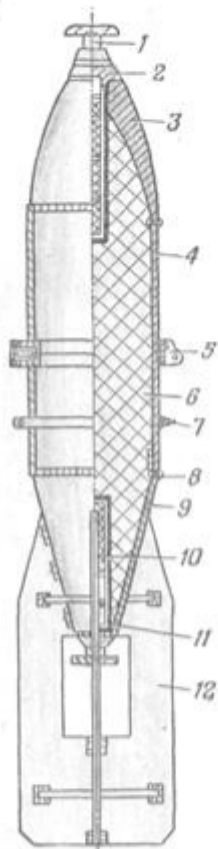
Рис. 9. ФАБ-250:
