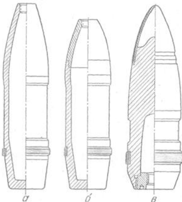
Рис. 40. Оболочки снарядов:
