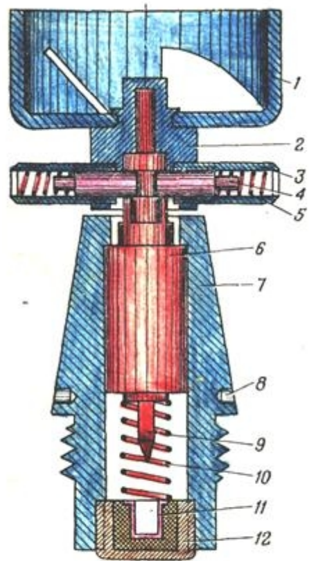
Рис. 87. Разрез взрывателя АДЦ:
