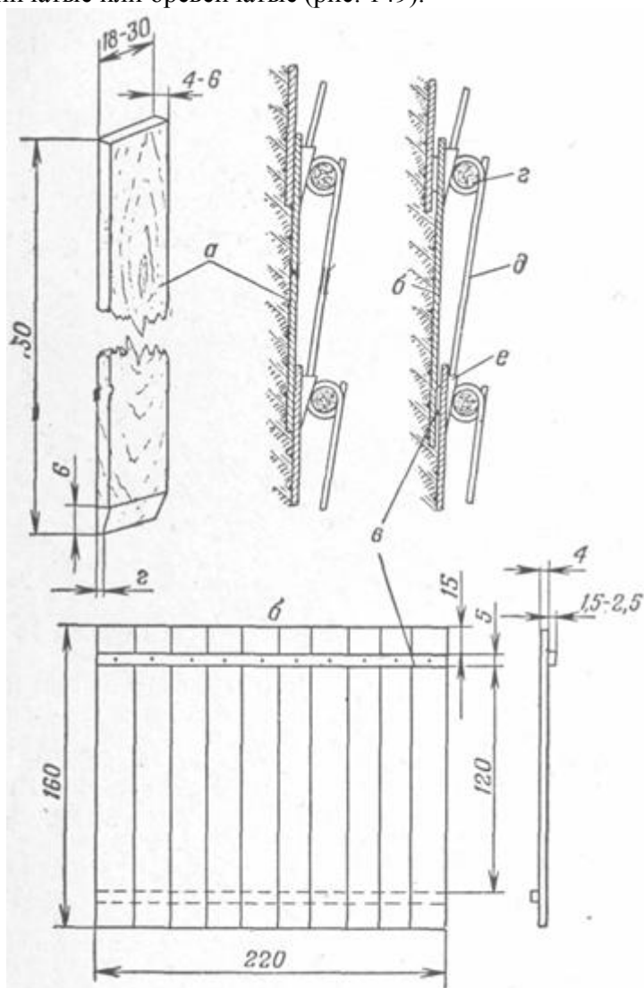
Рис. 147. Щит:
