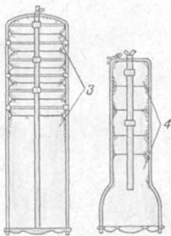
Рис. 36. Выстрел картузного заряжания: 1 — снаряд; 2 — взрыватель; 3 — полный переменный боевой заряд; 4 — уменьшенный переменный боевой заряд
