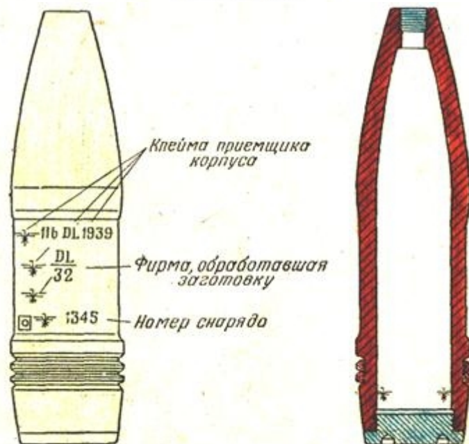
Рис. 50. Клейма на корпусах снарядов, штампованных через дно
