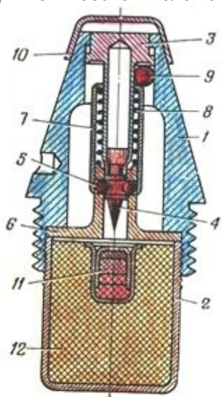
Рис. 109. Минный ударный взрыватель М-50:
