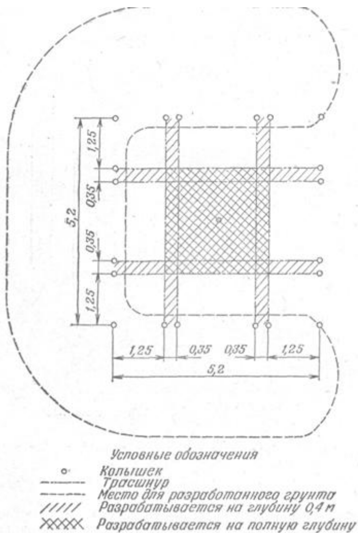
Рис. 154. Трассировка шахты
