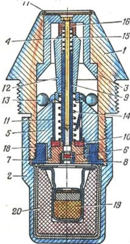
Рис. 115. Германский минный ударный взрыватель WgrZ38:
