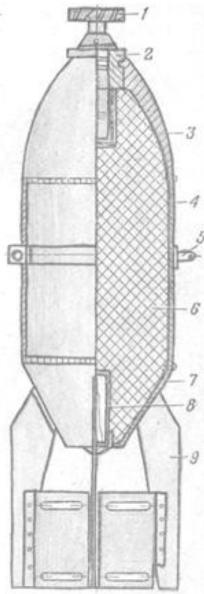
Рис. 8. ФАБ-100 М — литая головка:
