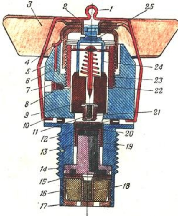
Рис. 86. Разрез взрывателя АВШ-2:
