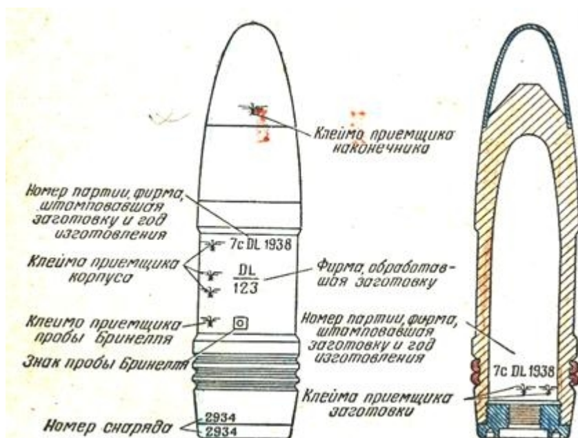
Рис. 51. Клейма на корпусах бетонобойных снарядов
