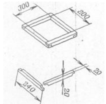
Рис. 146. Закладная рама из брусьев
