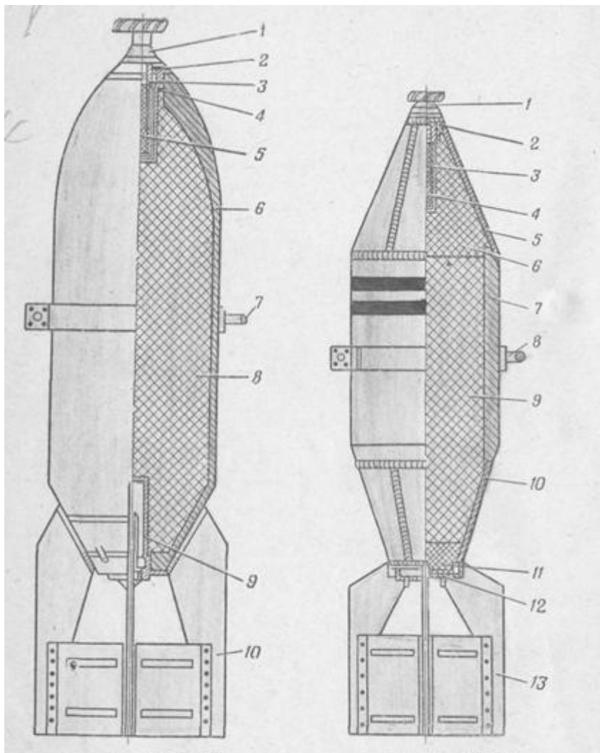
Рис. 13. ФАБ-100 СЧ:
