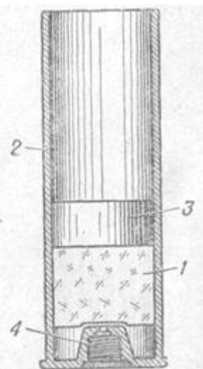
Рис. 37. Холостой выстрел:
