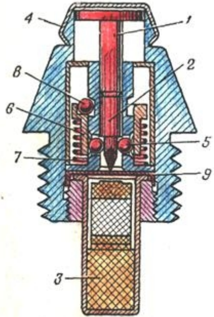
Рис. 98. Взрыватель с ударным механизмом мгновенного (реакционного) действия: „БМ“
