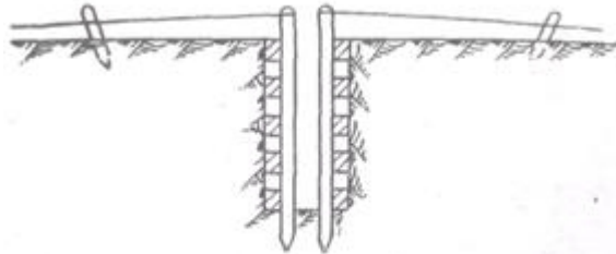
Рис. 164. Крепление стен предохранительной траншеи, пройденной в сыпучих грунтах
