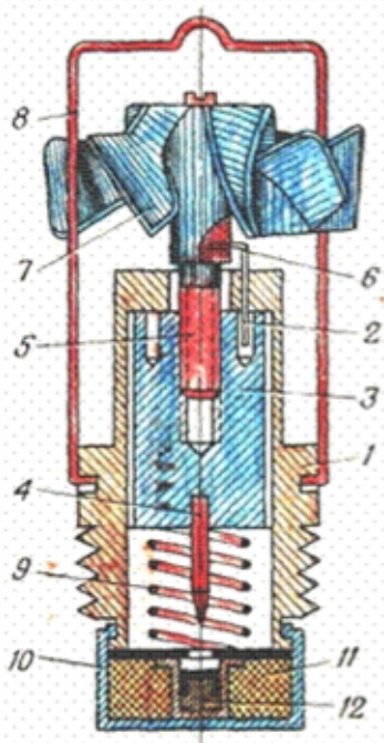
Рис. 68. Разрез взрывателя АД-А: 1 — корпус; 2 — шпилька фиксатора; 3 — ударник; 4 — жало; 5 — винт вст- ривки; 6 — штифт антиконтра; 7 — ветрянка; 8 — поддонная предохра- нительная чеша; 9 — предохранительная пружина; 10 — стакан детонатора; 11 — детонаторная чашка; 12 — капсюль-де- тонатор
