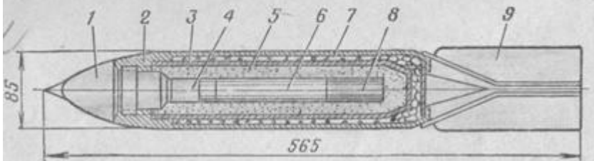
Рис. 31. Осколочная авиабомба BdC-10:
