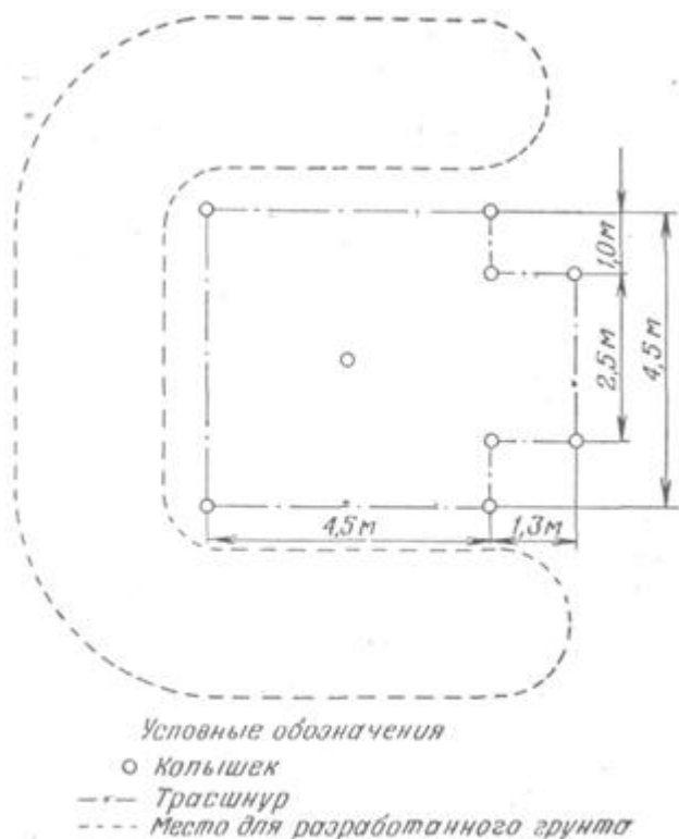
Рис. 153. Трассировка котлована с наклонными стенками
