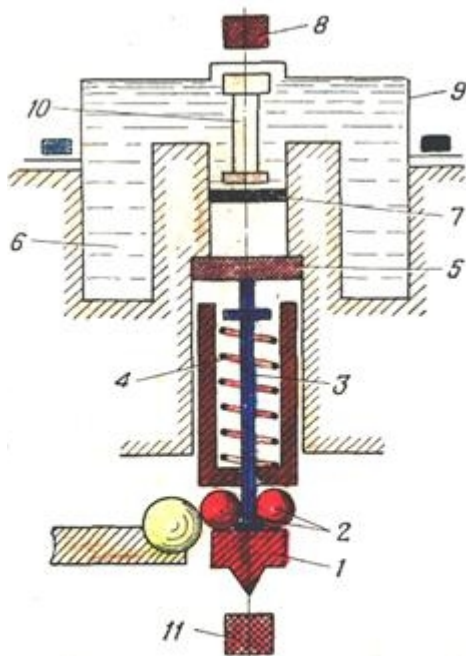
Рис. 76. Схема химического механизма длительного замедления:
