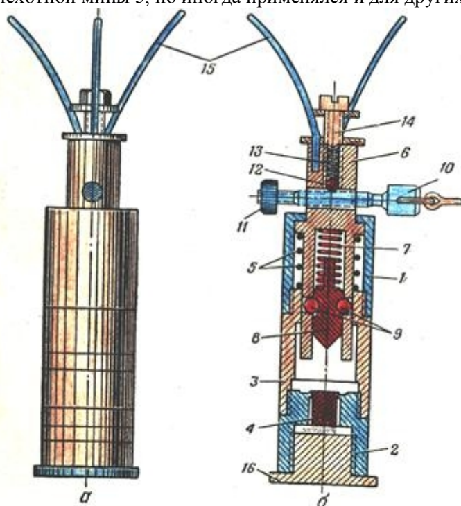
Рис. 122. Германский взрыватель SMiZ-35: а — общий вид; б — разрез; 1 — корпус; 2 — капсюль-держатель; 3 — соединительная муфта; 4 — капсюль-воспламенитель; 5 — нажимная пружина; 6 — головка; 7 — боевая пружина; 8 — ударник; 9 — шарик; 10 — предохранительная чека; 11 — гайка чеки; 12 — шарик чеки; 13 — пружина шарика; 14 — стопорный винт; 15 — усики; 16 — пробка, закрывающая капсюль-держатель.
