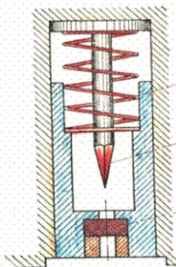
Рис. 73. Воспламенительный механизм
