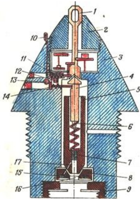
Рис. 91. Схема устройства германского механического взрывателя A.Z C10 (hut)*3:
