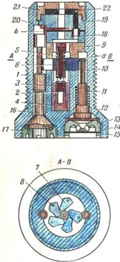
Рис. 113. Германская донная ударная трубка BdZf21cm Gr18 Be:
