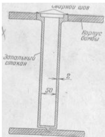
Рис. 23. Запальный стакан и его крепление в авиабомбе
