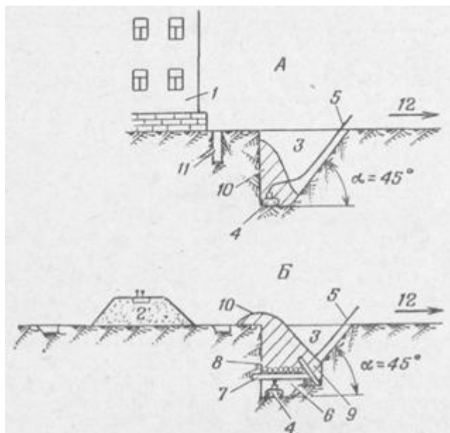
Рис. 166. «Отдушины»:
