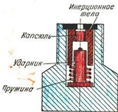
Рис. 90. Схема устройства взрывателя A.Z.8312, применявшегося в электронно-термитных авиабомбах
