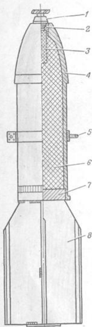
Рис. 15. ФАБ-50 М (из 152-мм снаряда):
