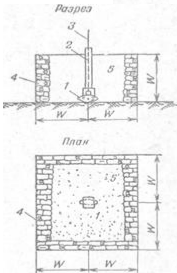
Рис. 169. Засыпка грунтом невзорвавшейся ФАБ, находящейся на поверхности земли:
