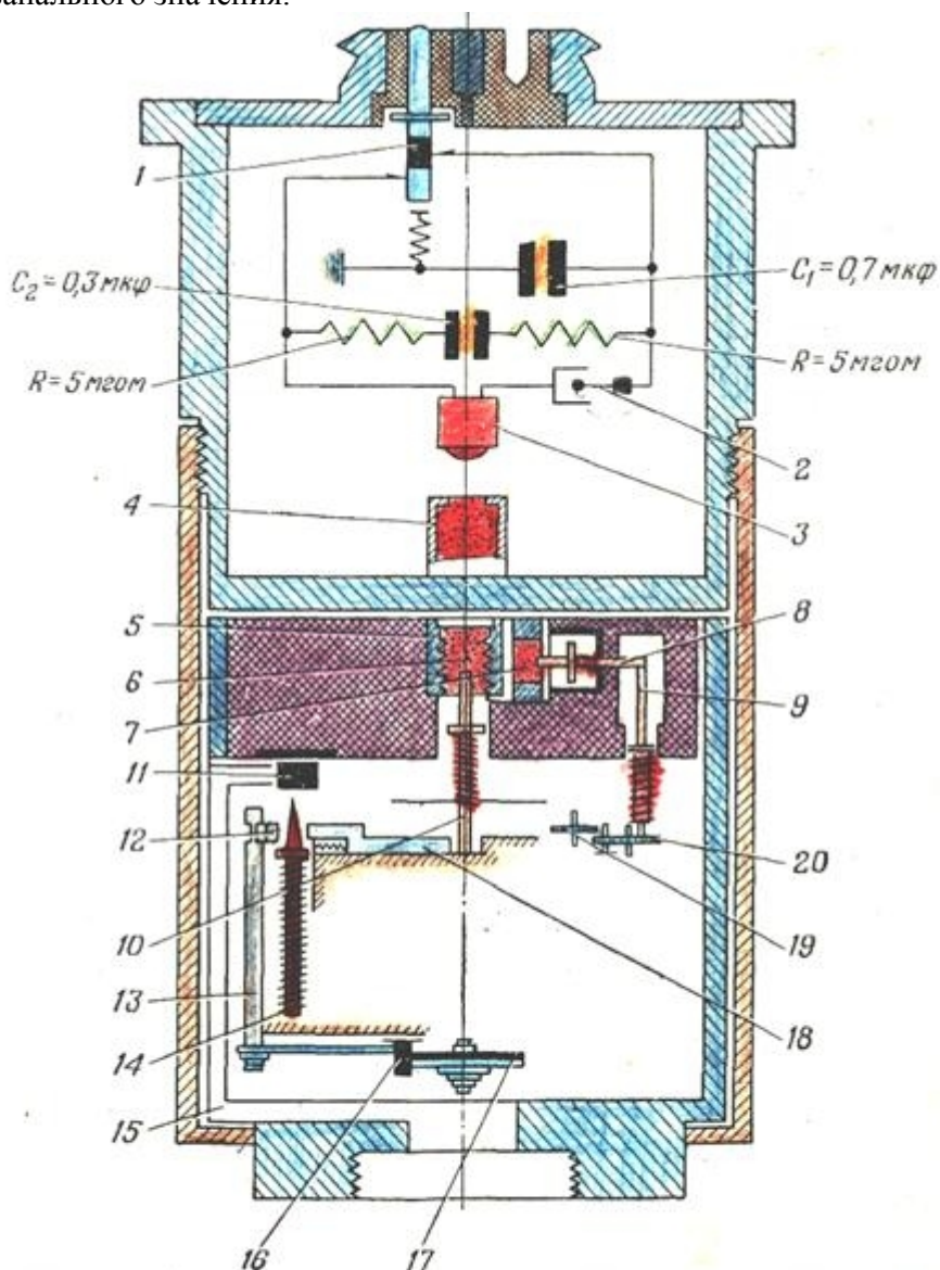
Рис. 95. Схема германского взрывателя с часовым механизмом замедления:
