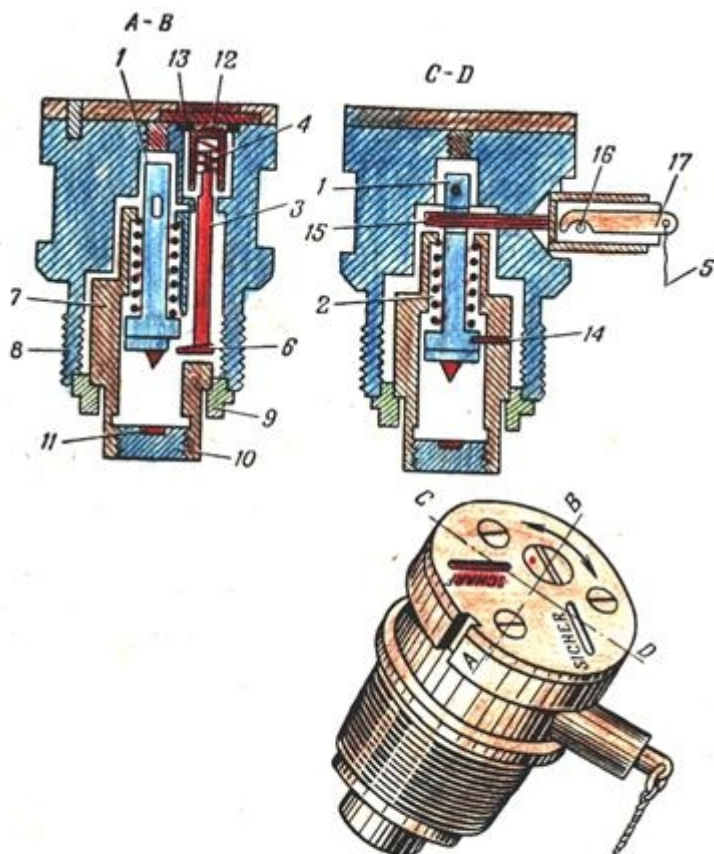
Рис. 123. Германский взрыватель TmZ-35;
