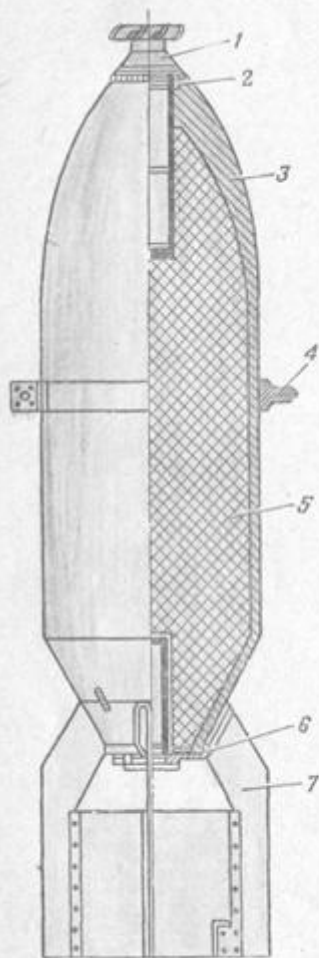
Рис. 11. ФАБ-100 ЦК: 1 — взрыватель; 2 — головной запальный стакан; 3 — корпус; 4 — бутель; 5 — взрывчатое вещество; 6 — дно с запальным стаканом; 7 — стабилизатор
