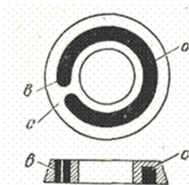
Рис. 102. Дистанционное кольцо:
