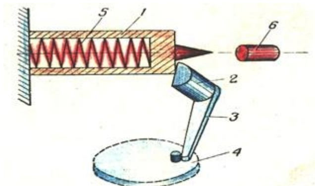
Рис. 75. Рычажный предохранитель: 1 — ударник; 2 — спусковой стержень; 3 — рычаг; 4 — дистанционный или замедлительный механизм; 5 — боевая пружина; 6 — капсуля-воспламенитель
