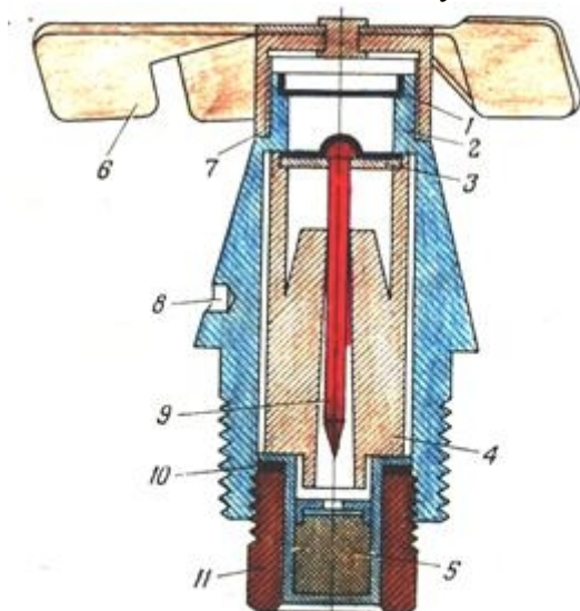
Рис. 85. Разрез взрывателя АМ-А;
