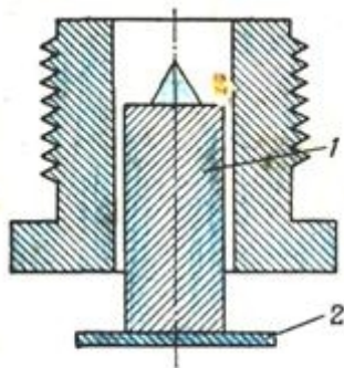
Рис. 60. Воспламенительный механизм с реакционным ударником:
