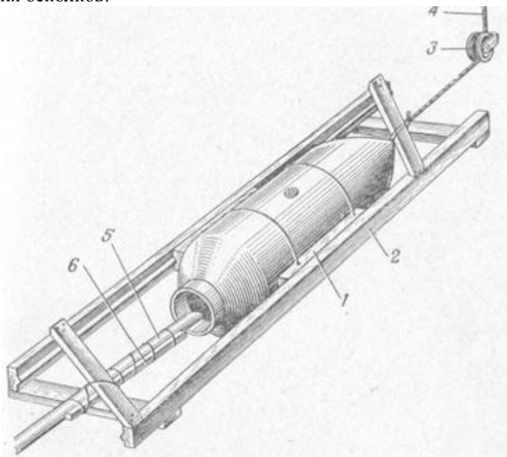
Рис. 160. Приспособление для подачи шлангов с паром внутрь корпуса авиабомбы:
