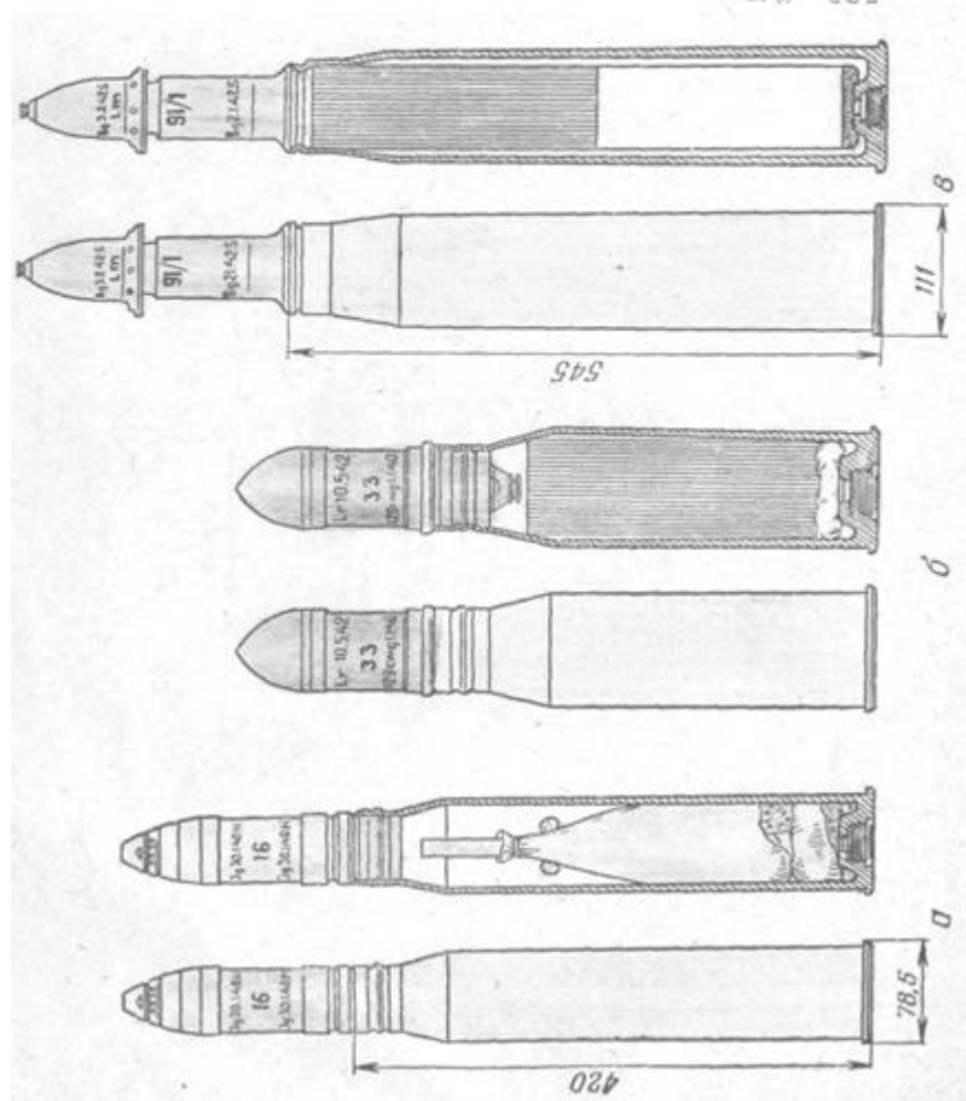
Рис. 34. Выстрелы патронного заряжания башней германской артиллерии:
