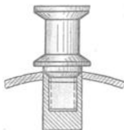
Рис. 4. Подвесная цапфа
