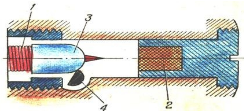
Рис. 65. Воспламенительный механизм с заранее взведенной боевой пружиной:
