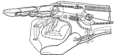
Рис. 10. Искусственная кисть системы Бете; сгибаются все фаланги всех пальцев.
