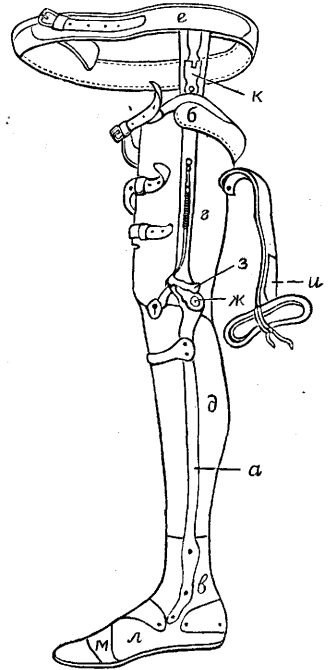
Рис. 1. Протез шинно-гильзовый при ампутации бедра: а—стальная наружная шина; б—обшивка сиденья; в—деревянная бедровая часть; г—кожаная бедренная гильза; д—кожаная голенная гильза; е—полая; ж—коленный шарнир; з—замок; и—плечевой тяг; л—металлическая ланка; м—деревянная стопа; н—пальцевой стиб.
