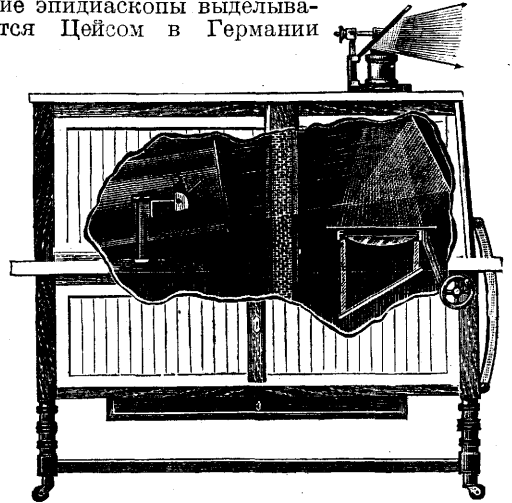
Рис. 5. Эпидиаскоп с изображением хода лучей.
