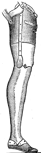
Рис. 2. Протез при ампутации бедра — полуамериканский, голень деревянная, верхняя часть бедренной гильзы кожаная.
