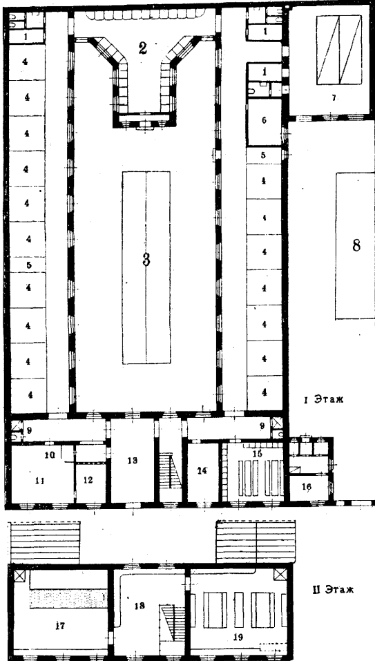
Рис. 1. Механическая самодеятельная общественная прачечная кабинного типа на 10 000 чел.: 1—кладовая; 2—замачивание; 3—навес для ручных тележек; 4—кабина; 5—двигатель; 6—механик; 7—котельная; 8—сарай для топлива; 9—лифт; 10—касса; 11—контора; 12—весы; 13—теплый проезд; 14—уборщица; 15—ожидание; 16—сторож; 17—сушило; 18—упаковка; 19—голландеры.
