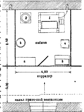
Рис. 2. Деталь кабины: 1—стиральная машина; 2—центрифуга; 3—бучильник; 4—тележка; 5—стиральное корыто; 6—стол.
