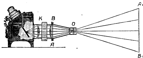
Рис. 2. Схема проекционного фонаря: АВ—предмет; A_1B_1 —изображение на экране; К—конденсор; О—объектив.
