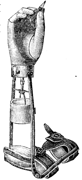
Рис. 8. Активный протез при ампутации предплечья; приводится в действие пронацией и супинацией культи (системы Г. Альбрехта).
