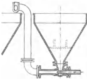
Fig. 13b. Schnitt.
