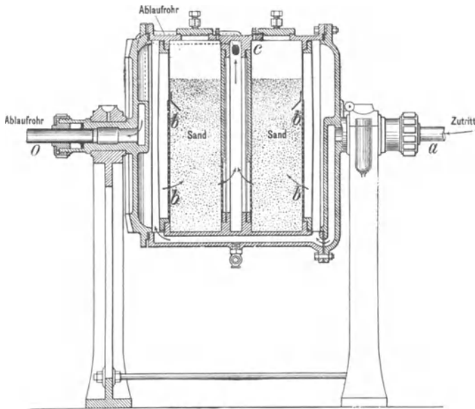
Fig. 31. Kröhnke-Filter.
