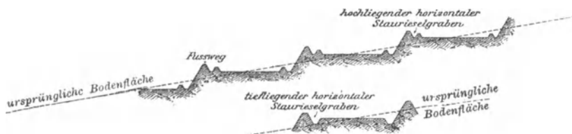
Fig. 77. Schnitt C—D.
