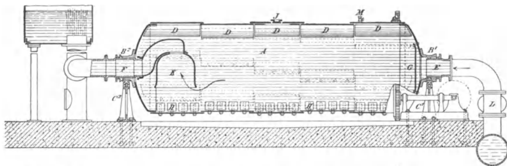
Fig. 19. Schnitt durch die Längsachse.
