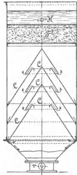
Fig. 115. Kläreylinder nach Dervaux.
