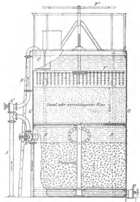
Fig. 28. Howatson-Filter. Das Reinheits-Filter.
