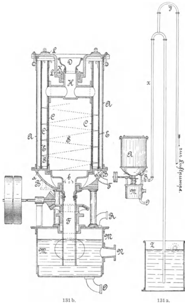
Vorrichtung zum Entwässern des Schlammes.
