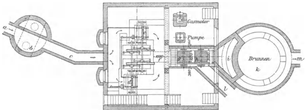
Fig. 106. Grundriss.
