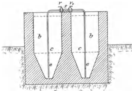
Fig. 110 b. Querschnitt.
