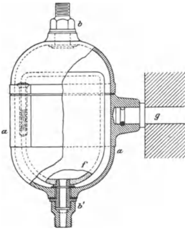
Fig. 43. Filter von Olschewsky.
