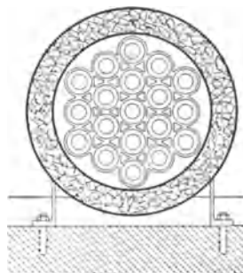
Querschnitt Fig. 41.
