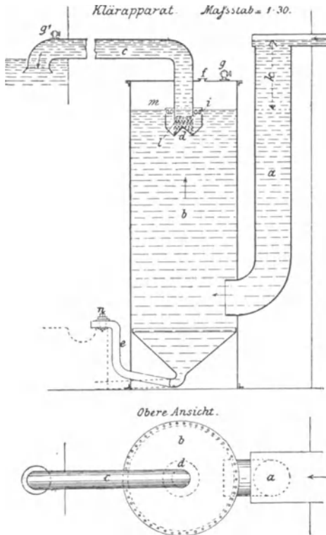
Fig. 97. Klärcylinder.
