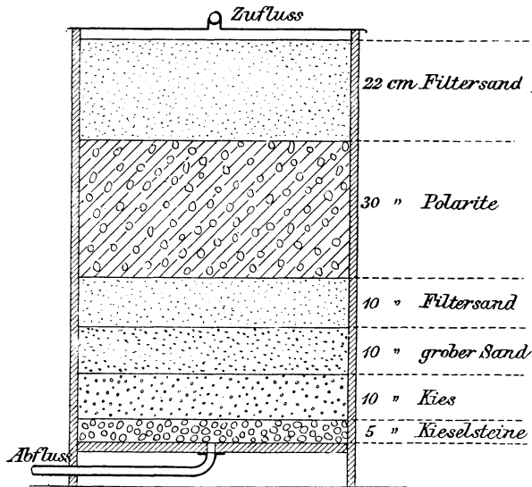
Fig. 86. Polarite-Filter.
