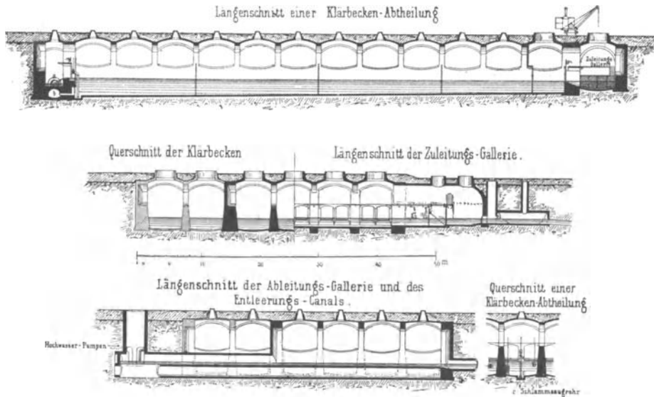
Fig. 99. Kläranlage in Frankfurt a. M.
