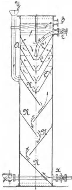
Fig. 114. Kalksättiger nach Dervaux.
