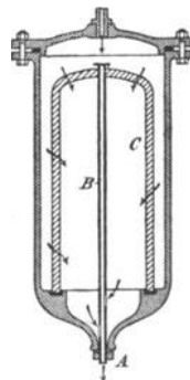
Fig. 42. Filter von Stavemann
