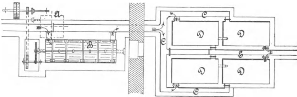
Grundriss.
