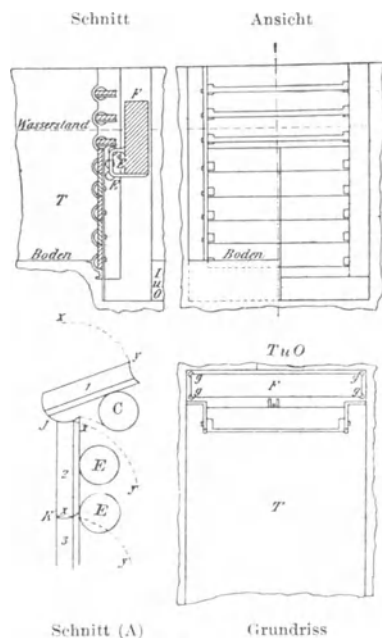
Fig. 1. Etagenwehr.
