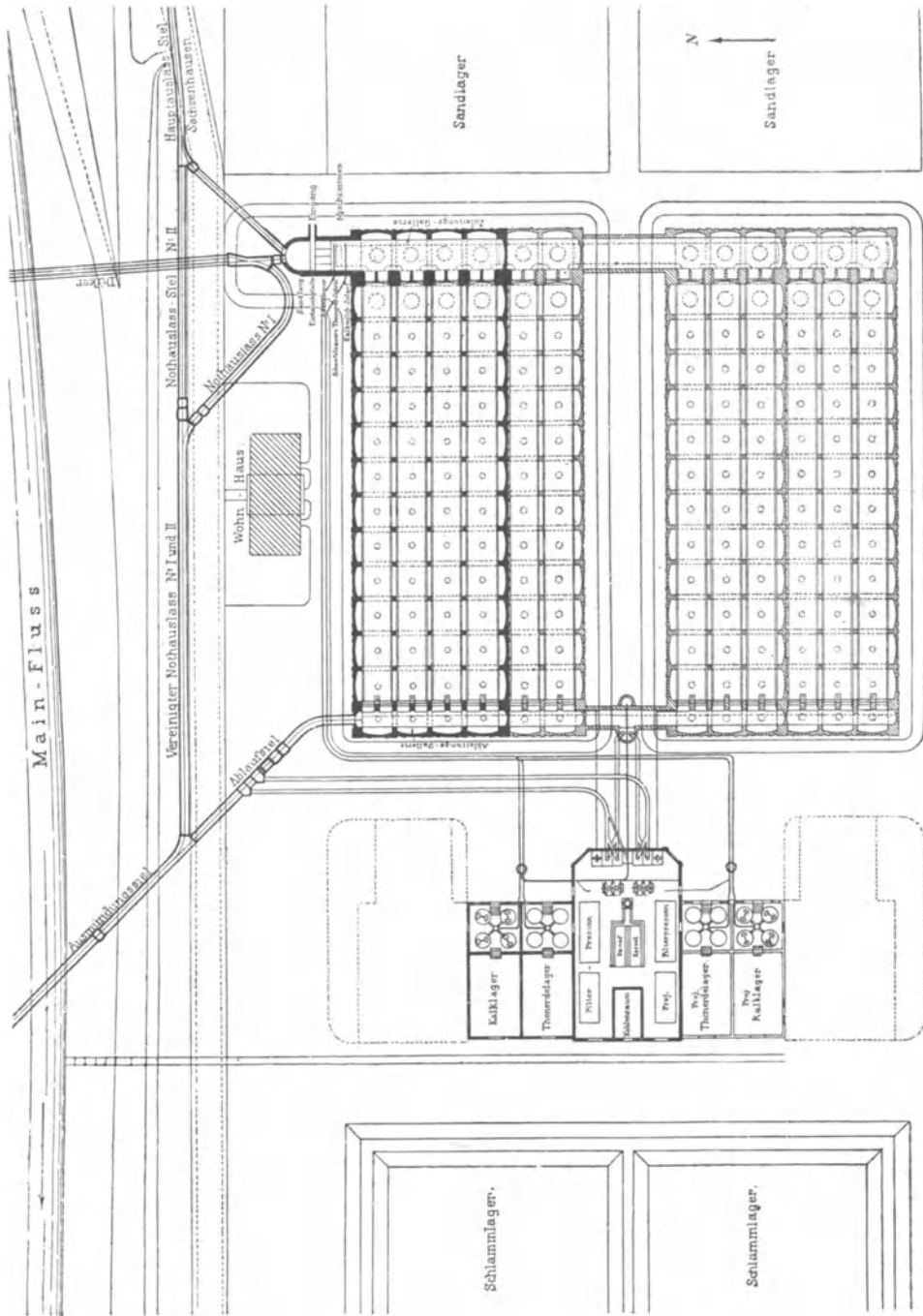
Fig. 98. Kläranlage in Frankfurt a. M.
