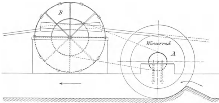
Fig. 128 a. Längsschnitt.
