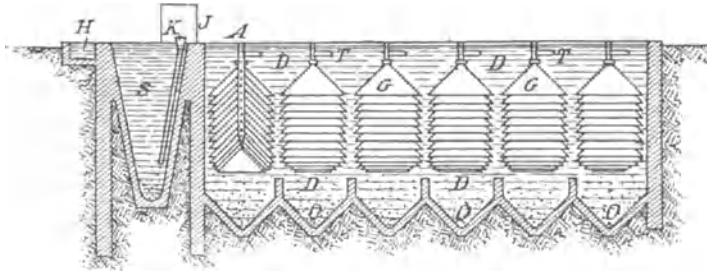
Fig. 116a. Längsschnitt.
