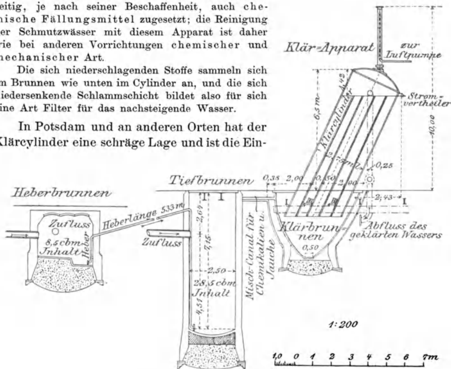
Fig. 112. Kläranlage in Potsdam.
