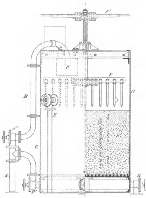
Fig. 27. Howatson-Filter. Industrie-Filter.
