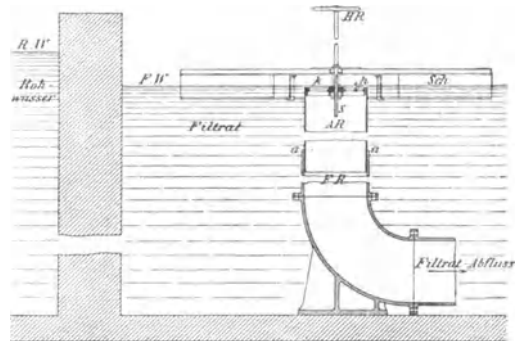
Fig. 18. Regulirungsapparat.
