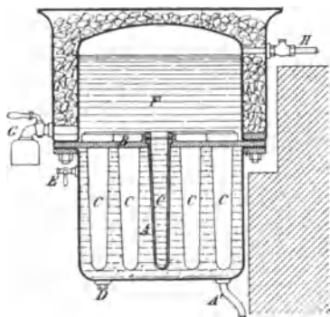
Längsschnitt Fig. 40.
