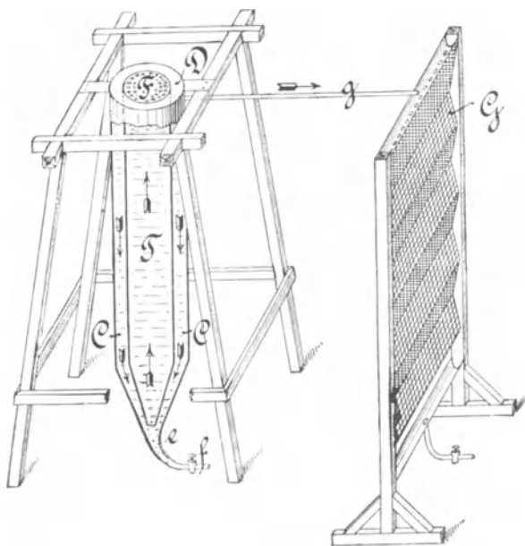
Fig. 132. Klär- und Lüftungs-Vorrichtung.
