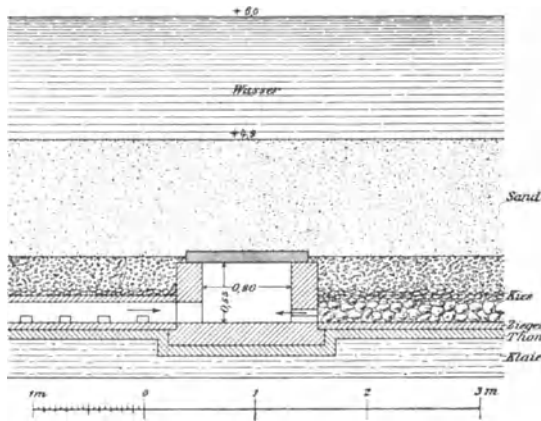
Fig. 6. Schnitt eines Hamburger Filters.
