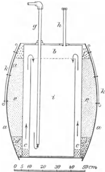
Fig. 64. Tauchfilter von Dunbar.
