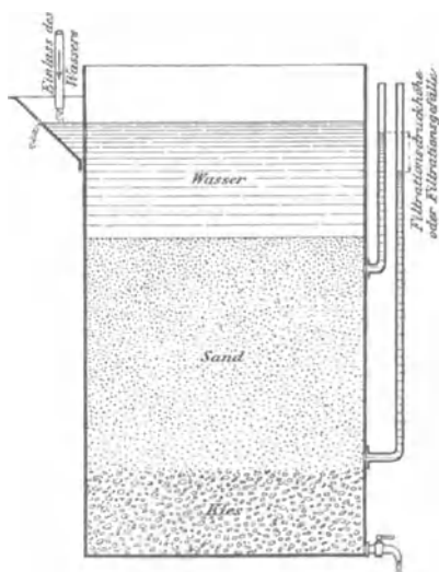
Fig. 3. Versuchs-Filter.
