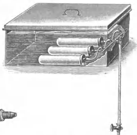
Fig. 37. Saugfilter von Berkefeld-Nordtmeyer.
