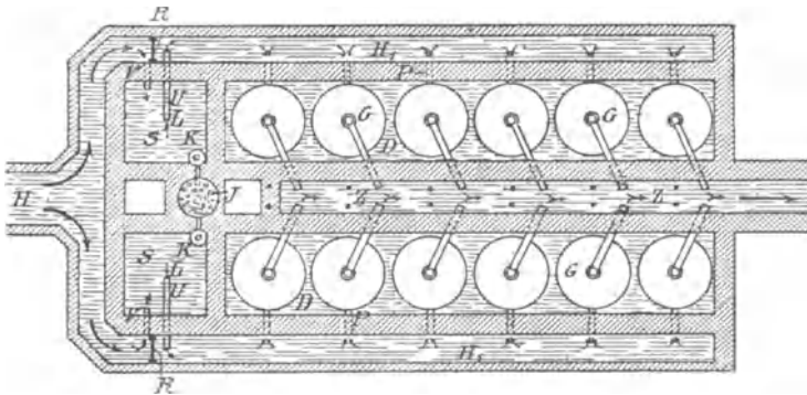
Fig. 116b. Flächenansicht.
