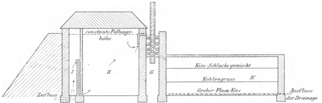
Längsschnitt
