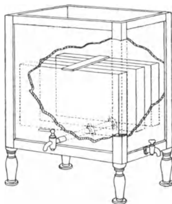
Fig. 51. Asbest-Filter von Trenkler.
