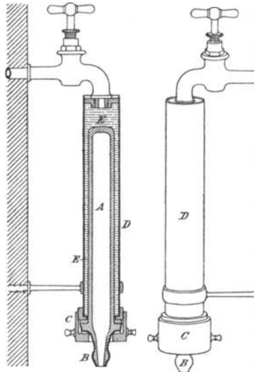
Durchschnitt des Filters. Umriss des eingesetzten Filters.
