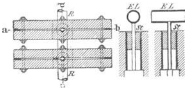
Fig. 16. Schnitt f—g.
