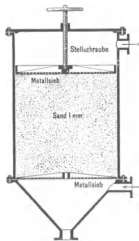
Fig. 63. Pressfilter von Dunbar.
