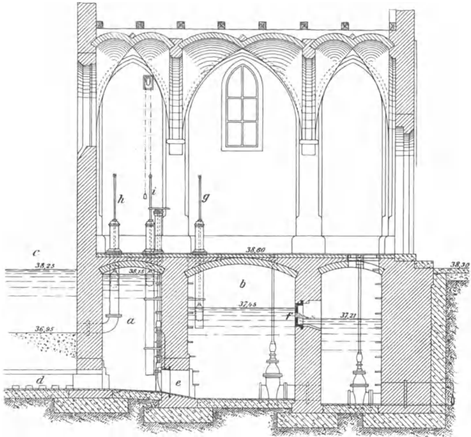
Fig. 12. Regulirkammer der Berliner Filter. (Längenschnitt.)
