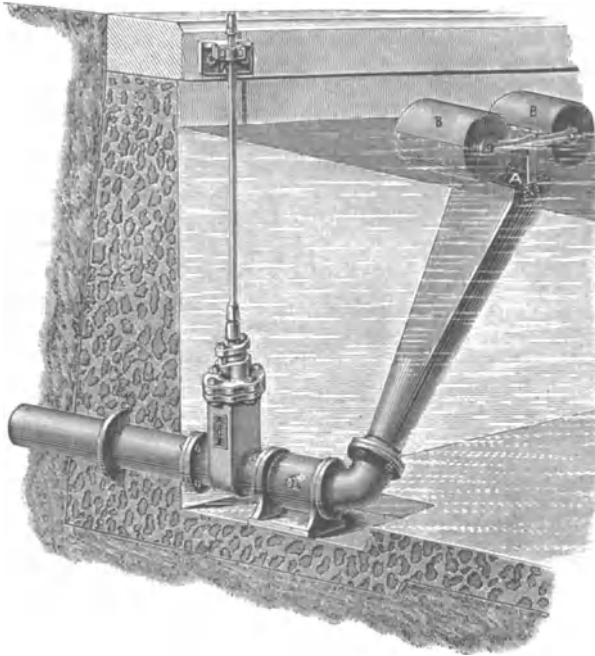
Fig. 2. Schieber mit Schwimmermundstück.
