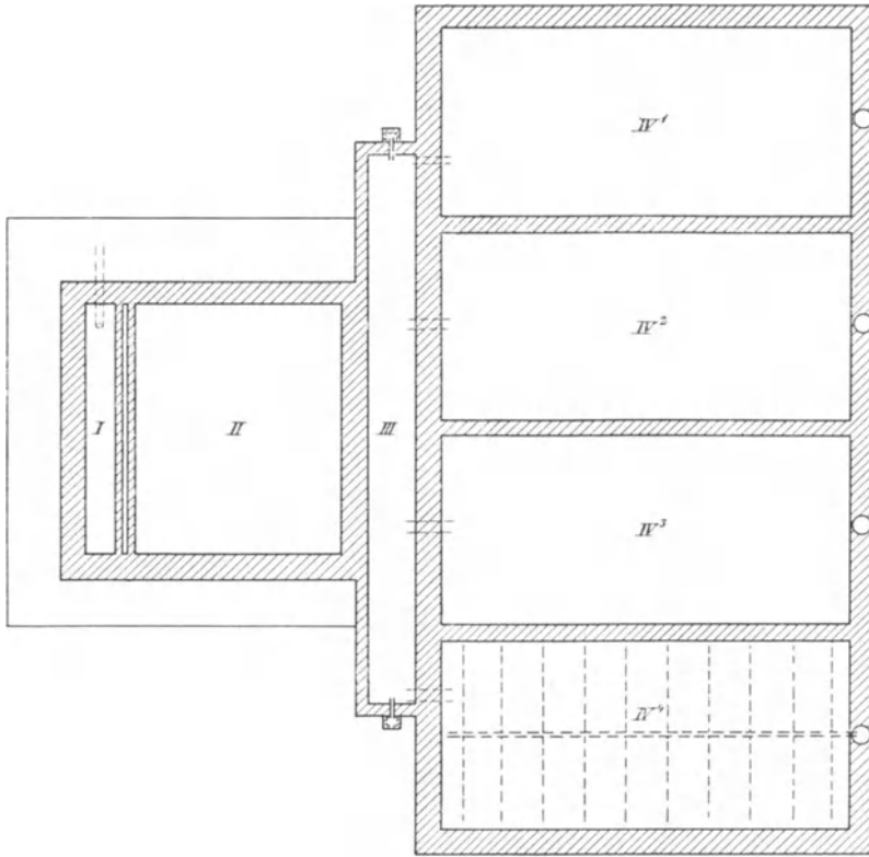
Grundriß
