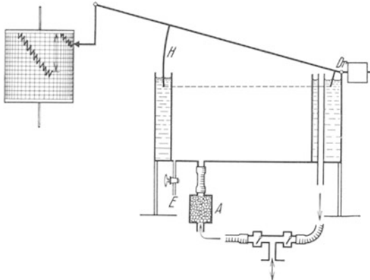
Abb. 115. Schema des KROGHschen Spirometers zur Messung des Sauerstoffverbrauches. Die Spirometerhaube H hat bei Dr ihren Drehpunkt und ist durch ein Gegengewicht ausbalanciert. Das Spirometer ist durch den Einlaß E mit Sauerstoff gefüllt. Die Versuchsperson atmet durch das unten gezeichnete Mundstück gleichmäßig ein und aus. Durch Ventile wird der Luftstrom so „gerichtet“, daß reiner Sauerstoff aus dem Spirometer eingeatmet wird. Dabei sinkt die Spirometerhaube um einen Betrag, der von der Tiefe des Atemzuges abhängt, ab. Dieses Absinken wird auf der Registriertrommel (links) aufgezeichnet. Die ausgeatmete Luft wird über das Ausatmungsventil durch eine kohlenensäureabsorbierende Natronkalkpatrone ( A ) in das Spirometer zurückgeleitet. Dabei steigt die Spirometerhaube wieder ein Stück an, kann jedoch die Ausgangsstellung nicht wieder erreichen, da ein Teil des bei der Einatmung entnommenen Sauerstoffes ja verbraucht und die Kohlenensäure in A festgehalten wird. Treppenartig wird mit jedem neuen Atemzug die Haube weiter und weiter absinken. Das auf der Trommel verzeichnete Absinken über einen bestimmten Zeitabschnitt ergibt, wenn das Spirometer auf Liter geeicht ist, den Sauerstoffverbrauch in der betreffenden Zeit an.
