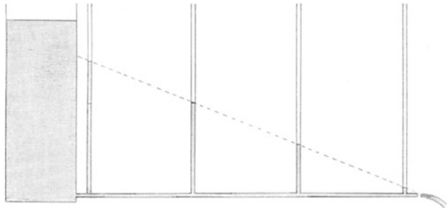
Abb. 49. Druckabfall in einem horizontalen Ausflußrohr. Der Anstieg der Flüssigkeit in den senkrechten Röhren gibt ein Maß für den Druck an den einzelnen Rohrpunkten. (Nach V. FREY.)
