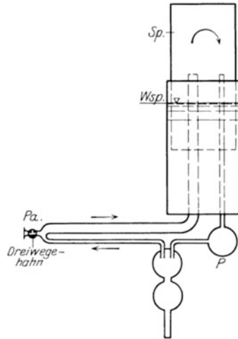
Abb. 116. Schema des Kreislaufapparates von KNIPPING zur Bestimmung des Sauerstoffverbrauches. Das Spirometer ( Sp. ) ist mit Sauerstoff gefüllt. In das Spirometer mündet eine Rohrschleife, aus welcher durch ein Mundstück ( Pa. ) die Versuchsperson reinen Sauerstoff einatmet. In die Rohrschleife ist bei P eine Umwälzpumpe eingebaut, welche den in Spirometer und Röhren befindlichen Sauerstoff in Richtung der Pfeile im Umlauf hält. Dabei passiert das Gas ein (nach abwärts gezeichnetes) Kohlensäureadsorptionsgefäß. Bei jeder Einatmung sinkt das Spirometer um den Volumbetrag der Einatmung ab. Die ausgeatmete Luft wird in Richtung der Pfeile in das geschlossene System gerissen und die Kohlensäure im Adsorptionsgefäß festgelegt. Daher wird bei der Ausatmung das Spirometer nicht zur Ausgangslage zurückkehren. Stufenweises Absinken zeigt den Sauerstoffverbrauch an.
