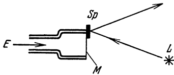
Abb. 47. Schema eines „Membranmanometers“ in natürlicher Größe. Bei Druckerhöhung im Inneren durch den Eingang E wird die Membran M ausgebaut und der Spiegel Sp gedreht, so daß der Lichtzeiger sich bewegt. L Lichtquelle.
