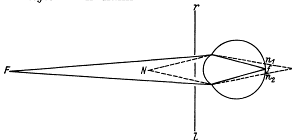
Abb. 350a. Strahlengang beim „SCHEINERSchen“ Versuch. Das Auge sieht durch eine Blende ( r l ) mit zwei feinen Löchern. Dicke Linie: Einstellung auf Ferne ( F ). Dabei wird eine nahe vor dem Auge stehende Nadel ( N ) im Doppelbild ( n_1 und n_2 ) gesehen.
