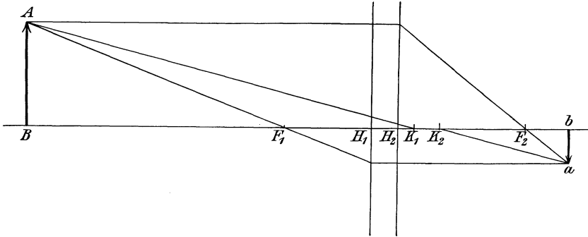
Abb. 340. Konstruktion des Bildes ( ab ) eines Gegenstandes ( AB ) mit Hilfe der sechs Kardinalpunkte: F_1, F_2 Brennpunkte, H_1, H_2 Hauptpunkte, K_1, K_2 Knotenpunkte eines Sammelsystems.
