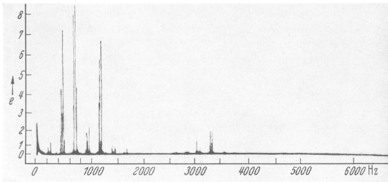
Abb. 330. „Klangspektrum“ des gesungenen Vokales A. Mit einer entsprechenden Vorrichtung gelingt es, die Frequenzbereiche und die Intensität der einzelnen Teiltöne aufzuzeichnen. Ordinate = Intensität, Abszisse = Schwingungszahl pro Sekunde. (Nach M. GRÜTZMACHER.)
