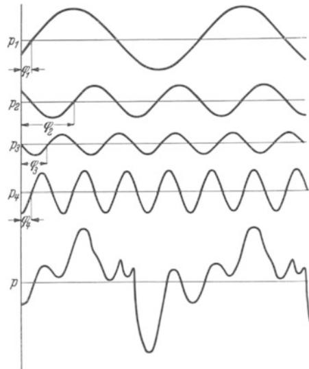
Abb. 329. Oszillogramm eines einfachen Klanges ( p ) und theoretische Analyse desselben. Er besteht aus 4 Tönen bzw. Sinusschwingungen ( p_1, p_2, p_3, p_4 ) von bestimmter Frequenz und bestimmter „Phasenverschiebung“ gegeneinander ( \varphi_1 - \varphi_4 ). Für die Qualität des Klanges beim Hören mit dem menschlichen Ohr sind letztere belanglos, nur die Frequenzen der Teiltöne sind entscheidend. (Nach F. TRENDLENBURG.)
