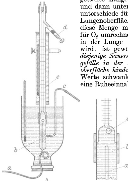
Abb. 105. Mikrotonometer von KROGH. Durch Schlauch und Röhre a strömt das Blut aus einem Blutgefäß in den Apparat ein und rollt die Luftblase (durch einen Stern bezeichnet!) hin und her, welche sich dabei mit den Blutgasen ins Gleichgewicht setzt. Bei c strömt das Blut wieder aus. Von Zeit zu Zeit wird die Luftblase in die Meßcapillare e mittels der Schraube d eingesaugt, um ihr Volumen zu messen. Dieses ändert sich nicht mehr, wenn Gleichgewicht zwischen Blutgasen und Bestandteilen der Luftblase eingetreten ist. Der ganze Apparat ist zur Wahrung gleichmäßiger Temperatur in ein Wasserbad eingebaut. Nach Eintritt des Gleichgewichtes wird die Luftblase in die Capillare aufgenommen, diese auf entsprechende Gefäße aufgesetzt, welche eine Absorption der CO 2 durch Lauge sowie eine solche des Sauerstoffes durch Pyrogallol gestatten, wobei jeweils das auf die beiden genannten Gase entfallende Volumen mittels der Capillare festgestellt werden kann.
