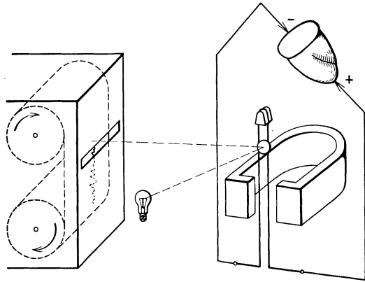
Abb. 38. Ableitung des Herzens von Basis und Spitze zu einem „Oszillographen“. Die Schleife dreht sich bei Stromfluß im Feld des Magneten. Der Lichtzeiger des Oszillographenspiegels fällt in den Spalt der Kamera, hinter welchem Bromsilberpapier abläuft.
