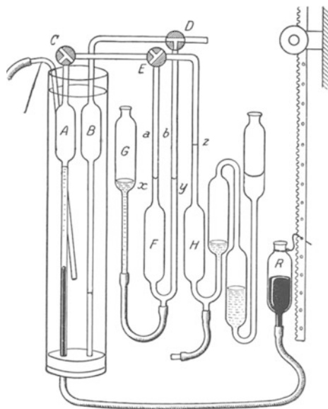
Abb. 102. Apparat zur Gasanalyse. (Nach HALDANE.) A Gasbürette (10–20 cm) in Wasserbad angeordnet mit Quecksilber als „Sperrflüssigkeit“ gefüllt. Bei entsprechender Stellung des Dreiwegehahnes C und Senkung des Überlaufgefäßes R kann das Hg unten aus der Bürette auslaufen und oben die zu analysierende Luft in dieselbe eintreten. Nach Umstellung von C wird über den entsprechend gestellten Hahn E das Gas nach F gedrückt (durch Hochheben von R !) wo \text{CO}_2 aus dem Gas durch Kalilauge gebunden wird. Der größte Teil der Lauge weicht dabei nach G aus. Nach Rücksaugung des Gasrestes in die Bürette A (so lange, bis der Laugenmeniscus wieder bei x steht!) kann die mit \text{CO}_2 gleichbedeutende Volumabnahme abgelesen werden. Nach Umstellung von Hahn E wird die \text{CO}_2 -freie Luft in H gepreßt. Die dort befindliche Pyrogalllösung bindet \text{O}_2 . Nach Rücksaugung des Gasrestes in A kann die neuerliche Volumabnahme (gleichbedeutend mit \text{O}_2 ) abgelesen werden.
