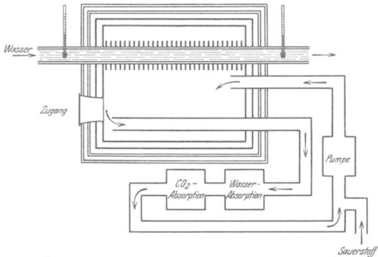
Abb. 113. Respirationcalorimeter. Das zu untersuchende Individuum wird in die gegen Wärmeabgabe entsprechend isolierte Calorimeterkammer gesetzt. Alle von ihm abgegebene Wärme wird an das die Kühlrohre durchströmende Wasser abgegeben. Aus der Temperaturdifferenz zwischen ein- und ausströmendem Wasser und der minutlichen Durchflußmenge lassen sich die in der Zeiteinheit abgeführten Calorien berechnen. Gleichzeitig kann, wie angedeutet, der Sauerstoffverbrauch und die Kohlensäureabgabe des untersuchten Organismus gemessen werden. (Nach ATWATER und BENEDICT.)
