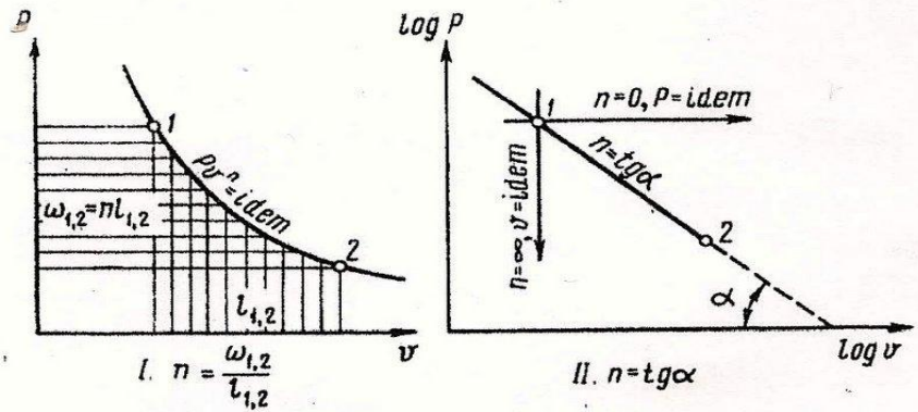
Фиг. 14. Политропа с постоянным показателем.
