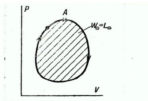
Фиг. 8. Круговой процесс (цикл).
