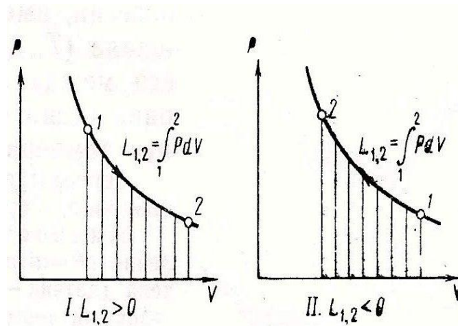
Фиг. 5. Термодинамическая работа изменения объема.
