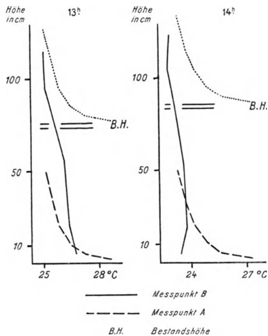
Abb. 17. Mittägliche Zustandskurven der Temperatur über nacktem Ackerboden (Meßpunkt A) und in einem Topinamburbestand (Meßpunkt B) im Mittel ausgewählter Tage. (Links Mittel für den 10.–13. August 1935 für 13 h , rechts 23.–27. August 1935 für 14 h . Die punktierte Linie stellt die bis zur Bestandshöhe gehobene Zustandskurve vom Meßpunkt A dar.)
