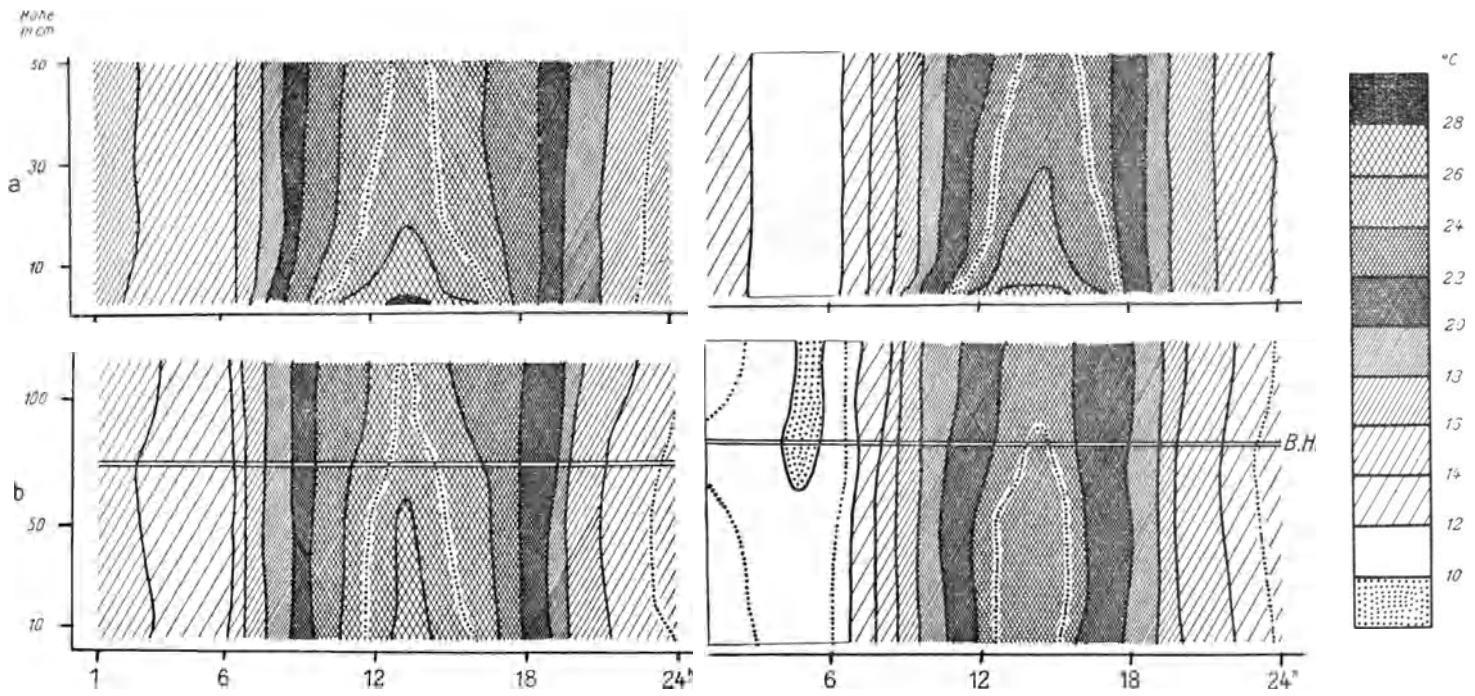
Abb. 16. Isoplethen der Temperatur über freiem Acker (a) und in einem Topinamburbestand (b) im Mittel ausgewählter Tage. Links: 10.–13. August 1935, rechts: 23.–27. August 1935. B.H. = Bestandshöhe.)
