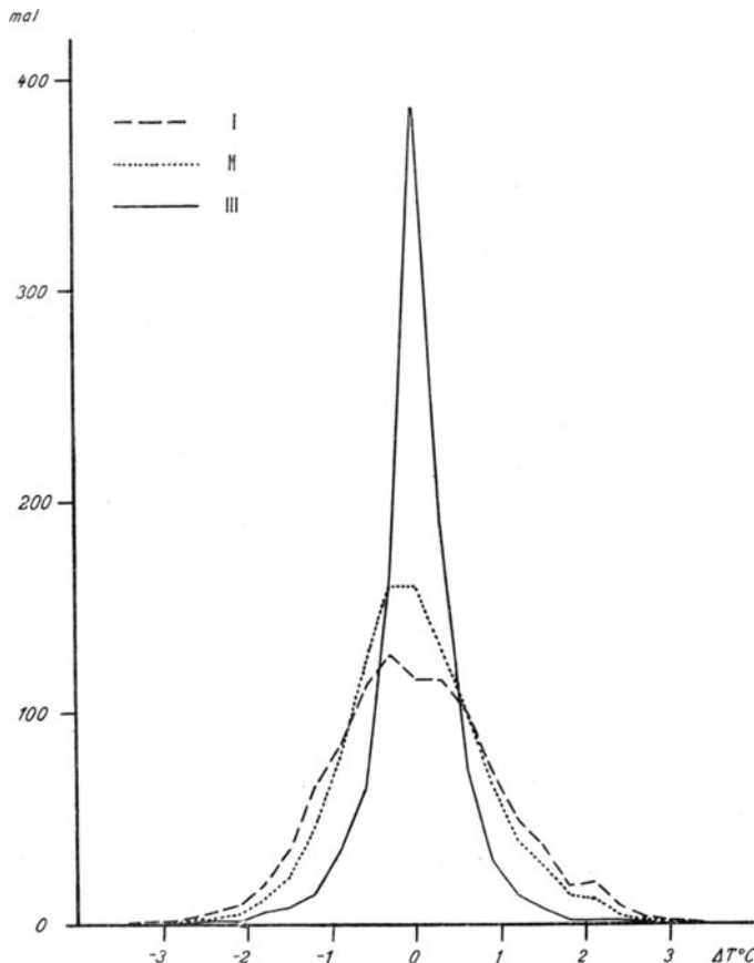
Abb. 1. Häufigkeit der Abweichungen der Minutenwerte vom zugehörigen 10-Minutenmittel für einen Sommertag und eine Winternacht auf 1000 normiert. I: Mittagsstunden des 26. Juli 1935 (5 Stunden); II: Tagesstunden des 26. Juli 1935 (10 Stunden); III: Ausstrahlungsnacht mit Schneedecke vom 25./26. Februar 1937. Zusammenfassung aller 6 Meßhöhen.
