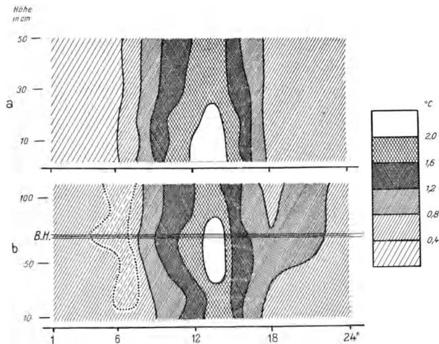
Abb. 18. Breite des Temperaturbandes über freiem Ackerland (a) und in einem Topinamburbestand (b) im Mittel des Monats August 1935 im Verlaufe eines Tages. (In b) punktiert: Bandbreite 0,6° C.)
