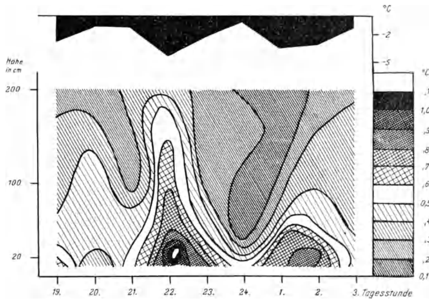
Abb. 4. Streuung der Temperatur über einer ausstrahlenden Schneeoberfläche in der Nacht vom 25./26. Februar 1937. (Abstand der Streuungsisoplethen: 0.1° C.) Oben Gang der Temperaturdifferenz zwischen 200 cm und 10 cm über dem Erdboden.).
