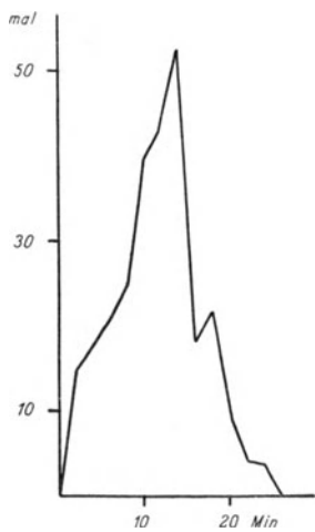
Abb. 8. Periodogramm der 15-Minutenschwankung nach den Differenzen; 7-Minutenmittel - 20-Minutenmittel für den 26. Juli 1935.
