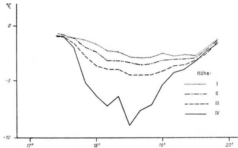
Abb. 2. Temperaturverlauf in verschiedenen Höhen über einer 6 cm hohen Schneedecke am 24. Februar 1937. (Himmelsbedeckung von 18 h –19 h : wolkenlos. Höhen der Thermometer über dem Erdboden: I: 200 cm, II: 50 cm, III: 20 cm, IV: 10 cm. IV also 4 cm über dem Schnee.)
