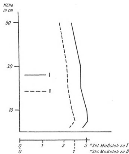
Abb. 6. Mittelwerte der Streuung (II) und der Bandbreite (I) der Temperatur am 26. Juli 1935 über nacktem Ackerboden für die 9.—16. Tagesstunde.
