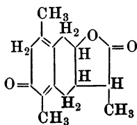
Santonin
