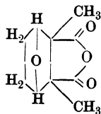
Kantharidin Zyklohexanfuranring
