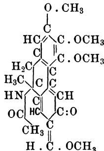
Kolchizin (Säureamid).
