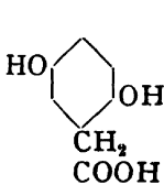
Homogentisinsäure
