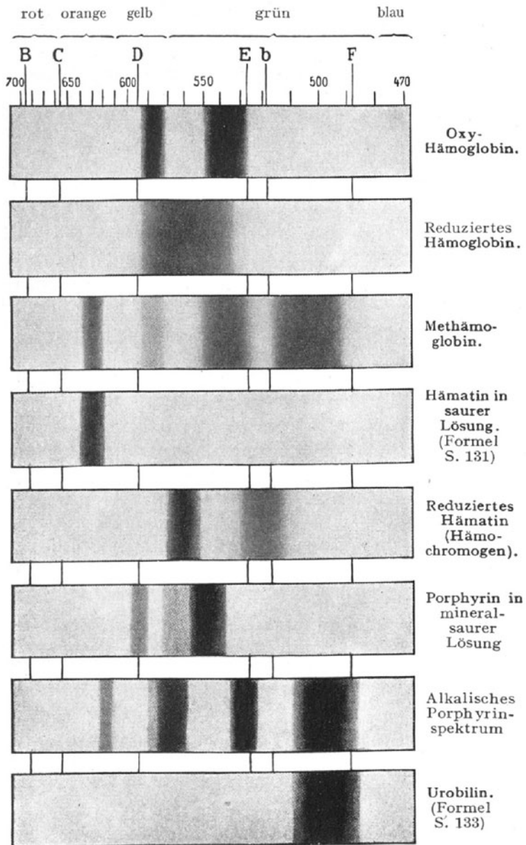
Abb. 58. Spektraltafel.
