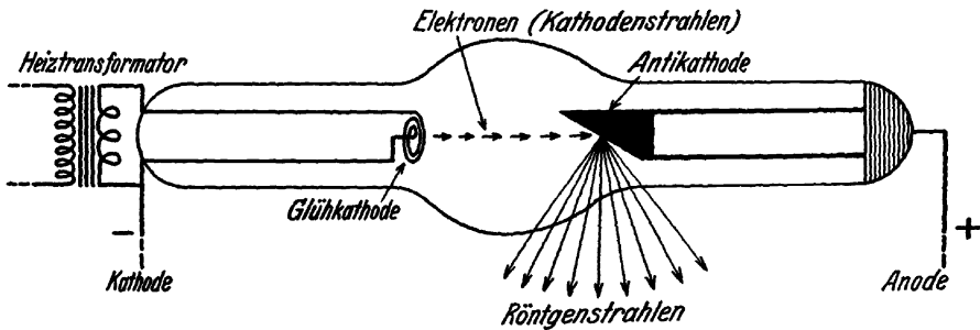
Abb. 1. Röntgenröhre.
