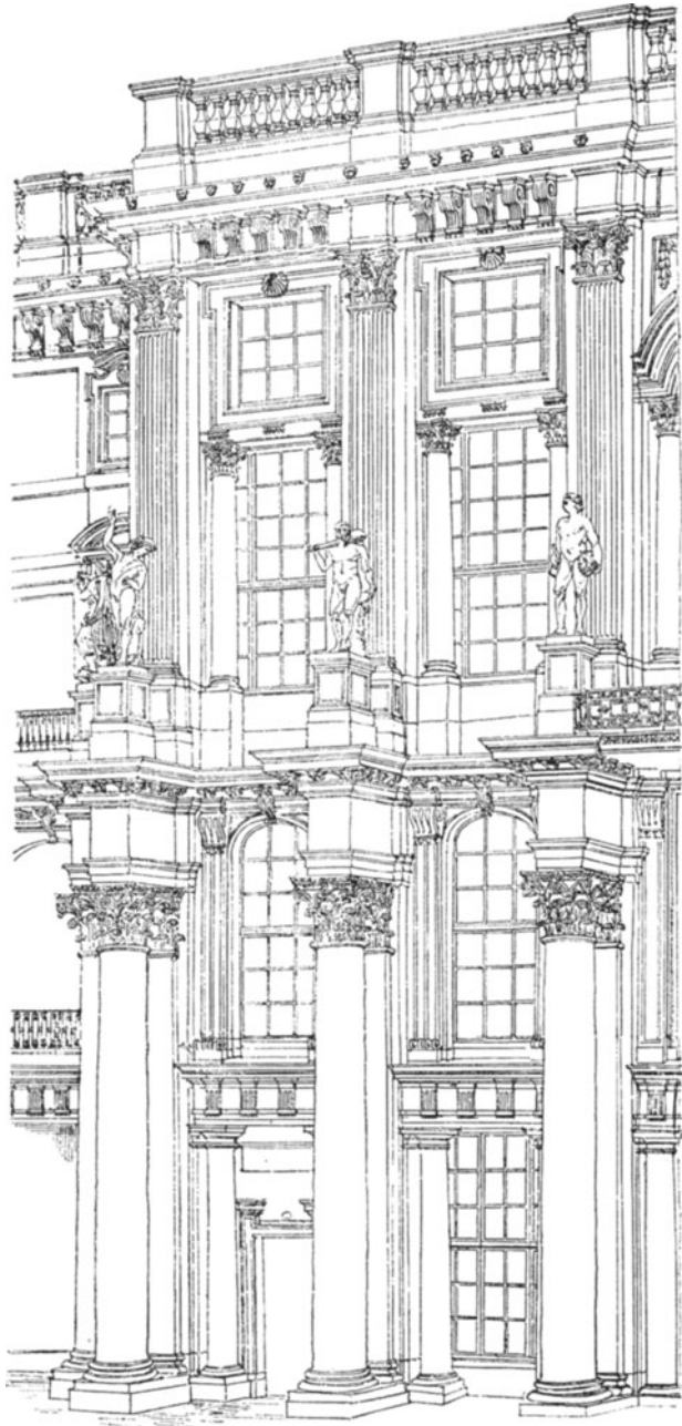
Fig. 213. Ansicht der Hoffront am grossen Treppenhaus des berliner Schlosses (n. Dohme).
