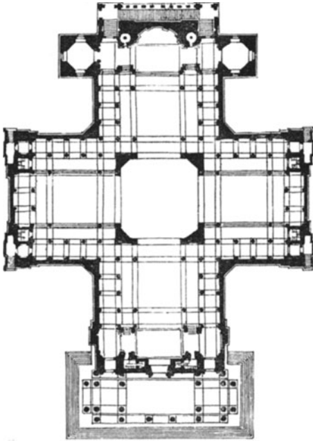
Fig. 301. Grundriss des Pantheon in Paris (n. Isabelle).
