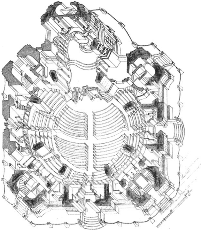
Fig. 274. Grundriss der Frauenkirche in Dresden.
