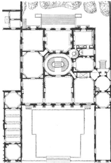
Fig. 308. Grundriss des Hauses St. Foix et Carene in Paris (n. Krafft u. Ransonette).
