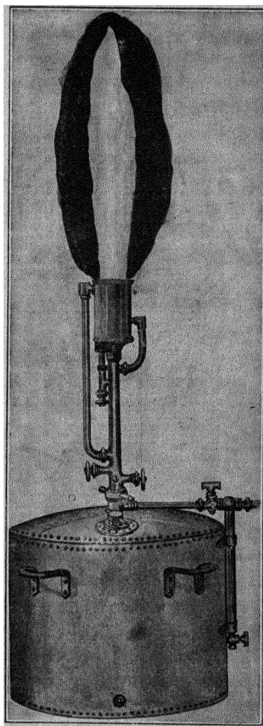
Fig. 18.—“ Lucigen ” Torch.
