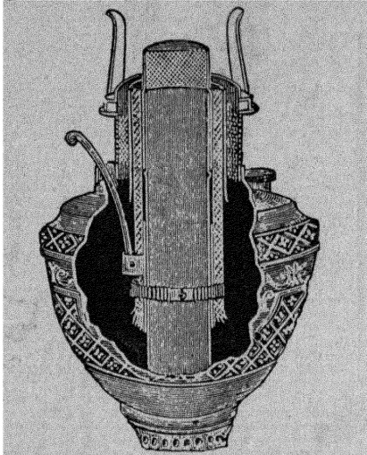
Fig. 17.—“Rochester” Kerosene Burner.
