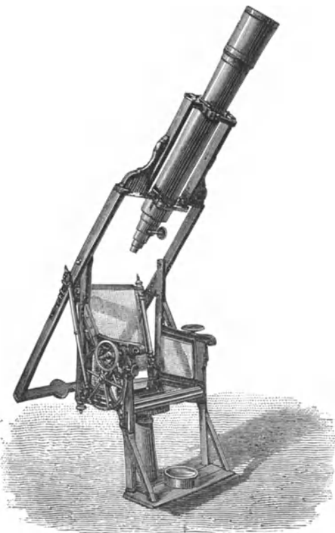
Fig. 292. Kometensucher von Merz.
