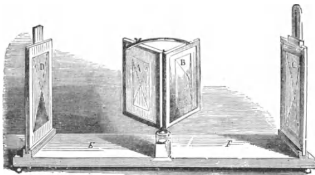
Fig. 278. Wheatstone'sches Spiegelstereoskop.
