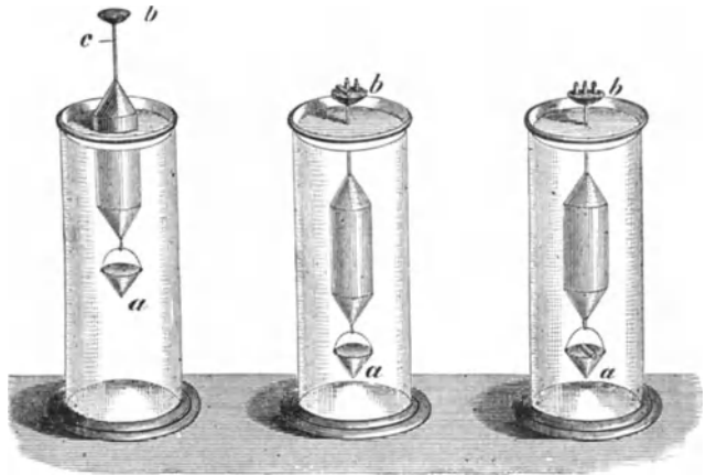
Fig. 76. Fig. 77. Fig. 78. Nicholson's Aräometer und seine Anwendung zur Bestimmung des spezifischen Gewichts.
