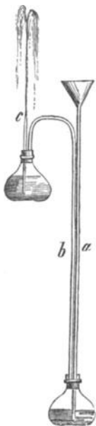
Fig. 198. Heronsbrunnen.
