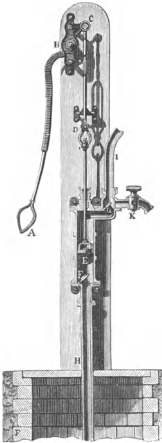
Fig. 187. Saugpumpe.
