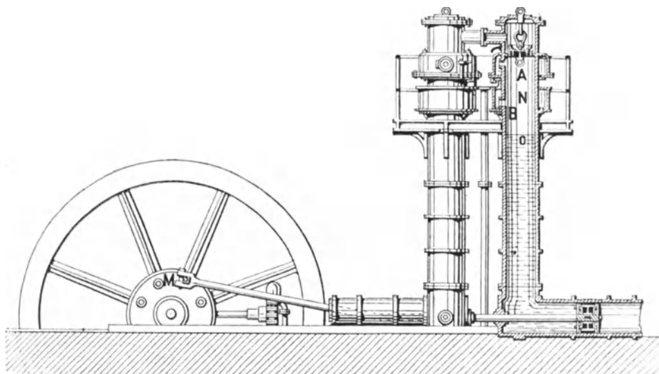
Fig. 155. Luftpumpe zur Herstellung komprimierter Luft im Mont-Cenis-Tunnel.
