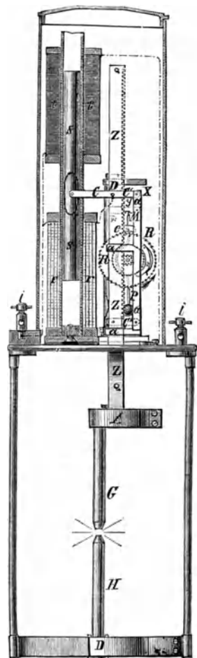
Fig. 373. Siemens-Halste-Differentialregulator im Durchschnitt.
