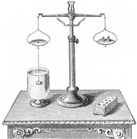
Fig. 75. Hydrostatische Wage zur Bestimmung des spezifischen Gewichts.
