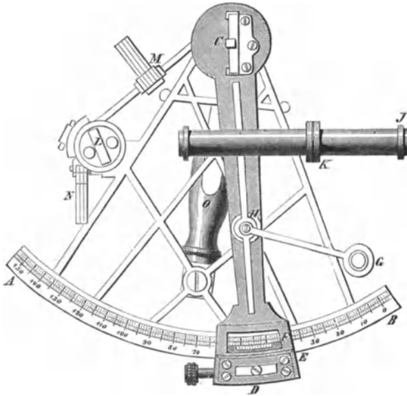
Fig. 213. Der Spiegelsextant.
