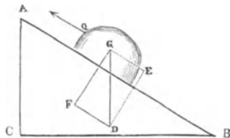
Fig. 17. Wirkungsweise der Kraft an der schiefen Ebene.
