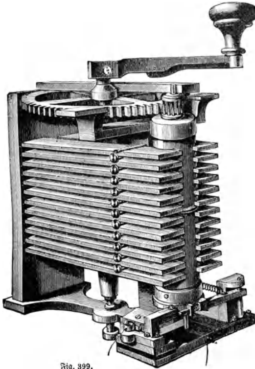
Fig. 399—401. Siemens'scher Cylinderinductor.
