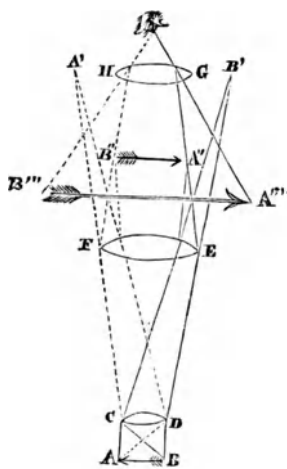
Fig. 311. Prinzip des zusammengesetzten Mikroskops.
