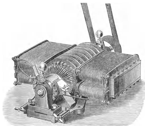
Fig. 408. Dynamoelektrische Maschine von v. Siemens-Altened.
