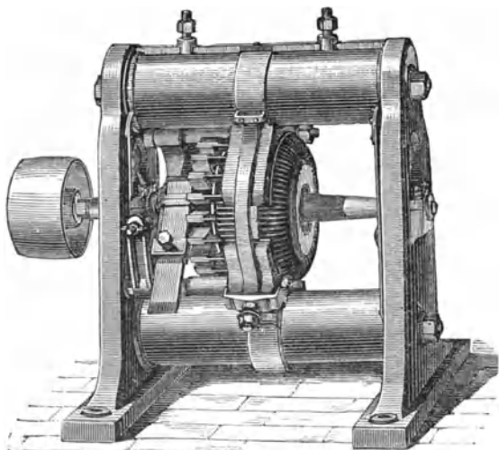
Fig. 407. Dynamoelektrische Maschine von Gramme.
