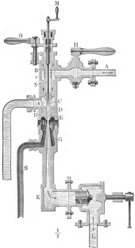
Fig. 584. Giffards Injektor.
