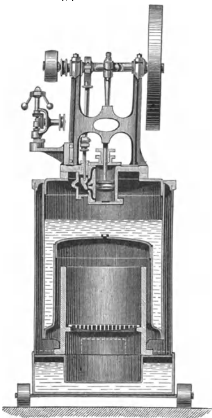
Fig. 586. Kleine Kesseldampfmaschine.
