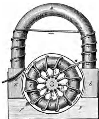
Fig. 402. Schema der Pacinottischen Ringmaschine nach Pfaunder.
