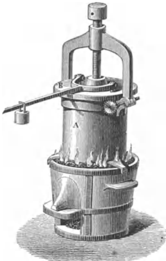
Fig. 568. Der Papinsche Topf.
