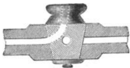
Fig. 144. Senquerbs doppelt durchbohrter Hahn.
