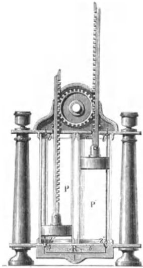
Fig. 149. Vorderansicht der zweistiefeligen Luftpumpe.
