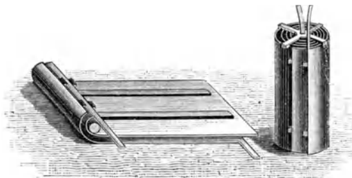
Fig. 366. Akkumulator.
