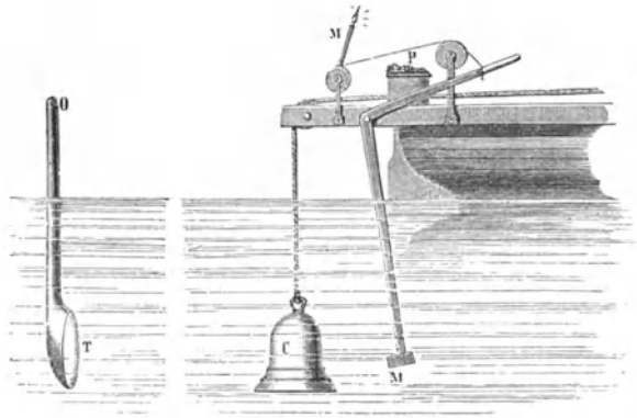
Fig. 462. Messung der Fortpflanzungsgeschwindigkeit im Wasser.
