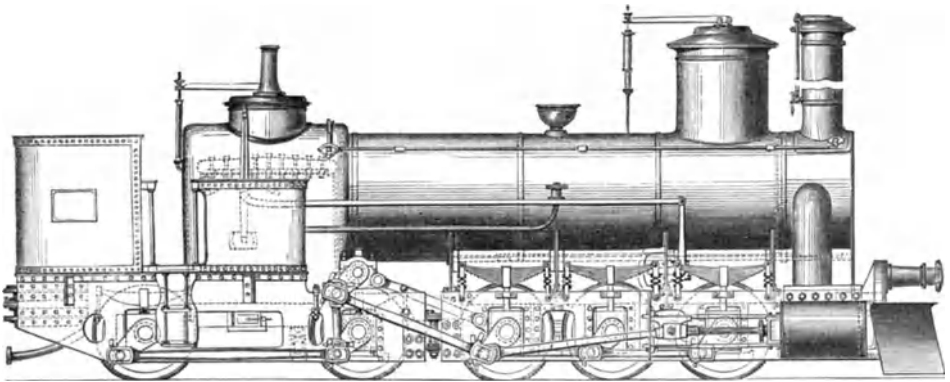
Fig. 609. Lokomotive nach Zinks System.
