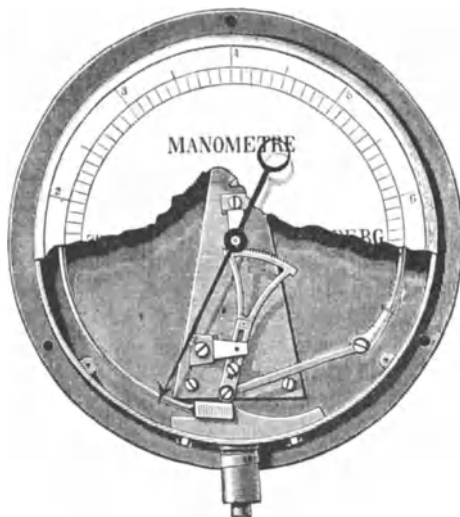
Fig. 107. Metallmanometer (System Bourdon).
