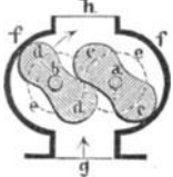
Fig. 190. Schematischer Durchschnitt einer Kapselfpumpe.
