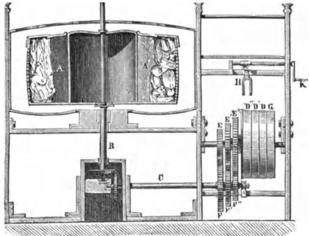
Fig. 96. Zentrifugaltrockenmaschine.
