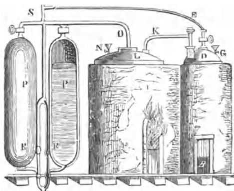
Fig. 569. Saverys Dampfmaschine.
