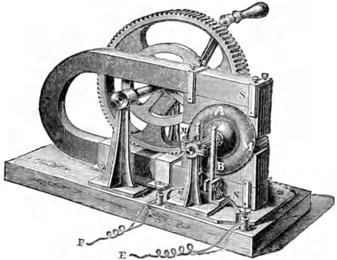
Fig. 403. Grammesche magnetoelektrische Ringmaschine für Handbetrieb.
