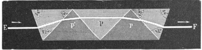
Fig. 238. Janssens geradflächiges Prismensystem.
