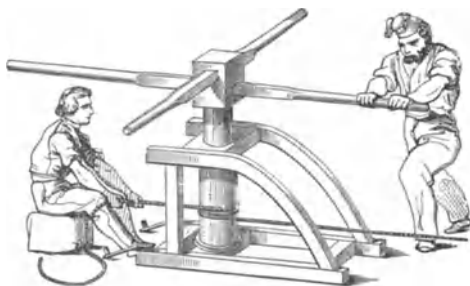
Fig. 55. Gaspel mit aufrecht stehender Welle.
