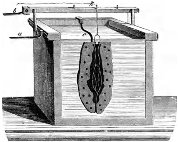
Fig. 381. Herstellung galvanoplastischer Gegenstände in Hohlform.
