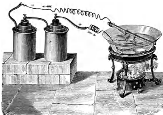
Fig. 382. Galvanische Versilberung.
