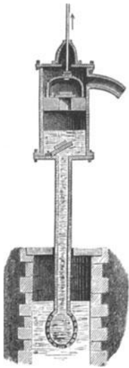
Fig. 183. Saugpumpe.
