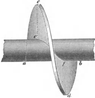
Fig. 29. Erste Form der Schiffschraube.
