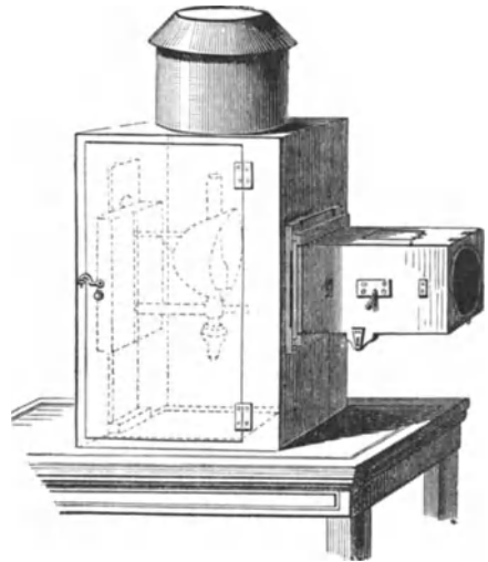
Fig. 259. Laterna magica.
