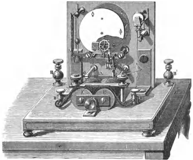
Fig. 423. Zeigertelegraph (Rückseite).
