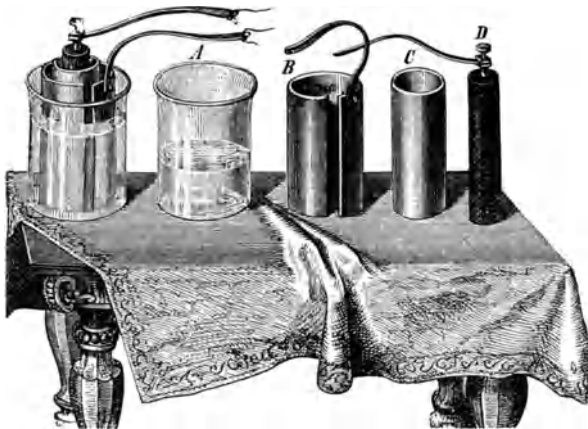
Fig. 364. Das Bunsensche Element.
