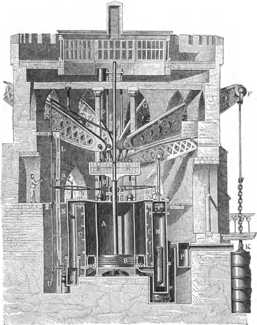
Fig. 196. Durchschnitt der Dampfmaschine Cruquius und Leeghwater.
