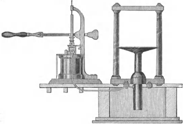
Fig. 200. Vorderansicht der hydraulischen Presse.
