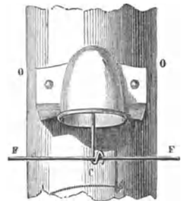
Fig. 437. Isolierende Befestigung des Telegraphendrabtes.
