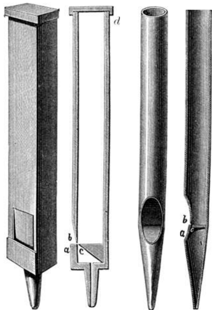
Fig. 475. Fig. 476. Fig. 477. Fig. 478. Gedackte und offene Pfeifen.
