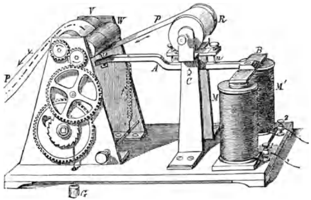
Fig. 430. Der Morse'sche Schreibapparat.
