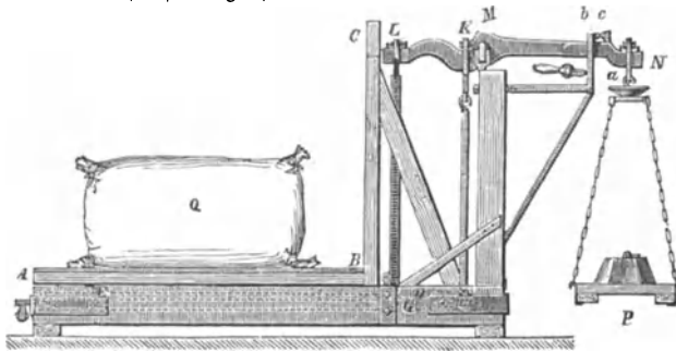
Fig. 65. Brückenwaage.
