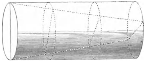
Fig. 206. Drehung der Schwingungsebene im Saccharometer.
