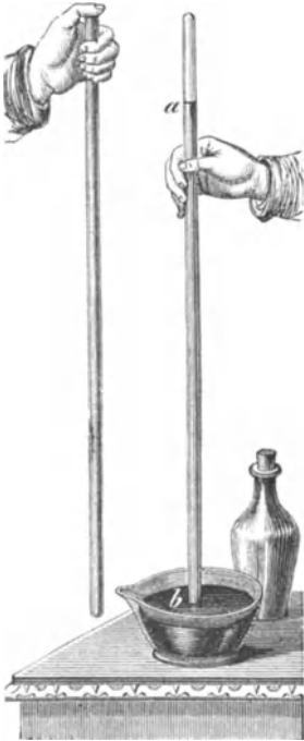
Fig. 96. Der Torricellische Versuch.
