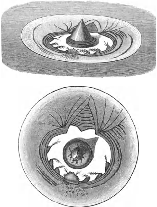
Fig. 220 und 221. Verzerrte Bilder im kugelförmigen Spiegel.
