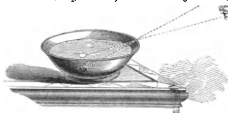
Fig. 223. Lichtbrechung durch Wasser.
