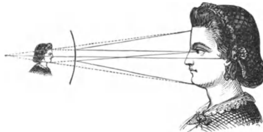
Fig. 219. Virtuelles Bild beim Konvexspiegel.
