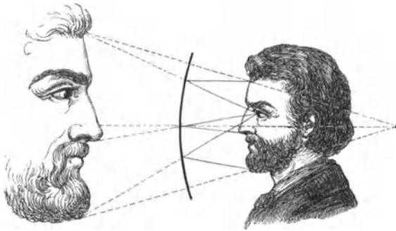
Fig. 218. Virtuelles Bild beim Konkavspiegel.
