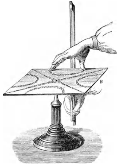
Fig. 470. Hervorbringen der Chladnischen Klangfiguren.
