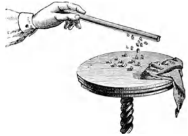
Fig. 330. Anziehende Kraft der Elektrizität.
