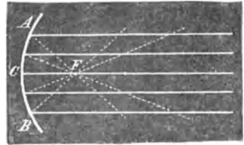
Fig. 215. Zurückwerfung parallel auffallender Strahlen durch den Hohlspiegel.
