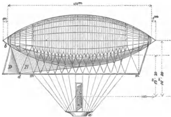
Fig. 134. Luftschiff von Dupuy de Lôme.
