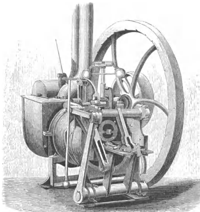
Fig. 591. Ottos Heißluftmaschine. Vorderansicht.
