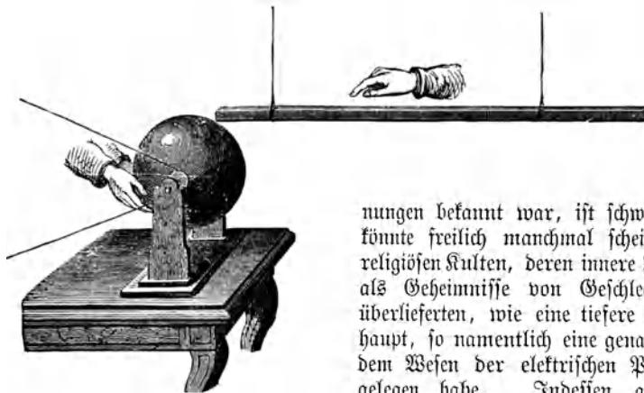
Fig. 329. Erste Elektrifiziermaschine Otto von Guericke's.
