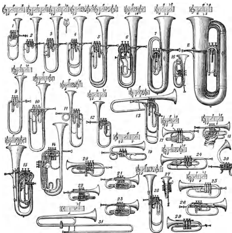
Fig. 540. Metallblasinstrumente von A. Sax in Paris. — 1 Saxhorn (sharp). 2 Sopranhorn. 3 Althorn. 4 Alttromba. 5 Baritontromba. 6 Basshorn. 7 Kontrabaß. 8 Schwerer Kontrabaß. 9 Kontra-Alt. 10 Trombone à pistons. 11 Trompette à cylindres. 12 Cornet à pistons. 13 Trombone à pistons. 14 Saxtrombone mit sieben Pistons. 15 Bass-Saxhorn. 16, 17 und 18 Cornet à pistons. 19 Cornet à pistons. 20 Saxhorn. 21 Cornet à pistons à deux clés. 22 Saxtromba alto à clés et à pistons. 23 Cornet à pistons. 24 Trompette à cylindres. 25–30 Saxhorn et Instruments à pistons avec addition de clés. 31 Trombone (Posaune).
