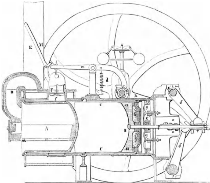
Fig. 593. Ericssons Heißluftmaschine. Vertikaldurchschnitt.
