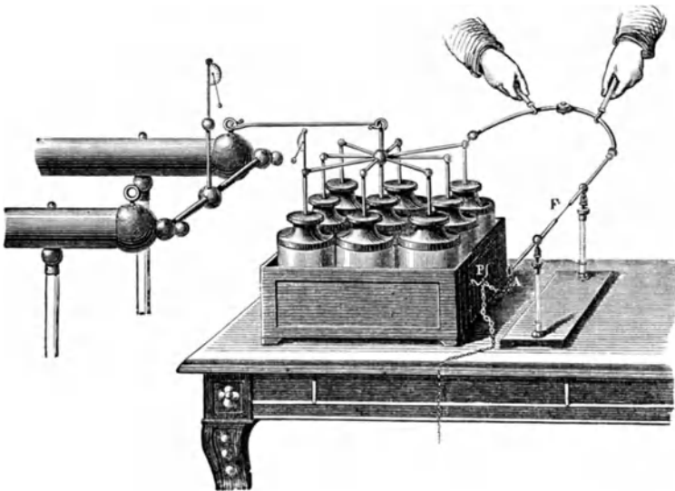
Fig. 339. Elektrische Batterie.
