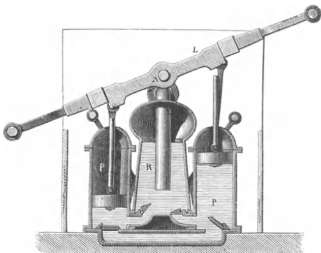
Fig. 199. Feuerspritze im Durchschnit.
