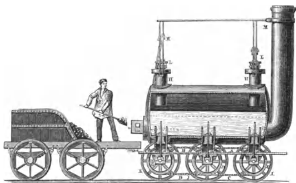
Fig. 608. Georg Stephenson's Lokomotive von 1814.
