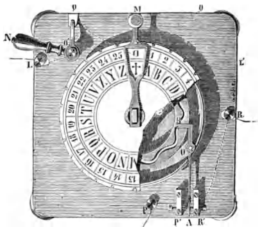
Fig. 425. Der Manipulator.
