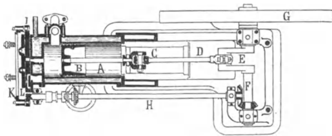
Fig. 590. Durchschnittsanficht von Ottos neuestem Gasmotor.
