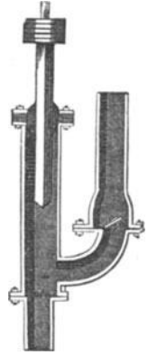
Fig. 188. Druckpumpe mit Mönchskolben.
