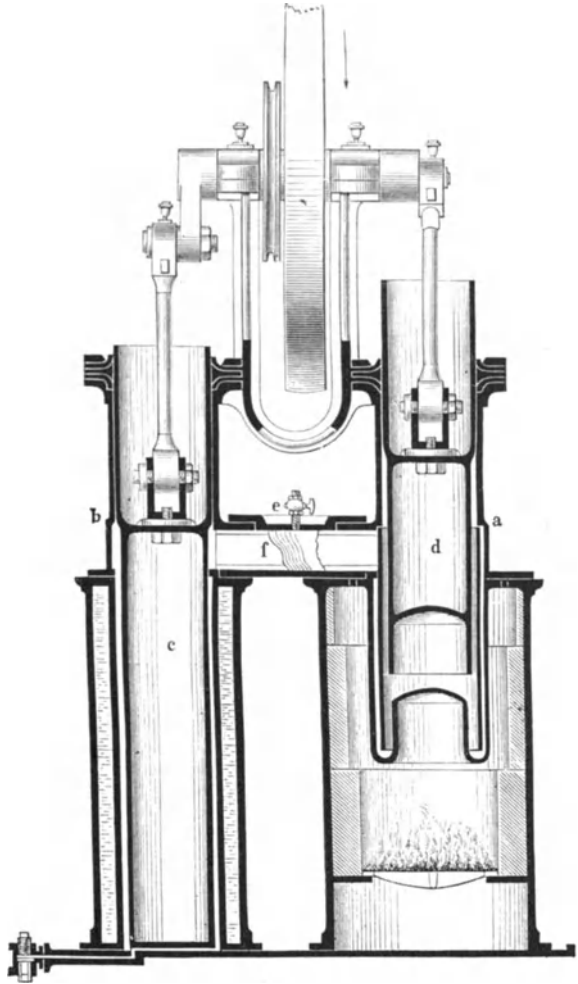
Fig. 596. Die Moberger Luftmaschine.
