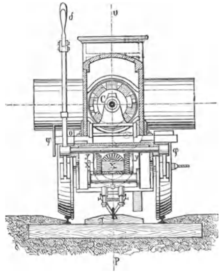
Fig. 410. Elektrische Lokomotive im Querschnitt.
