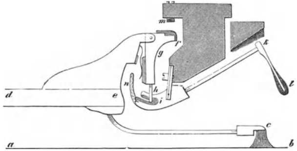
Fig. 511. Niederschlagende Mechanik.
