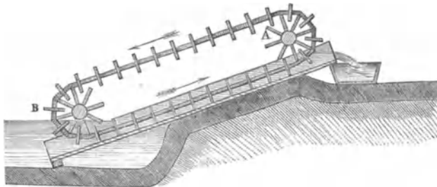
Fig. 176. Paternosterwerk.
