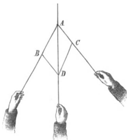
Fig. 10. Parallelogramm der Kräfte. AB und AC eigentlich wirkende Kräfte (sog. Seitenkräfte), AD die Resultante oder Mittelkraft aus beiden.
