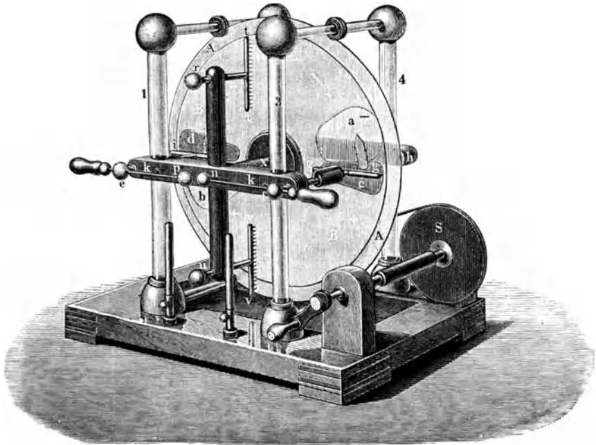
Fig. 341. Influenz-Elektrifiziermaschine von Holz. (Vorderansicht.)
