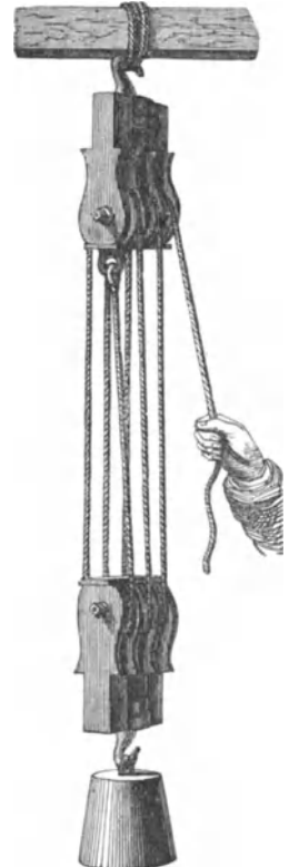
Fig. 54. Flasenzug mit nebeneinander liegenden Rollen.
