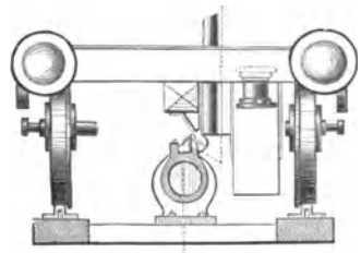
Fig. 160. Vorderansicht der Eisenbahn.
