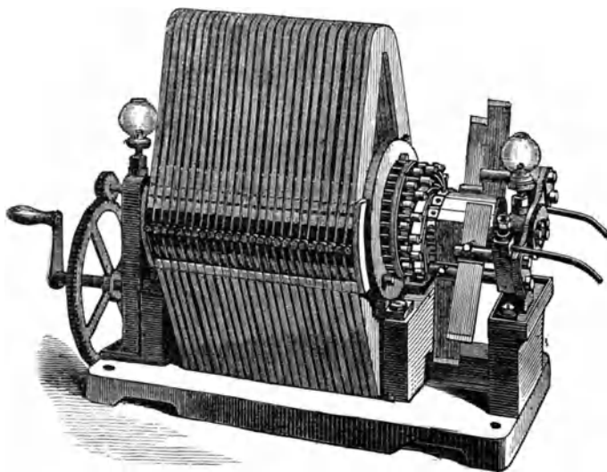
Fig. 405. Magnetoelektrische Maschine von v. Hefner-Alteneck.
