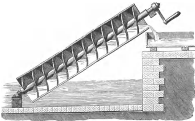
Fig. 177. Wasserschnecke.
