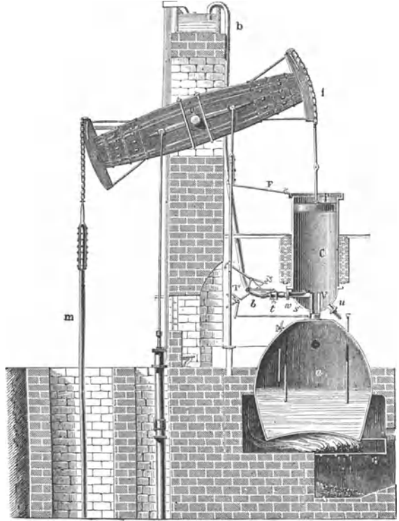
Fig. 570. Newcomens Dampfmaschine.
