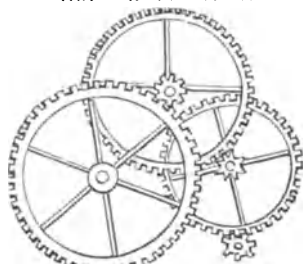
Fig. 49. Umsehung der Zahnräder.
