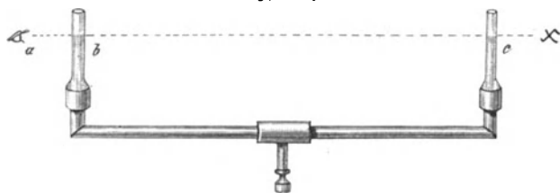
Fig. 166. Kanalwasserwage. a Auge, bc Oberfläche des Wassers, x Gegenstand.
