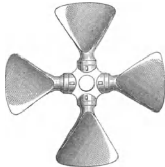
Fig. 32. Viergängige Schraube des „Great Britain“.
