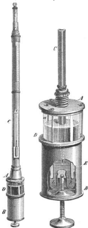
Fig. 100. Fortins's Gefäßbarometer.
