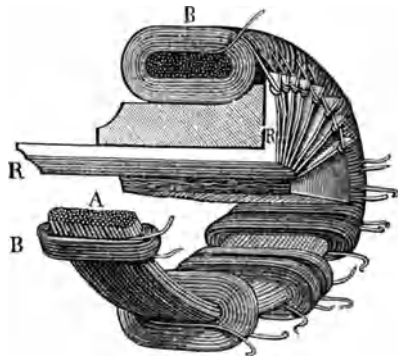
Fig. 404. Ring der Grammeschen Maschine durchschnitten.
