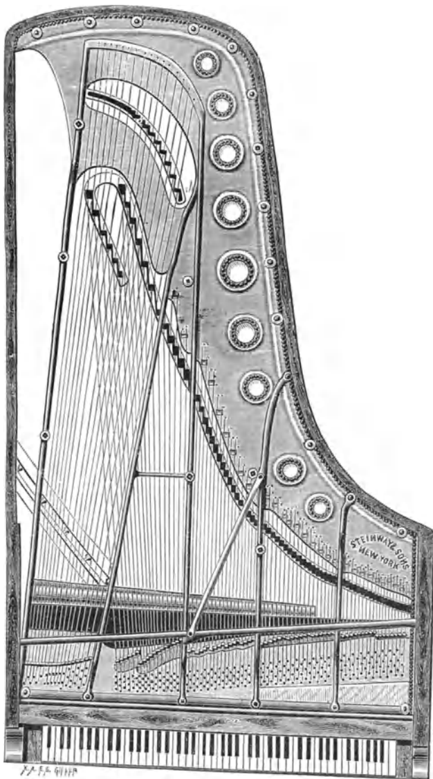
Fig. 515. Das Eisengerippe eines neueren Konzertflügels, von oben gesehen.
