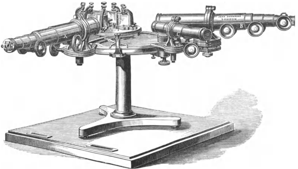
Fig. 241. Großes Spektroskop der Sternwarte zu Kiew.
