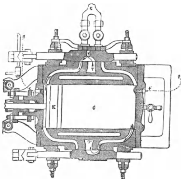
Fig. 588. Lenoir's Gasmaschine. Horizontaldurchschnitt.
