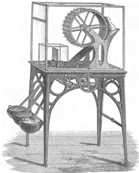
Fig. 72. Französische Goldwage.
