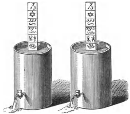
Fig. 415. Hydraulischer Telegraph.
