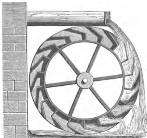
Fig. 172. Oberschlächtiges Wasserrad.
