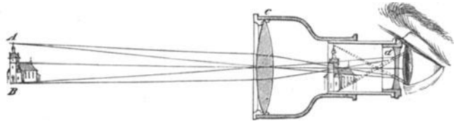
Fig. 286. Holländisches Fernrohr.
