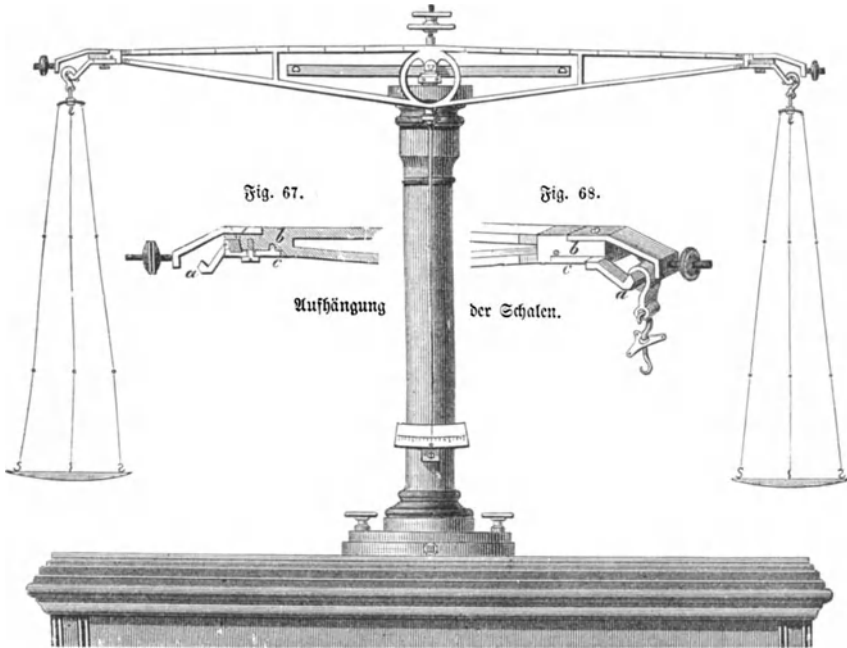
Fig. 69. Chemische Wage.
