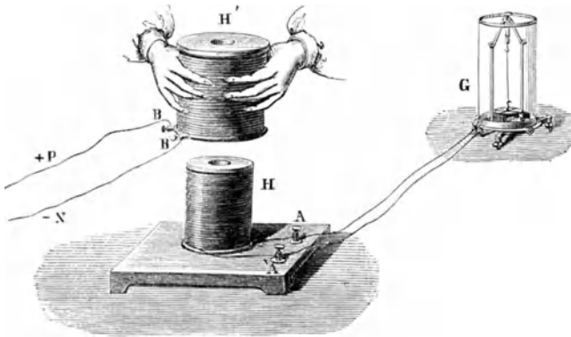
Fig. 393. Induzierte Ströme.
