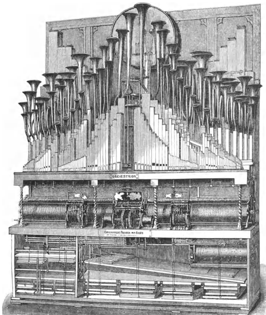
Fig. 647. Automatisches Musikspielwerk von M. Welte in Böhrenbach. Internationale Ausstellung zu London 1862.
