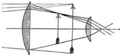
Fig. 288. Campanisches Okular.
