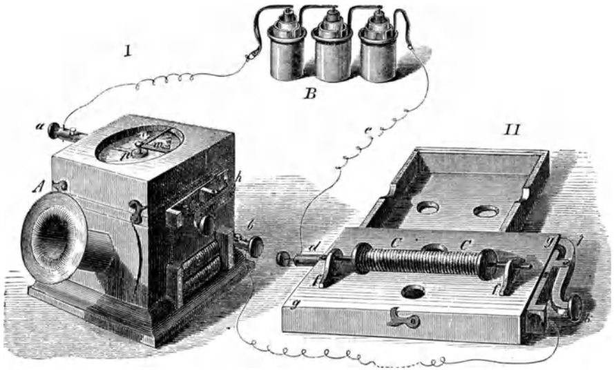
Fig. 480. Das Telephon.
