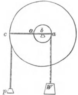
Fig. 47. Zur Theorie des Rades an der Welle.
