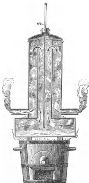
Fig. 560. Bestimmung des Siedepunktes der Thermometerskala.
