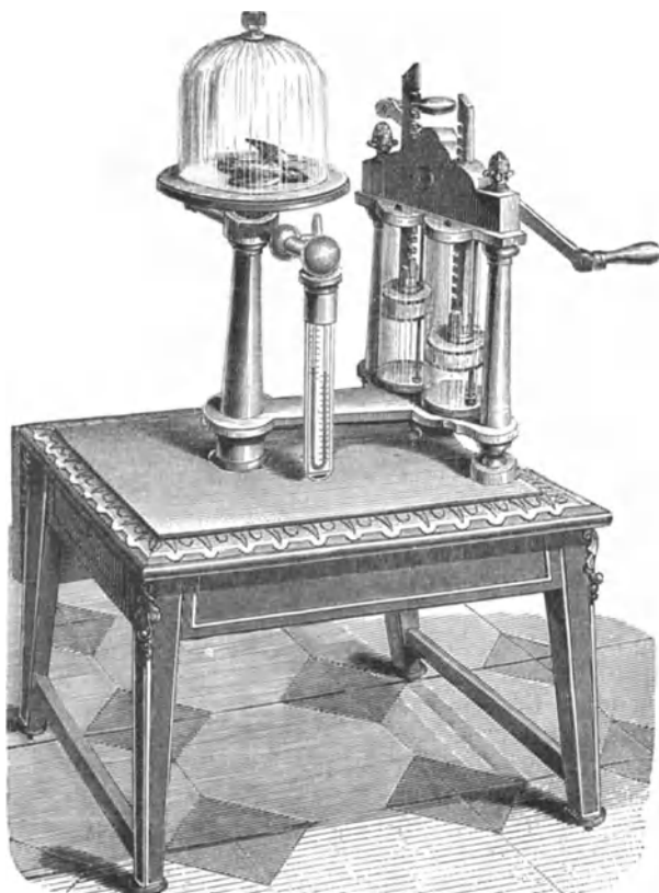
Fig. 145. Zweistufige Luftpumpe.
