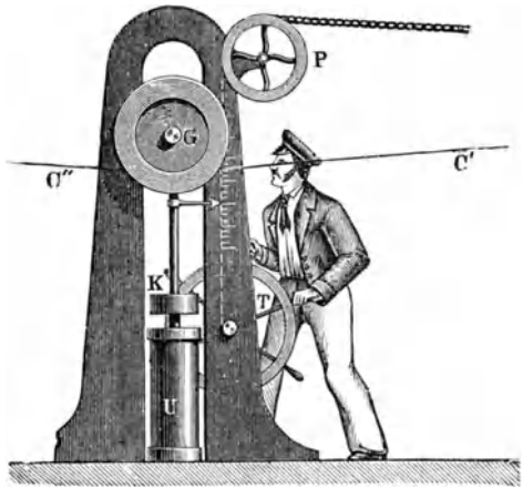
Fig. 441. Dynamometer und Bremsvorrichtung.
