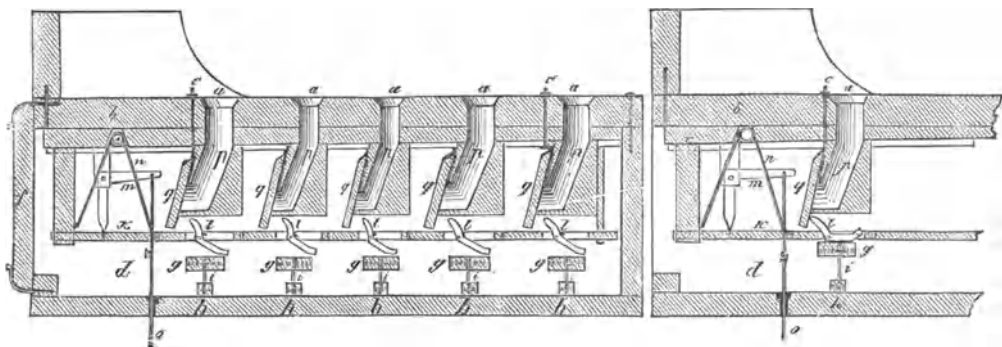
Fig. 550 und 551. Saphnenlade für Orgelwerke von Randebrod.
