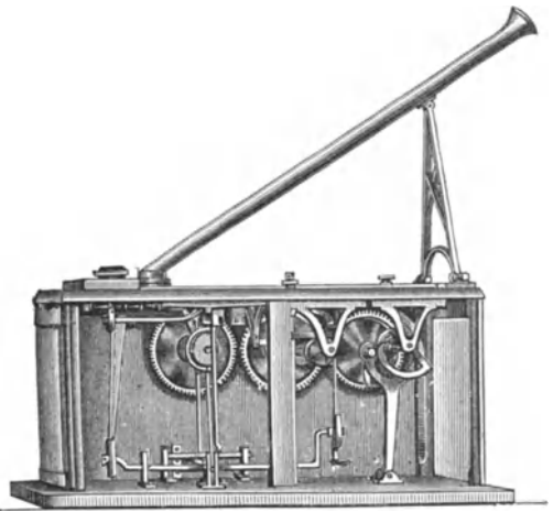
Fig. 73. Goldwaage von Stülkraft.
