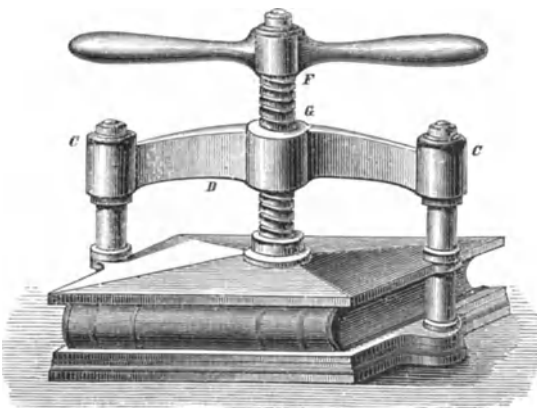
Fig. 24. Schraubenpresse mit unbeweglicher Mutter.
