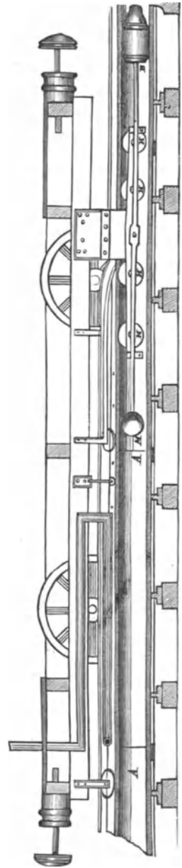
Fig. 157. Die atmosphärische Götterbahn. Längsdurchschnitt.
