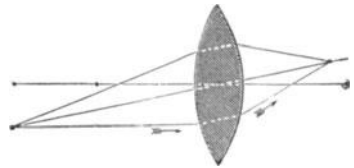
Fig. 246. Wirkung der Linse auf seitwärts auffallende Strahlen.
