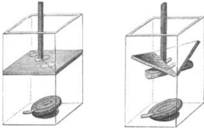
Klappenkolben.
