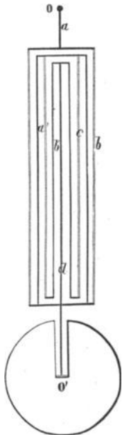
Fig. 87. Kompensationspendel.
