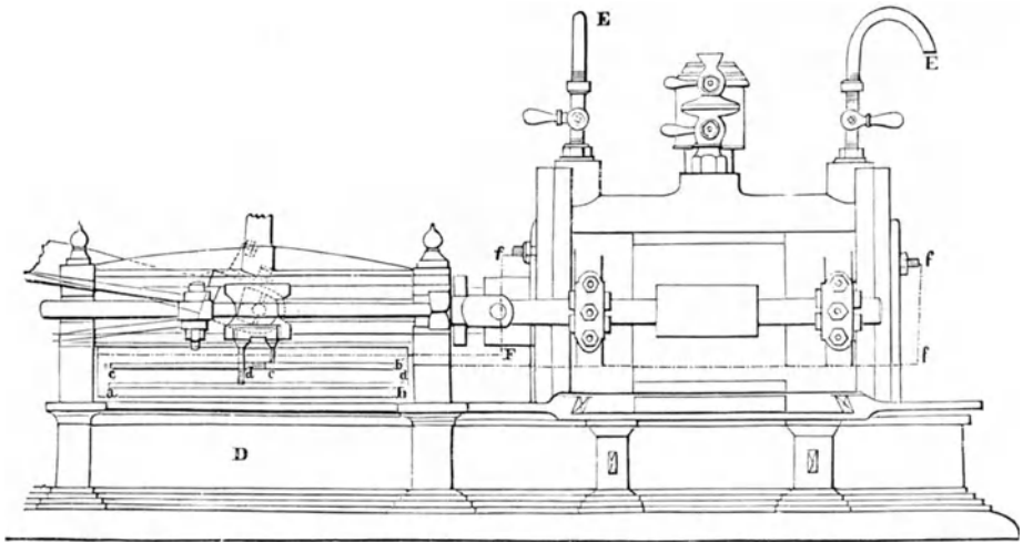
Fig. 587. Lenoirs Gasmaschine. Seitenansicht.
