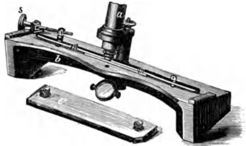
Fig. 327. Mikroskop des Fleischbeschauers.
