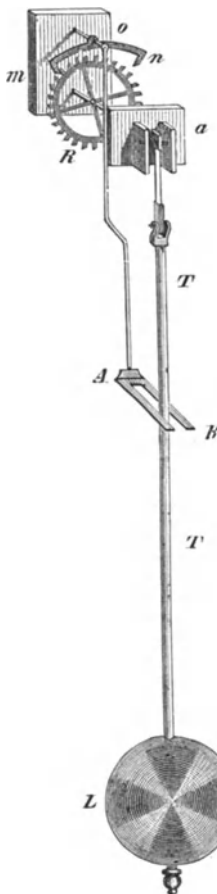
Fig. 85. Uhrpendel.
