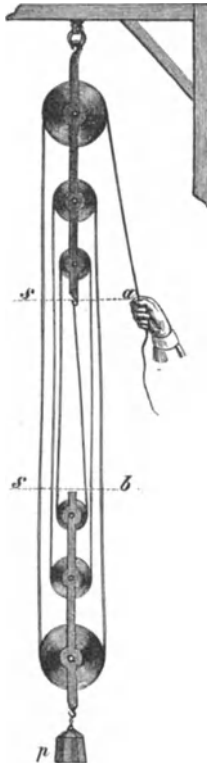
Fig. 53. Flasenzug mit drei festen und drei beweglichen Rollen.
