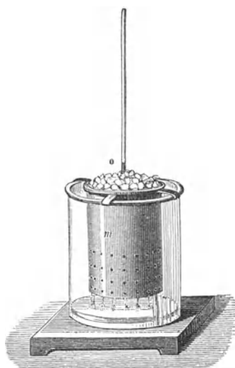
Fig. 559. Bestimmung des Nullpunktes der Thermometerskala.
