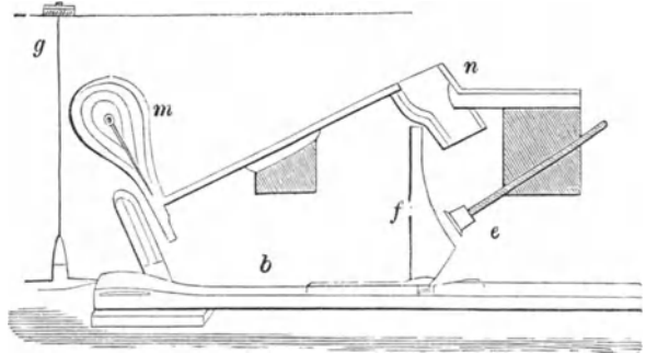
Fig. 507. Englische Mechanik.
