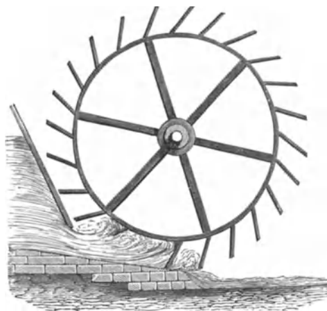
Fig. 173. Unterschlächtiges Wasserrad.
