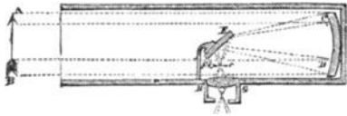
Fig. 299. Newtons Spiegelteleskop.
