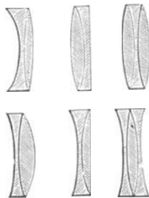
Fig. 254. Achromatische Linsen.
