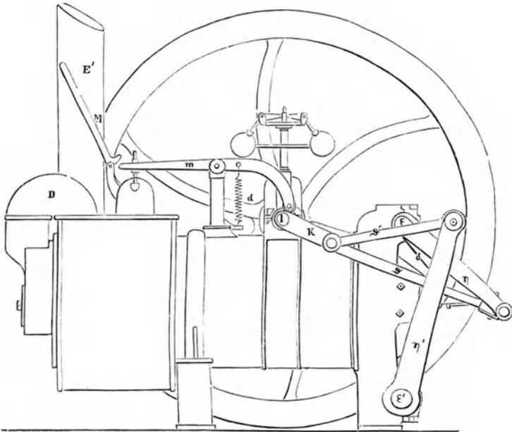
Fig. 592. Ericsson's Heißluftmaschine. Seitenansicht.
