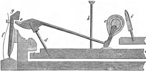
Fig. 506. Wiener Mechanismus.
