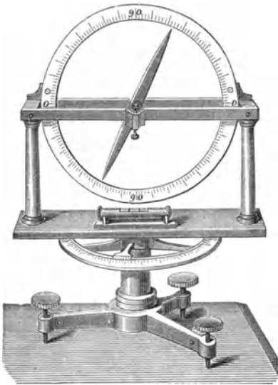
Fig. 455. Inklinatorium.
