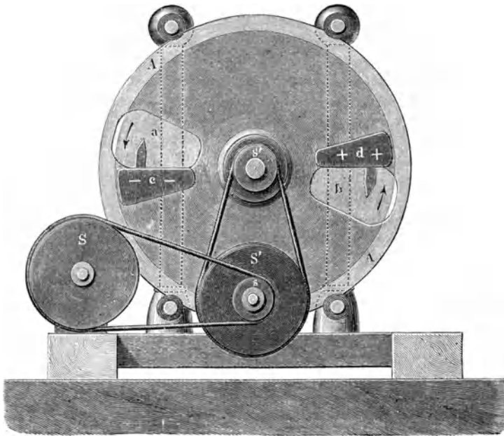
Fig. 342. Influenz-Elektrifiziermaschine von Holtz. (Sinteransicht.)
