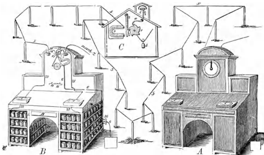
Fig. 421. Schema des Zeigertelegraphen von Wheatstone.
