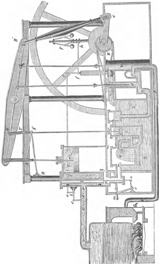
Fig. 573. Watts doppelwirkende Dampfmaschine in schematischer Uebersicht
