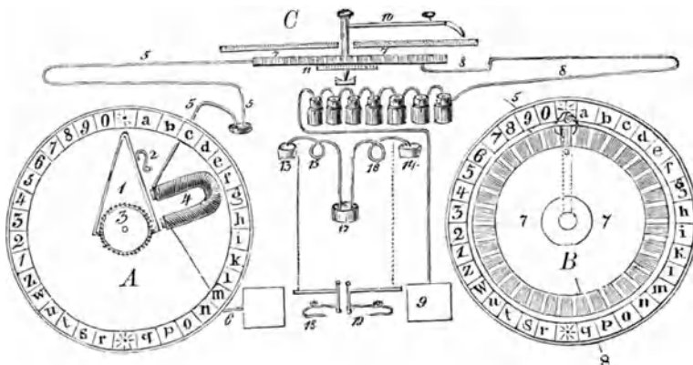
Fig. 422. Meldescheibe und Zeichengeber des Wheatstone'schen Zeigertelegraphen.
