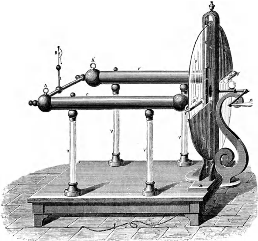
Fig. 334. Scheibenelektrifiziermaschine.
