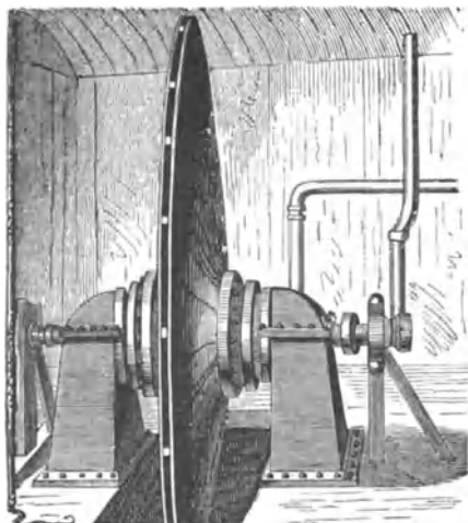
Fig. 161. Luftpumpe der pneumatischen Patentbeförderung in London.
