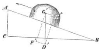
Fig. 18. Wirkungsweise der Kraft an der schiefen Ebene.
