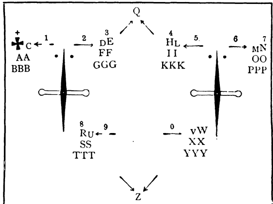
Fig. 420. Doppelnadeltelegraph von Wheatstone und Coote.
