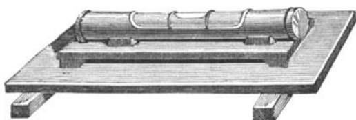
Fig. 167. Wasserwage.
