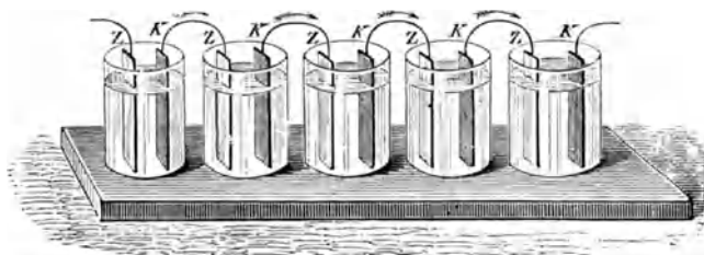
Fig. 362. Der Becherapparat.
