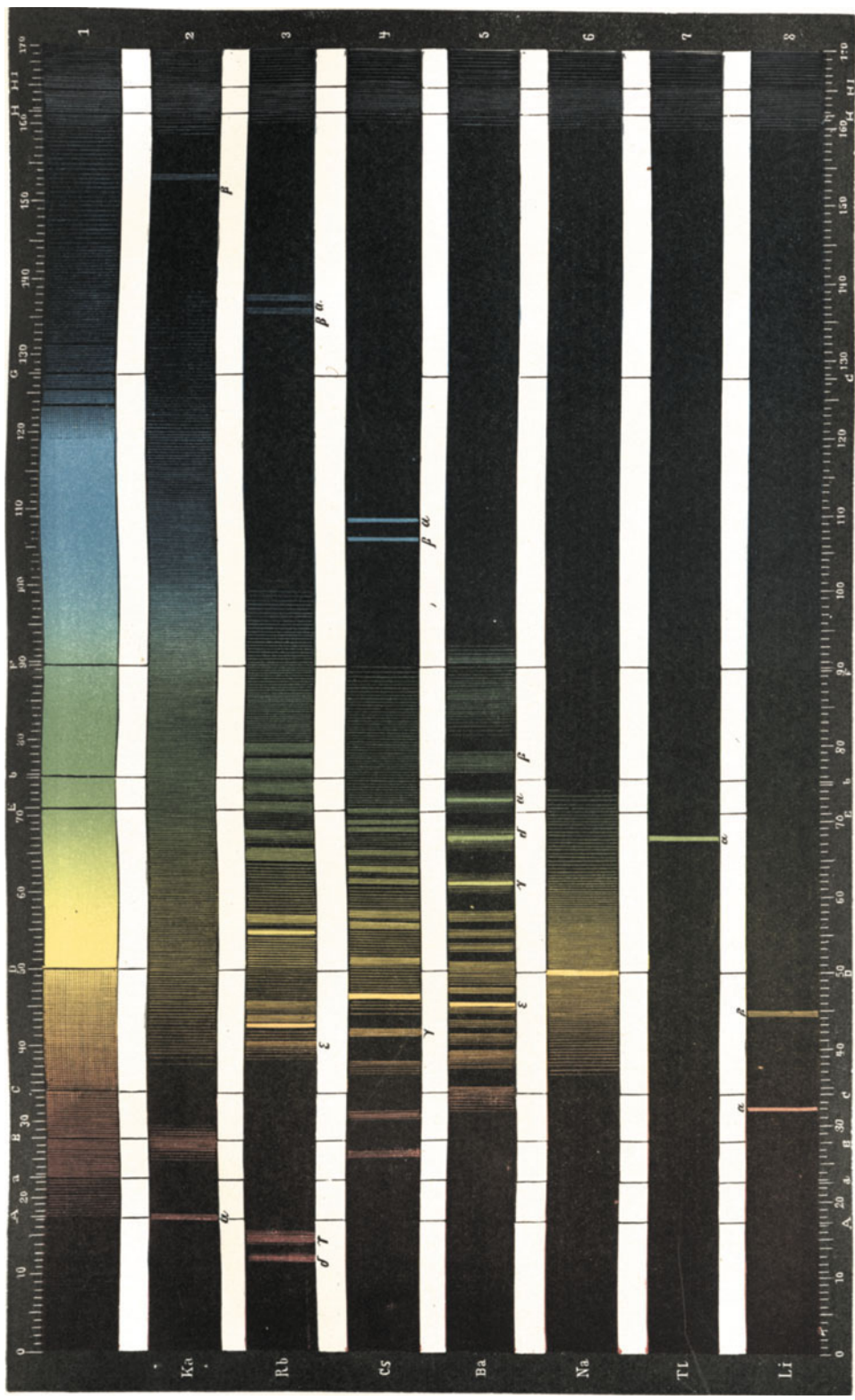
Zusammenstellung des Sonnenspektrums (1), mit den Spektren der Flammen von Kalium (2), Rubidium (3), Cäsium (4), Baryum (5), Natrium (6), Thallium (7), Lithium (8).
