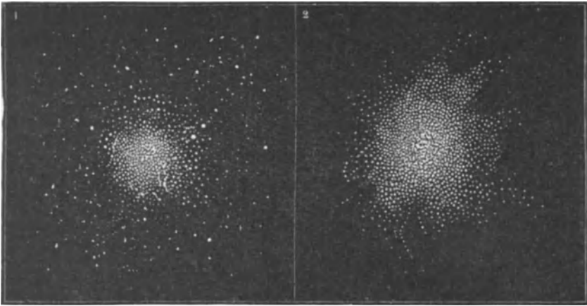
Fig. 306. Sternhaufen, 1 in der Waage, 2 im Herkules.
