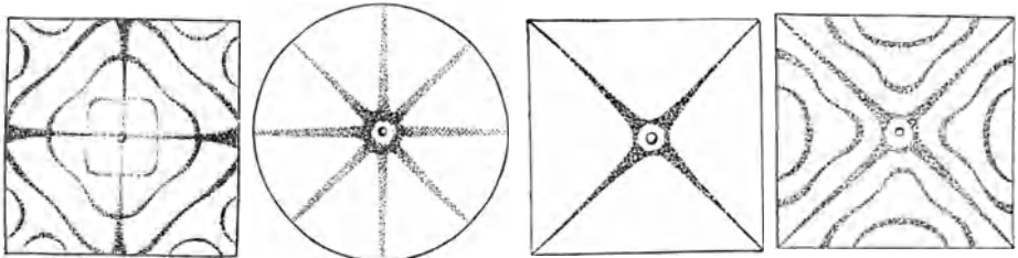
Fig. 471—474. Chladnische Klangfiguren.
