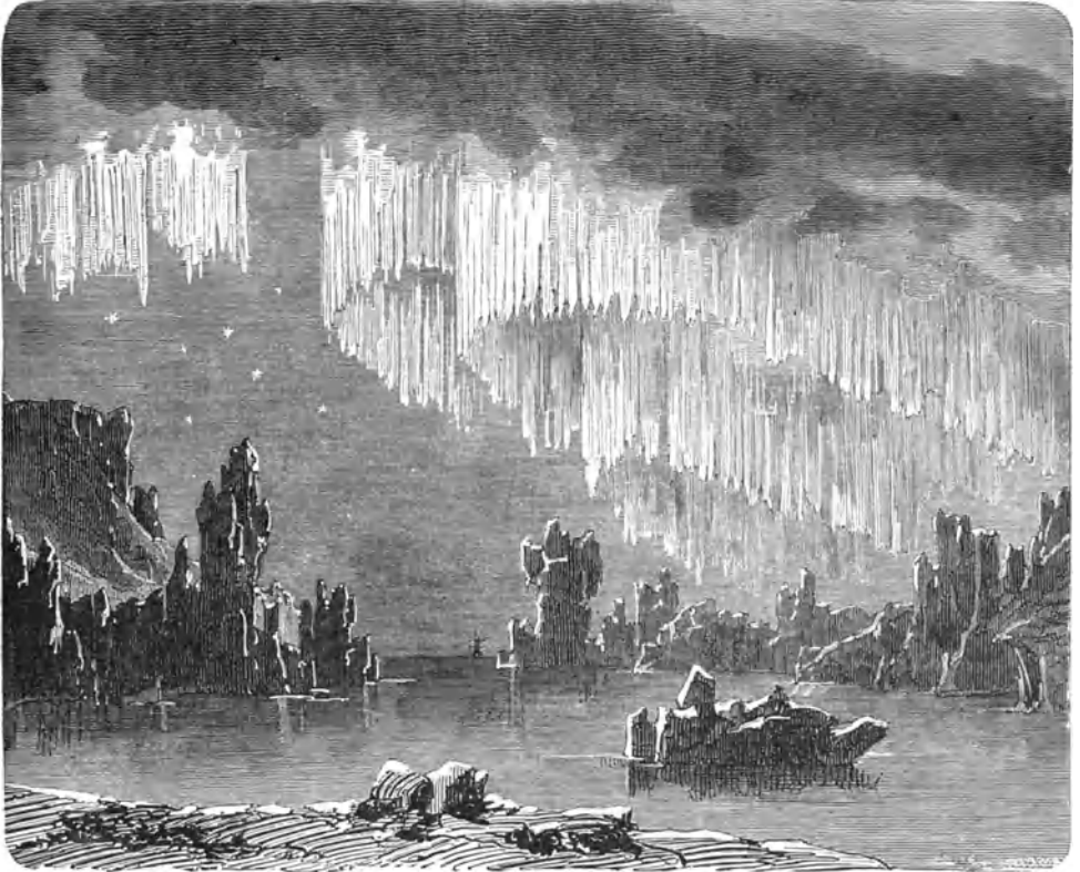
Fig. 457. Nordlichterscheinung in dem Eismeer.
