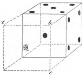
Fig. 273. Würfel von vorn betrachtet.
