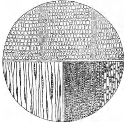
Fig. 320. Anatomie des Lannenhölzes; obere Hälfte Querschnitt; untere Hälfte rechts Radialschnitt; links Tangentialschnitt.
