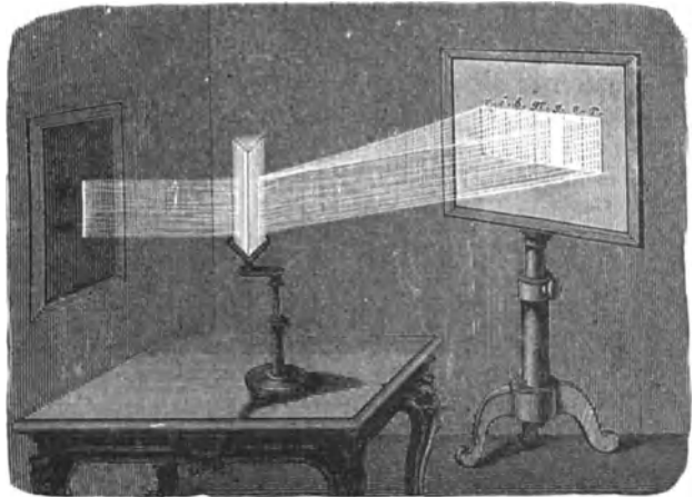
Fig. 231. Zerlegung des Sonnenlichtes durch das Prisma.
