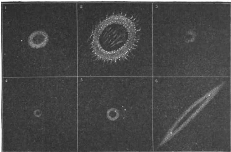
Fig. 307. Ringförmige Nebel in der Leier (1 nach Herschel, 2 nach Rosse), im Schwan (3), im Ophiuchus (4), im Storpion (5), bei Gamma in der Andromeda.
