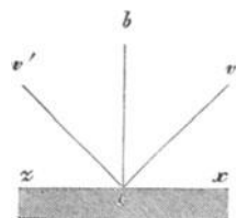
Fig. 208. Reflexion des Lichtes.
