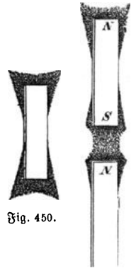
Fig. 450. Mitteiling des Magnetismus durch Verteilung.
