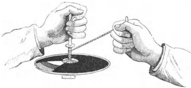
Fig. 269. Zur Erklärung des Farbkreisels.
