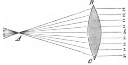
Fig. 245. Wirkung der biconvexen Linse auf gerade auffallende Strahlen.
