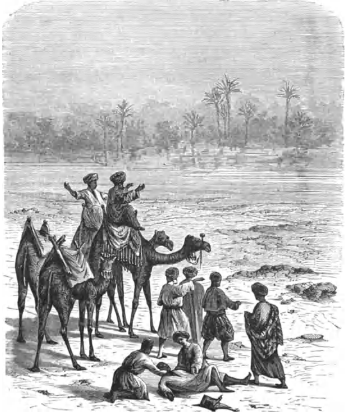
Fig. 225. Fata morgana.
