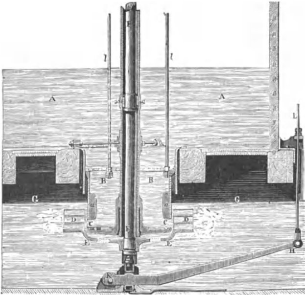
Fig. 174. Vertikaldurchschnitt einer Turbine.
