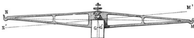
Fig. 70. Der Wagebalken.
