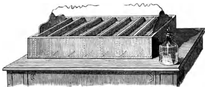
Fig. 361. Der Trogapparat.
