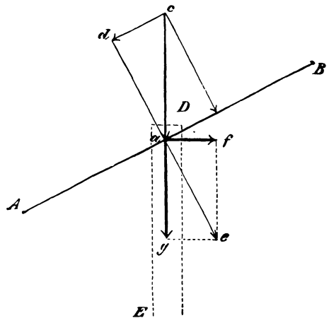
Fig. 84. Wirkung des Windes auf den Flügel der Windmühle.
