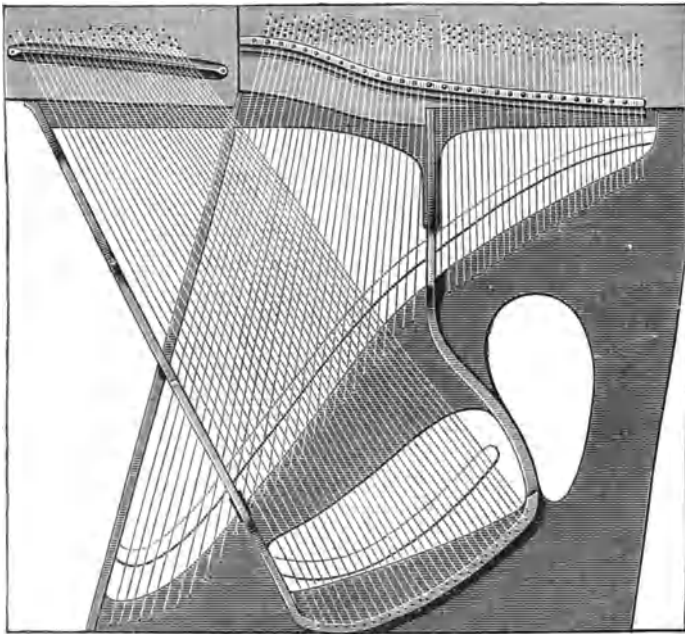
Fig. 514. Grundkörper und Saitenbezug eines Pianinos von Steinway.
