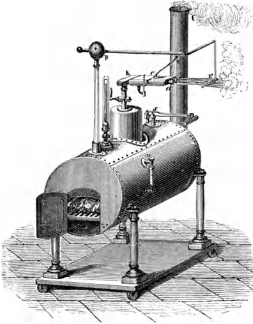
Fig. 335. Armstrongs Dampfelektrifiziermaschine.
