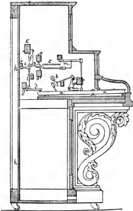
Fig. 516. Seitendurchschnitt des Adiaphons.
