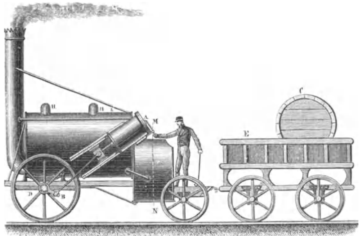
Fig. 605. Stephensons Dampflokomotive die „Rakete“.
