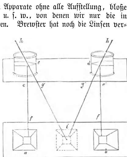
Fig. 280. Prinzip des stereoskopischen Apparates.
