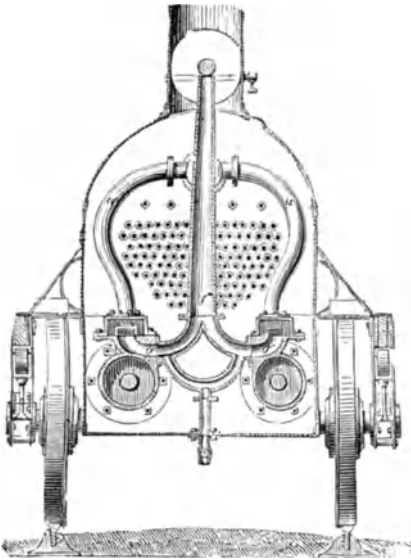
Fig. 607. Vorderer Querschnitt einer Lokomotive.
