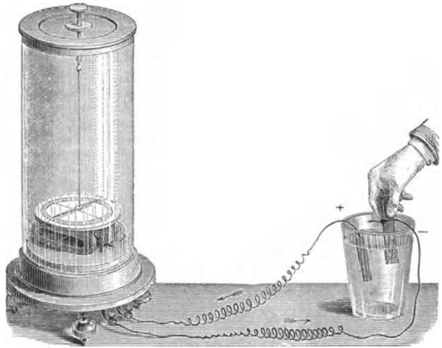
Fig. 388. Schweigger's Multiplikator.
