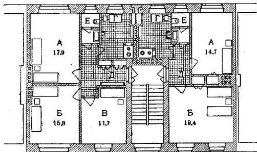
Рис. 2. План средней секции блочного 4-этажного кирпичного дома. 2 квартиры в этаже в 2 и 3 комнаты с жилой площадью в 34,1 м 2 и 45,4 м 2 (из альбома ЦКВанка). А, Б и В—жилые комнаты; Г—кухня; Е—уборная; Д—передняя.
