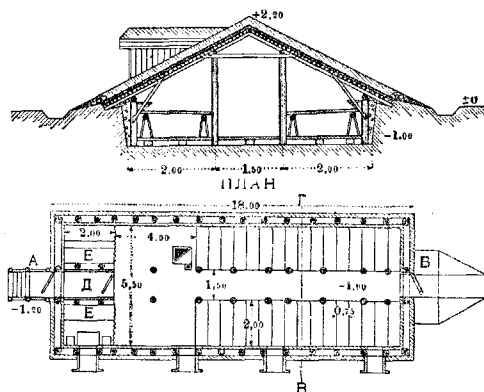
Рис. 2. Зимняя двускатная З. вместимостью на 32 чел.: А — вход; Б — запасный выход; Д — внутренний тамбур; Е — места для коммодов (отторженные занавеской).
