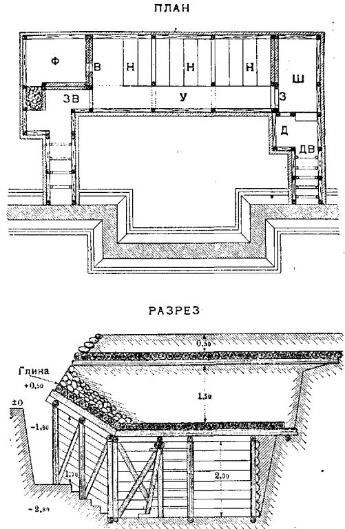
Рис. 4. Котлованное убежище: ДВ—вход действующий; ЗВ—вход запасный; У—убежище; Н—нары; Д—камеры предварительной дегазации; Ш—шлюз; З—занавесы; В—место вентилятора; Ф—земляной фильтр.
