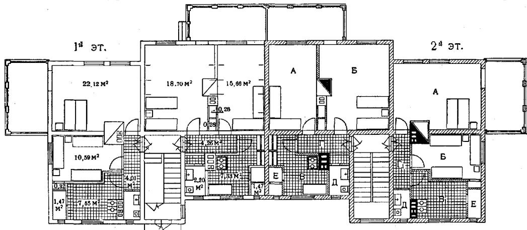
Рис. 3. План отдельного деревянного 2-этажного жилого дома в поселке. 8 квартир по 2 комнаты с жилой площадью в 32,7—34,4 м 2 при ориентации жилой площади на юг (из альбома ЦКВанка). А и Б—жилые комнаты; В—кухня; Г—передняя; Д—уборная; Е—кладовая.
