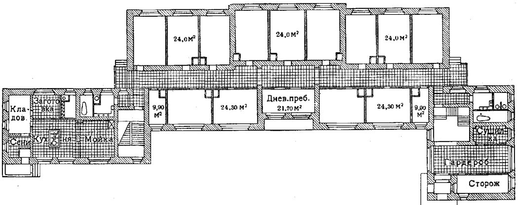
Рис. 4. План кирпичного 3-этажного общежития на 120 человек. Средняя часть (жилые комнаты)—с большей высотой, боковые части (службы)—ниже (из альбома ЦКБанка).
