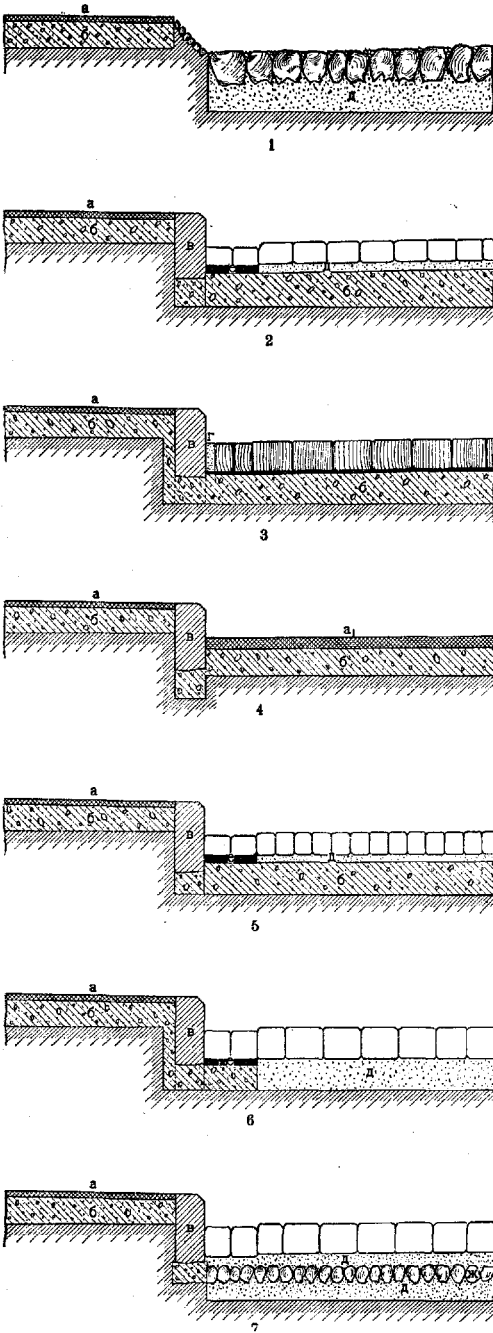
Типы мостовых покрытий. 1. Поперечный профиль бульжной мостовой. 2. Поперечный профиль мостовой «брюкештейн» с заполнением швов цементом. 3. Поперечный профиль торцовой мостовой с заполнением швов цементом. 4. Поперечный профиль асфальтовой мостовой. 5. Поперечный профиль мостовой «клейнпфистер» с заполнением швов песком. 6 и 7. Поперечный профиль брусчатой мостовой на песчаном основании и на бульжном основании. а—тротуар асфальтовый; б—бетонное основание тротуара; в—бортовой камень; г—песчаный шов; д—песчаное основание мостовой; е—цементная подушка; жс—бульжное основание под мостовой.
