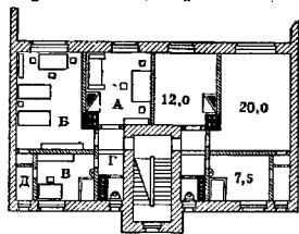
Рис. 1. План средней секции 2-этажного кирпичного дома. 2 квартиры в этаже по 2 комнаты с жилой площадью в 32 м 2 (тип Укр. техн. стр. к-та). А и Б—жилые комнаты; В—кухня; Г—уборная; Д—кладовая.
