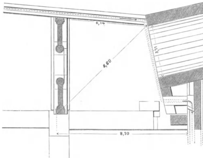
Grundriss des Stadioneingangs. Fig. 86.
