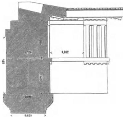
Metroon: Gebälk. Fig. 90.
