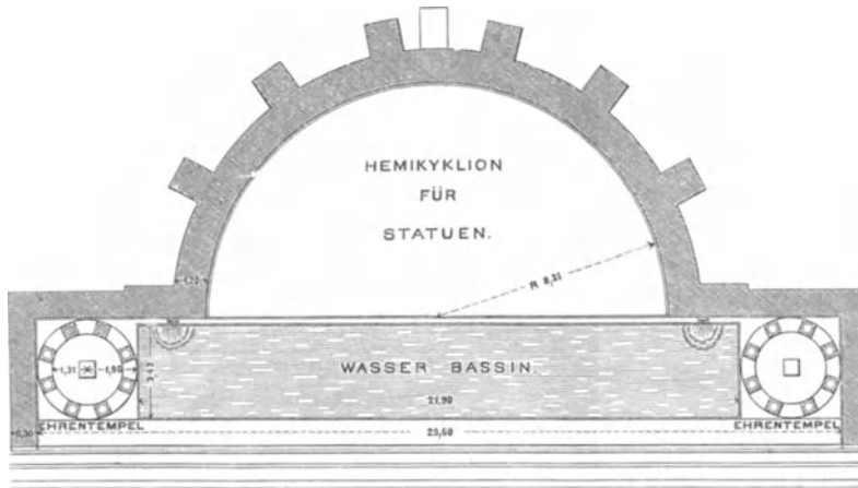
Exedra des Herodes Atticus. Fig. 94.
