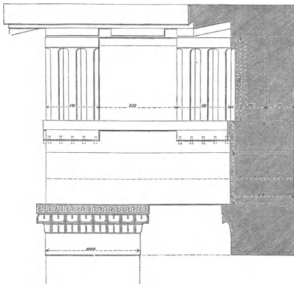
Ante und Gebälk des Buleuterions. (Nordbau.)
