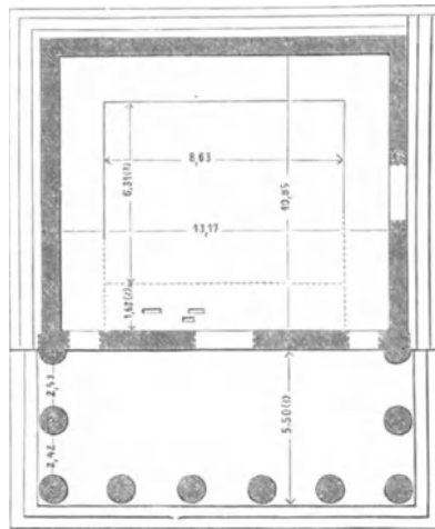
Schatzhaus von Gela.
