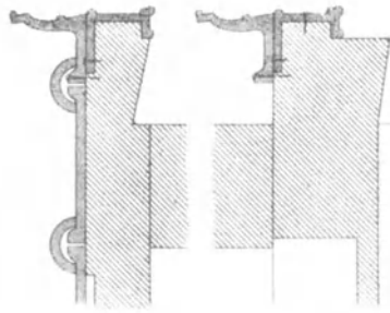
II. SCHNITT DURCH DEN GIEBEL.
