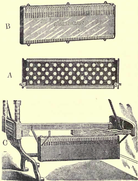
FIG. 29.—CAR-HEATER.
