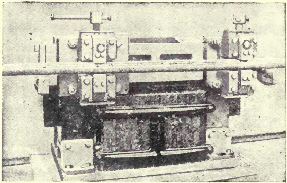
FIG. 73.—PIPE-BENDING APPARATUS.
