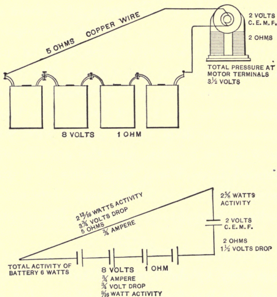
FIG. 2.—DISTRIBUTION OF C. E. M. F. IN A CIRCUIT.
