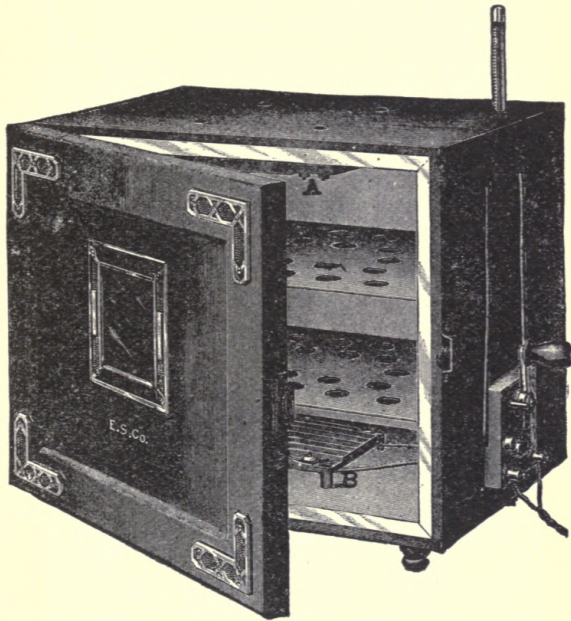
FIG. 41.—ELECTRIC OVEN.
