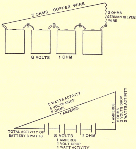
FIG. 1. —DISTRIBUTION OF C. E. M. F. IN A CIRCUIT.
