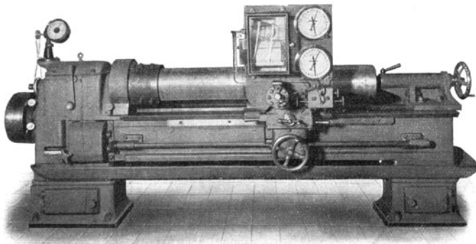
Abb. 16. Prüfrehbank für Drehstähle.
