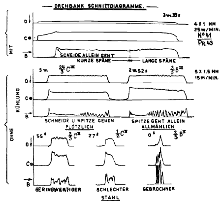
Abb. 14. Schnittdruckschaubilder der Abstumpfungsversuche.
