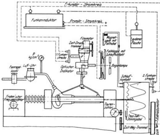
Abb. 22. Schema des Prüfstandes.
