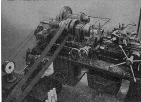
Abb. 41. Normale Revolverbank von L. Loewe & Co., Berlin eingestellt für Leichtmetallversuche.
