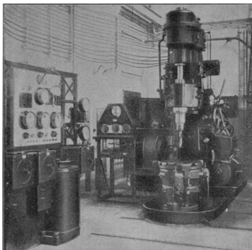
Abb. 9. Große Versuchsbohrmaschine mit der zweiten Ausführung des Meßtisches.
