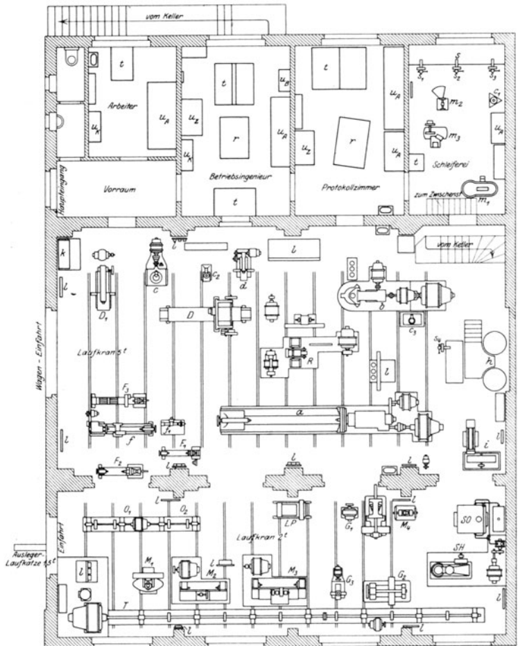
Abb. 2. Grundriß des Versuchsfeldes für Werkzeugmaschinen (ebenerdig).
