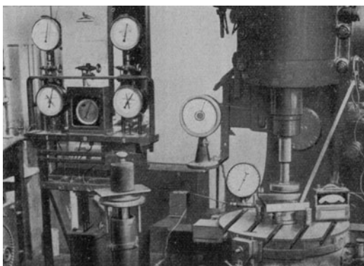
Abb. 11. Reibungsversuche mit Kammlagerplatten-Material auf der Versuchsbohrmaschine Nr. 7.
