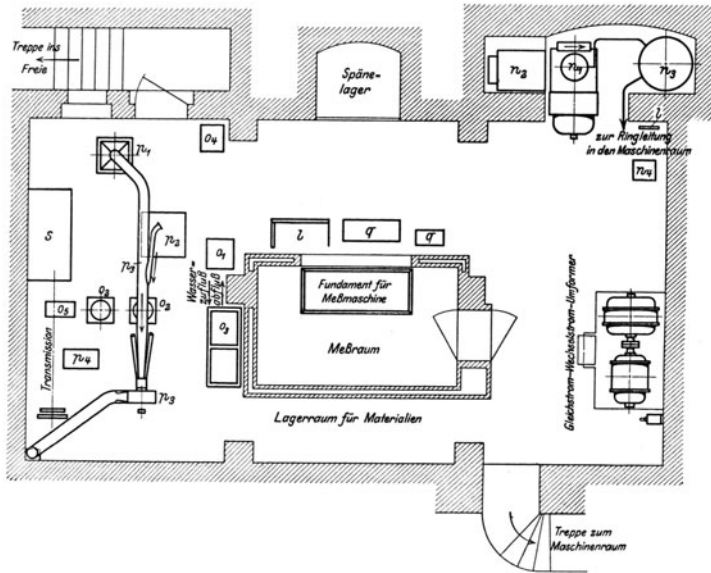
Abb. 3. Versuchsfeld für Werkzeugmaschinen. Grundriß des Kellers.
