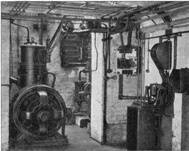
Abb. 4. Kompressoranlage.
