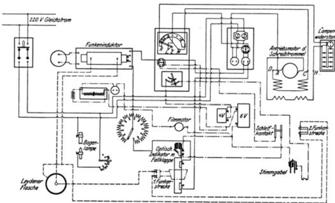
Abb. 23. Elektrische Schaltung des Prüfstandes für Preßluftwerkzeuge.
