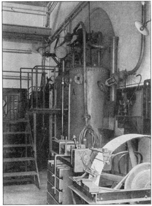
Abb. 6. Meßeinrichtung zur Untersuchung von Preßluftwerkzeugen.
