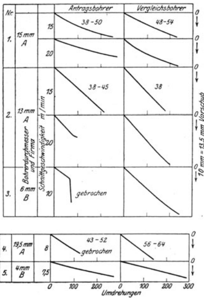
Abb. 32. Keep-Kurven für Spiralbohrerprüfung.
