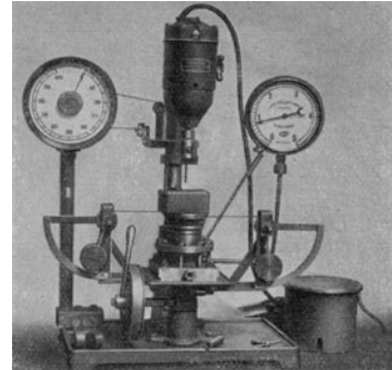
Abb. 17. Versuchsbohrmaschine für Bohrer bis 8 mm \varnothing mit Druck- und Drehmomentsmessung.
