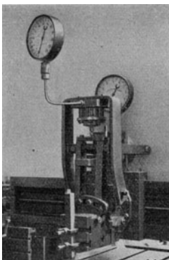
Abb. 20. Zwei-Komponenten-Meß-Support für die Tischhobelmaschine.
