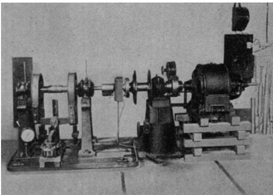
Abb. 24. Öl- und Lagerprüfstand, Bauart Kurrein.
