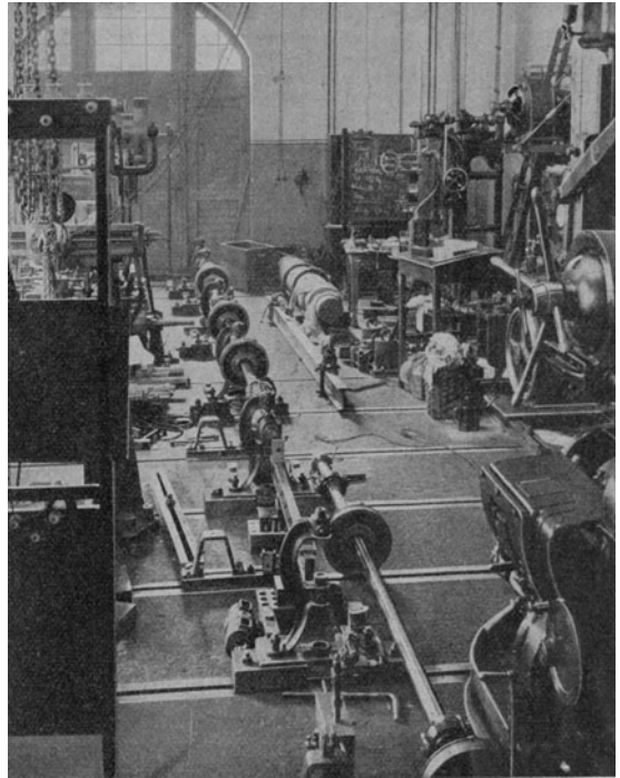
Abb. 25. Versuchstransmission (I. Aufbau).
