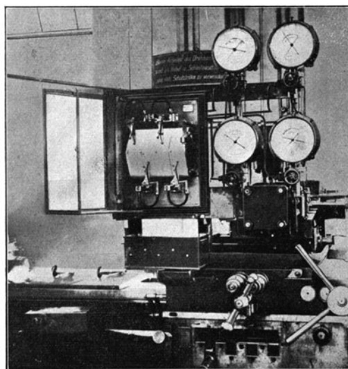
Abb. 12. Meß-Support der Versuchs-drehbank mit Vierfachsreiber.
