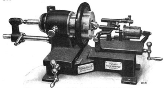
Abb. 19. Spiralbohrer-Meßapparat (Bauart R. Stock & Co.).
