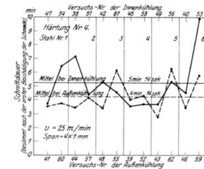
Abb. 30. Einfluß der Innenkühlung an Drehstählen.
