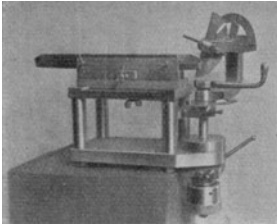
Abb. 15. Drehstahlmeßapparat.
