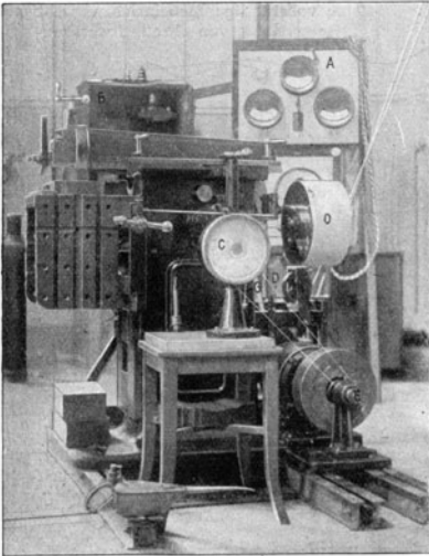
Abb. 7. Wagrecht-Stoßmaschine.
