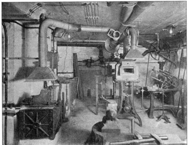
Abb. 8. Härterei.
