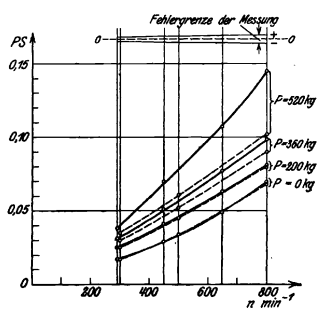
Abb. 45. Gegenüberstellung von berechneten und beobachteten Reibungswerten an der Versuchstransmission.
