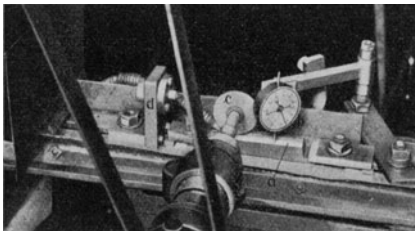
Abb. 29. Prüfung von Schleifscheiben.
