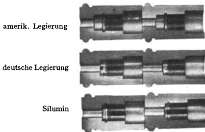
Abb. 42a. Werkstück im Schnitt.
