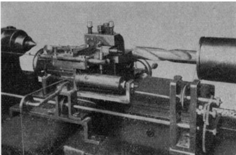
Abb. 18. Spiralbohrer-Meßapparat (1. Ausführung).
