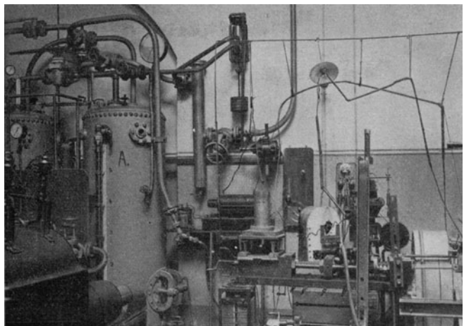
Abb. 21. Ansicht des Prüfstandes für Preßluftwerkzeuge.
