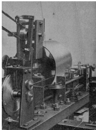
Abb. 10. Selbsttätiger Schreibapparat für die Zeit-Weg-Schaubilder, Umsteuerpunkte und Riemenleitung.
