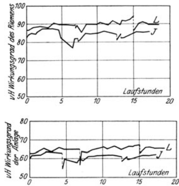
Abb. 43—44. Wirkungsgrad des Jaguriemens.
