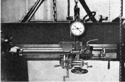
Abb. 38. Messung des Abstumpfungskriteriums an der Mechanikerdrehbank.
