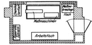
Abb. 4. Feinmeßraum im Keller.
