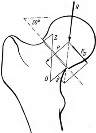
Abb. 115. Mechanische Analyse einer Fraktur 2. Grades. Wirksam auf das Knochenregenerat ist die freie Scherkraft K_S . Die Druckkomponente P hat keine Wirkung auf das Regenerat, sie ruft jedoch in einem Teil der Bruchfläche latente Druckspannung hervor. (Schema nach PAUWELS.)
