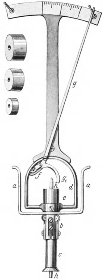
Abb. 222. Druckmesser nach SCHIÖTZ.
