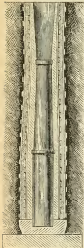
MOULE D'UN CANON. — Ce moule se trouve placé sous terre. On verse dedans le métal fondu; ensuite, quand le métal est refroidi, on brise le moule; le métal a pris la forme d'un canon.
