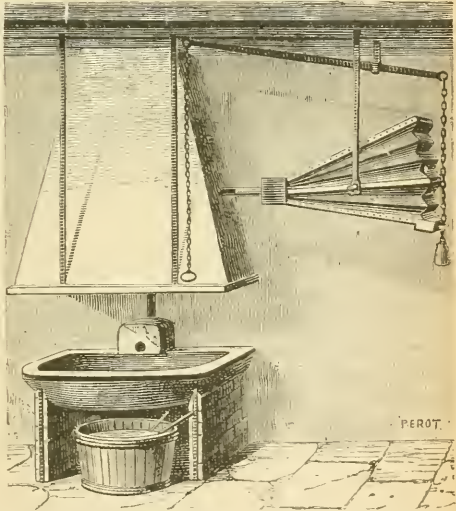
FORGE DE SERRURIER — On voit derrière l'âtre un petit trou noir : c'est par ce trou qu'arrive le vent du soufflet, qui sert à exciter le feu de charbon de terre. Au-dessous du foyer se trouve un baquet rempli d'eau ; on s'en sert pour mouiller le charbon.
