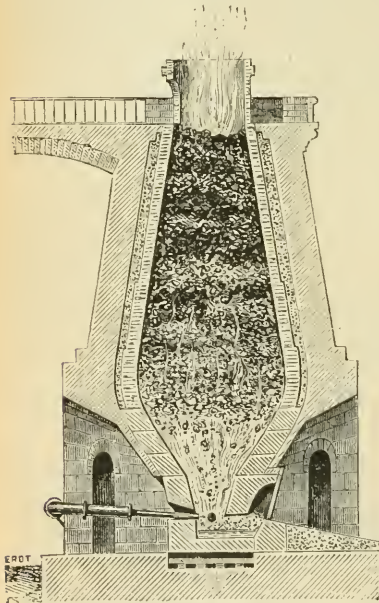
UN HAUT FOURNEAU. — Les hauts fourneaux sont des espèces de tours solides qu'on remplit par en haut de minerai de fer. Une fois que le haut fourneau est allumé, on le remplit jour et nuit sans interruption pour avoir la plus grande chaleur possible, jusqu'à ce que les murs usés se fendent et éclatent. A mesure que le fer se fond, il tombe en dessous, dans un réservoir.
