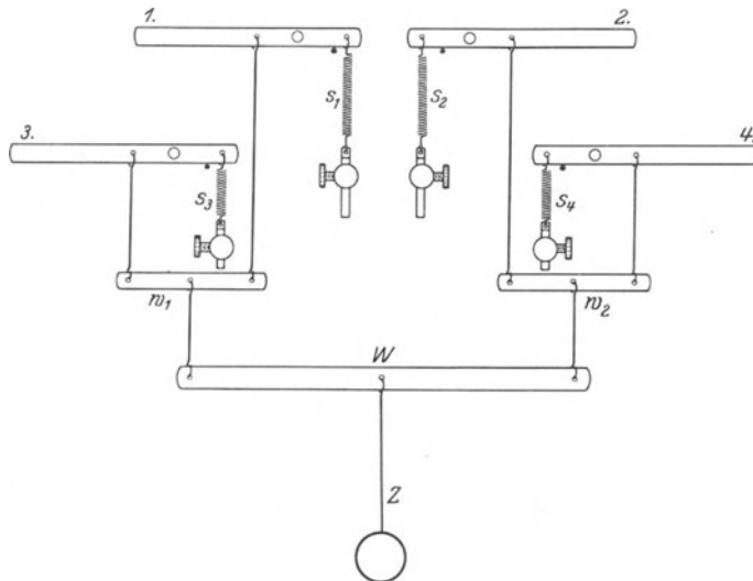
Abb. 384. Modell zur Demonstration einer gleitenden Kopplung.
