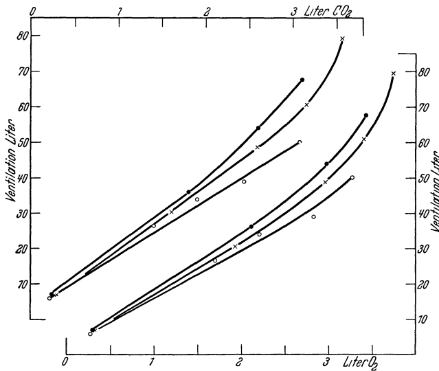
Abb. 306. Abhängigkeit der Ventilation von der \text{CO}_2 -Ausscheidung (oben) und der \text{O}_2 -Aufnahme (unten). (Nach HOHWÜ CHRISTENSEN.)
