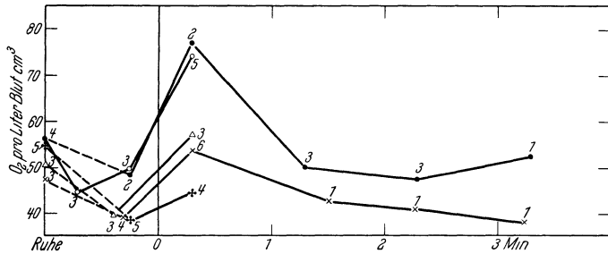
Abb. 316. Sauerstoffaufnahme pro Liter Blut während und nach statischer Arbeit. Absz.: Zeit in Minuten nach dem Aufhören der Arbeit. Die Ziffern an den Kurven geben die Zahl der Einzelbestimmungen an. (Nach LINDHARD.)
