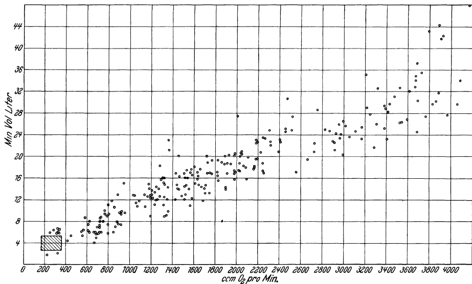
Abb. 314. Minutenvolumen im Verhältnis zum Sauerstoffverbrauch. Bestimmungen in der Ruhe und während des Radfahrens mittels der Stückoxydul- und der Acetylenmethode 3 . Das gestrichelte Gebiet umfaßt im ganzen 52 Ruhewerte.
