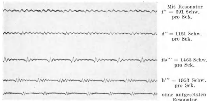
Abb. 460. Lufttraumsvingungen nach Aufsetzen von Resonatoren auf eine Pfeife mit aufschlagender Zunge. Grundton d mit 145 Schwingungen pro Sekunde. (Aus LULLIES: Pflügers Arch. 211.)
