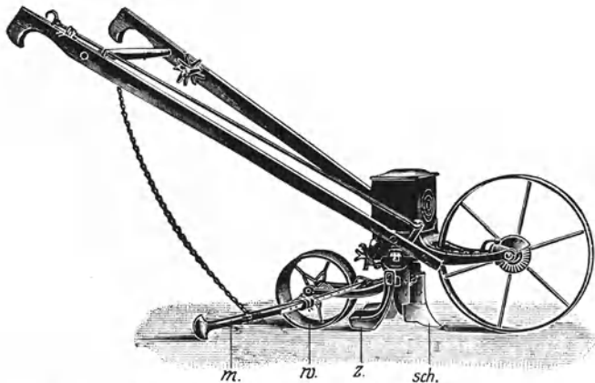
Abb. 187. Sämaschine Planet oder Senior. sch = Scharnase zum Furchenziehen; z = Starre Zustreicher zum Bedecken; w = Walze; m = Markierstange.
