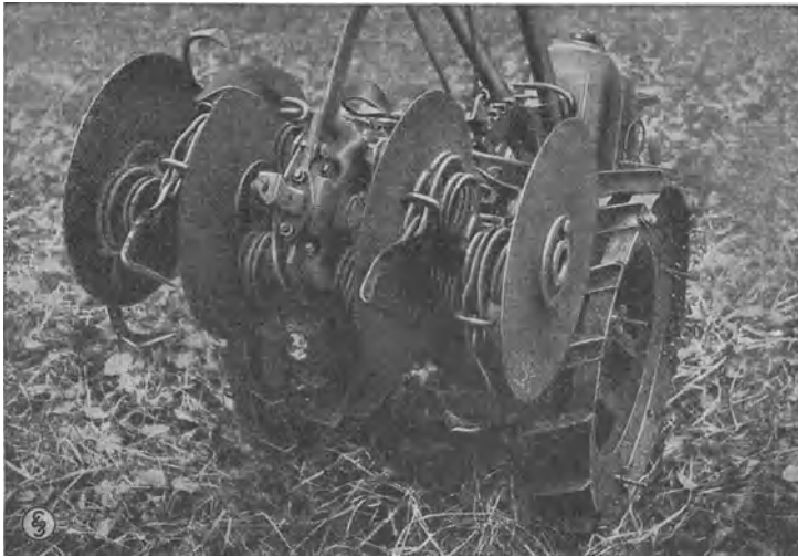
Abb. 175. Siemens-Fräse mit Schälhaken und Waldscheiben. (Aus der Sammlung des Iffa, Eberswalde.)
