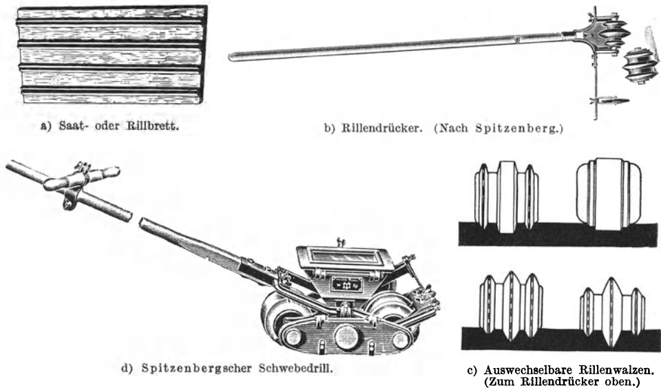
Abb. 203 a—d. Geräte zur Kamparbeit.
