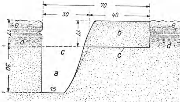
Abb. 165. Profil des Neuruppiner Hochstreifens nach der Herstellung. (Nach dem Setzen oder Anwalzen des aufgehöhten Bodens liegt dieser etwas tiefer.) a Ausgeworfener Graben; b aufgehöhter, lockerer Boden; c Waldpflugssole; d Bodendecke; e umgeklappte Plaggen.
