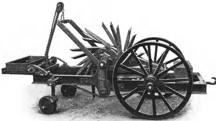
Abb. 170. Geistscher Wühlgrubber „Keller“.
