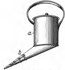
Abb. 186. Sähorn aus Blech. a = Saatgefäß. b = Auslauf mit verschieden weiten, abnehmbaren Auslaufmündungen.
