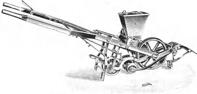
Abb. 188. Nagelsche Präzisionssämaschine (verbesserte Titze-Drewitzsche).
