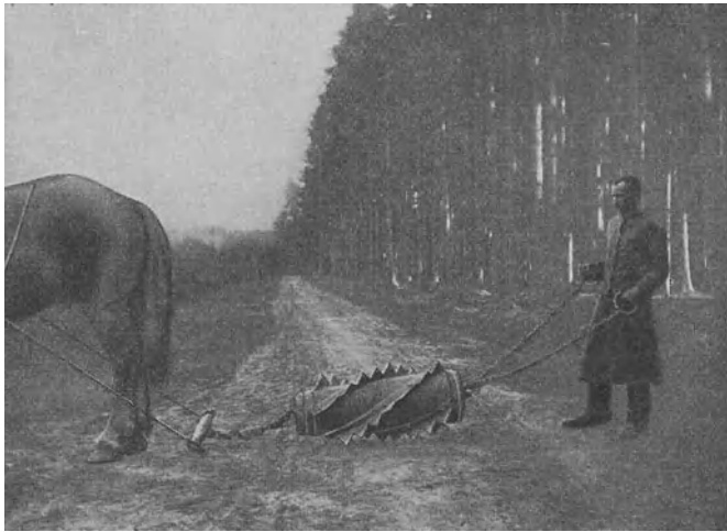
Abb. 177. Der Lindwurm von Forstmeister Auerochs. Hersteller: Erich Krieger (vorm. Epple & Buxbaum), Nürnberg.
