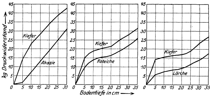
Abb. 80. Die Bodenlockerheit unter Akazie, Roteiche und Lärche im Vergleich zur Kiefer. Gemessen am Druckwiderstand bis zu 30–35 cm Tiefe mit der Meyenburgschen Bodensonde. (Nach Albert und Penschuck.)
