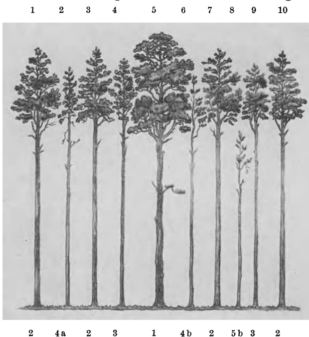
Abb. 214. Die Kraftschen Stammklassen. (Nach Kraft, etwas abgeändert.) (Die Zahlen unter den Stämmen geben die entsprechende Stammklasse an.)
