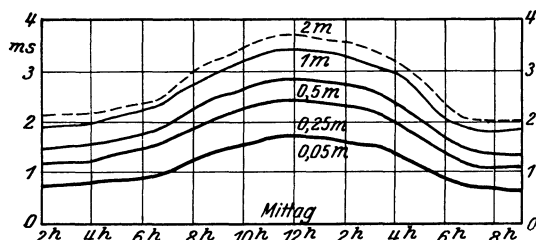
Abb. 67. Täglicher Gang der Windgeschwindigkeit in verschiedenen Höhen (0,05—2 m) über dem Boden. (Nach Geiger.)
