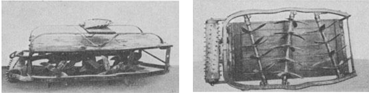
Abb. 169. Finnische Rollegge mit Stubbenkletterwalze. (Aus der Sammlung des Iffa, Eberswalde.)
