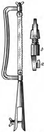
Abb. 227. Aler'sche Flügelsäge zur Aufästung von Waldbäumen.
