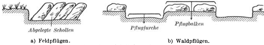
Abb. 160a und b. Arbeit des Feld- und Waldpfluges.
