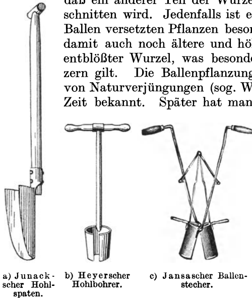
Abb. 202 a—c. Geräte zur Ballenpflanzung.
