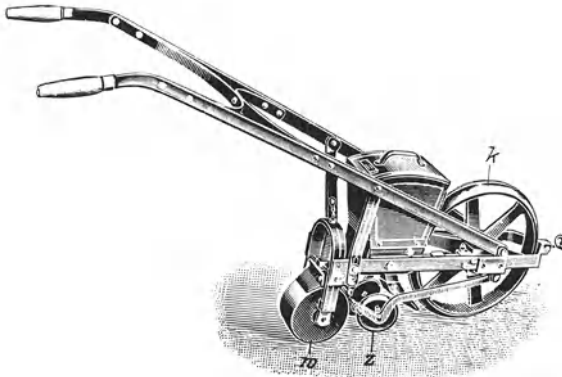
Abb. 189. Sämaschine Walddank der Firma Nagel-Forstgeräte, Eberswalde (vorm. E. E. Neumann). k = Kammer zum Eindringen der Saatrille; z = bewegliche Zustrreicher; w = Druckwalze. z u. w leicht abnehmbar zum Säen in offener Rille zwecks Nachprüfung der richtigen Tiefenlage und gleichmäßigen Verteilung des Samens.
