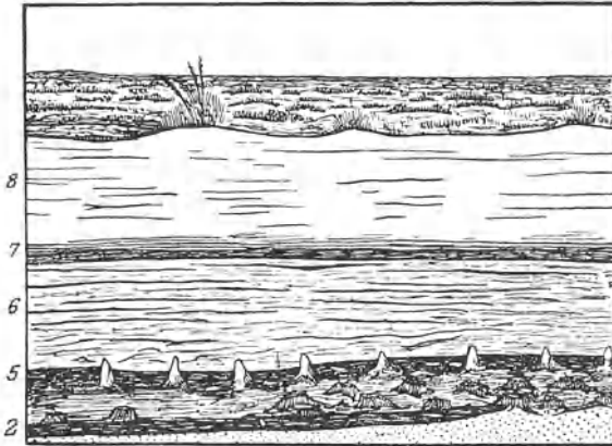
Abb. 35. Aufbau eines typischen norddeutschen Moores. (Nach C. A. Weber, Bremen.) 1. Diluvialsand. 2. Schilftorf (verlandende Wasserfläche). 3. Auenwaldtorf (feuchter Waldboden). 4. Föhrenwaldtorf mit Stubbenresten (fortgeschrittene Hochmoorbildung). 5. Scheuchzeriatorf (neue Vernässung, in der der Kiefernbestand abstirbt). 6. Älterer Sphagnumtorf, stark zersetzt und zusammengeleget. 7. Grenzhorizont; Stillstandsphase der Torfbildung (Trockenzeit?), Eriophorum- und Heidereste. 8. Jüngerer Sphagnumtorf (neues Anwachsen der Moore, lockerer, wenig zersetzter Moostorf). An der Oberfläche Moosrasen mit Bünten.
