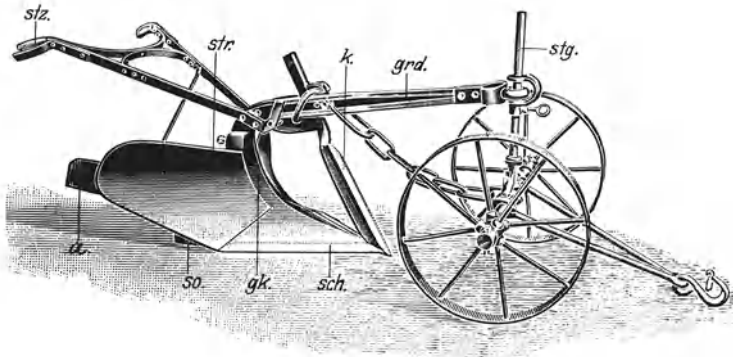
Abb. 159. Choriner Wald- oder Forstkulturpflug CFM in Arbeitsstellung (Hersteller: E. E. Neumann, Eberswalde).
