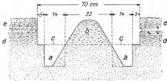
Abb. 167. Profil des Zehdenicker Hochstreifens nach der Herstellung. (Nach dem Setzen des Dammes ist dieser etwas niedriger und breiter.) a Ausgeworfener Graben; b aufgehöhter lockerer Boden; c Waldpflugschle; d Bodendecke; e umgeklappte Plaggen.
