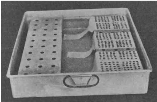
Abb. 179. Haackscher Keimkasten, rechts mit eingelegten Keimproben (zum Gebrauch noch mit einer Glasscheibe zu bedecken). Hersteller: Klempnerei A. Marwitz, Eberswalde.
