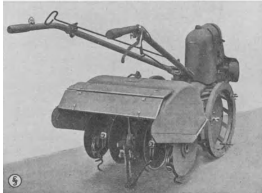
Abb. 173. Siemens-Kleinfräse KV (5 PS) für Forstwirtschaft mit Tiefenlockerungshaken (Gesamtansicht mit Transportradkränzen). Hersteller: Siemens-Schuckert-Werke.
