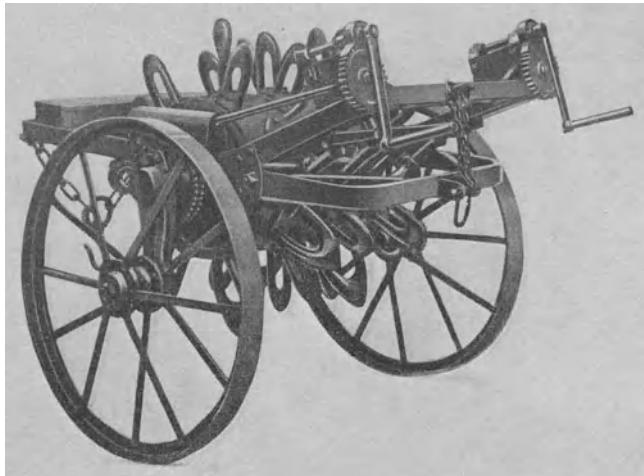
b) Spitzenbergs Wühlrad.
