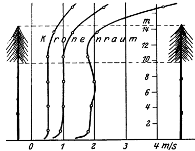
Abb. 68. Vertikale Verteilung der Windstärke im Walde bei verschiedener Windgeschwindigkeit. (Nach Geiger.)
