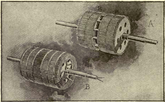
FIG. 77.—MOTOR ARMATURES.
