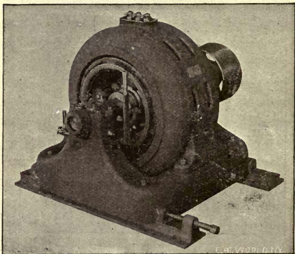
FIG. 73.—MONOCYCLIC MOTOR.
