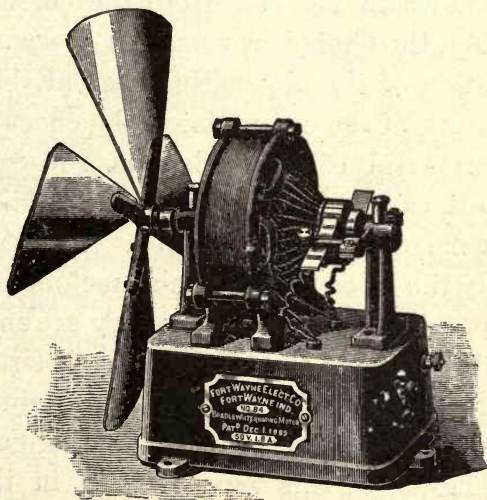
FIG. 57 —ALTERNATING-CURRENT FAN MOTOR.
