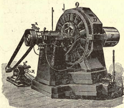
FIG. 22.—2000-LIGHT ALTERNATOR.
