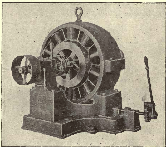
FIG. 23.—1000-LIGHT ALTERNATOR.
