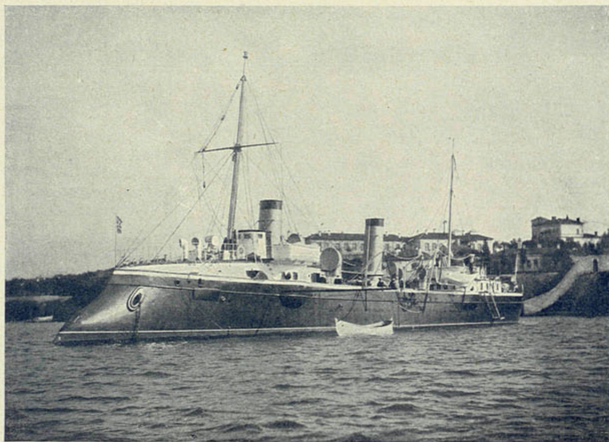
„КАПИТАНЪ САКЕНЪ“, МИННЫЙ КРЕЙСЕРЪ.
