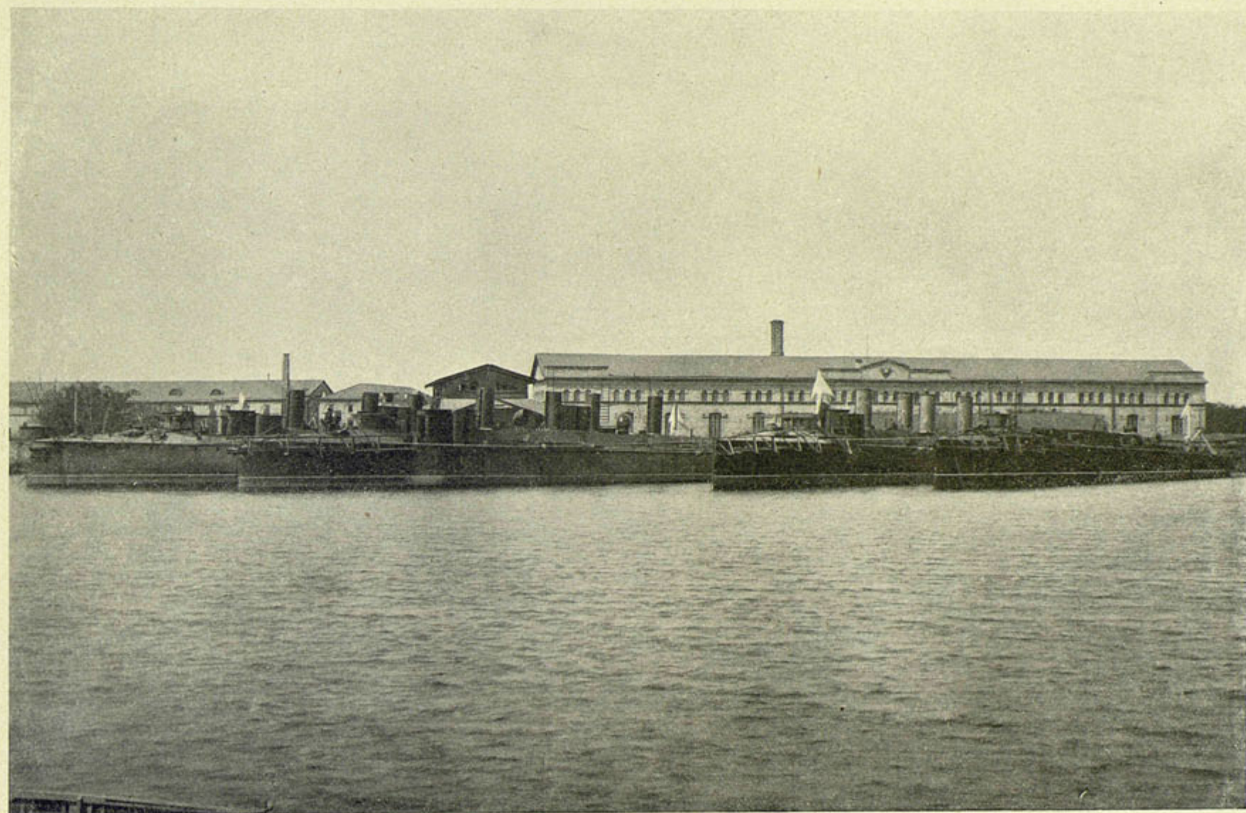
миноносцы „ЖИВОЙ“, „ЖИВУЧИЙ“, „ЖУТКИЙ“, „ЖАРКИЙ“ въ николаевскомъ адмиралтействѣ.
