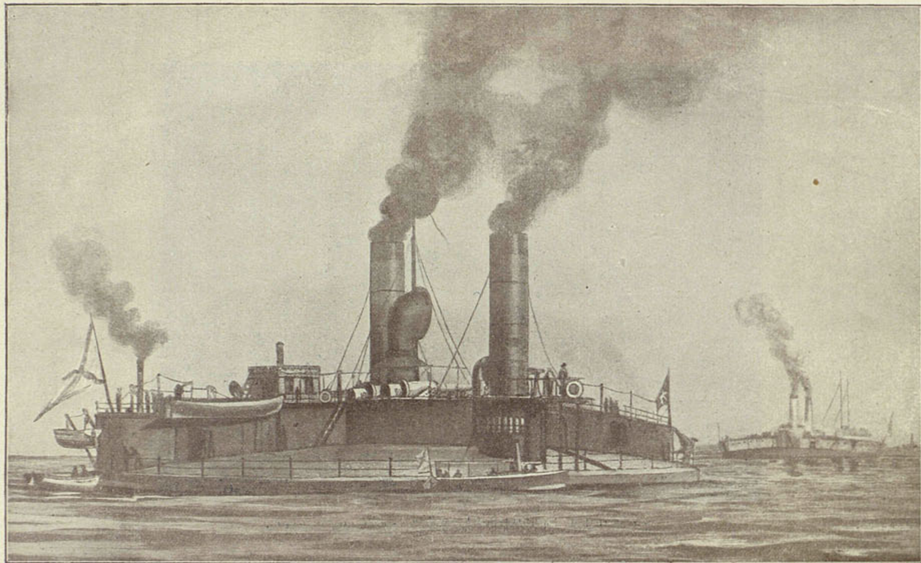
„ВИЦЕ-АДМИРАЛЪ ПОПОВЪ“, ПОПОВКА.
