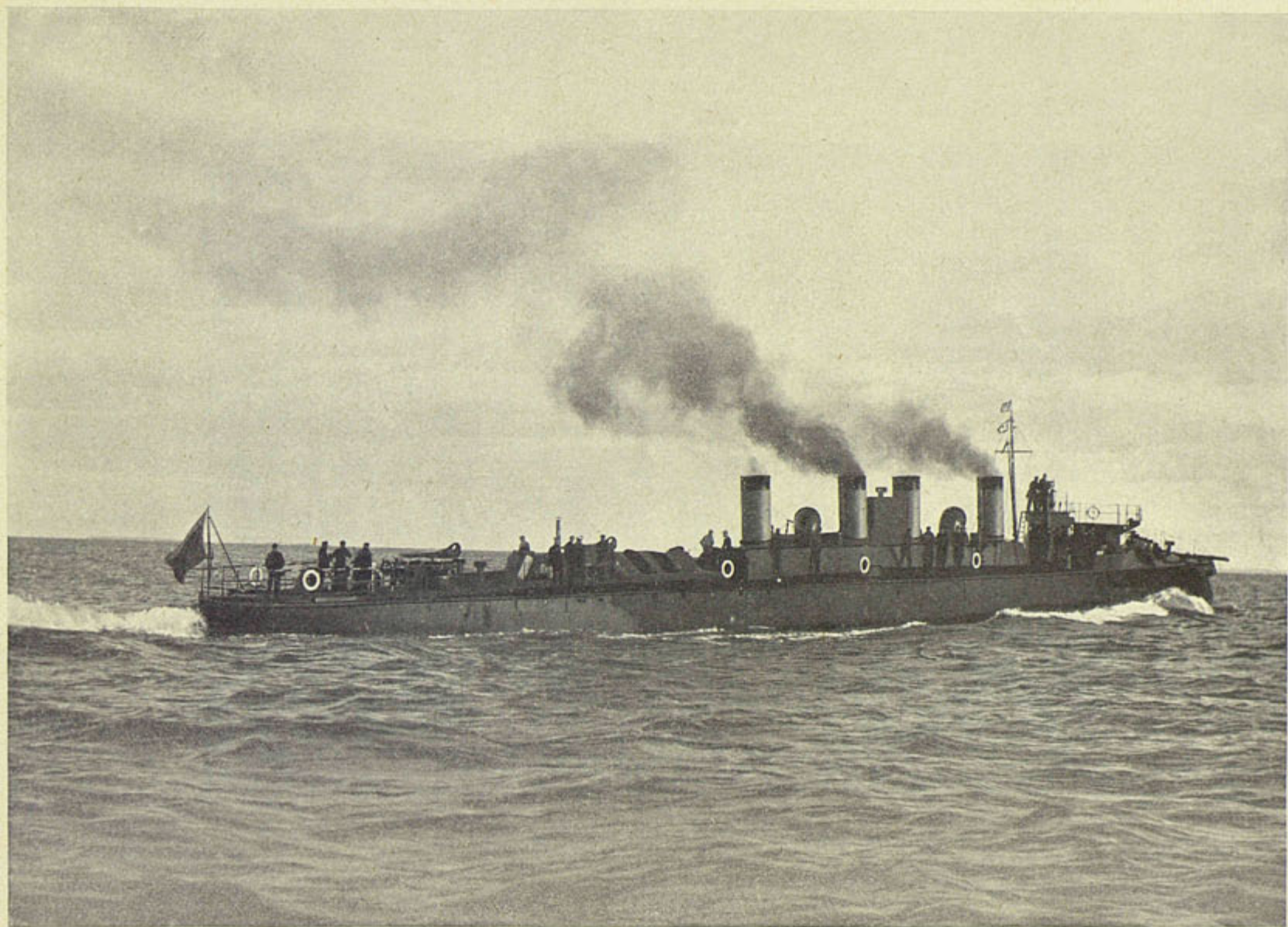
„СТЕРЕГУЩИЙ“, миноносецъ. типа Буинскій
