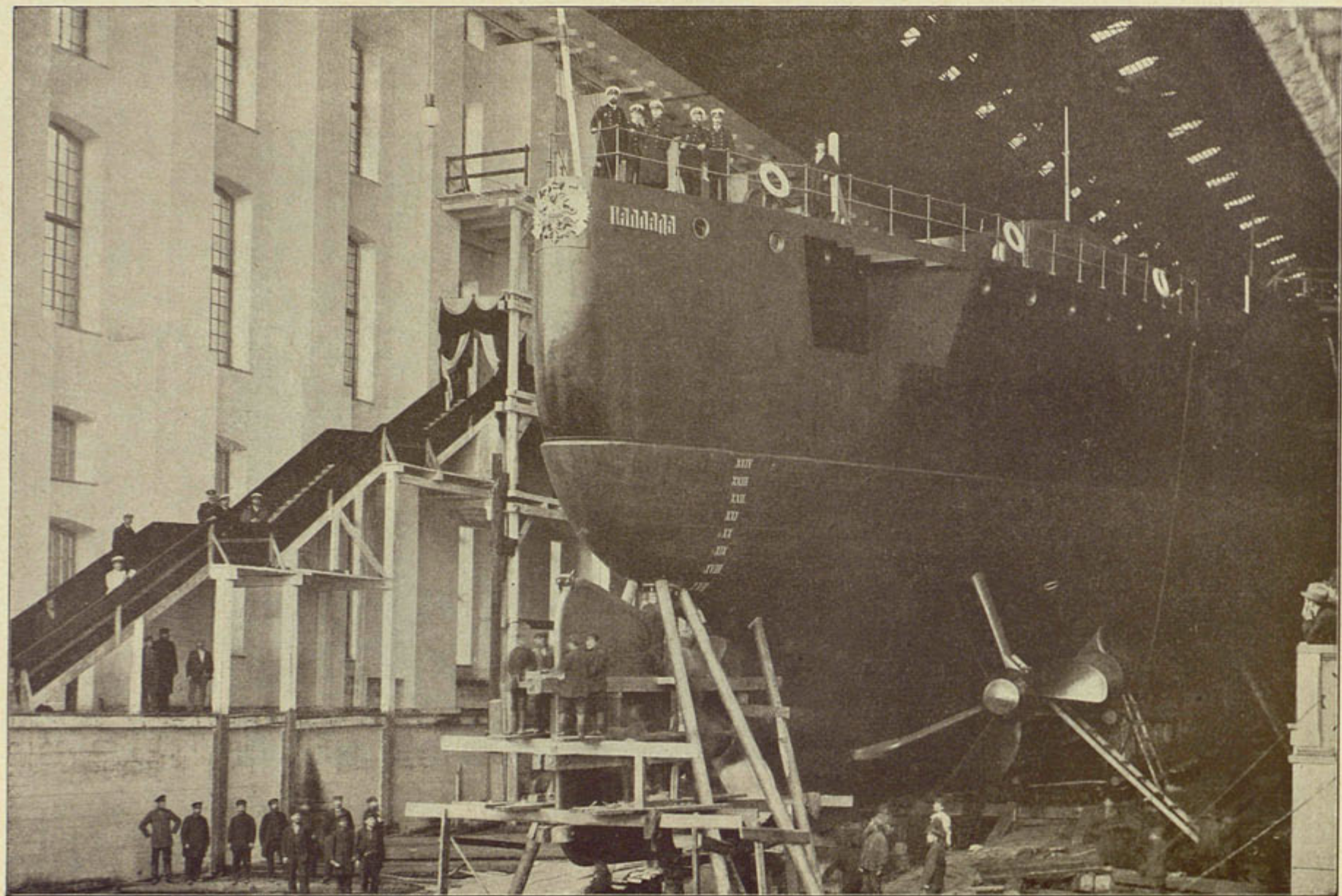
„ПАЛЛАДА“, КРЕЙСЕРЪ 1 РАНГА НАКАНУНЪ СПУСКА ИЗЪ КАМЕННАГО ЭЛИНГЪ НА ГАЛЕРНОМЪ ОСТРОВЪ ВЪ СПБ.
