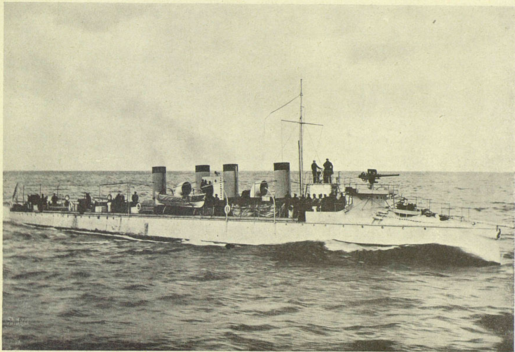
„БУРНЫЙ“, ЭСКАДРЕННЫЙ МИНОНОСЕЦЪ.
