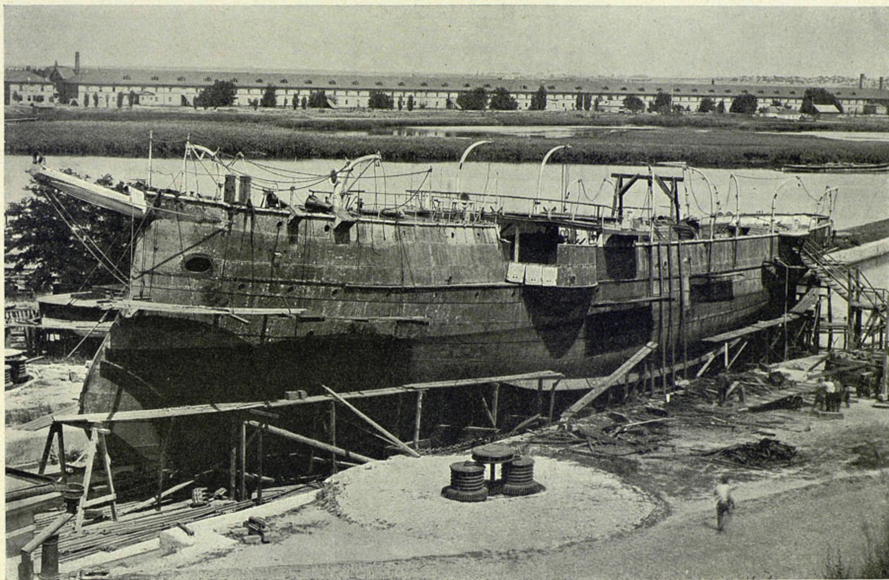
„ДОНЕЦЪ“, КАНОНЕРСКАЯ ЛОДКА ВЪ НИКОЛАЕВСКОМЪ АДМИРАЛТЕЙСТВѢ.
